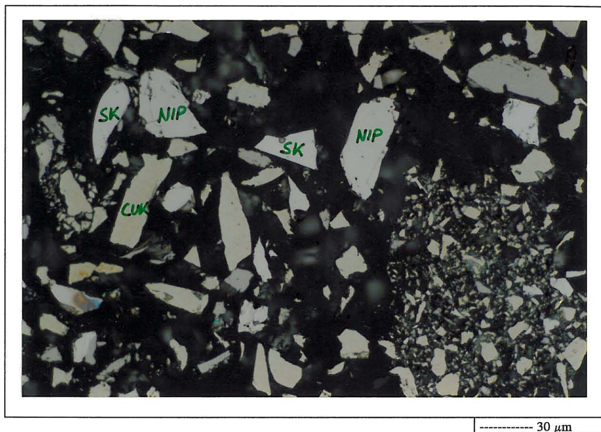
Kuva 1. Kertausrikaste 3/1. CUK=kuparikiisu, NIP=pentlandiitti, SK=pyriitti ja FEK=magneettikiisu.
