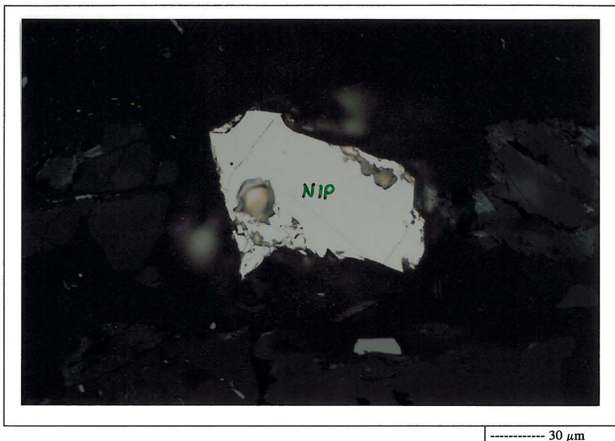
Kuva 1. Pääosa pentlandiitista esiintyy puhtaina partikkeleina jo 20 min jauhatuksen jälkeen (NIP). Kuvassa tyypillinen puhdas 130 μm pentlandiittipartikkeli.
