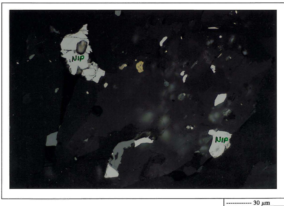
Kuva 2. Pentlandiitti esiintyy myös silikaattien sulkeumina. Kuvassa tyypillisiä pentlandiittisulkeumia (NIP). Kuvassa on myös keltaisia kuparikiisusulkeumia.
