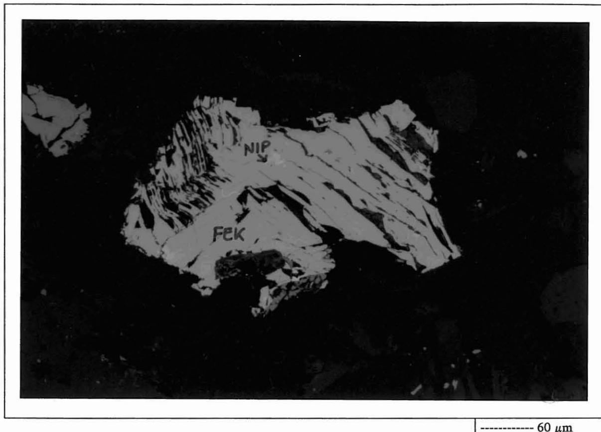
Kuva 5. Näytteessä esiintyy erittäin vähän rautakiisuja. Harvalukuiset magneettikiisupartikkelit ovat yleensä isoja ja niissä on hyvin vähän pentlandiittisuotumia.
