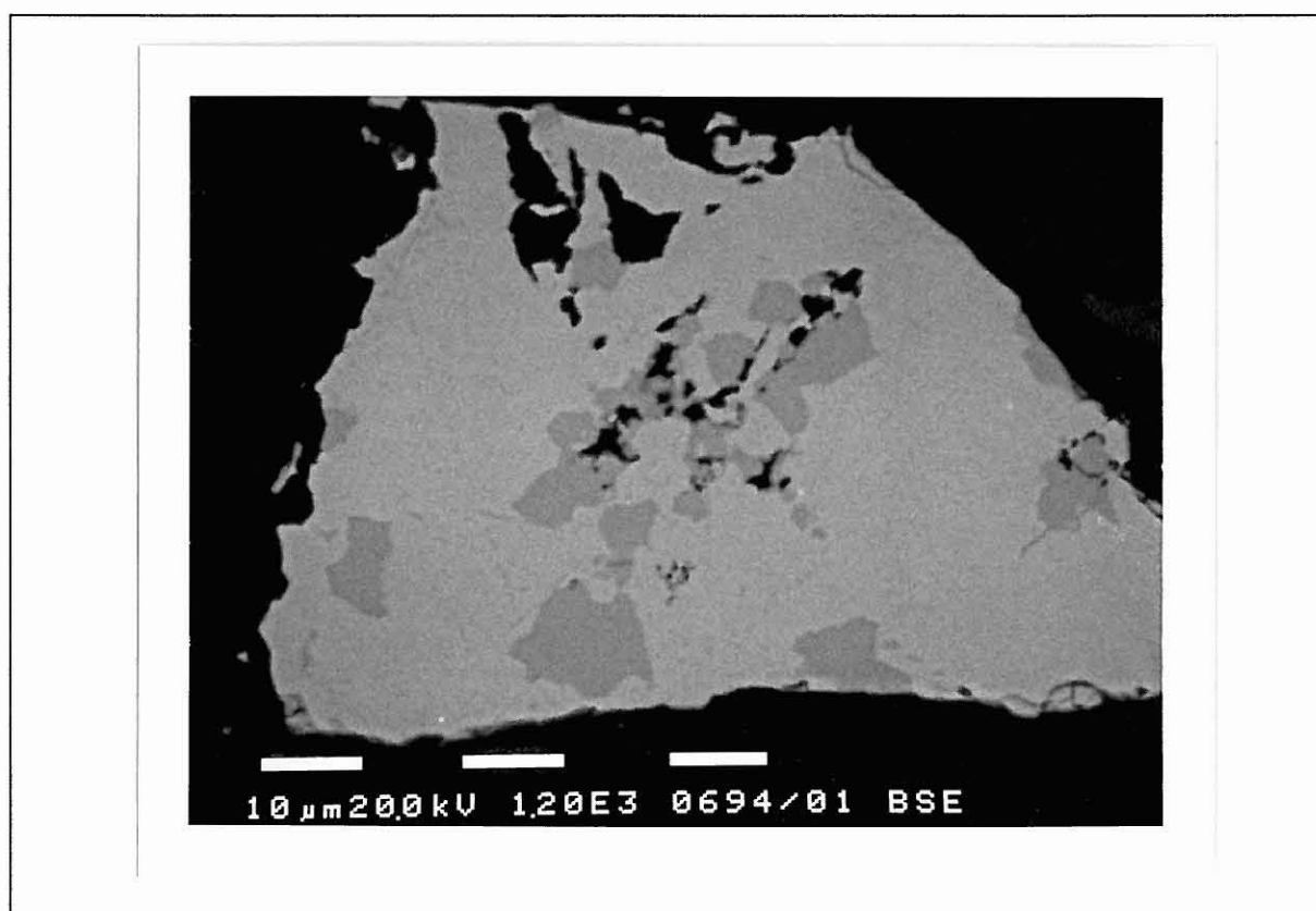
Kuva 4. Backscatter-kuvassa on noin 80 μm heazlewoodiittipartikkeli, jossa on tummempia pentlandiittisulkeumia. Mittajanan pituus on 10 μm.
