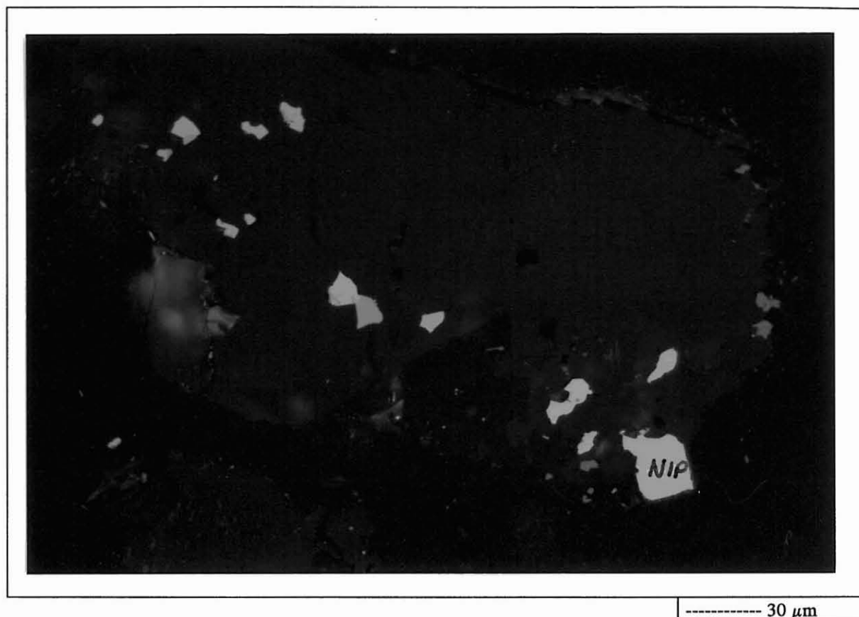
Kuva 3. Pentlandiittisulkeumia (NIP) silikaatissa.
