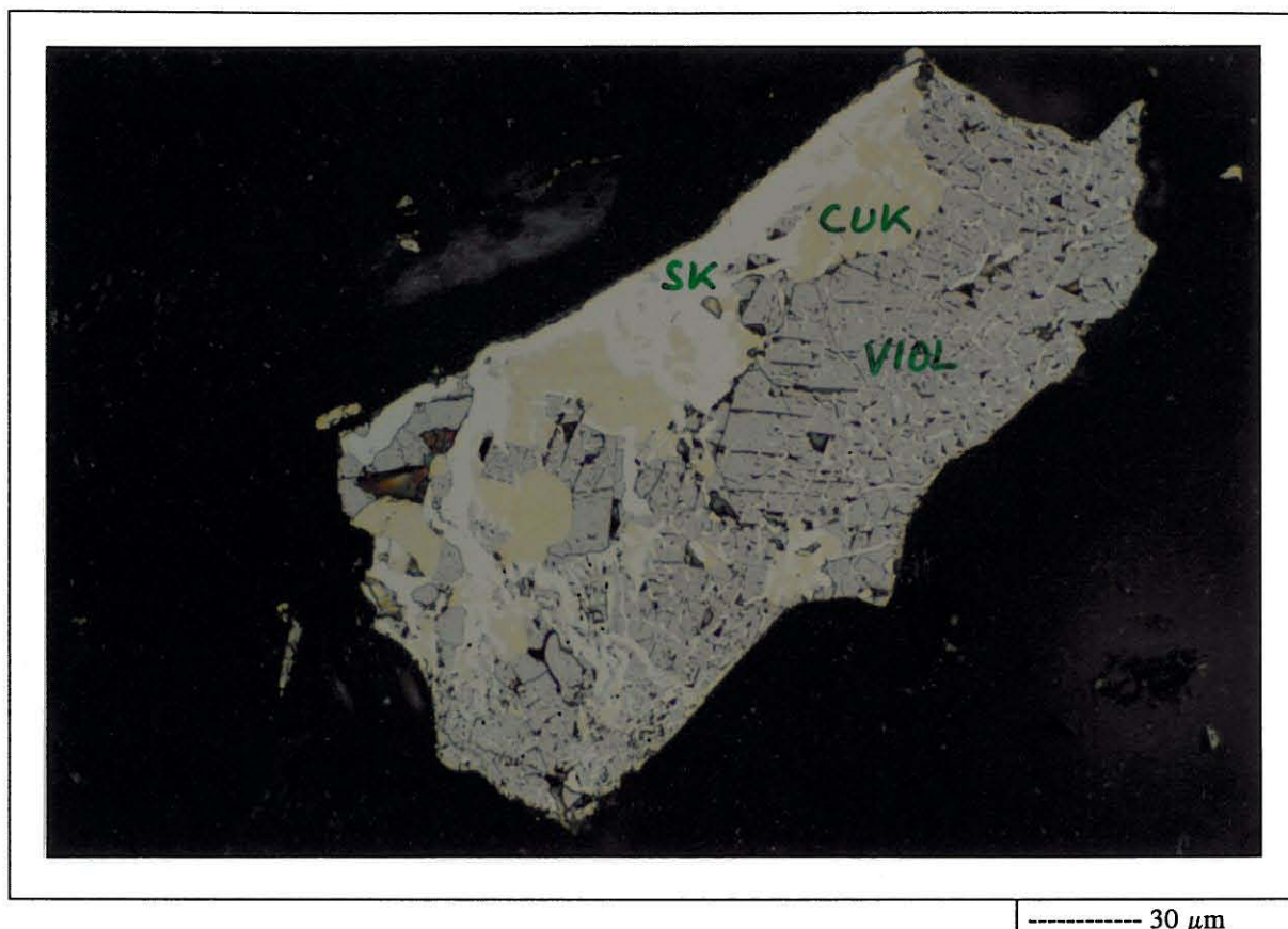
Kuva 5. Kuvassa on violariitti (VIOL)-kuparikiisu-pyriittirae.
