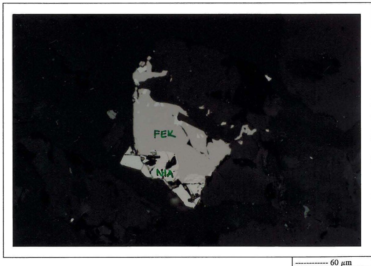
Kuva 2. Kuvassa magneettikiisu-pentlandiitti-silikaattirae, jossa on myös pieniä keltaisia kuparikiisusulkeumia.
