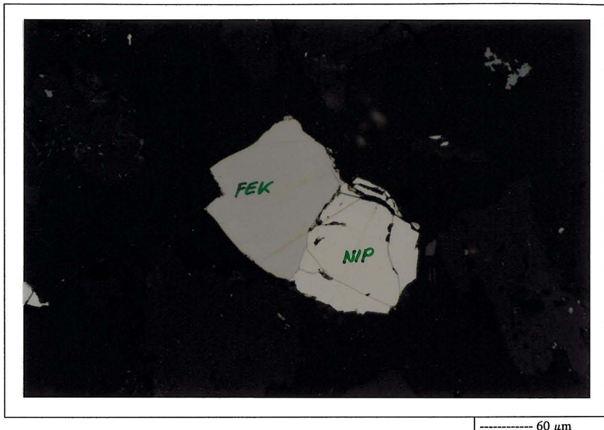
Kuva 1. Pentlandiitti esiintyy näytteessä puhtaina partikkeleina (raekoko alle 125 \mu\text{m} ) ja sekarakeina magneettikiisun, magnetiitin ja silikaattien kanssa. Lisäksi magneettikiisua on silikaattien sulkeumina. Kuvassa on tyypillinen Magneettikiisu (FEK)-pentlandiitirae.
