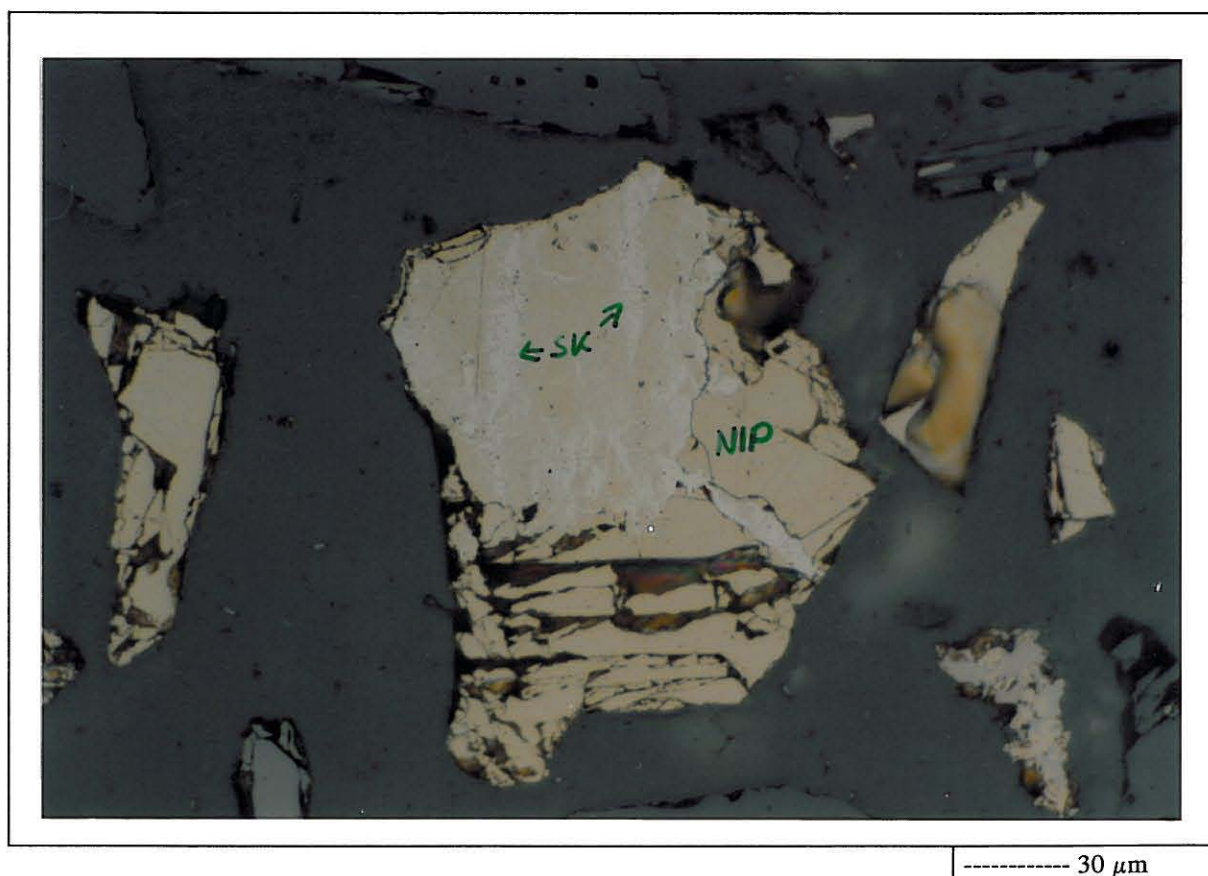
Kuva 8. Osassa pentlandiittirakeissa tavataan pienikiteistä pyriittiyhteenkasvettumaa. SK=pyriitti .
