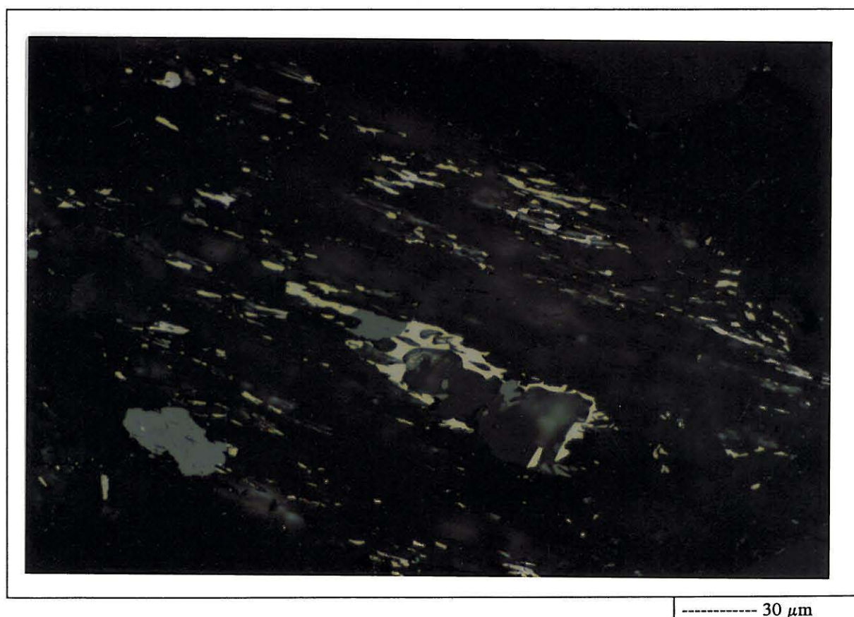
Kuva 10. Kuparikiisusulkeumia silikaatissa.
