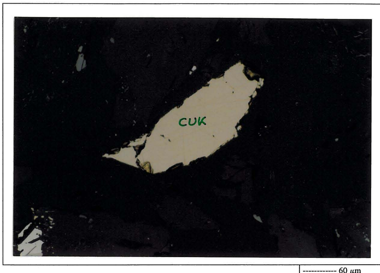
Kuva 9. Kuparikiisu esiintyy näytteessä vapaina partikkeleina, sekarakeina eri mineraalien kanssa ja silikaattien sulkeumina. Kuvassa on iso vapaa kuparikiisupartikkeli (CUK).
