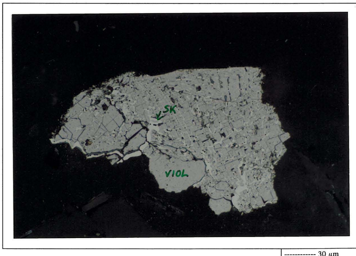
Kuva 6. Kuvassa on näytteelle hyvin tyypillinen violariitti-pyriittisekarae.
