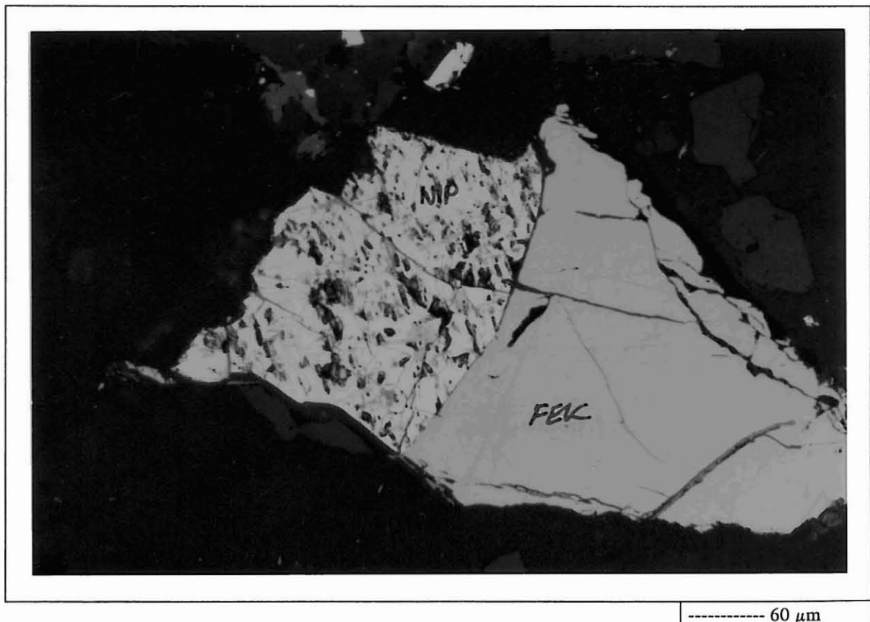
Kuva 2. Pentlandiitti sekarakeena magnetiitin (FEK) kanssa. Pentlandiitissa on havaittavissa heikkoa violariittituumista.
