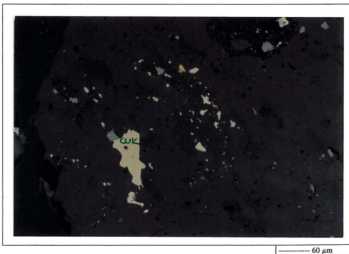
Kuva 8. Kuvassa on kuparikiisusulkeumia silikaatissa. Pienet hapettuneet (tummankehtaiset) kiteet ovat ilmeisesti talnahiittia.
