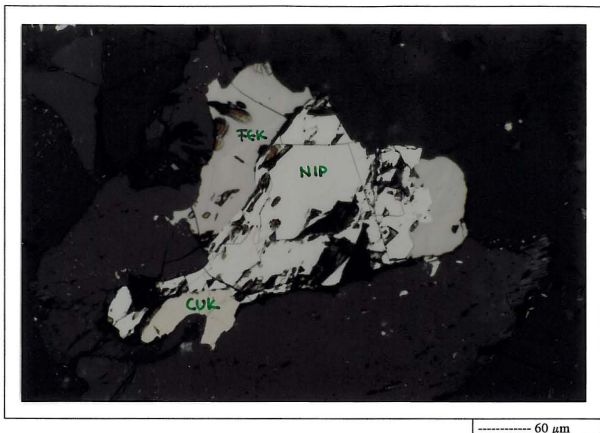
Kuva 3. Pentlandiitti sekarakeena magneettikiisun (FEK), kuparikiisun (CUK) ja silikaatin kanssa.
