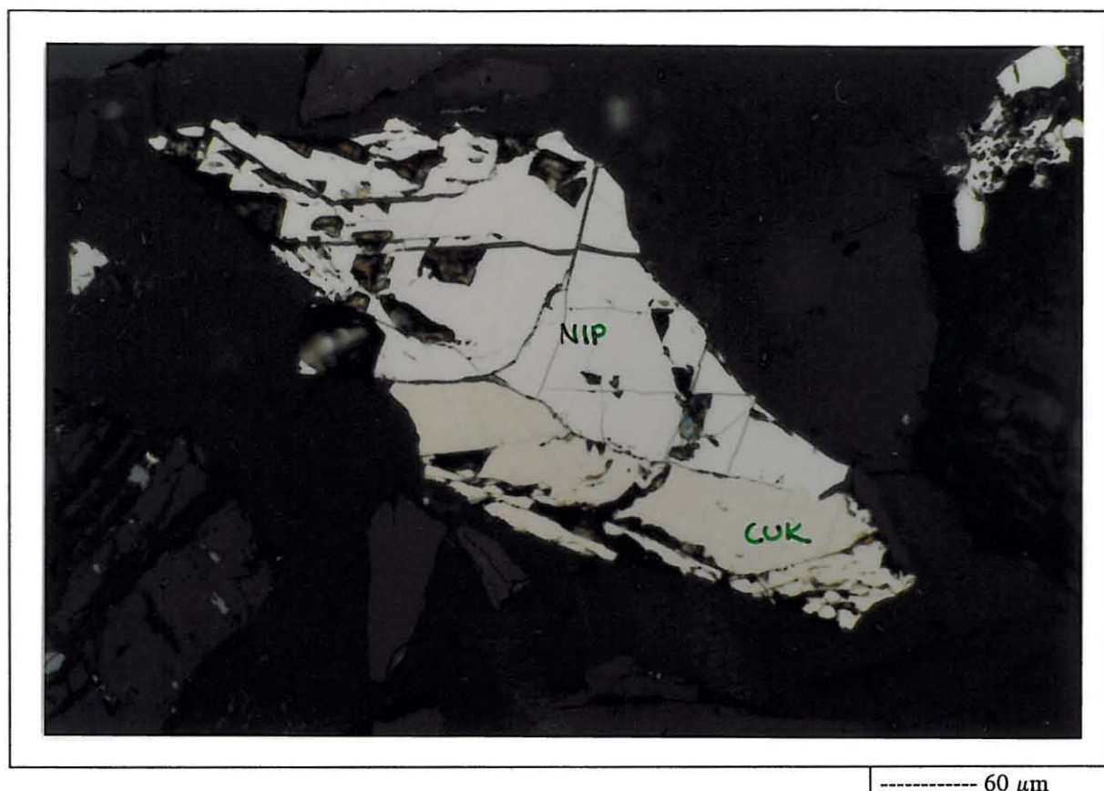
Kuva 5. Pentlandiitti sekarakeena kuparikiisun (CUK) kanssa.
