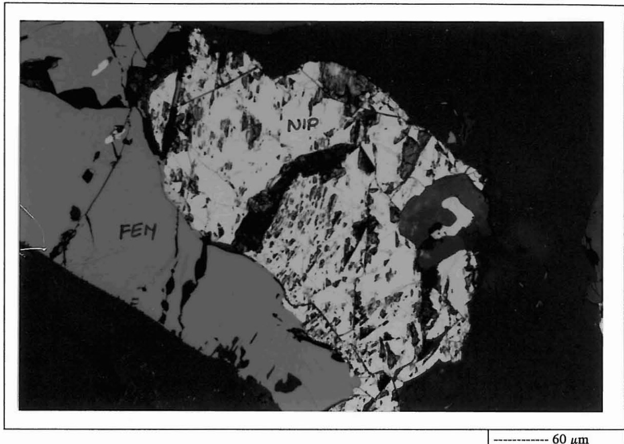
Kuva 1. Pentlandiitti esiintyy näytteessä pääasiassa isoina rakeina. Isoimmat rakeet ovat jopa 1000 \mu\text{m} . Kuvassa on pentlandiitti (NIP) sekarakeena magnetiitin (FEM) kanssa. Pentlandiitissa on havaittavissa heikkoa violariittituumista.
