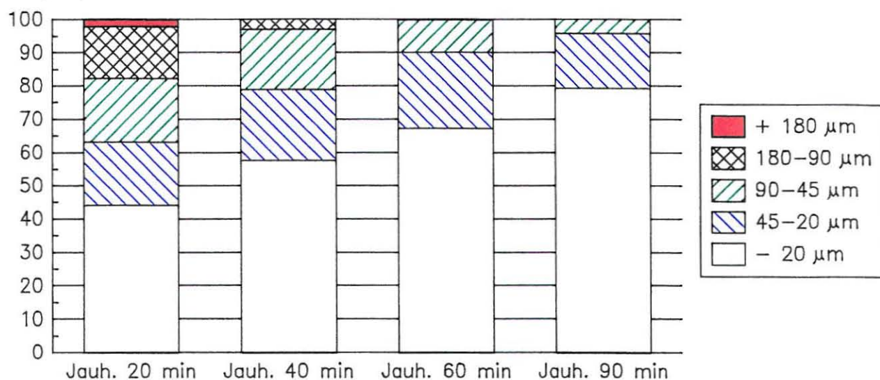
R (Cu), % Cu-saantijakaumat seulafraktioissa
