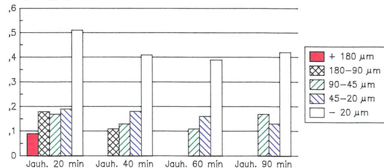
Pt-pitoisuudet seulafraktioissa
