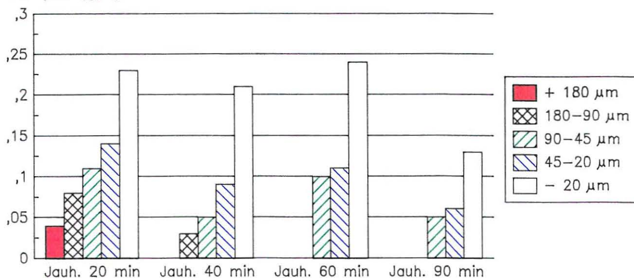
Pd-pitoisuudet seulafraktioissa
