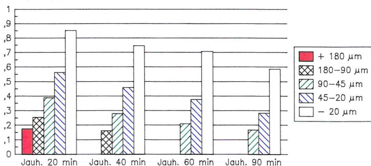
Cu-pitoisuudet seulafraktioissa
