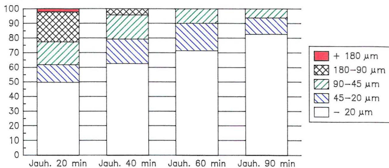
Pt-saantijakaumat seulafraktioissa
