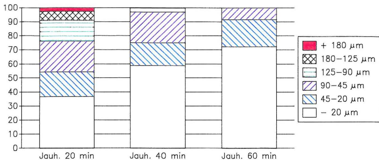
R (Os), % Os-saantijakaumat seulafraktioissa
