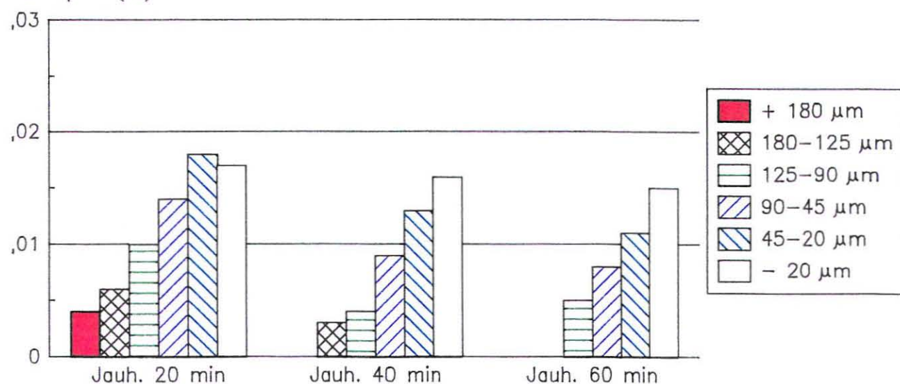
Co-pitoisuudet seulafraktioissa
