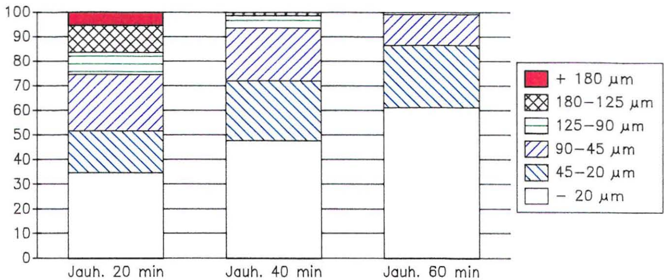
R (Cu), % Cu-saantijakaumat seulafraktioissa
