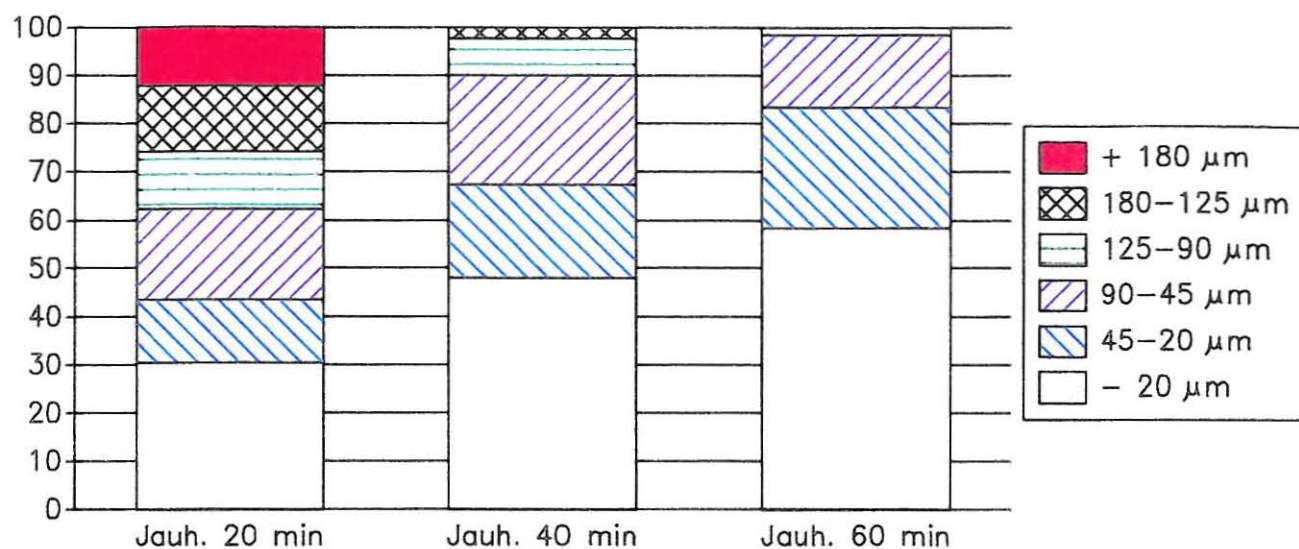
R (Au), % Au-saantijakaumat seulafraktioissa
