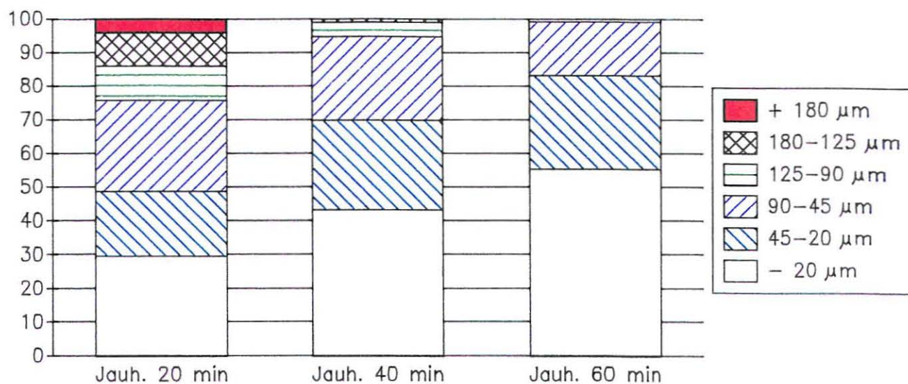
R (Co), % Co-saantijakaumat seulafraktioissa
