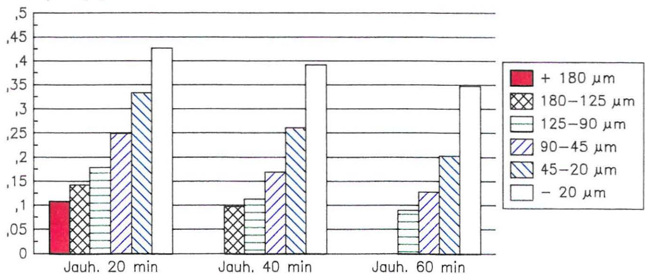
Cu-pitoisuudet seulafraktioissa
