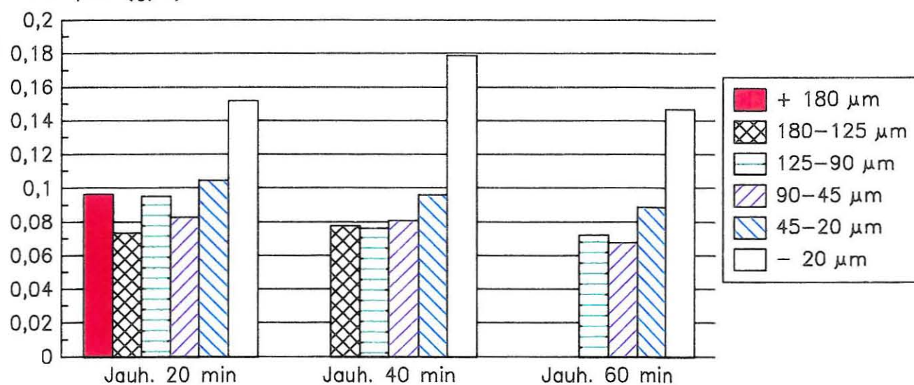
Au-pitoisuudet seulafraktioissa
