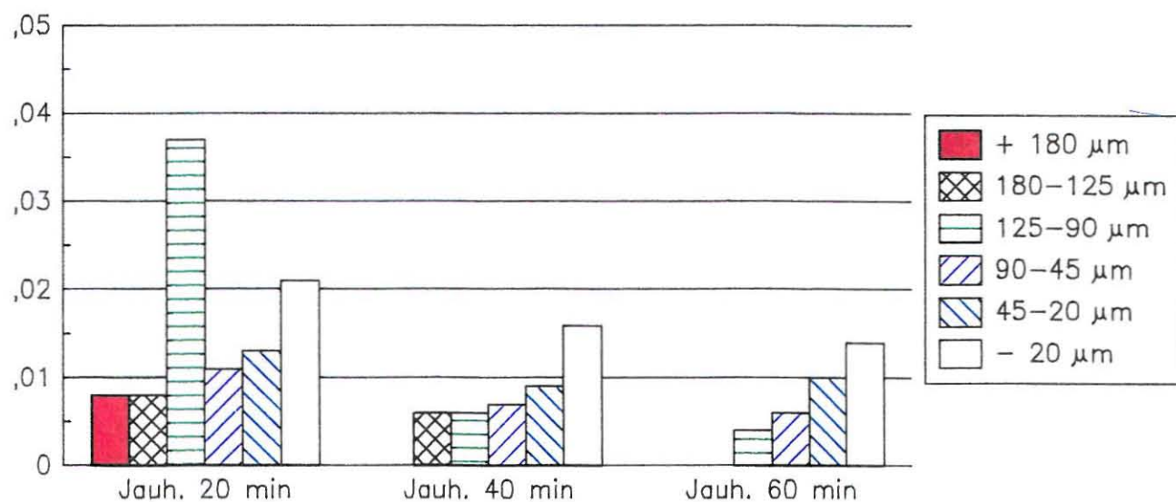
Cu-pitoisuudet seulafraktioissa
