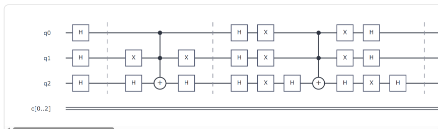
图 4: Qiskit 量子电路的交互式操作视图
