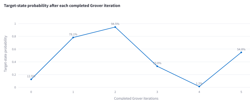
图 3: 目标态概率随完整 Grover 迭代次数变化的曲线
