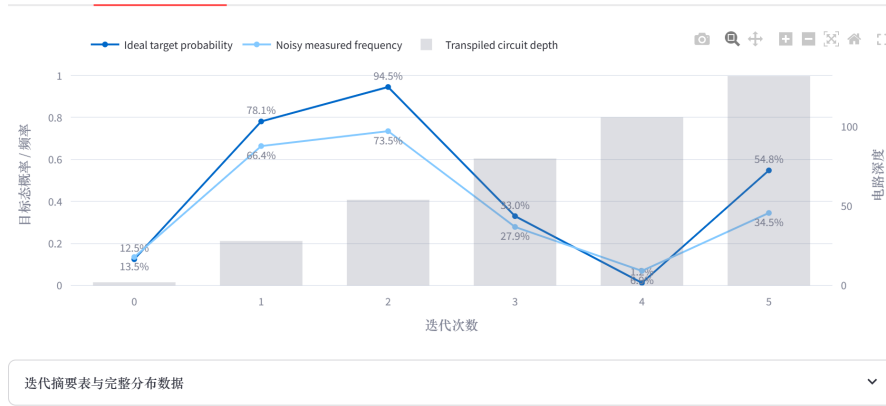
图 5: 理想概率分布与带噪声测量结果的对照视图
