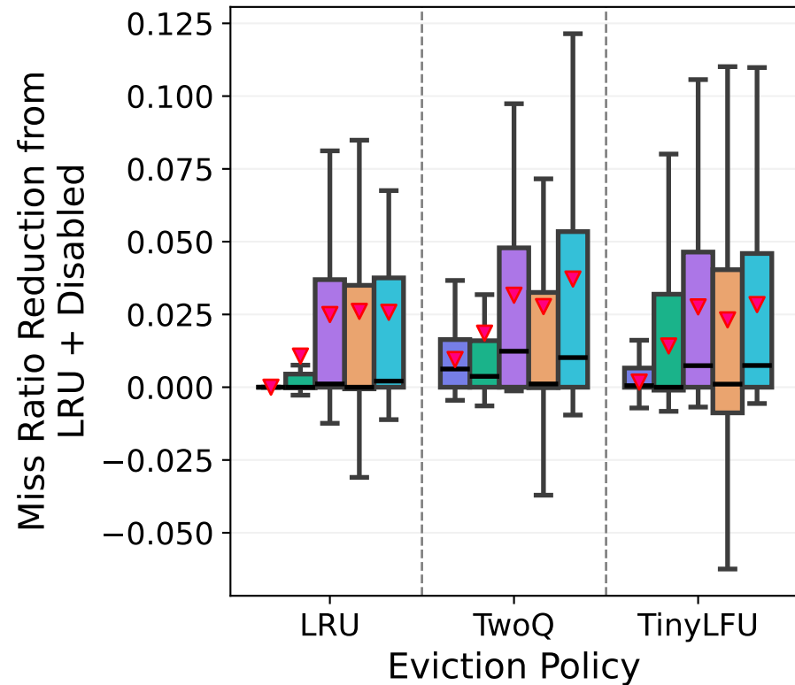
a. Twitter traces, small cache size
