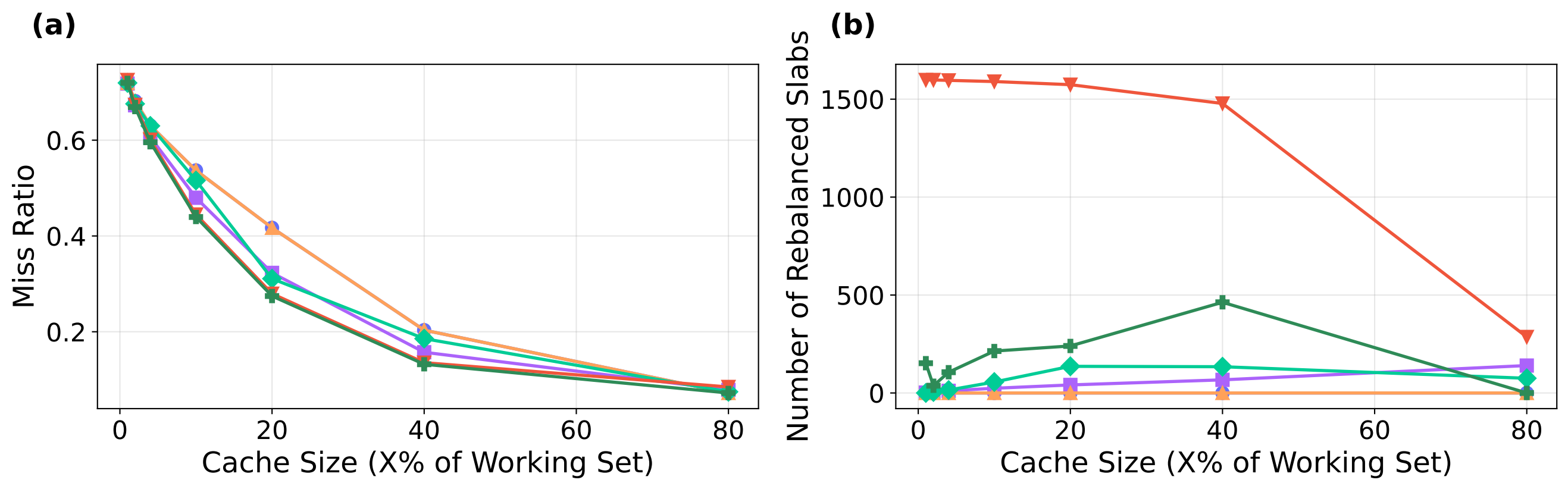
LRU
