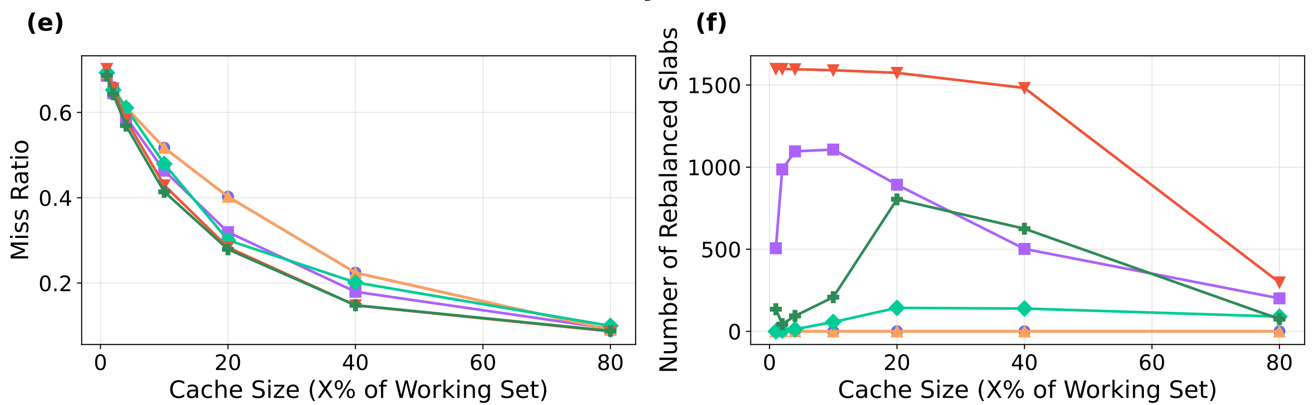
TinyLFU
