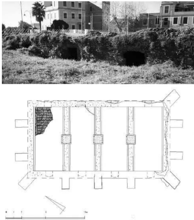
La cisterna prima del recente intervento di scavo e la planimetria attuale (rilievo di F. Graziani). Fonte: Aglietti–Arena, Lazio e Sabina 8, 2012, fig. 2.
