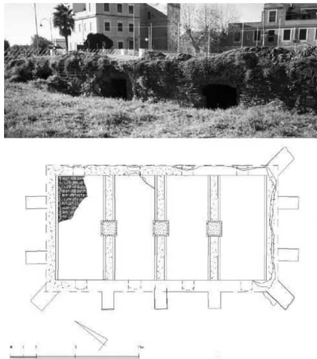
La cisterna prima del recente intervento di scavo e la planimetria attuale (rilievo di F. Graziani). Fonte: Aglietti–Arena, Lazio e Sabina 8, 2012, fig. 2.
