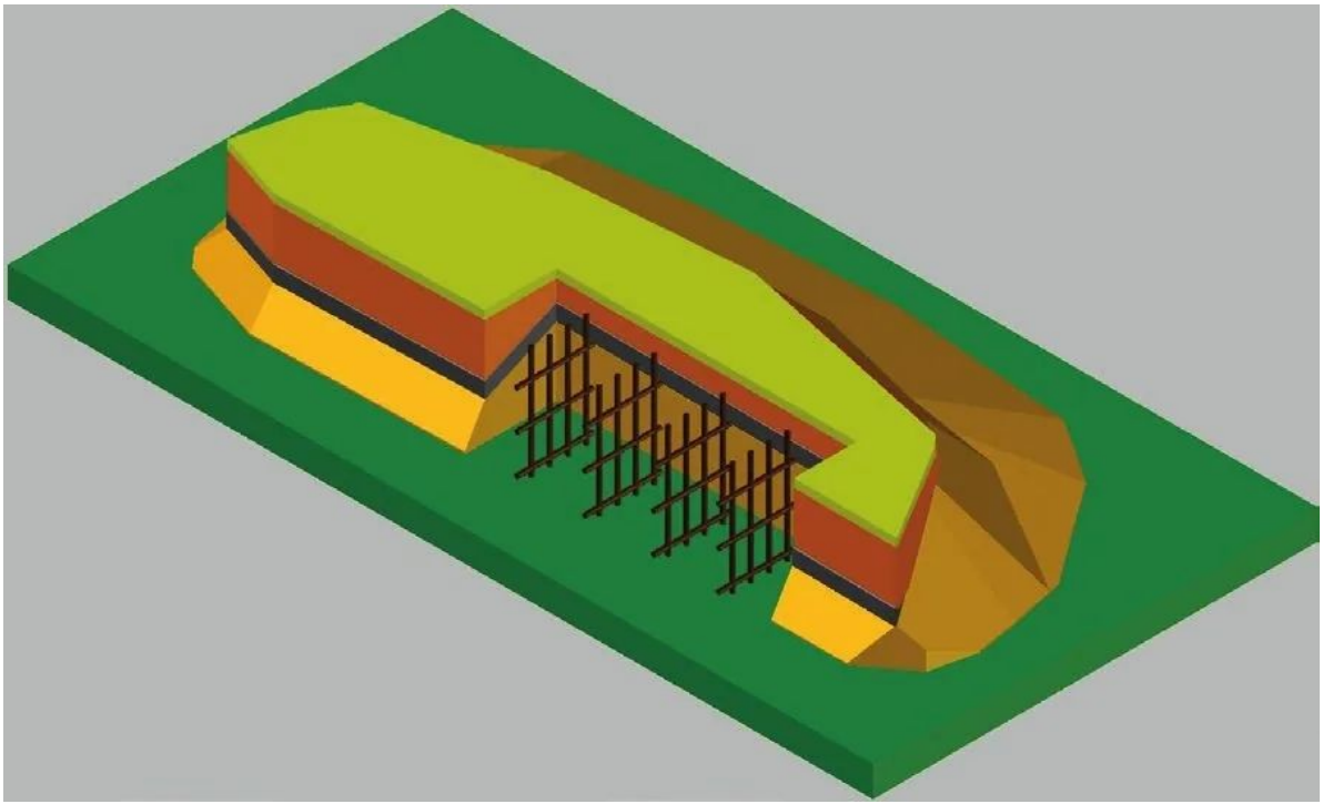
Ricostruzione tridimensionale della struttura del primo agger di Colle Rotondo (XI–X sec. a.C.): nucleo compatto di terra (giallo), strato esterno di carboni e concotti (arancione/rosso), armatura interna di pali lignei (cervoli). (da Nomi 2013 e Guidi–Nomi 2014, in Cifani–Guidi 2016)
