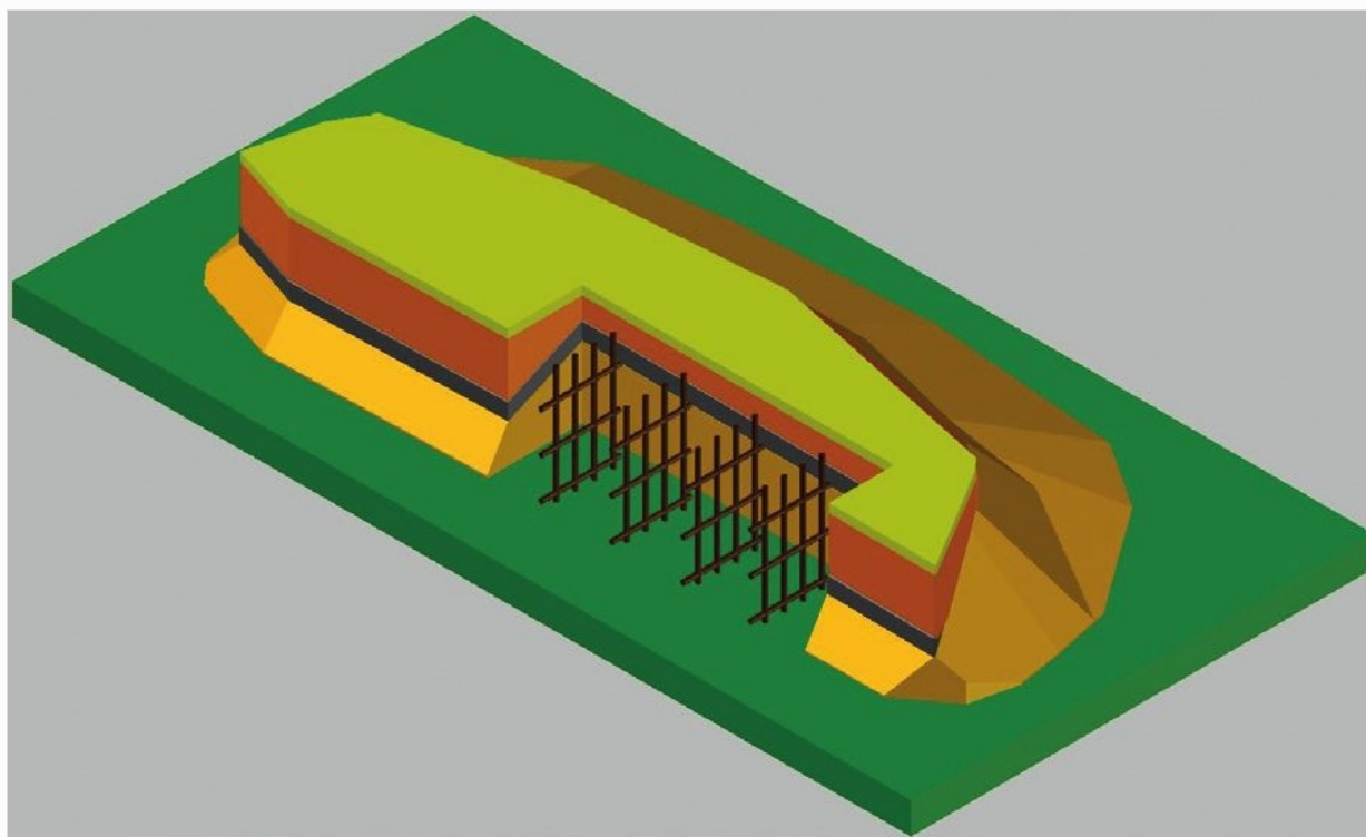
Fig. 5 — Ricostruzione tridimensionale della struttura del primo aggere di Colle Rotondo (XI-X sec. a.C.): nucleo compatto di terra (giallo), strato esterno di carboni e concotti (arancione/rosso), armatura interna di pali lignei (*cervoli*). (da Nomi 2013 e Guidi-Nomi 2014, in Cifani-Guidi 2016, fig. 9)
