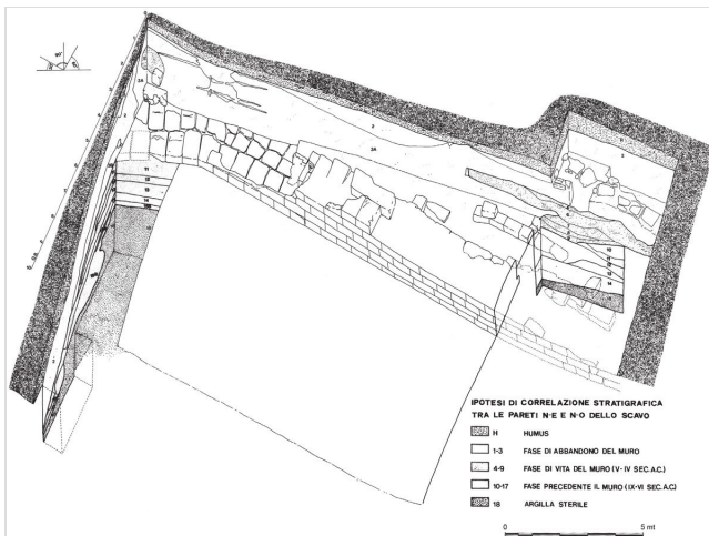
Fig. 6 — Anzio, Vallo Volsco. Assonometria della parte di muro in opera quadrata messa in luce dagli scavi della Soprintendenza (campagne 1980-1981). La legenda stratigrafica mostra: fasi 10-17 precedenti il muro (IX-VI sec. a.C.); fasi 4-9 di vita del muro (V-IV sec. a.C.); fasi 1-3 di abbandono. (da Egidi-Guidi 2009, in Cifani-Guidi 2016, fig. 16)
