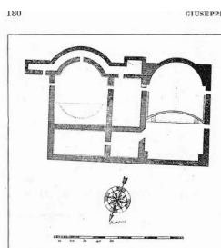
FIG. 24 - SALE TERMALI PRESSO L'ARCO MUTO (Volpi)
