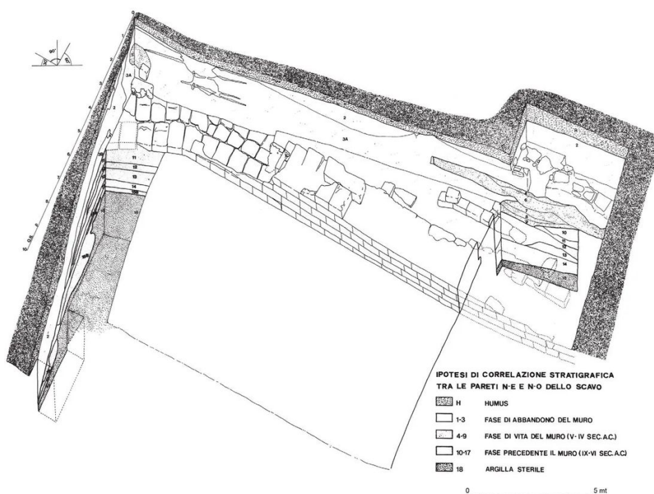
Anzio, Vallo Volsc. Assonometria del muro in opera quadrata (scavi Soprintendenza 1980–1981). Fasi 10–17: precedenti il muro (IX–VI sec. a.C.); fasi 4–9: vita del muro (V–IV sec. a.C.); fasi 1–3: abbandono. (da Egidi–Guidi 2009, in Cifani–Guidi 2016)
