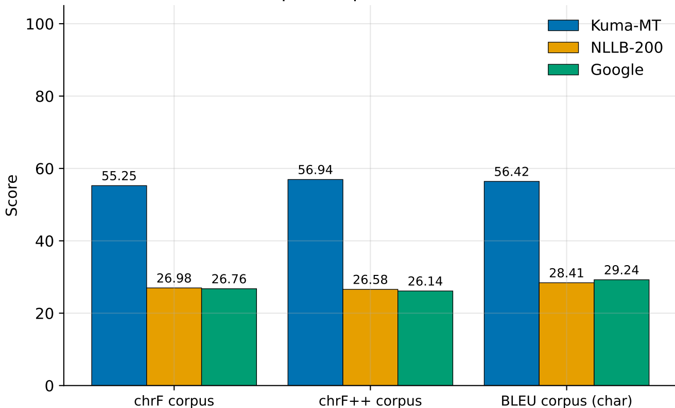
Métriques corpus FR→Bambara
