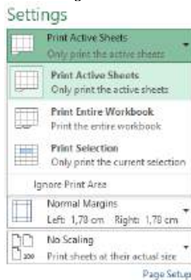
Gambar 71 Setingan Printer
