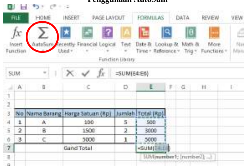
Gambar 64 Penggunaan AutoSum
