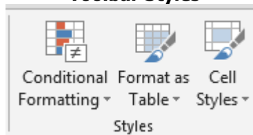
Gambar 24 Toolbar Styles
