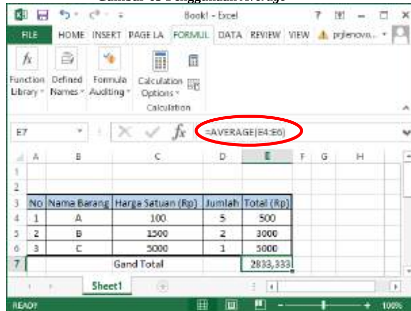
Gambar 65 Penggunaan Average
