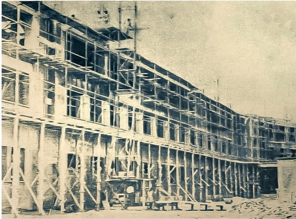
Figura superior: fotografía reportada como “ hospital general de Barquisimeto en construcción ”. Aparece en la Memoria y Cuenta del MOP, año 1952.
