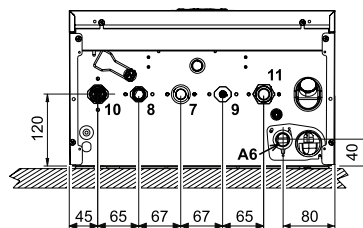
VISTA INFERIORE
