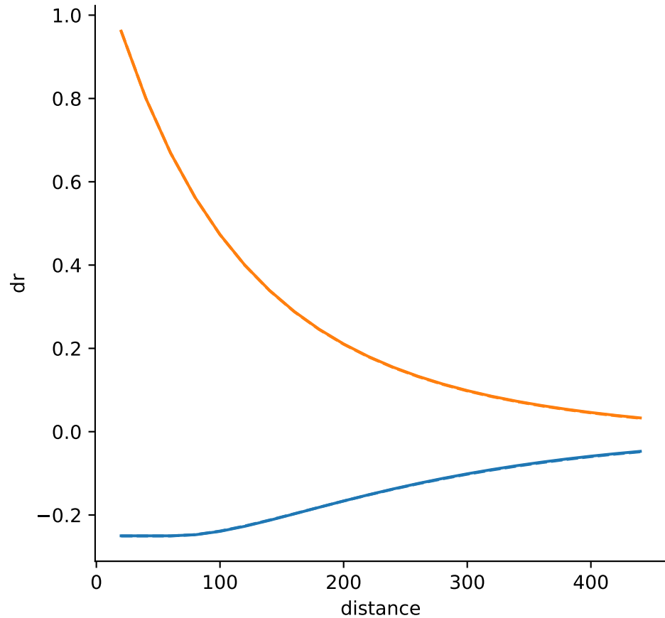
cell_type = PV
