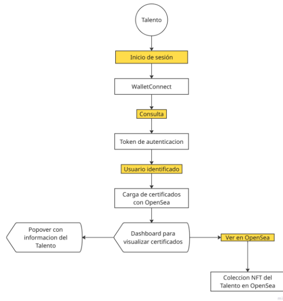
Figura 2. Dashboard del talento.
