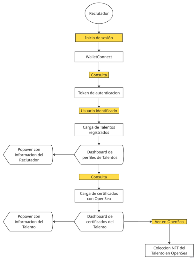
Figura 4. Dashboard del reclutador.
