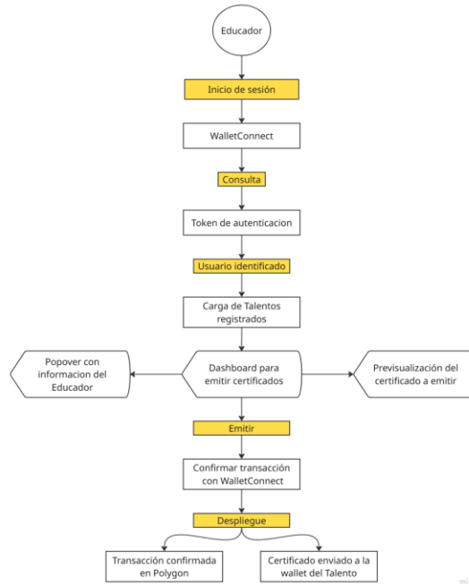
Figura 3. Dashboard del educador.
