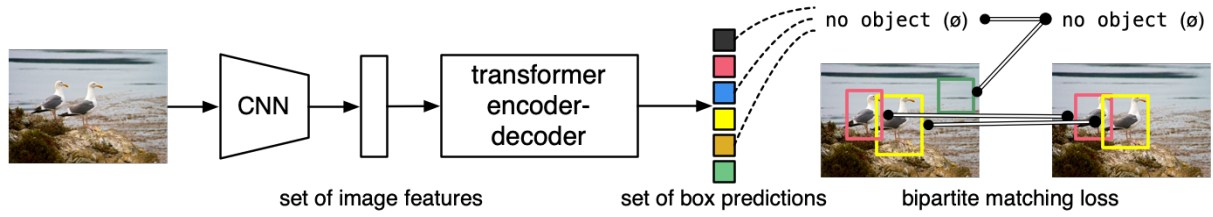
Hình 13: Kiến trúc tổng quan DETR: Backbone CNN (ResNet-50) trích xuất feature map, Transformer Encoder mã hóa ngữ cảnh toàn cục qua self-attention, Transformer Decoder nhận N object queries và sinh ra dự đoán song song, cuối cùng FFN heads xuất lớp và tọa độ bounding box. Nguồn: Carion et al., ECCV 2020.
