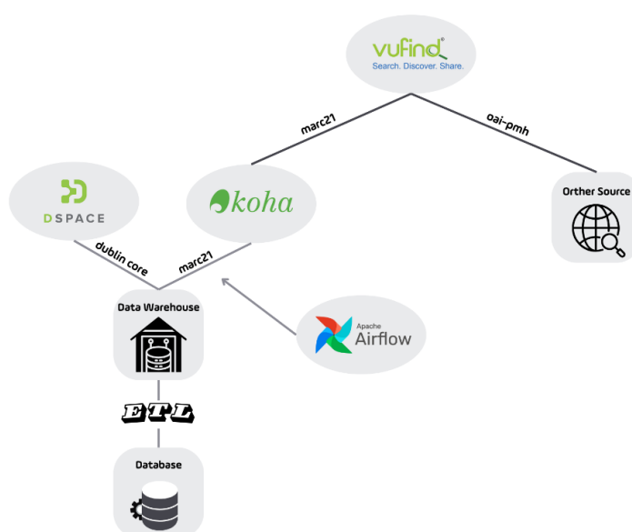
Hình 2.2 Kiến trúc hệ thống thư viện
