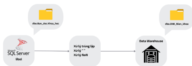
Hình 2.8 Quy trình ETL dữ liệu vào bảng DIM_Nien_khoa
