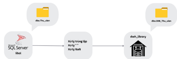
Hình 2.16 Quy trình ETL dữ liệu vào bảng DIM_Thu_vien
