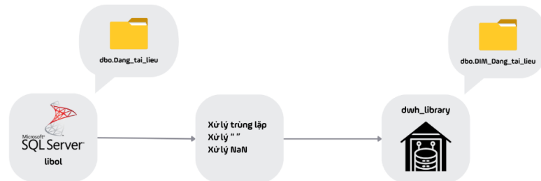
Hình 2.14 Quy trình ETL dữ liệu vào bảng DIM_Dang_tai_lieu
