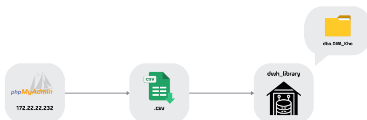
Hình 2.5 Quy trình ETL dữ liệu vào bảng DIM_Khoa
