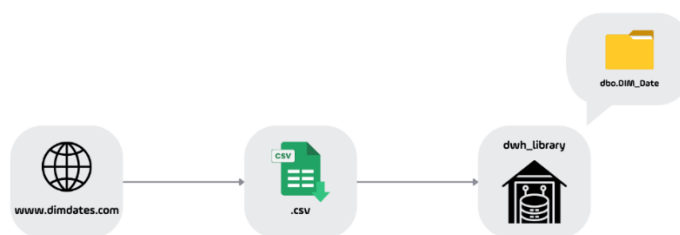
Hình 2.4 Quy trình ETL dữ liệu vào bảng DIM_Date
