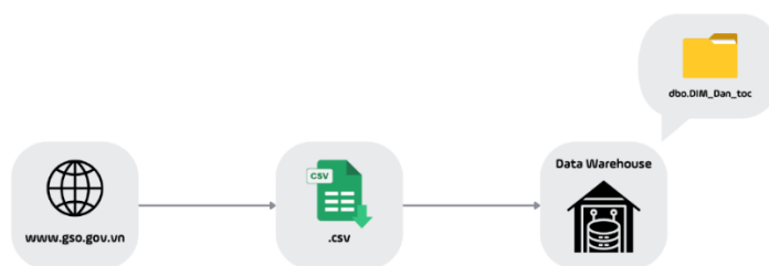
Hình 2.4 Quy trình ETL dữ liệu vào bảng DIM_Dan_toc
