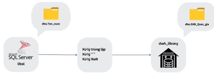
Hình 2.12 Quy trình ETL dữ liệu vào bảng DIM_Quoc_gia
