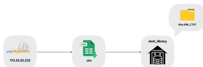
Hình 2.10 Quy trình ETL dữ liệu vào bảng DIM_CTDT
