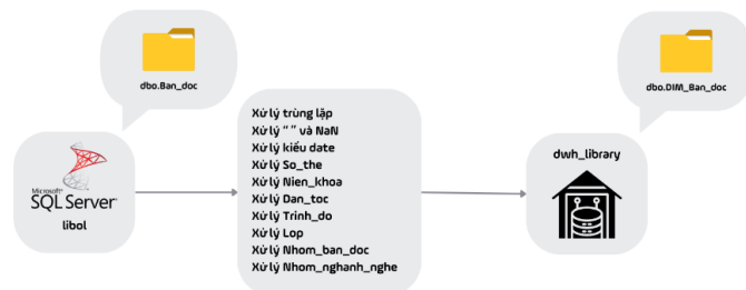
Hình 2.18 Quy trình ETL dữ liệu vào bảng DIM_Ban_doc
