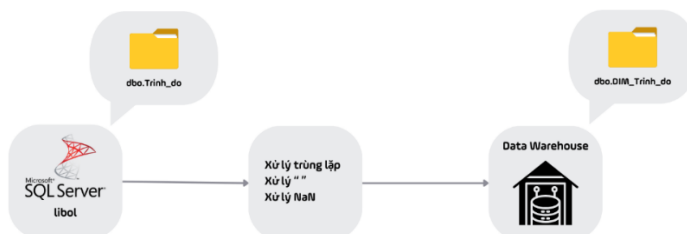
Hình 2.5 Quy trình ETL dữ liệu vào bảng DIM_Trinh_do
