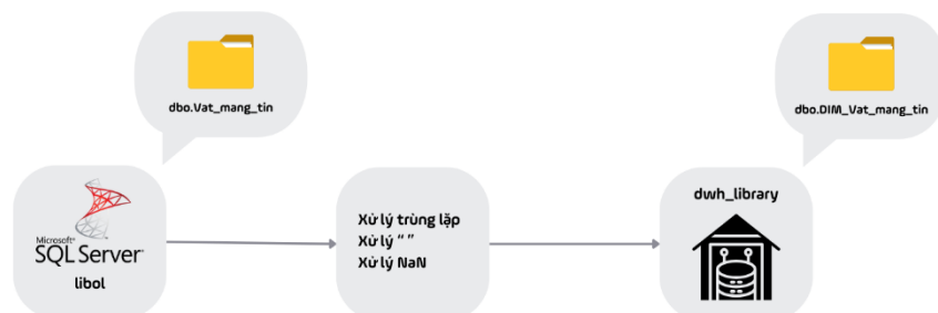
Hình 2.13 Quy trình ETL dữ liệu vào bảng DIM_Vat_mang_tin
