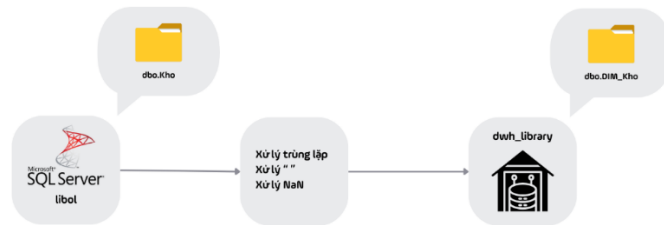
Hình 2.17 Quy trình ETL dữ liệu vào bảng DIM_Kho
