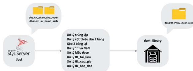
Hình 2.21 Quy trình ETL dữ liệu vào bảng DIM_Phieu_muon_sach
