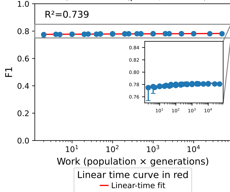
D) F1 vs Work ( \mu=0.2 , meta=rf)
