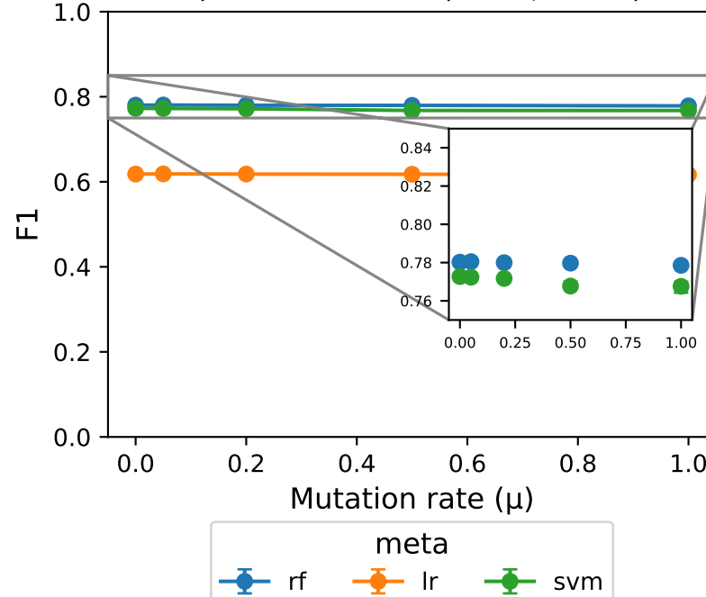
E) F1 vs Mutation ( P=50 , G=10 )
