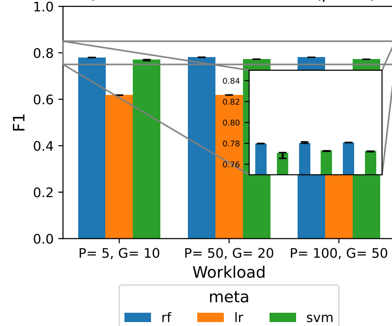
F) F1 vs Meta at 3 Workloads ( \mu=0.2 )
