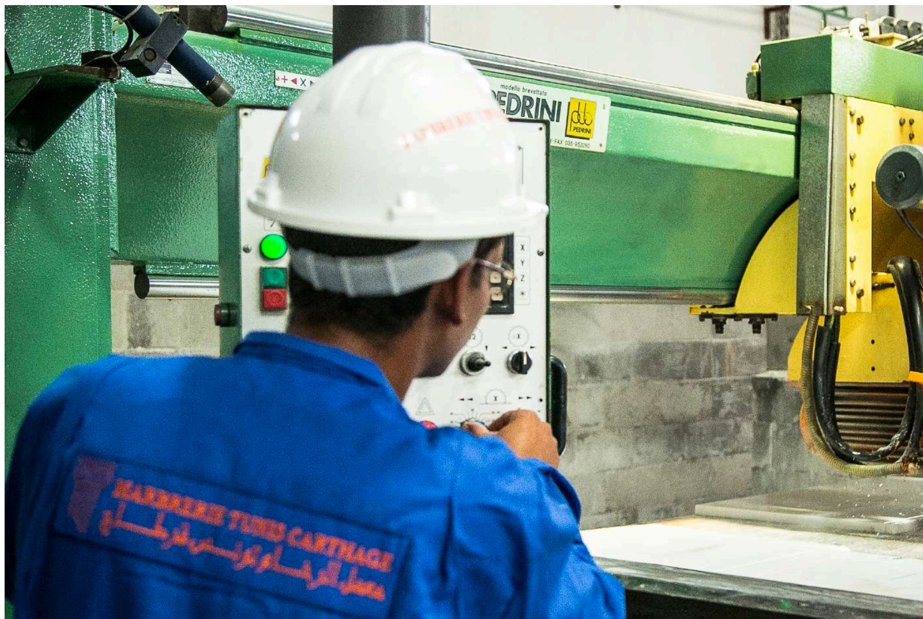
Débiteuse à pont / Bridge Saw
