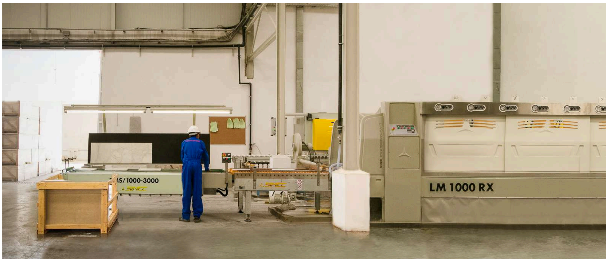
Ligne de polissage / Polishing line
