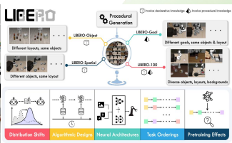
LIBERO ✓
