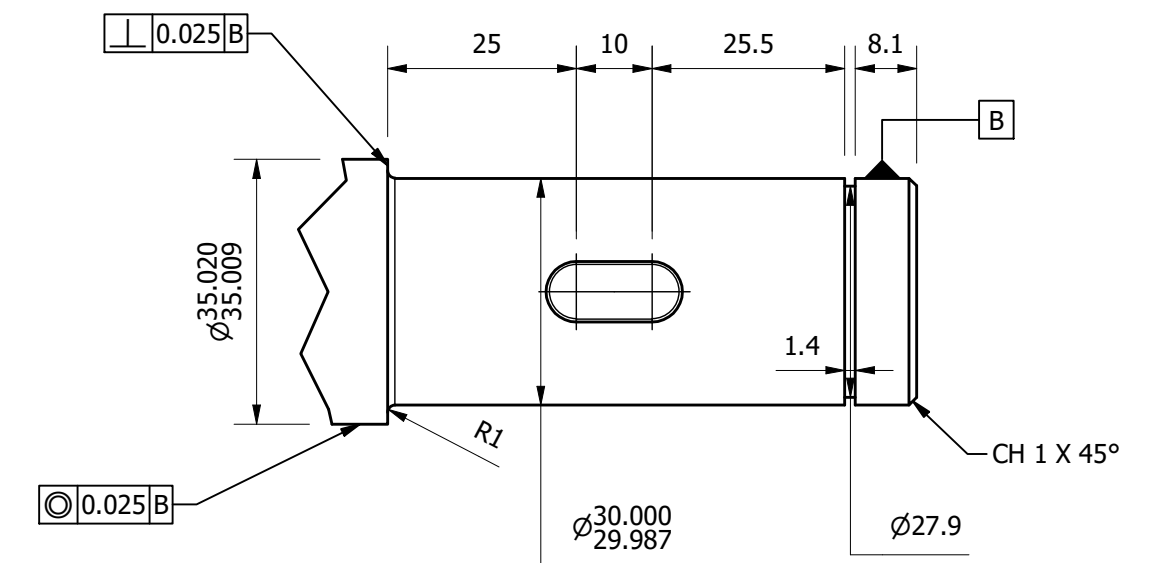
DETAIL C ( 1 : 1 )
