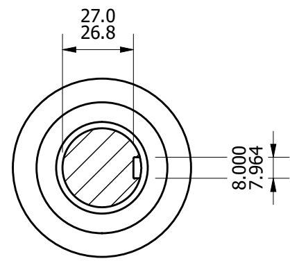
SectionX-X ( 1 : 2 )
