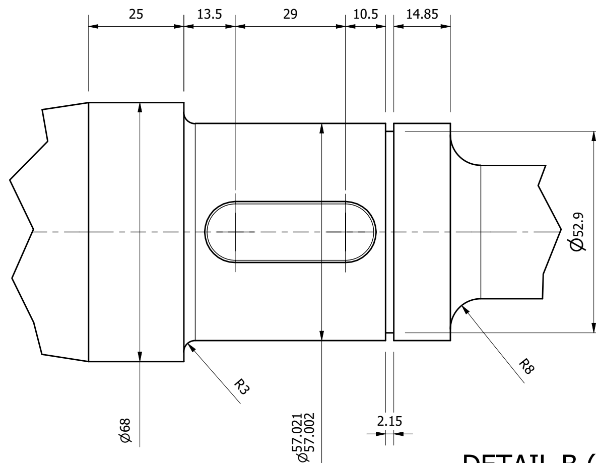
DETAIL B ( 1 : 1 )
