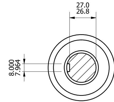
SectionZ-Z ( 1 : 2 )
