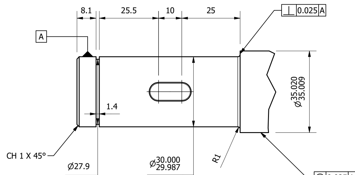
DETAIL A ( 1 : 1 )
