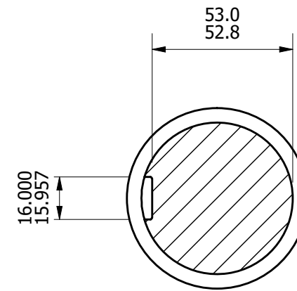
Section Y-Y ( 1 : 2 )
