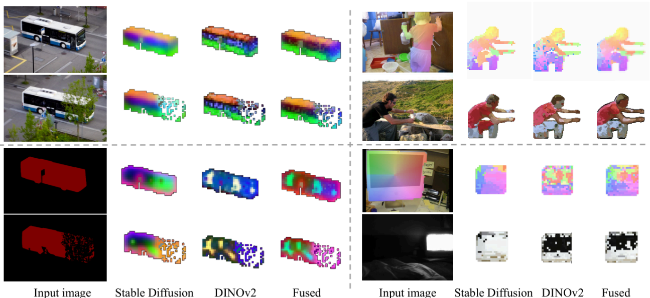
그림 3 대응 관점에서 본 특징별 분석. 왼쪽 은 DAVIS[43] 입력의 PCA 시각화, 오른쪽 은 SPair-71k[36]의 밀집 대응이다. 그림은 입력 조건에 따라 SD 특징과 DINO 특징의 성능이 어떻게 달라지는지 보여 준다. 같은 인스턴스(왼쪽 위), 순수 객체 마스크(왼쪽 아래), 의미 이해가 필요한 어려운 입력(오른쪽 위), 공간 정보가 필요한 어려운 입력(오른쪽 아래) 발표 15 · 16p 을 비교한다. 결과는 보충 자료 B.1에 더 실었다.
