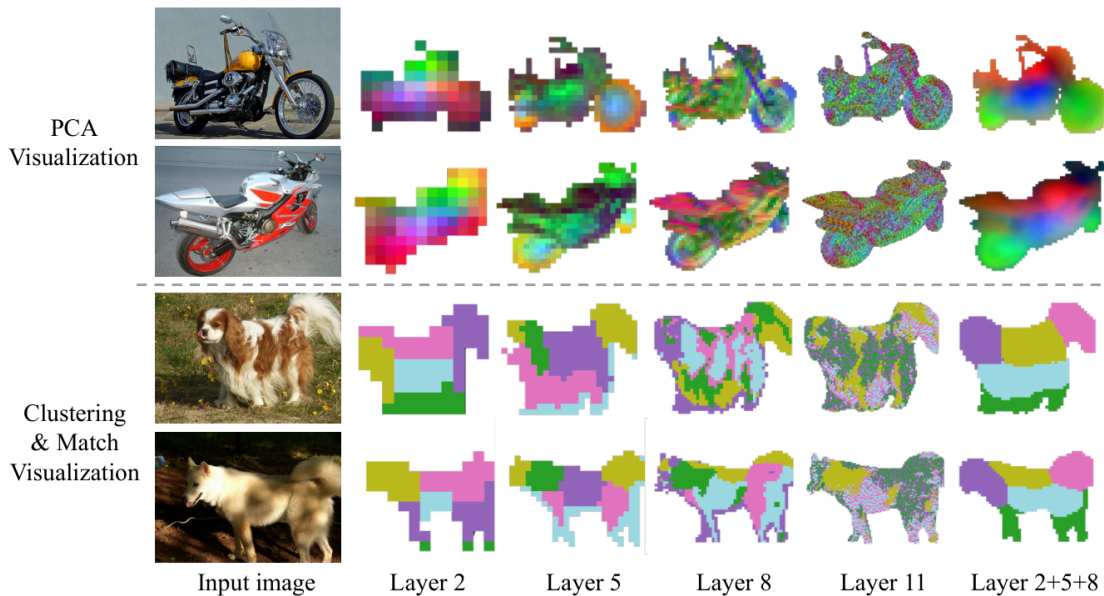
그림 2 SD 디코더 레이어별 특징 분석. 위: 초기(레이어 2), 중간(레이어 5와 8), 마지막(레이어 11) 레이어 특징을 PCA로 시각화했다. 분할한 인스턴스 쌍 전체에서 구한 PCA의 처음 세 성분을 색 채널로 쓴다. 초기 레이어는 의미에, 후기 레이어는 질감에 더 집중한다. 발표 11p 아래: 같은 특징을 K-평균(K-Means)으로 군집화했다. 이미지마다 따로 K-평균 군집을 구한 다음, 헝가리안 방법(Hungarian method)으로 군집 사이의 최적 짝 발표 12p 질문 대비 을 찾는다. 각 열의 색은 서로 짝지어진 군집 한 쌍을 나타낸다.
