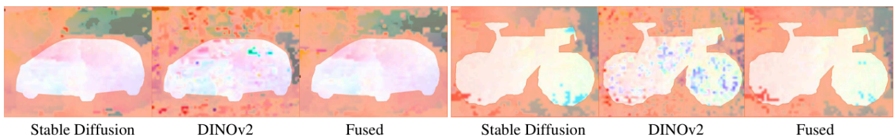
그림 4 특징별 시맨틱 흐름 맵. 흰 마스크는 유효한 화소를, 주황 마스크는 배경 흐름을 구분한다. SD 특징은 매끄러운 흐름 필드를 내고, DINOv2에는 고립된 이상치가 보인다. (발표 17p)
