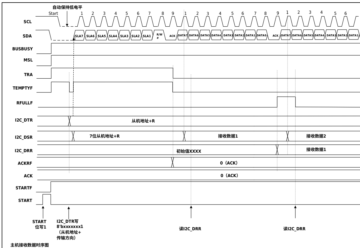
图 28-6 7 位地址格式的主机接收数据的时序图 (例)
