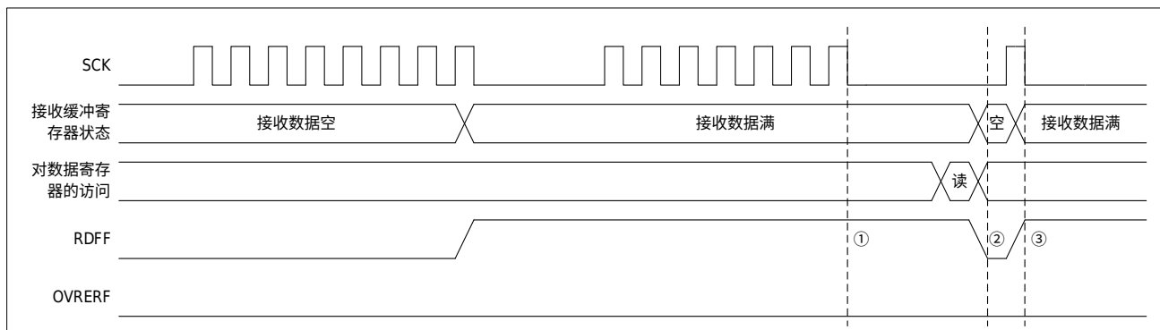
图 29-12 启用时钟自动停止功能时的动作示意图 (CPHA=0)
