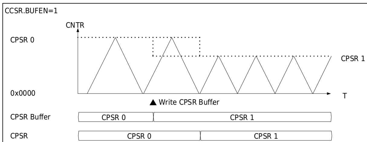
图 21-10 缓存使能时修改三角波计数周期
