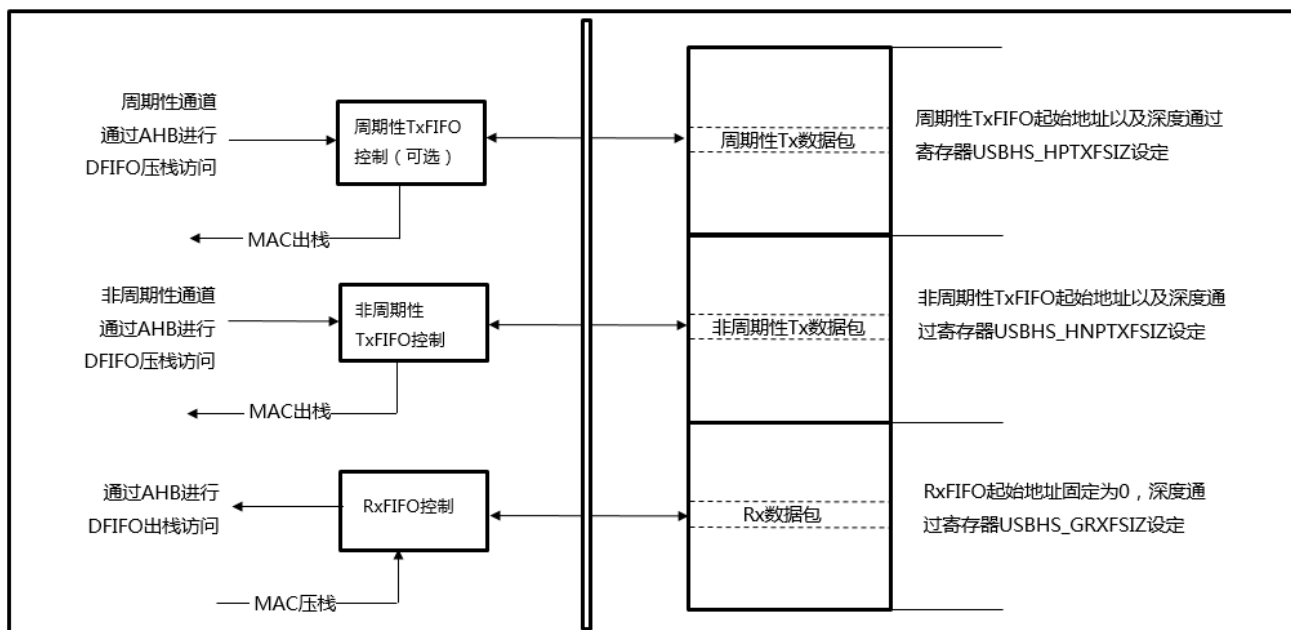
图 32-5 USBHS 主机模式下 FIFO 架构示意图
