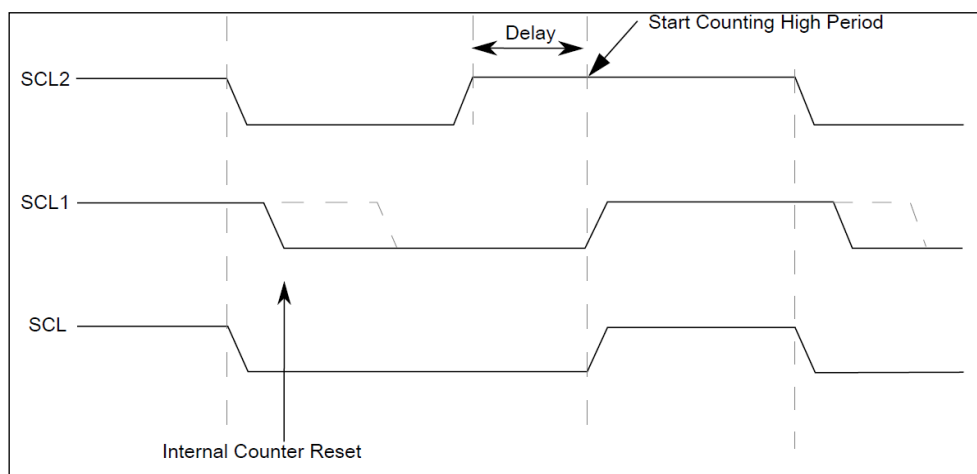
图 28-9 SCL 同步时序
