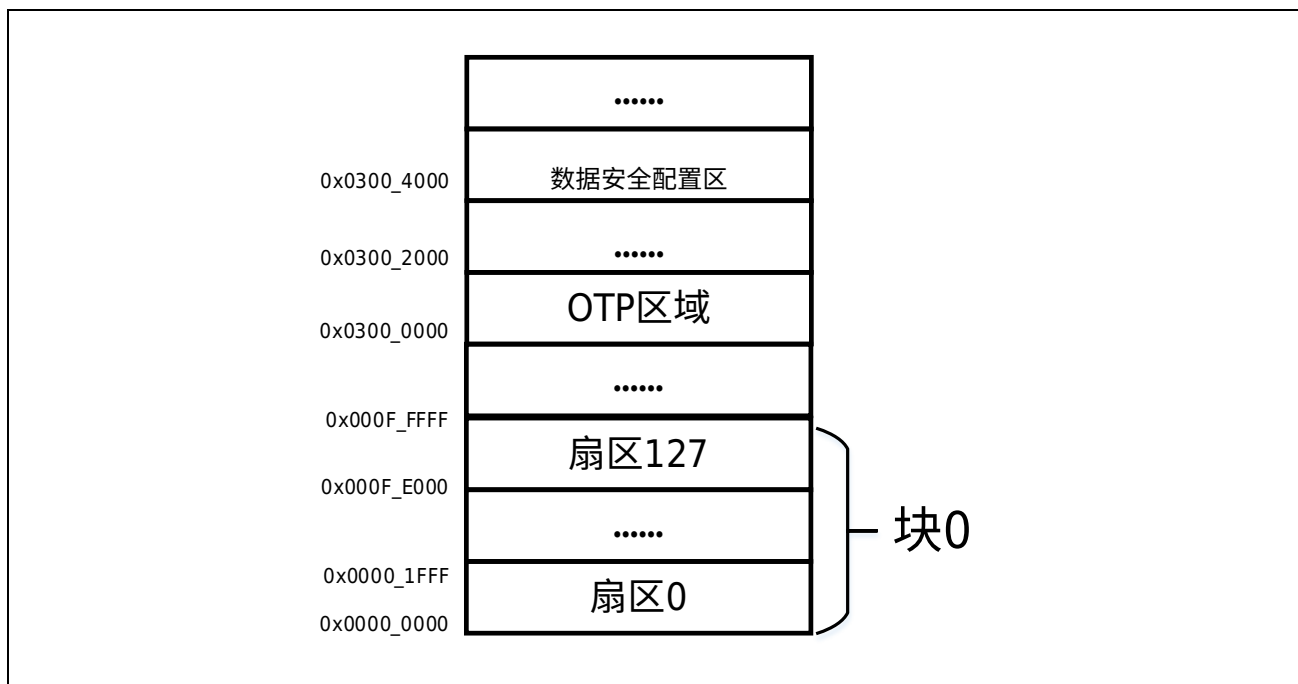
图 7-1 1MBytes 产品单 FLASH 地址分布
