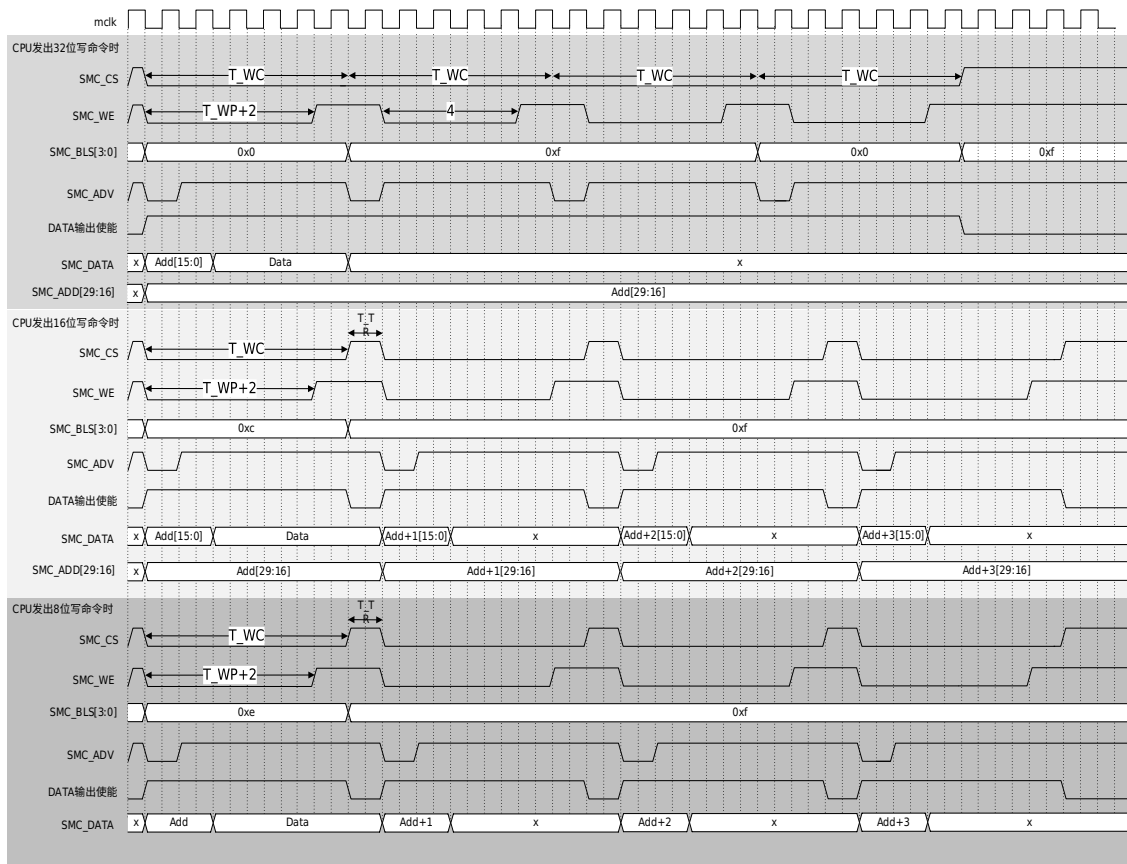
图 37-24 地址数据复用突发写动作基本时序（异步方式（WSYN=0）&32 位位宽（MW=10） &WBL=001&BLSS=0）
