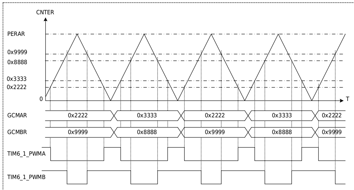
图 20-18 双边对称独立 PWM
