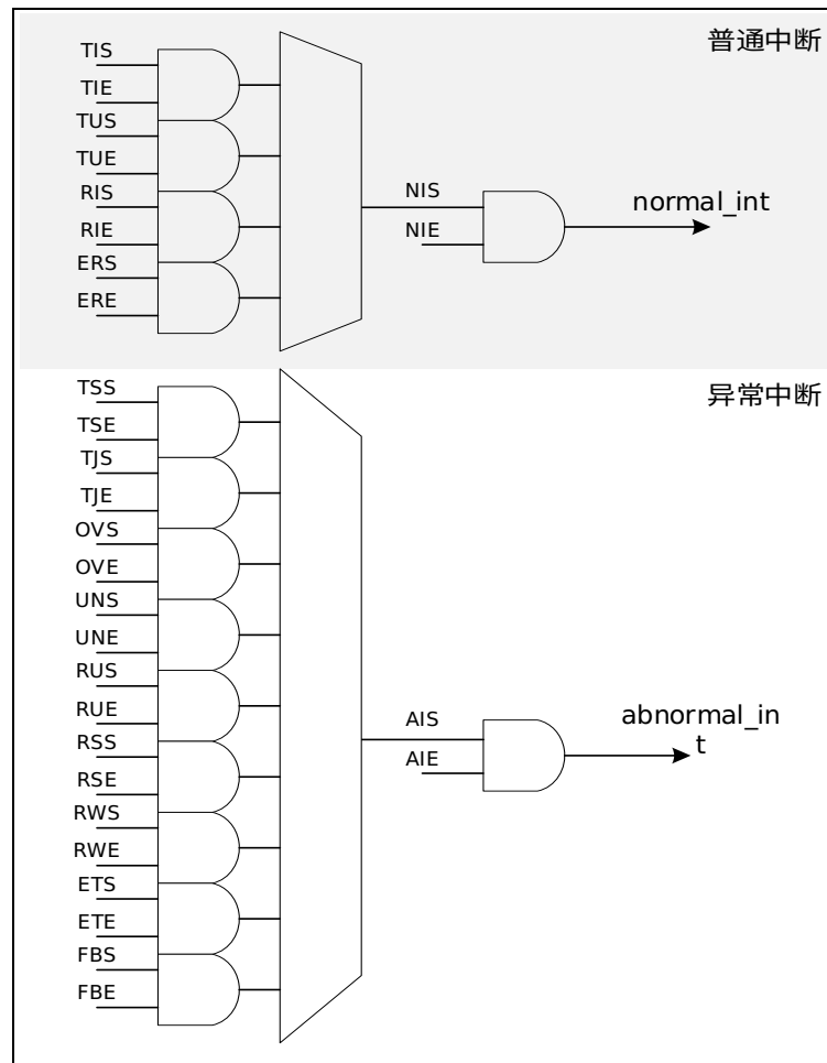
图 36-22 DMA 中断组成
