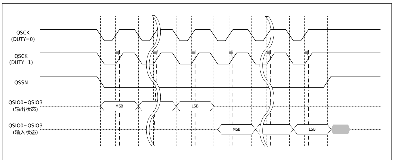
图 30-9 基准时钟选择 HCLK 三分频时输出时钟占空比校正示意图
