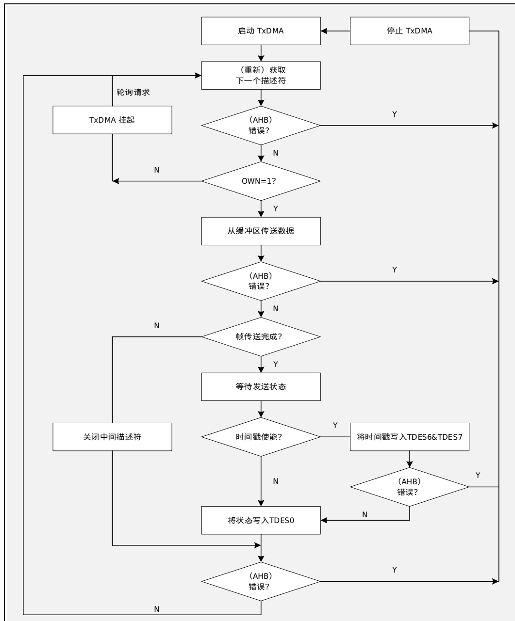
图 36-18 TxDMA 动作流程（非 OSF 模式）
