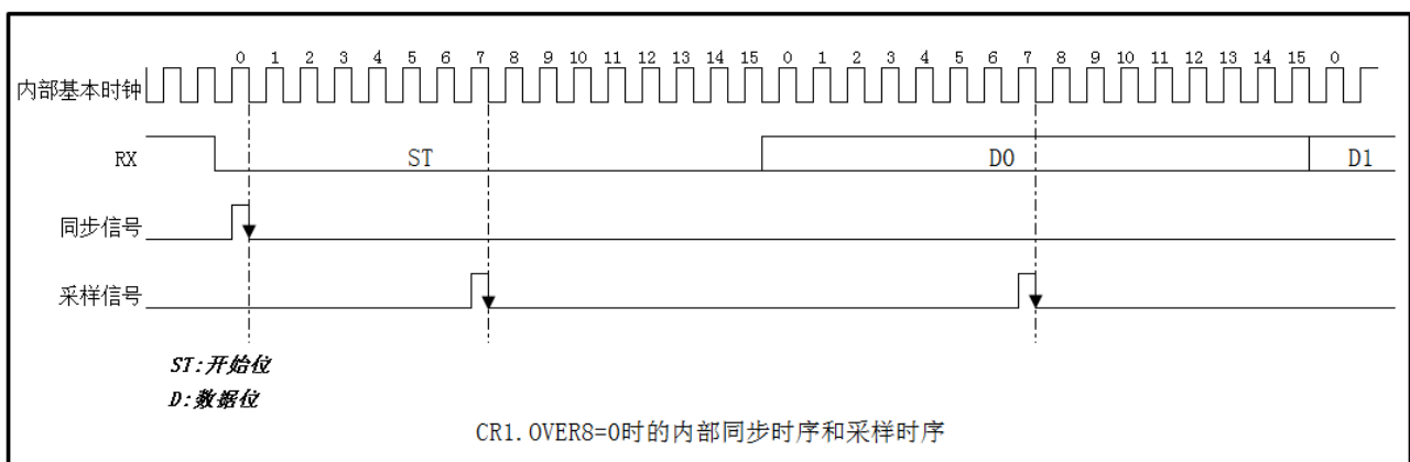
图 27-5 UART 内部同步和采样时序
