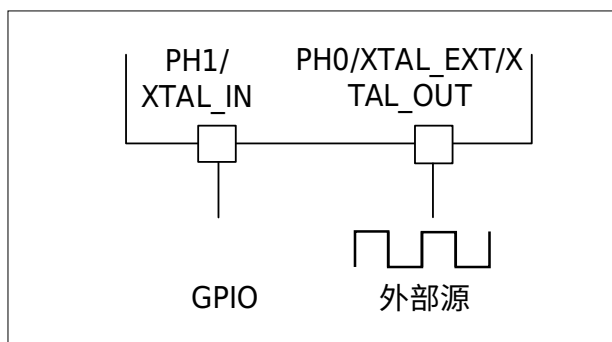
图 4-4 外部高速时钟输入的连接示例
