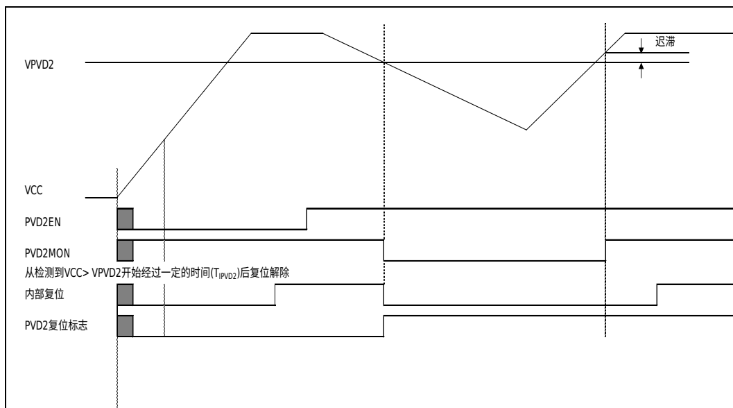
图 5-10 电源监视 2 复位运行时序图
