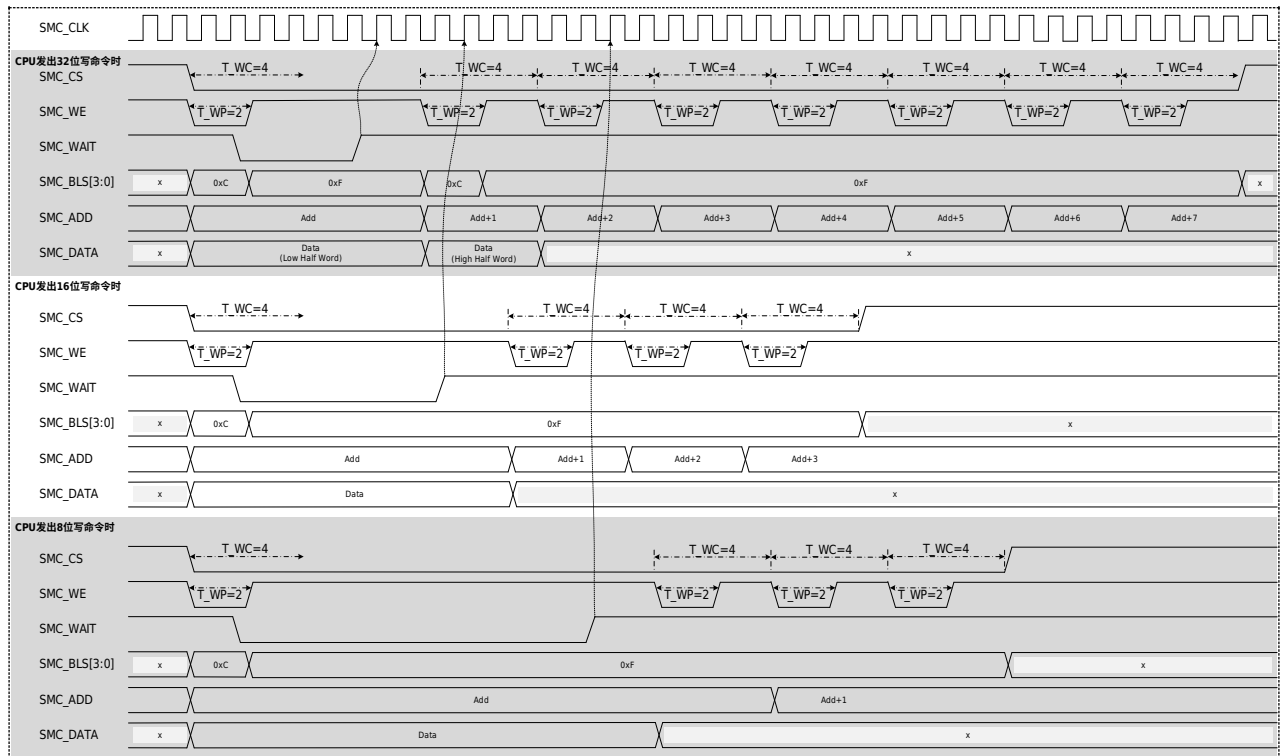
图 37-16 单次写动作基本时序（同步方式（WSYN=1）&16 位位宽（MW=01）&BLS=1）
