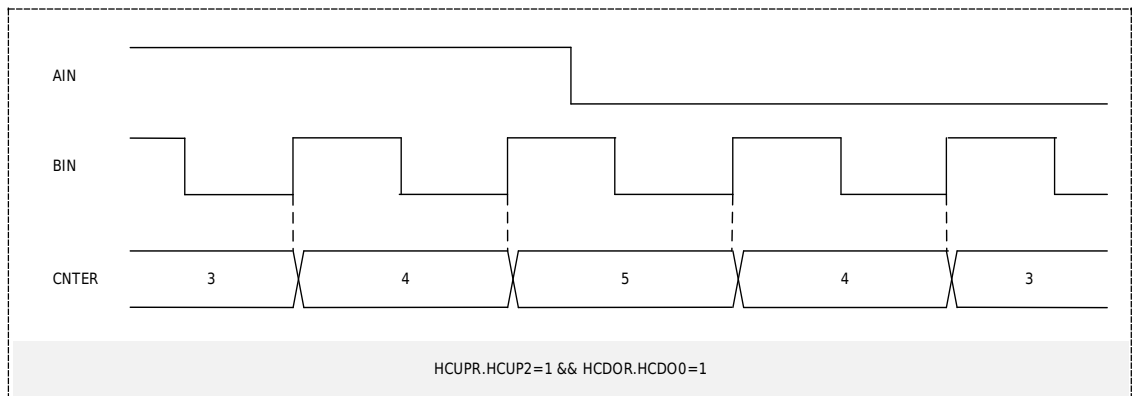
图 20-29 位置计数模式-方向计数
