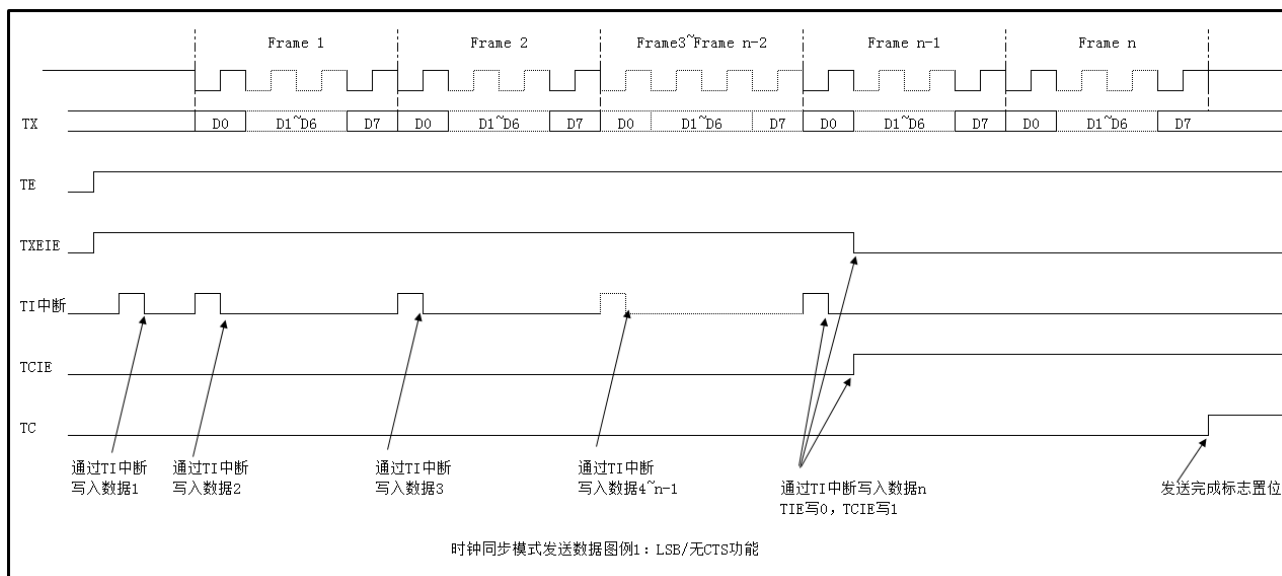
图 27-20 时钟同步模式发送数据图例 1
