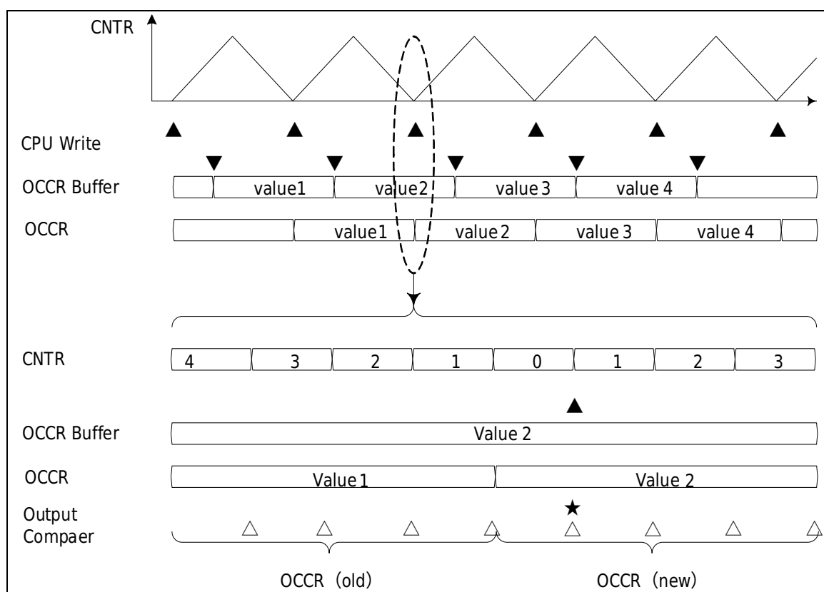
图 21-11 OCCR 缓冲数据传输 (周期间隔响应链接禁止时)
