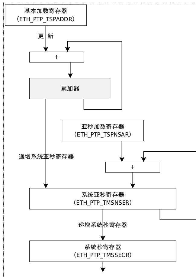
图 36-16 系统时间校准
