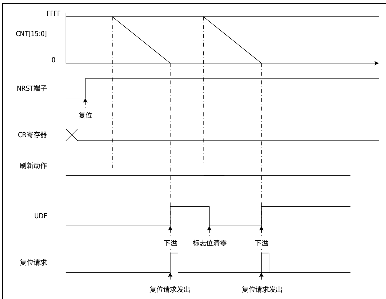
图 26-1 硬件启动例
