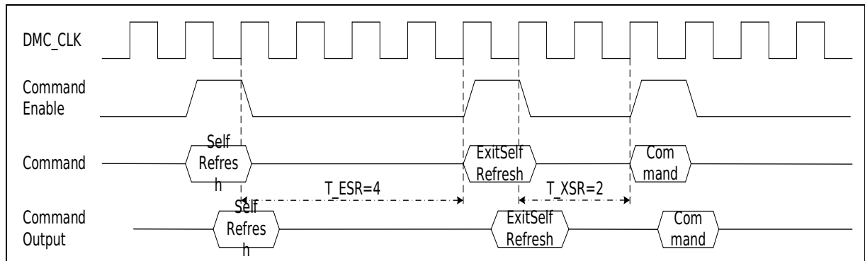
图 37-28 自刷新动作的进入和退出时序
