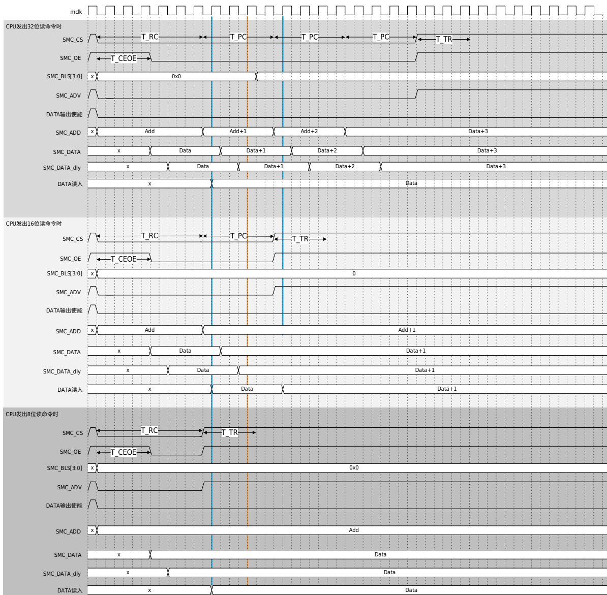
图 37-22 地址数据非复用突发读动作基本时序（同/异步方式（RSYN=1/0）&amp;32 位位宽（MW=10）&amp;RBL=001）
