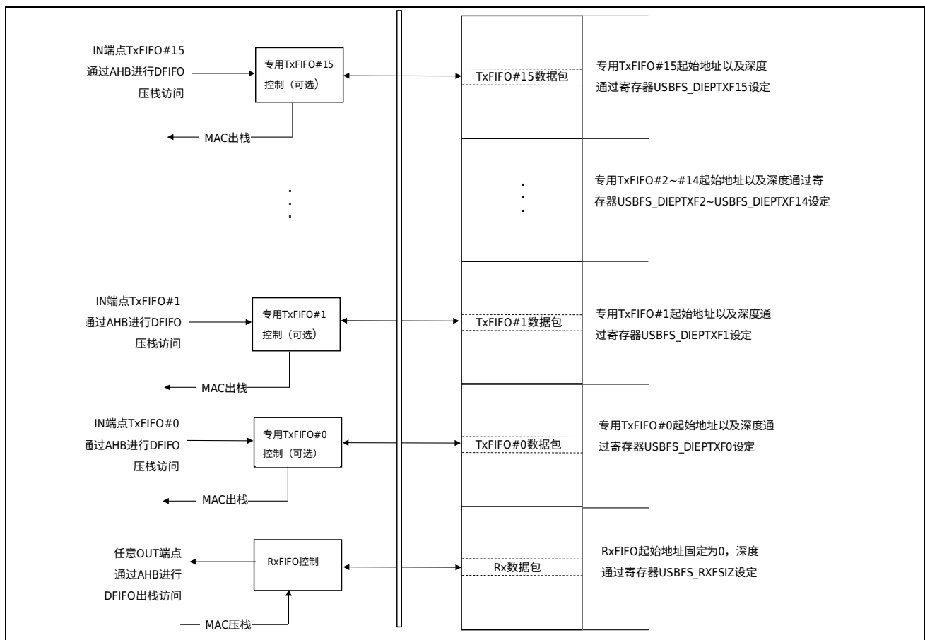
图 33-6 USBFS 设备模式下 FIFO 架构示意图
