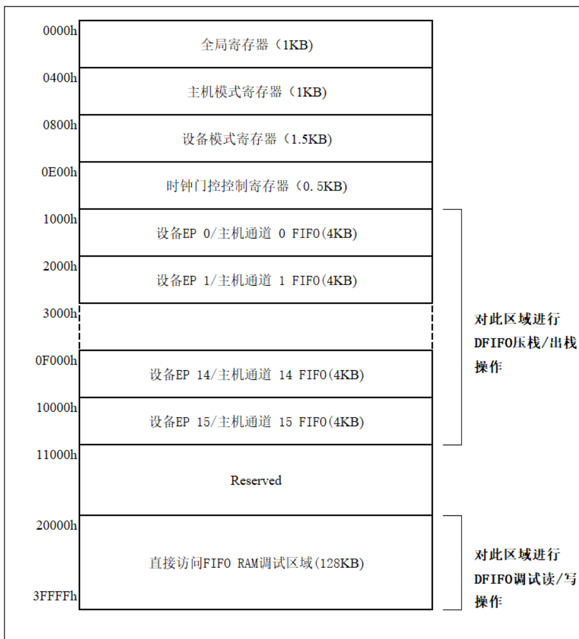
图 33-7 USBFS 控制状态寄存器存储器映射
