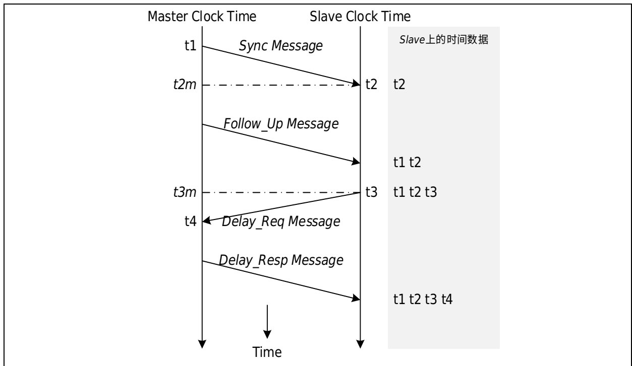
图 36-15 时钟同步图
