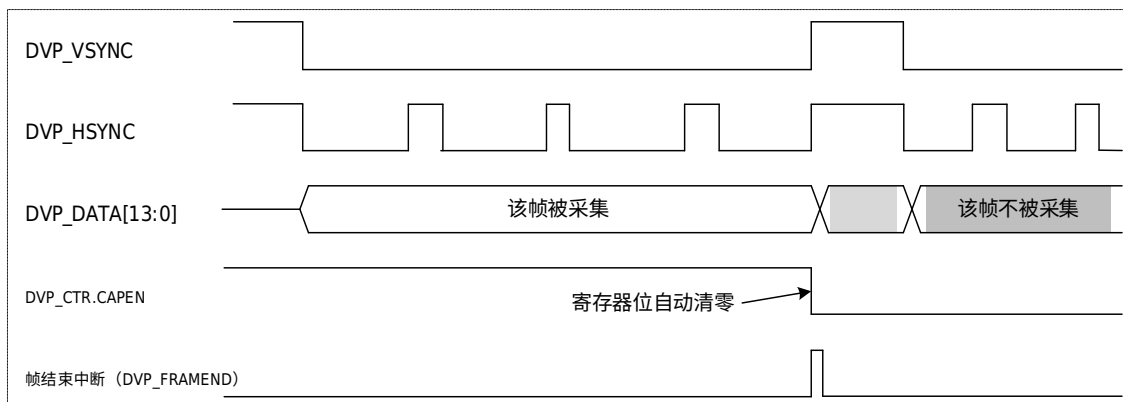
图 38-3 单帧模式数据采集动作
