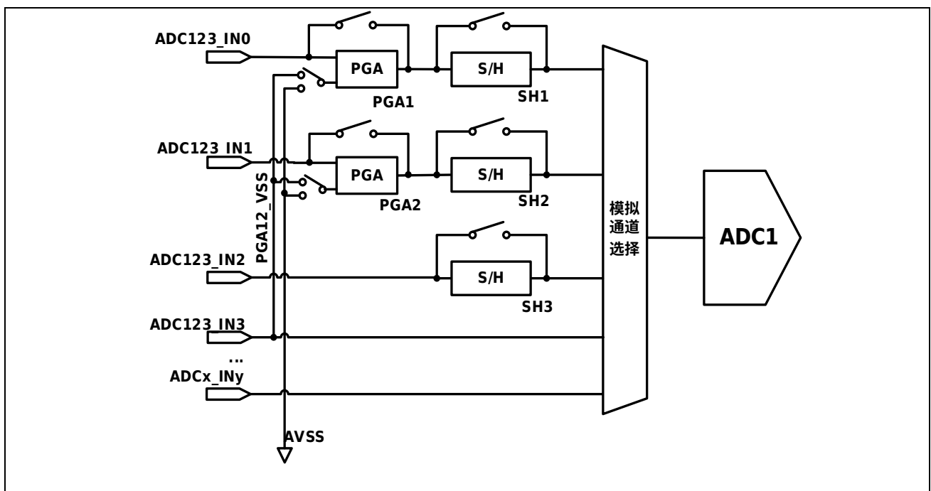
图 17-11 ADC 单元 1 的 PGA 与 SH 通道示意图
