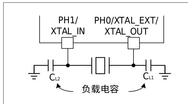
图 4-3 外部高速振荡器连接示例
