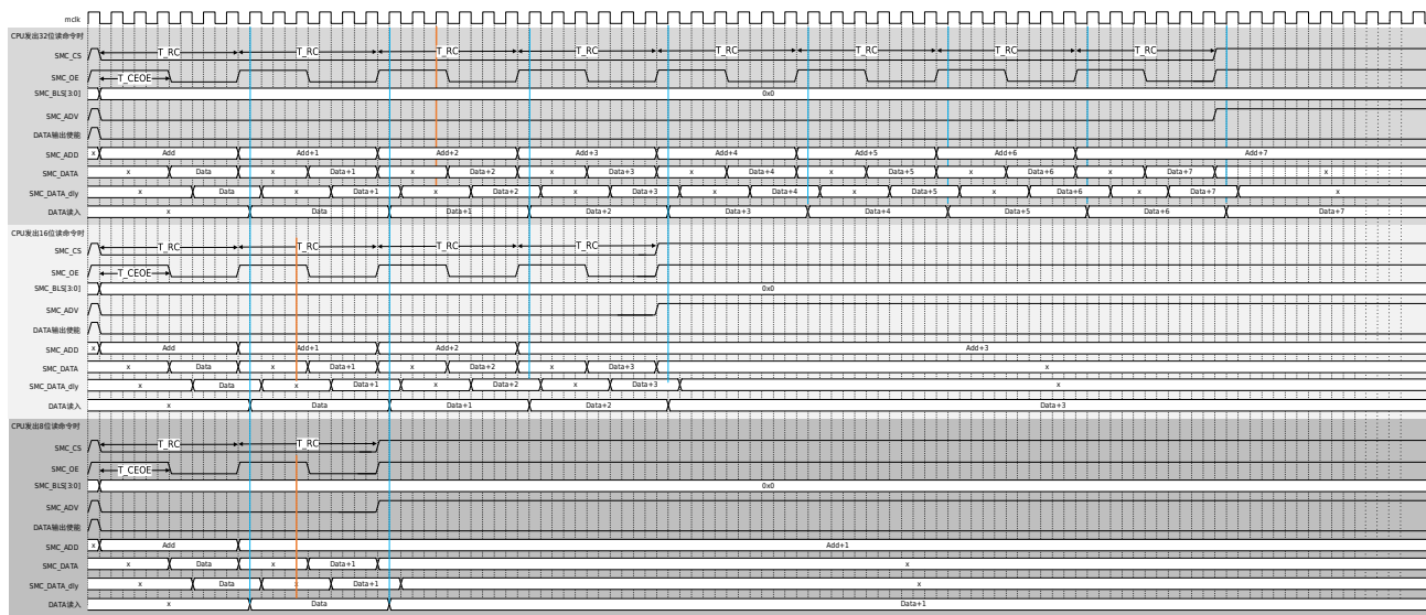
图 37-8 单次读动作基本时序（异步方式（RSYN=0）&16 位位宽（MW=01））
