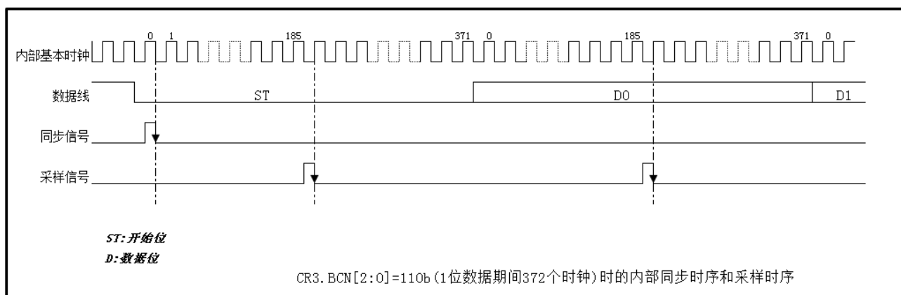
图 27-15 智能卡模式同步时序和采样时序图
