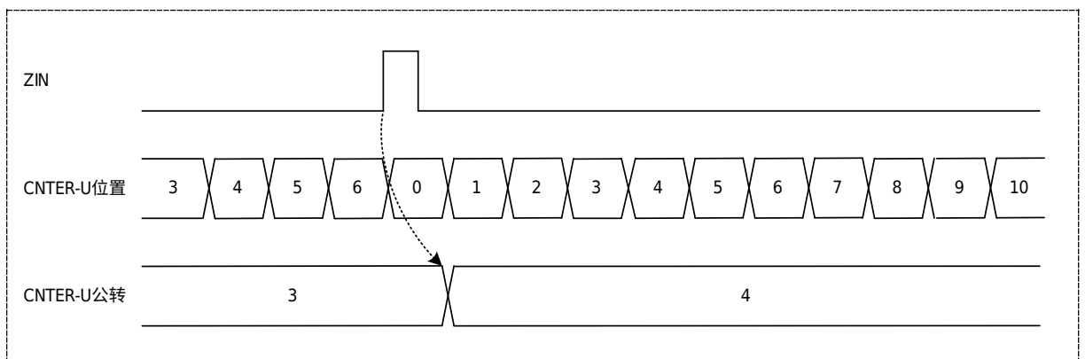
图 20-30 公转计数模式-Z 相计数
