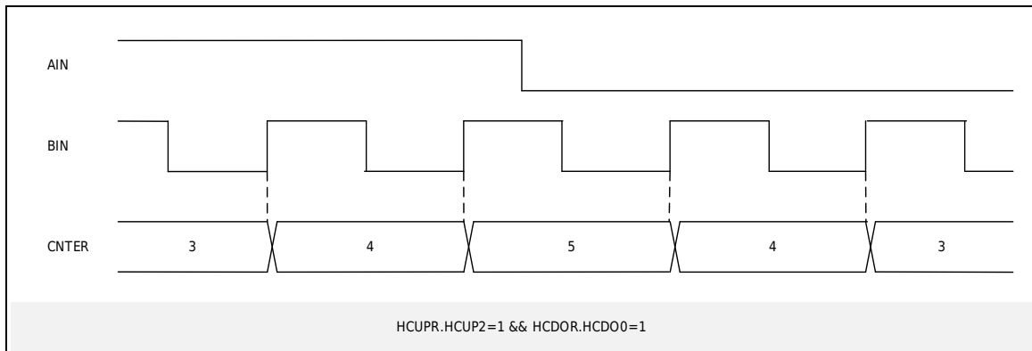
图 23-16 位置计数模式-方向计数
