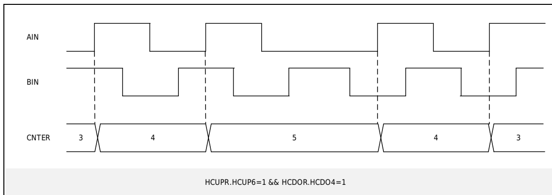
图 23-13 位置计数模式-相位差计数（1 倍计数）
