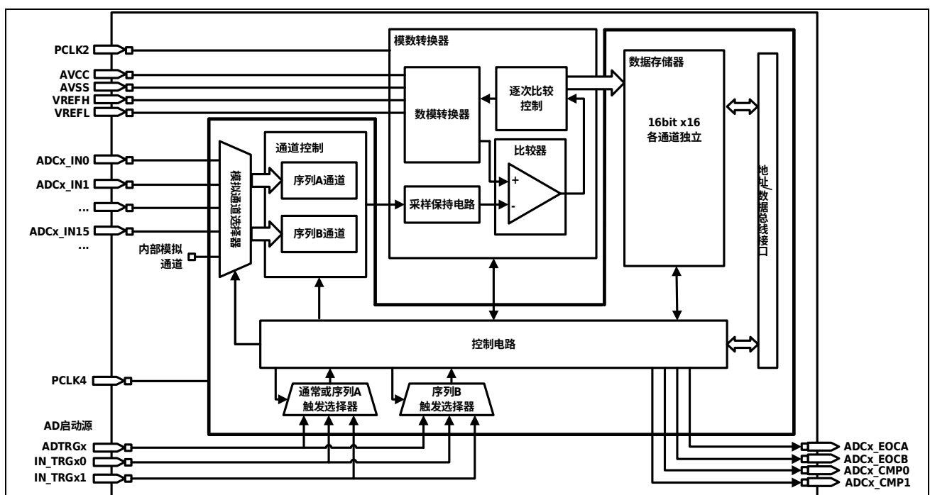
图 17-1 ADC 框图
