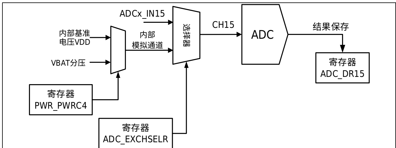
图 17-3 内部模拟通道选择
