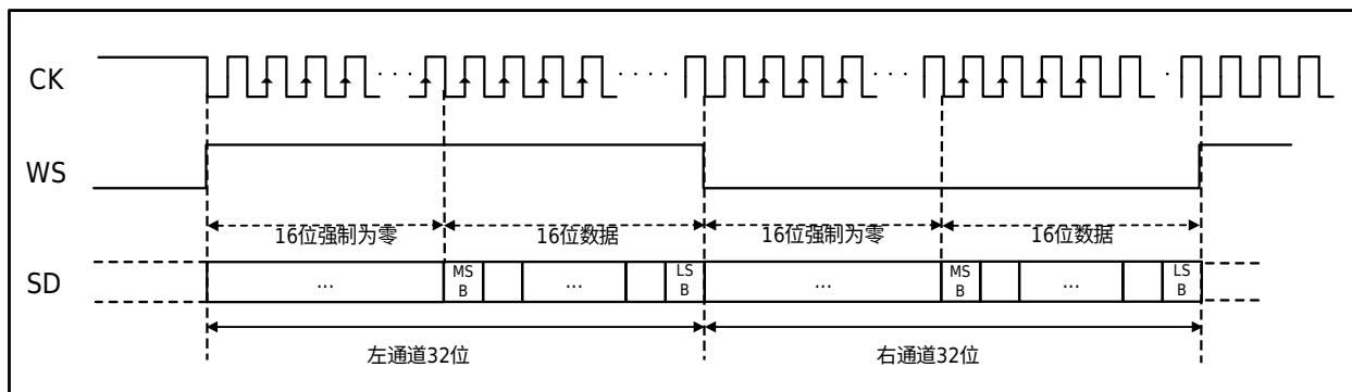
图 31-9 I2S LSB 协议波形（16 位数据封装在 32 位帧中）
