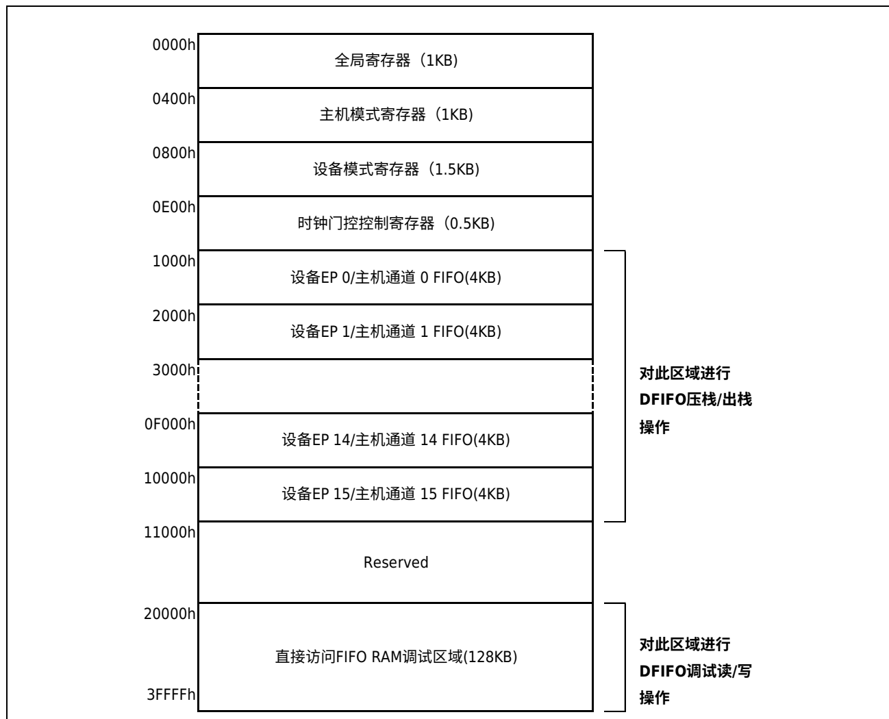
图 32-7 USBHS 控制状态寄存器存储器映射
