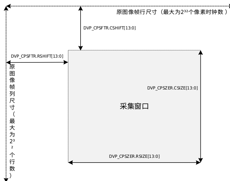
图 38-6 DVP 窗口设定图
