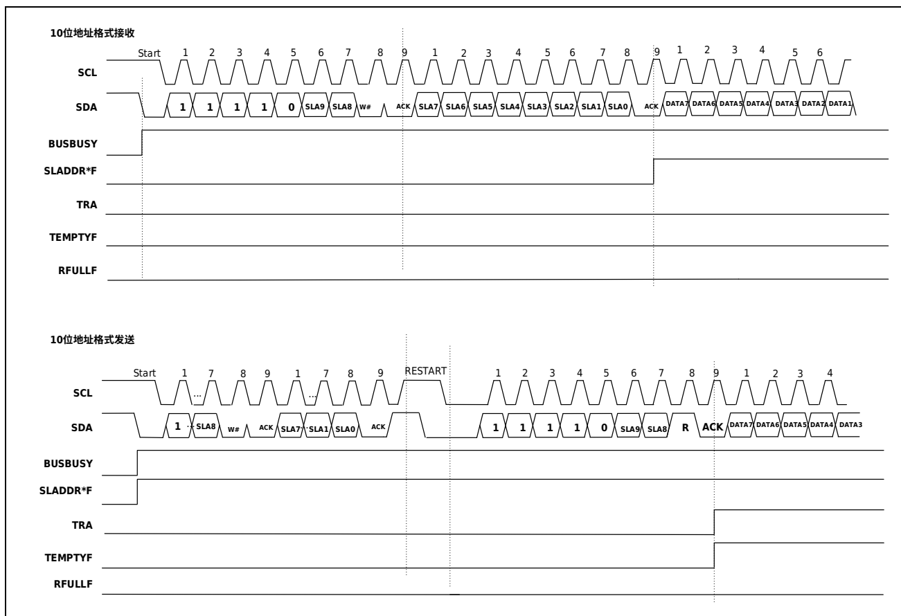
图 28-15 选择 10 位地址格式时的时序
