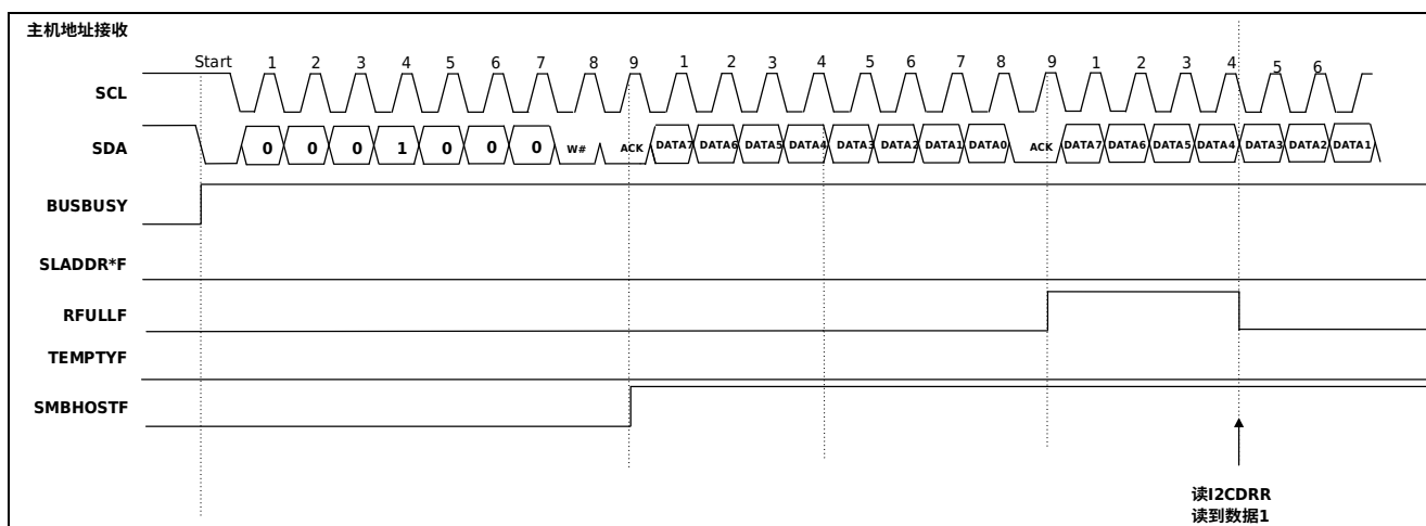
图 28-17 SMBus 主机地址接收时序图
