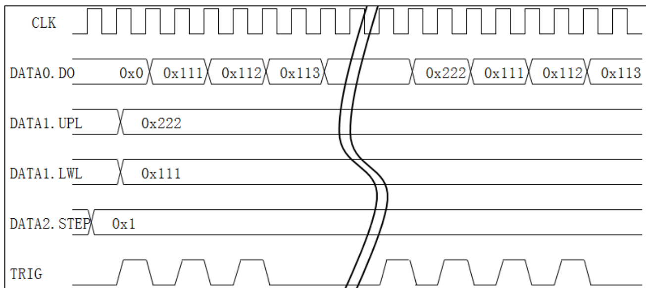
图 41-5 递增锯齿波输出示例时序图
