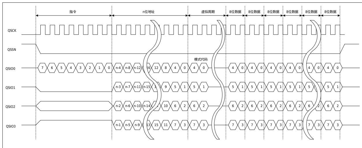
图 30-5 扩展式 SPI 协议动作示意图 2（四线式输入输出快速读模式）
