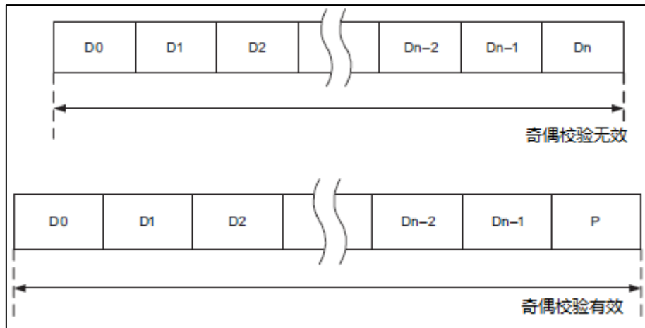
图 29-4 数据格式
