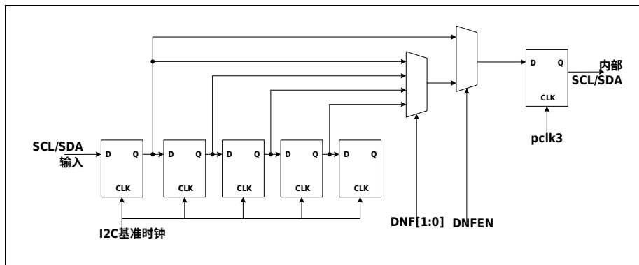
图 28-20 数字滤波电路框图
