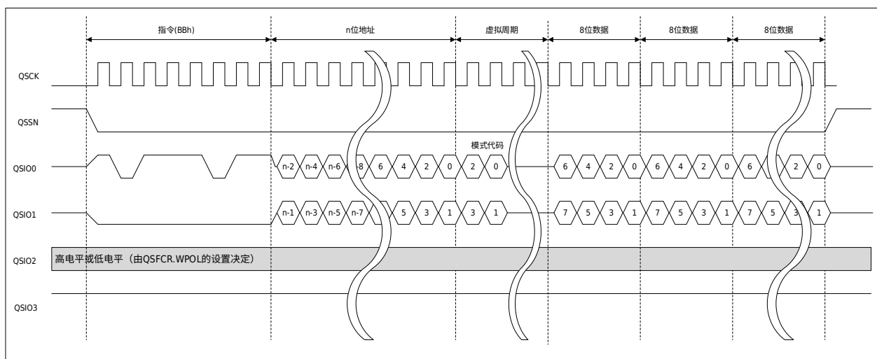
图 30-18 二线式输入输出快速读总线周期示意图
