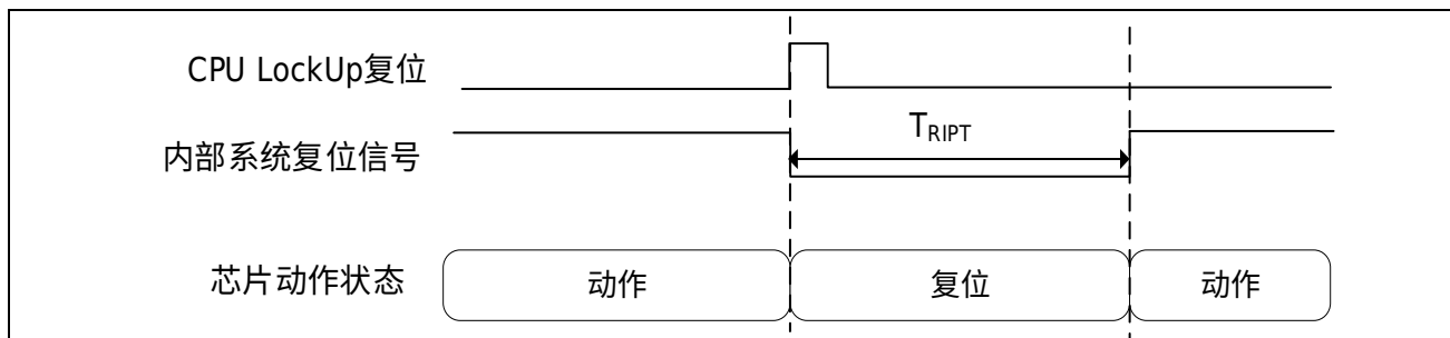
图 3-14 M4 Lockup 复位
