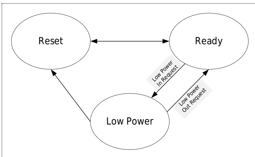
图 37-6 SMC 状态图
