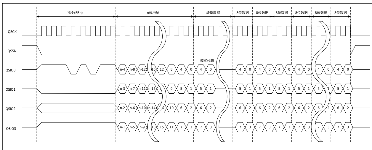
图 30-22 四线式输入输出快速读总线周期示意图
