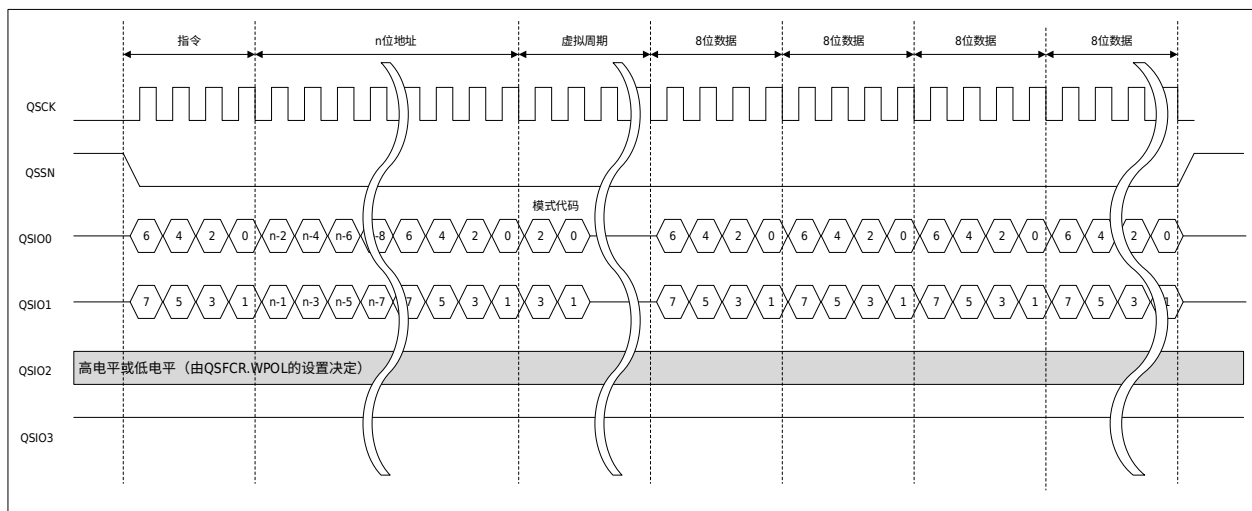
图 30-6 二线式 SPI 协议动作示意图（快速读模式）
