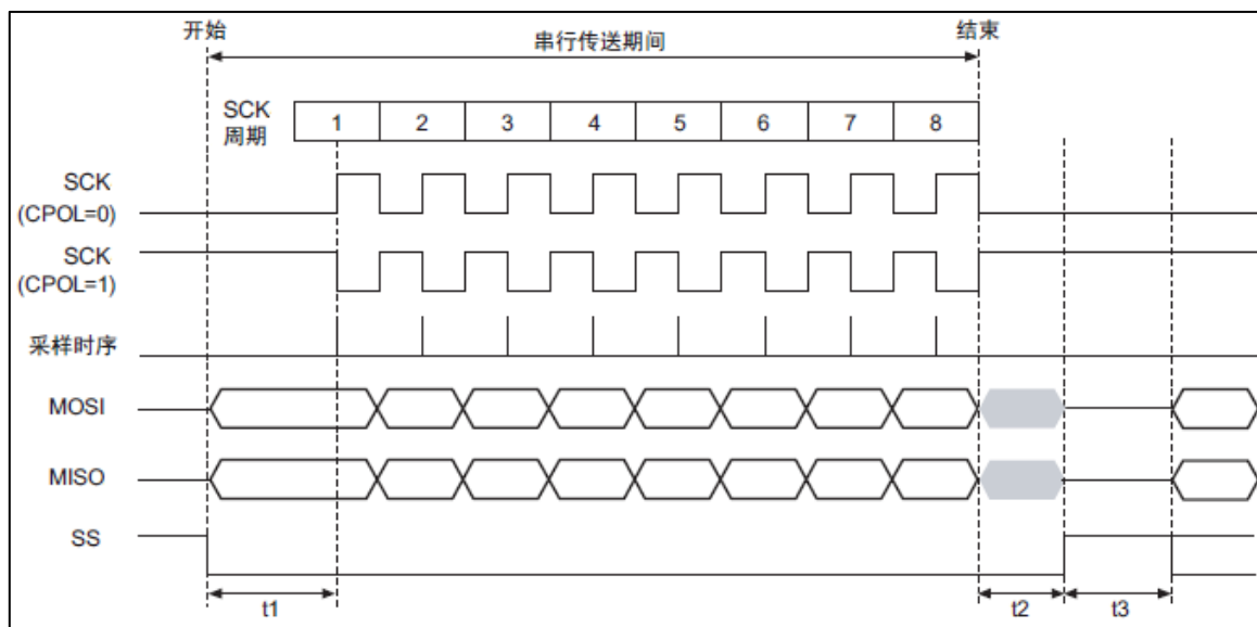
图 29-5 数据传送格式图 (CPHA=0)
