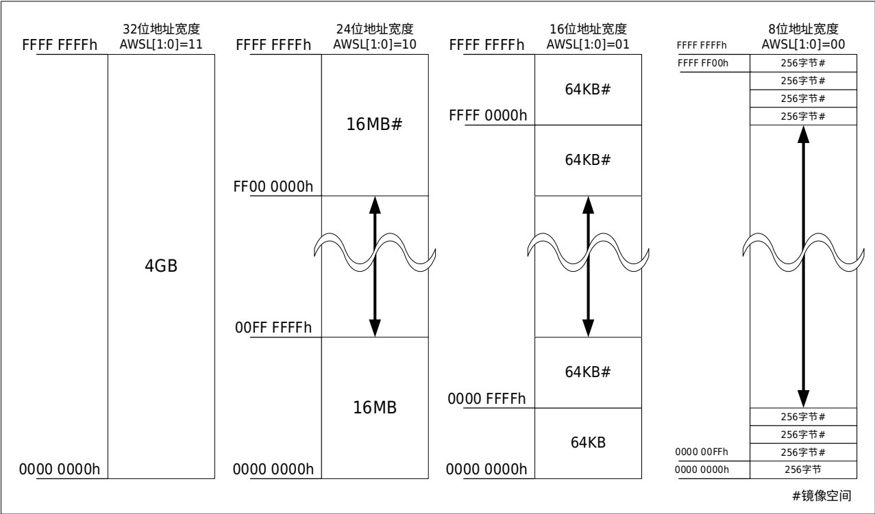
图 30-3 QSPI-ROM 空间内存映像图
