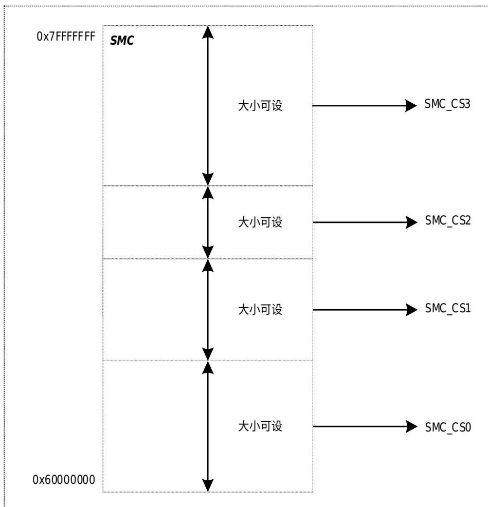
图 37-3 SMC 的地址空间划分
