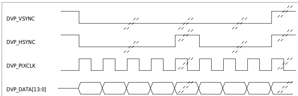
图 38-2 DVP 信号波形示意图
