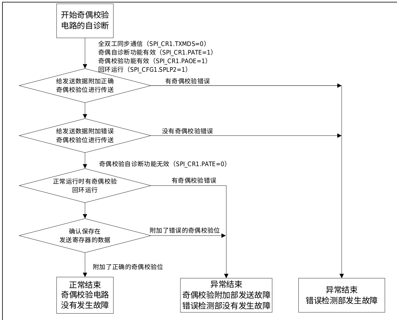
图 29-9 奇偶校验流程
