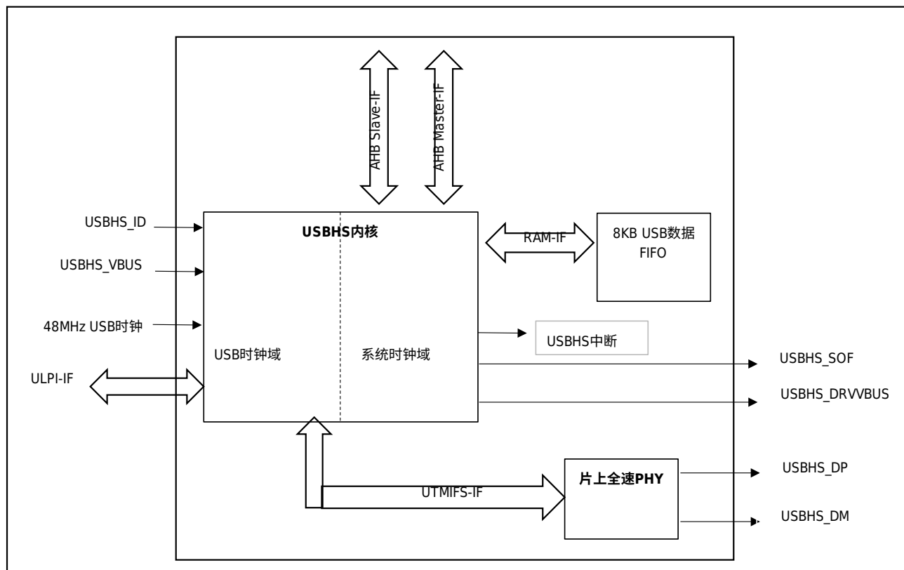
图 32-1 USBHS 系统框图
