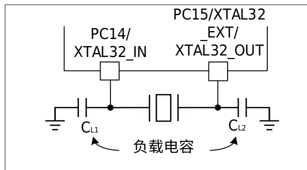
图 4-7 外部低速振荡器连接示例
