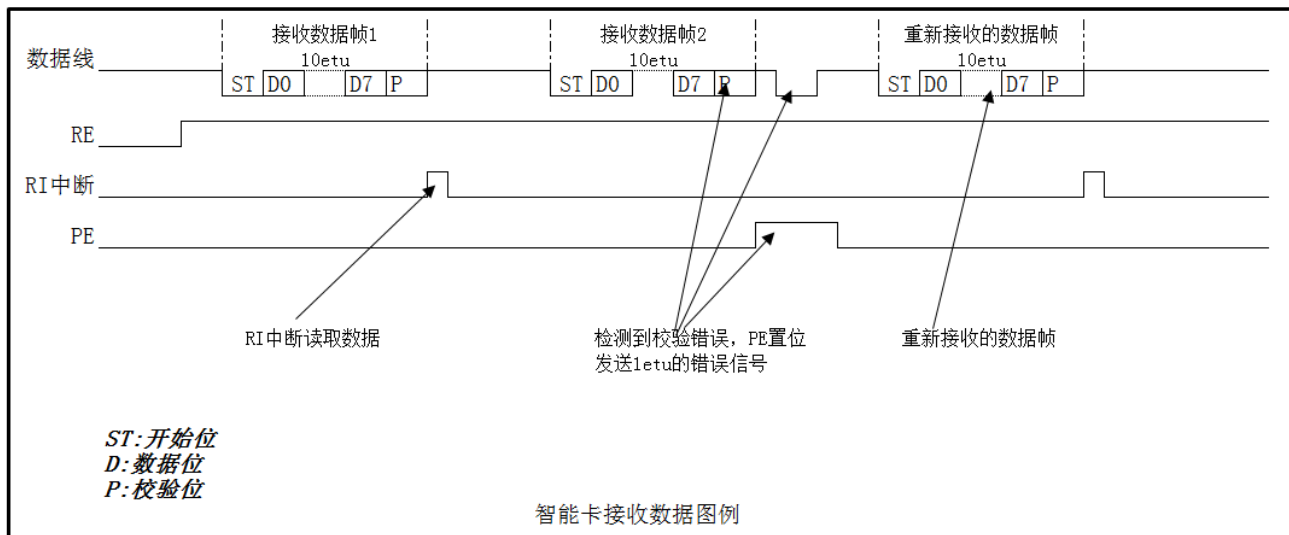
图 27-18 智能卡模式接收数据图例
