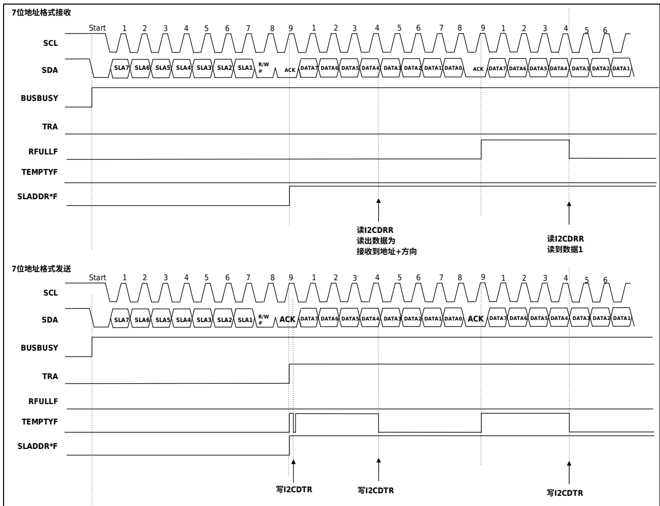
图 28-14 选择 7 位地址格式时的时序
