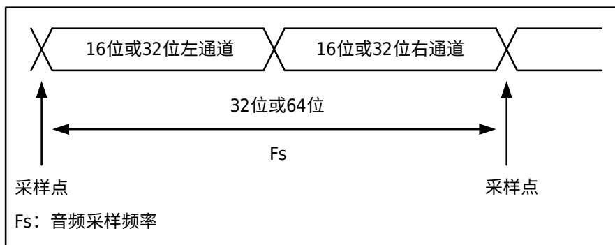
图 31-14 音频采样频率定义
