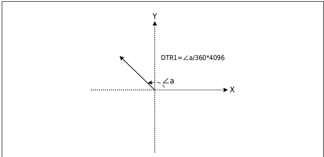
图 42-1 正弦运算角度值示意图
