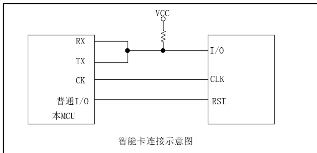
图 27-14 智能卡连接示意图
