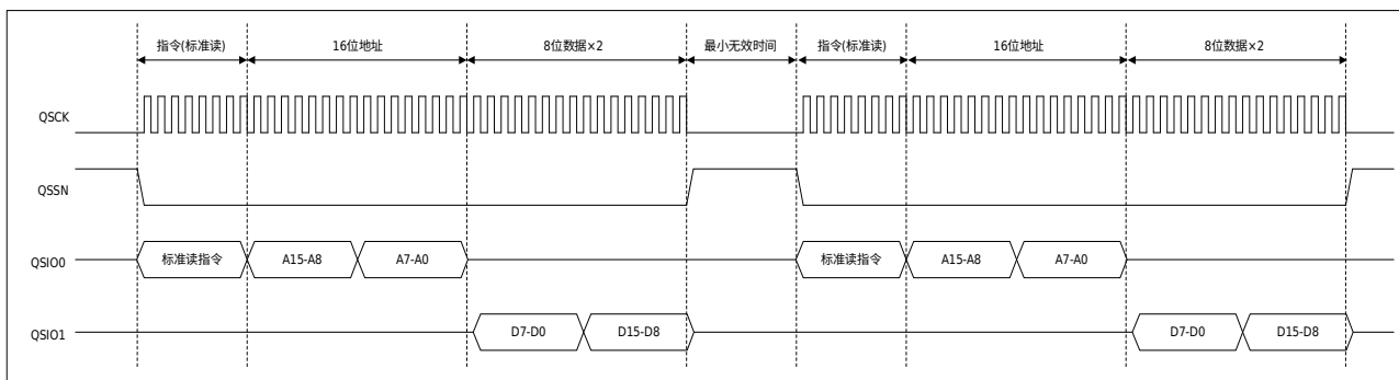
图 30-30 独立转换的单一闪存数据读取操作示意图
