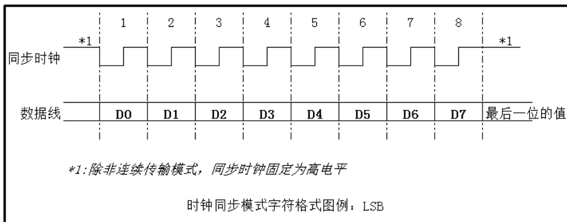
图 27-19 时钟同步模式数据格式
