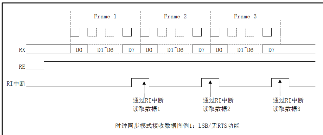
图 27-22 时钟同步模式接收数据图例 1
