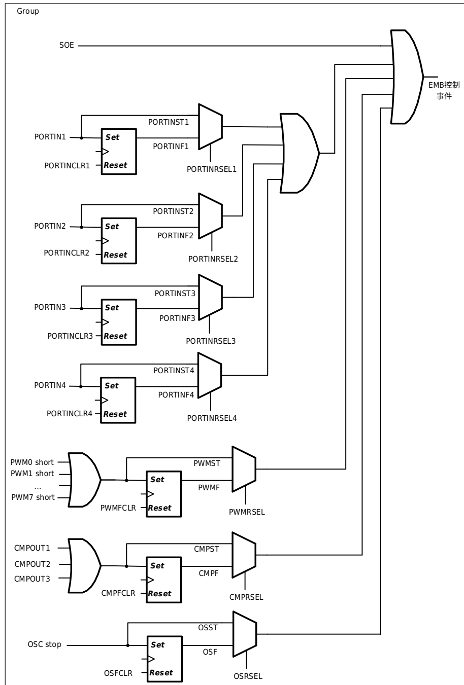
图 22-2 EMB 组群控制
