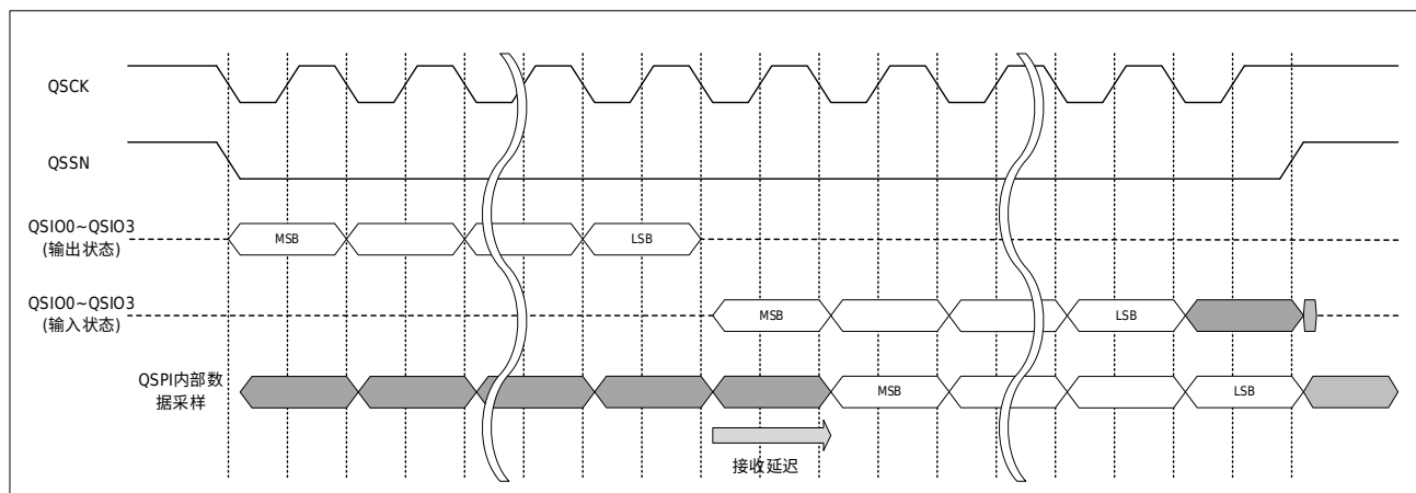
图 30-12 数据接收延迟示意图
