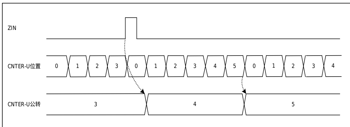
图 23-19 公转计数模式-混合计数
