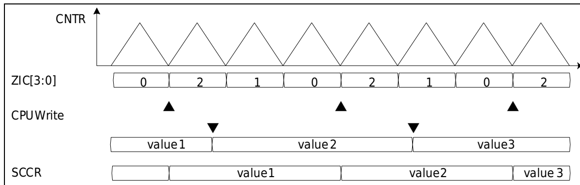
图 21-15 SCCR 缓冲传输操作（周期间隔响应链接传输使能时）
