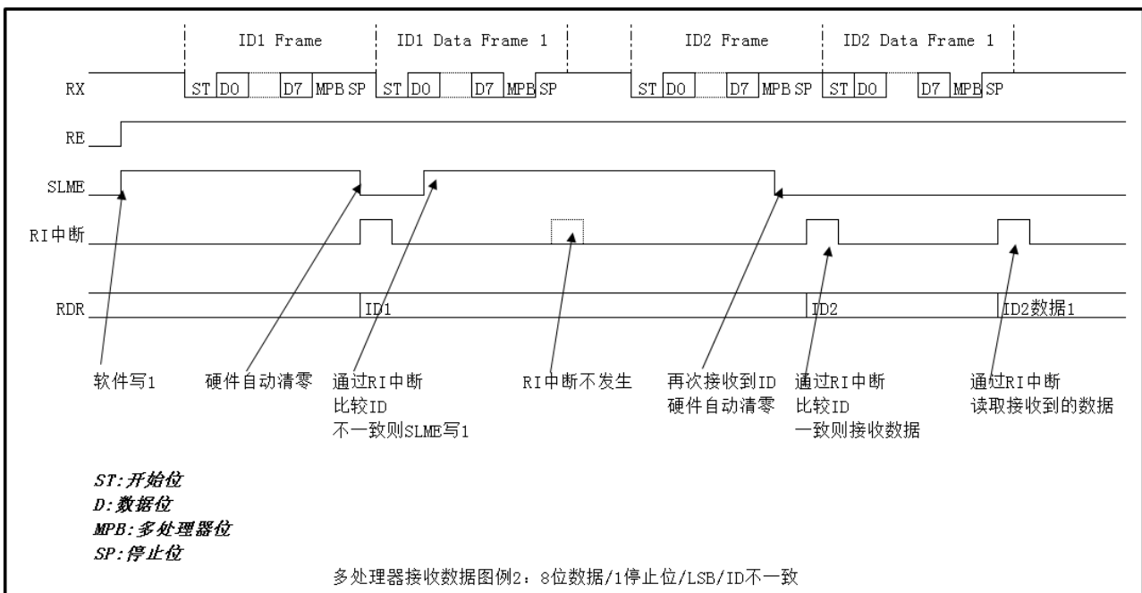
图 27-12 多处理器模式接收数据图例 2
