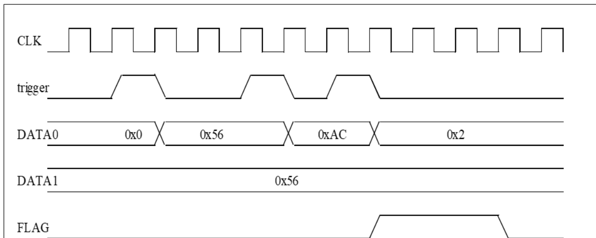
图 41-1 硬件触发启动加模式示例时序图
