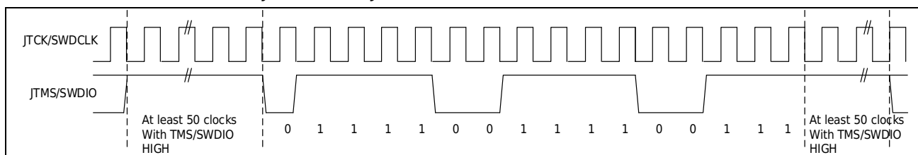
图 44-3 JTAG-DP 到 SW-DP 切换时序
