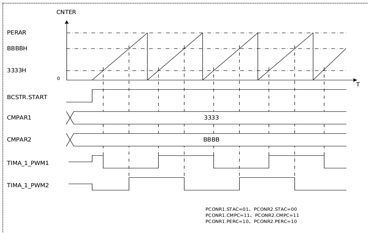
图 23-4 比较输出动作
