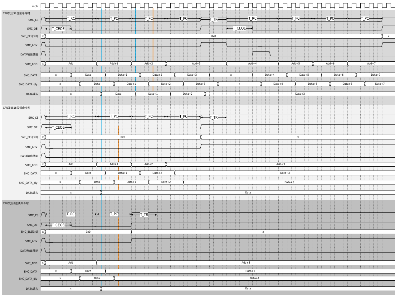
图 37-20 地址数据非复用突发读动作基本时序（同/异步方式（RSYN=1/0）&16 位位宽（MW=01）&RBL=001）
