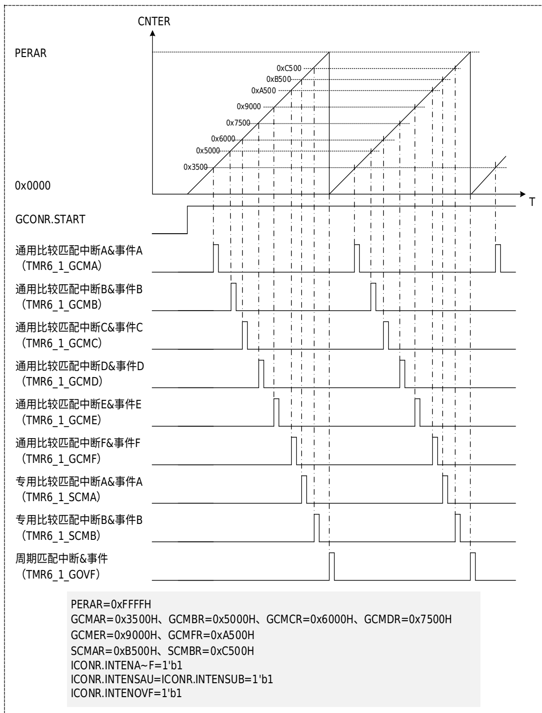
图 20-35 锯齿波模式时中断&事件输出例
