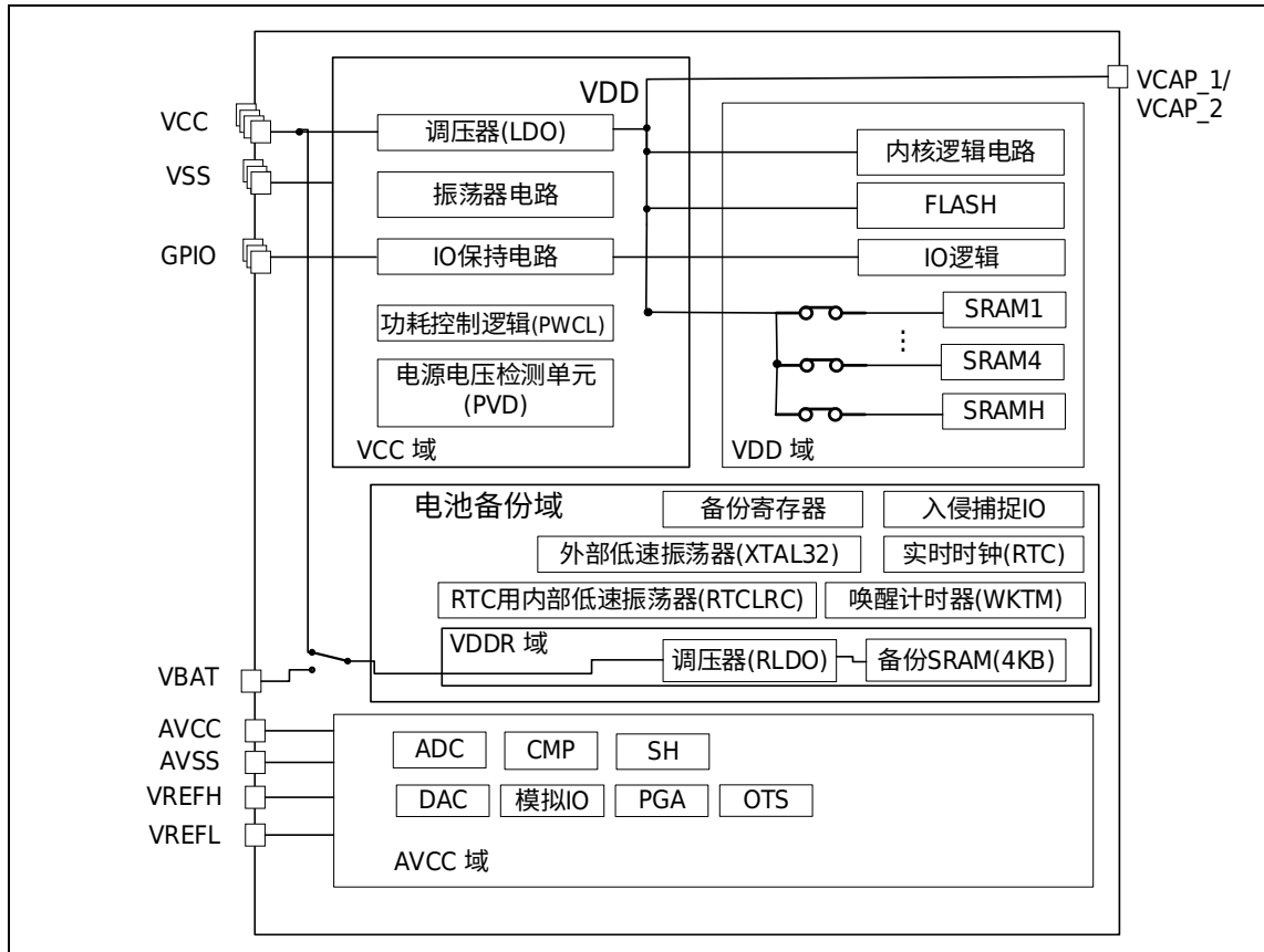
图 5-1 电源构成图
