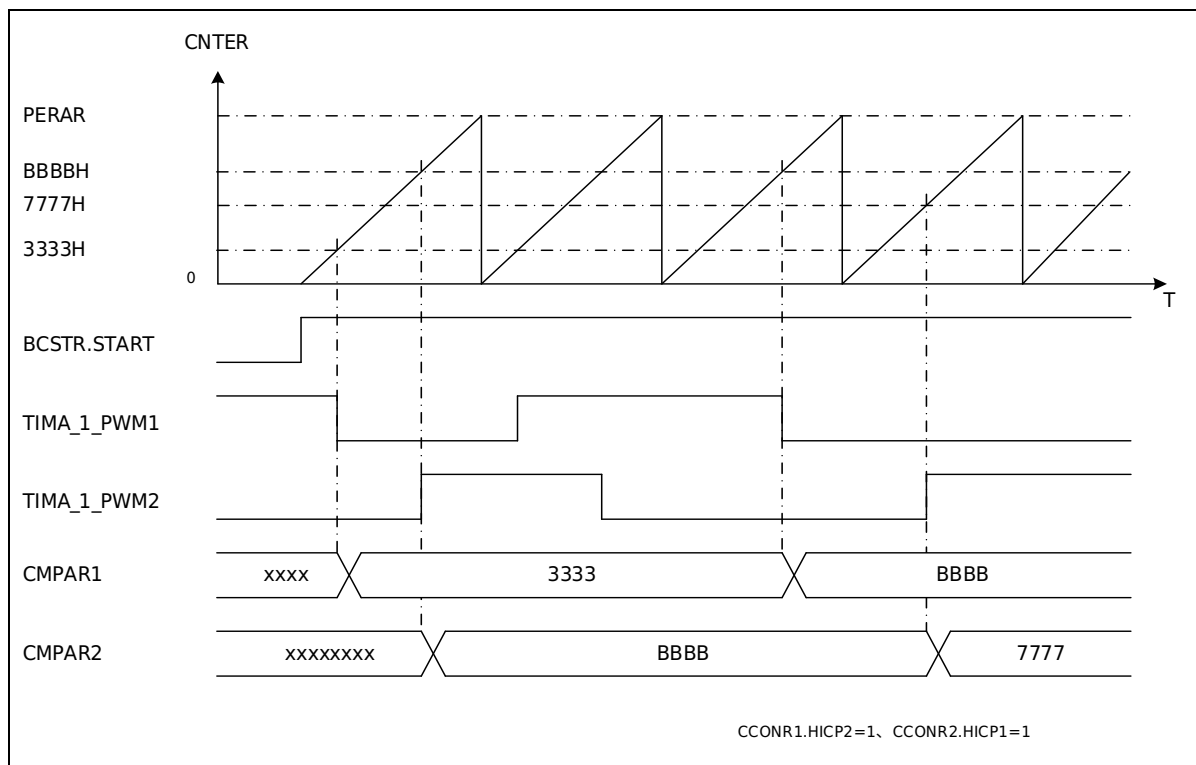
图 23-5 捕获输入动作
