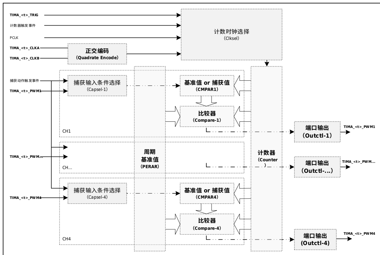
图 23-1 TimerA 基本框图
