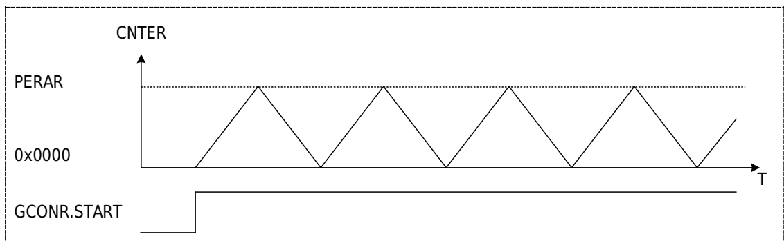
图 20-3 三角波波形
