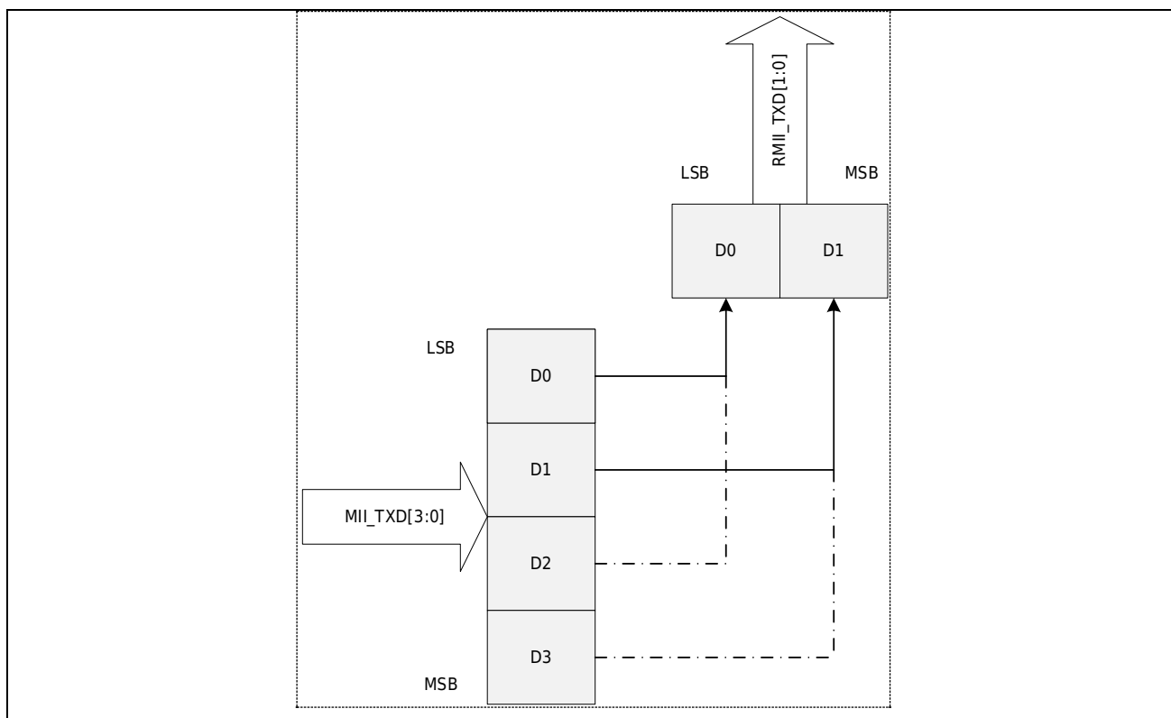
图 36-6 MII/RMII 发送位序
