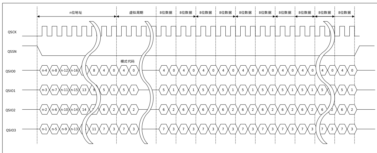
图 30-29 选择 XIP 模式的自定义快速读总线周期示意图
