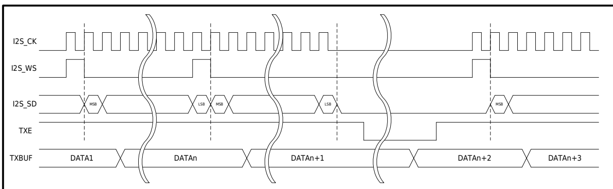
图 31-17 PCM 短帧主机发送暂停后重新发送方式一
