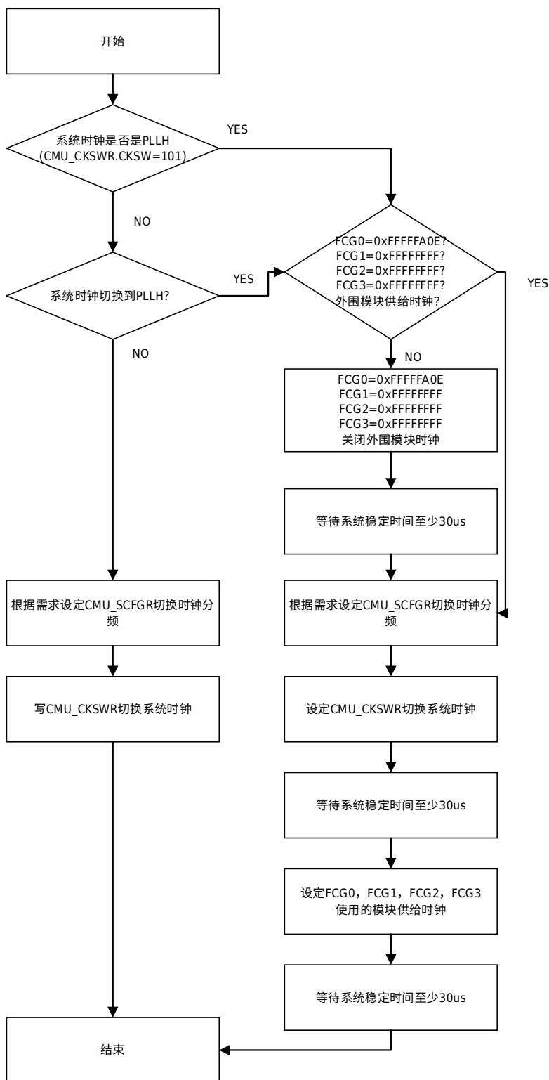
图 4-9 时钟源切换
