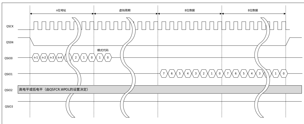
图 30-15 选择 XIP 模式的快速读总线周期示意图
