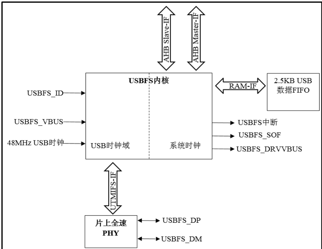
图 33-1 USBFS 系统框图
