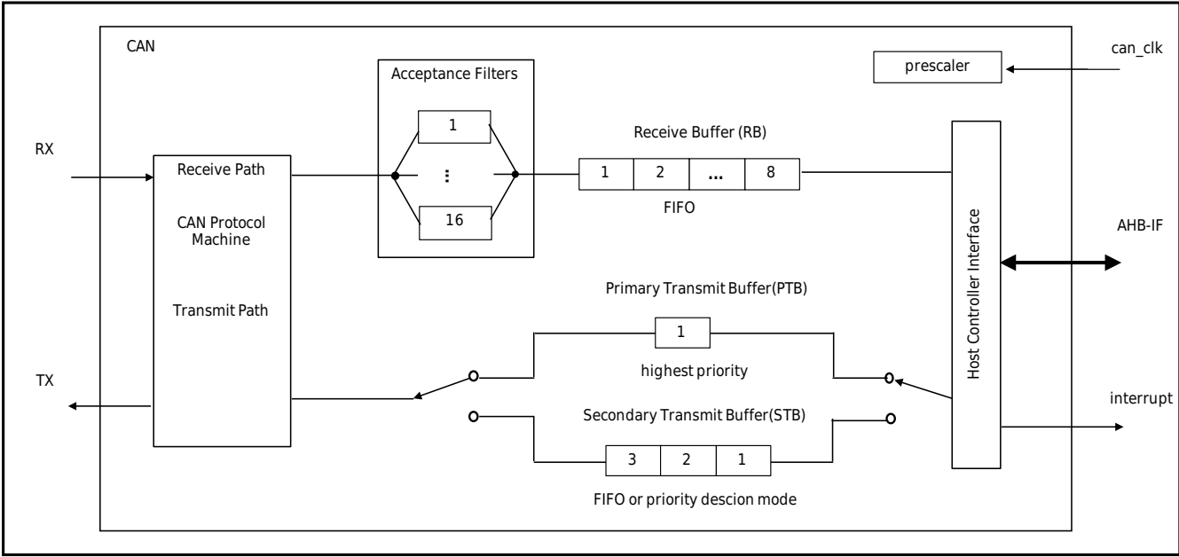
图 34-1 CAN 系统框图
