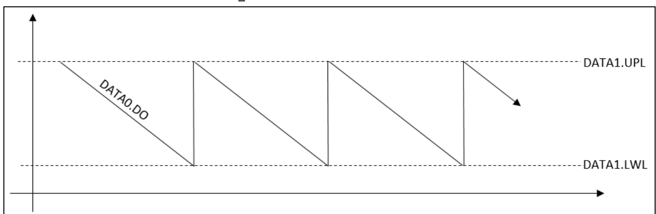
图 41-6 递减锯齿波输出模式
