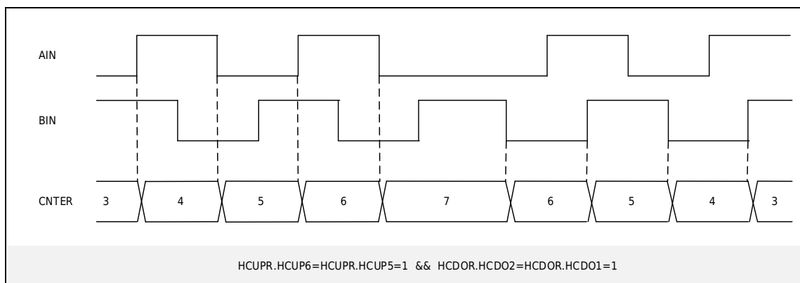
图 23-14 位置计数模式-相位差计数（2 倍计数）
