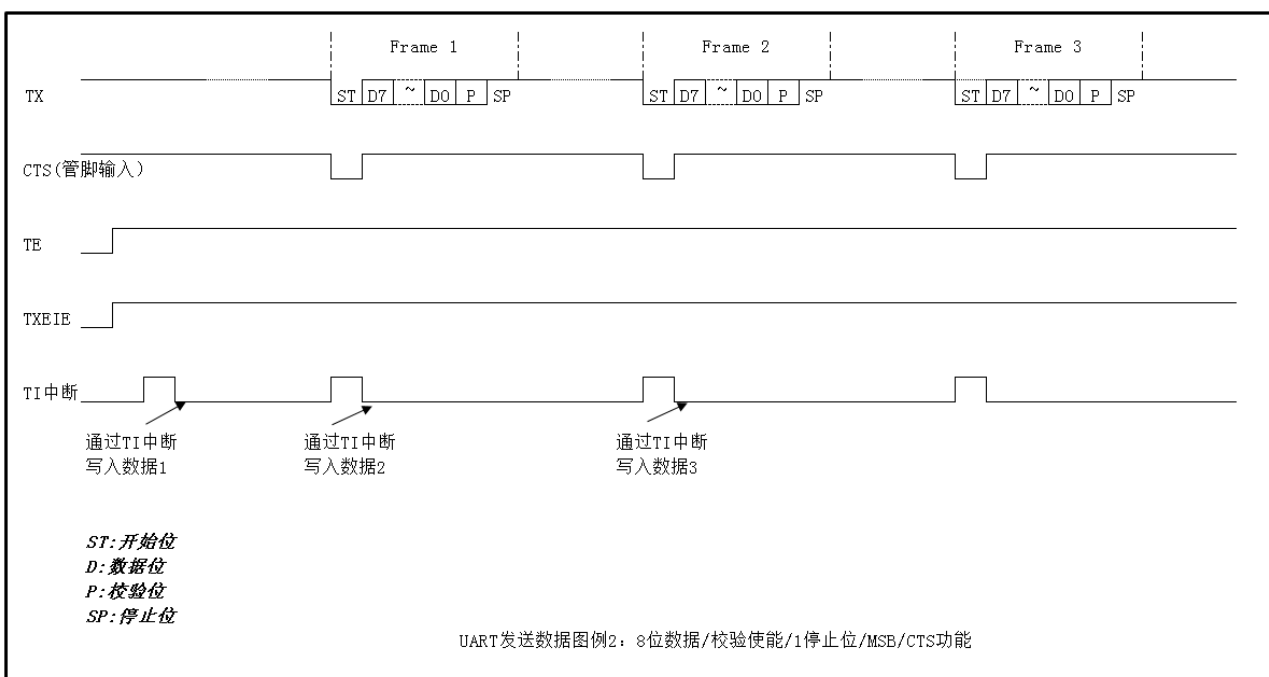
图 27-4 UART 发送数据图例 2
