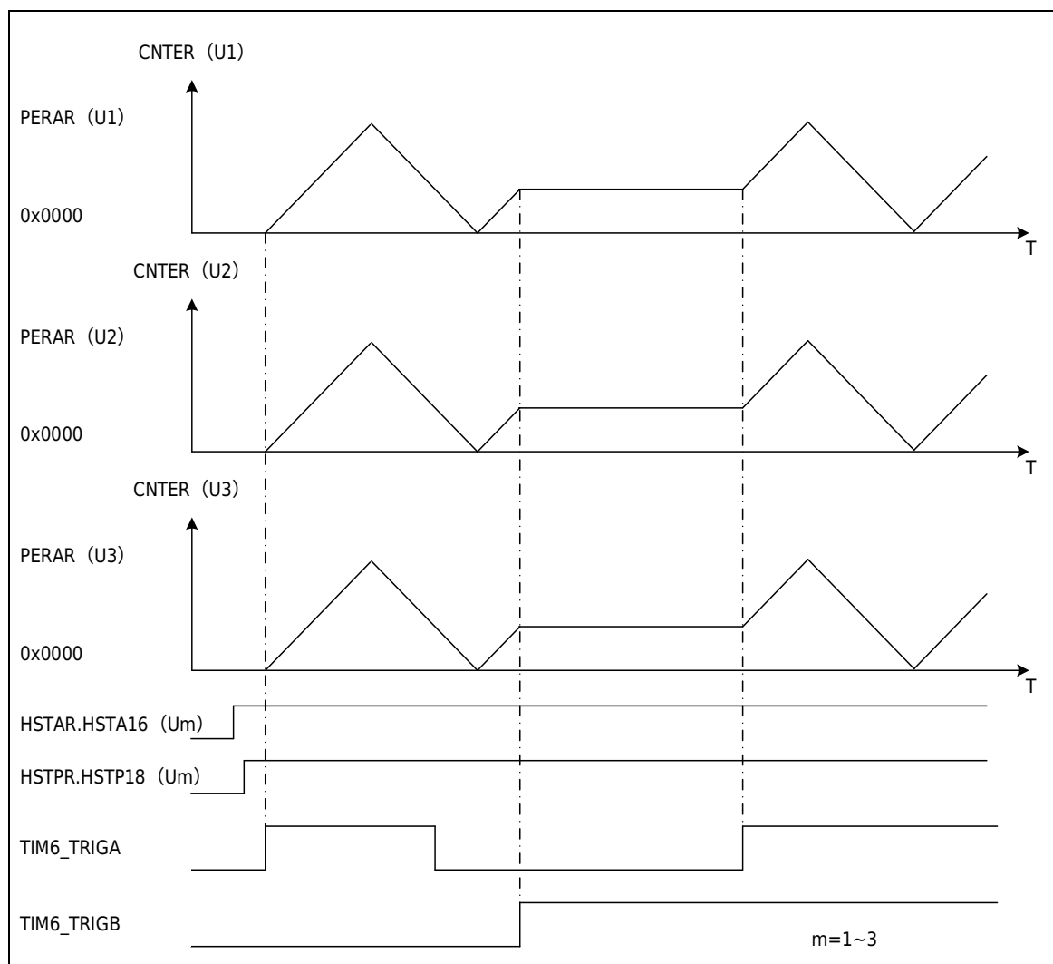
图 20-8 硬件同步动作
