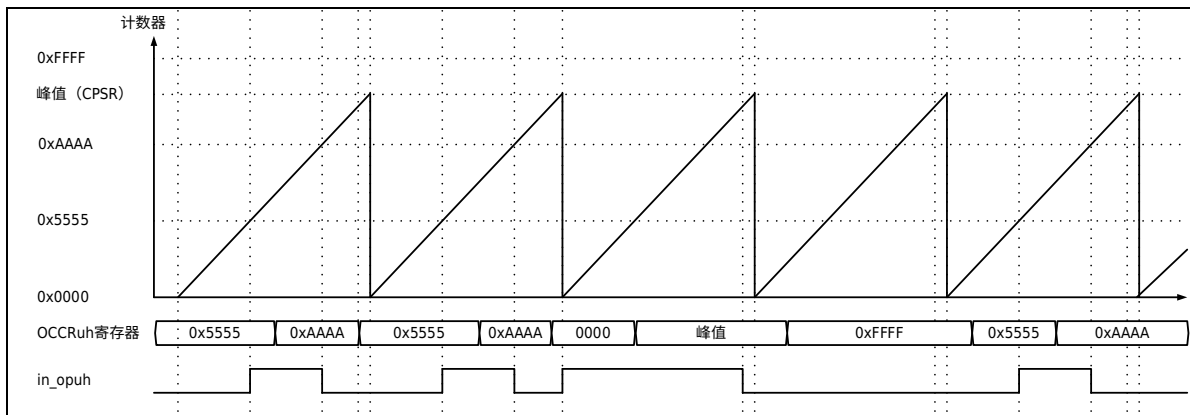
图 21-6 锯齿波模式波形输出例
