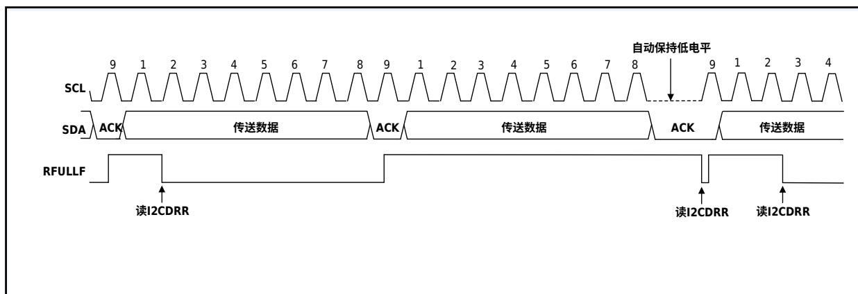
图 28-12 从机接收时序图
