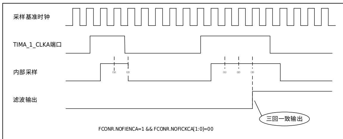
图 23-7 时钟输入端口的滤波功能
