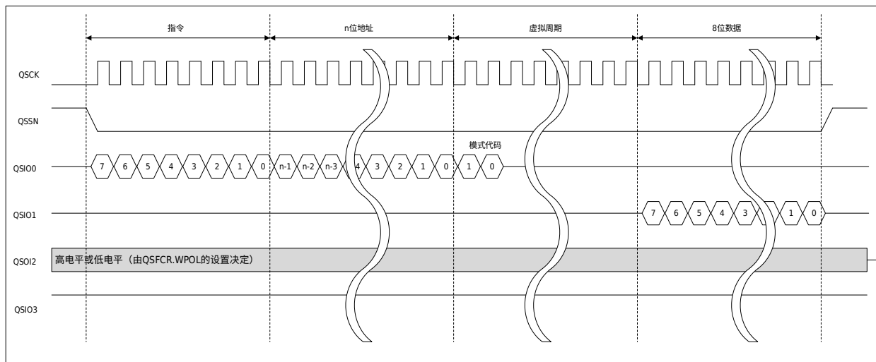
图 30-4 扩展式 SPI 协议动作示意图 1（快速读模式）
