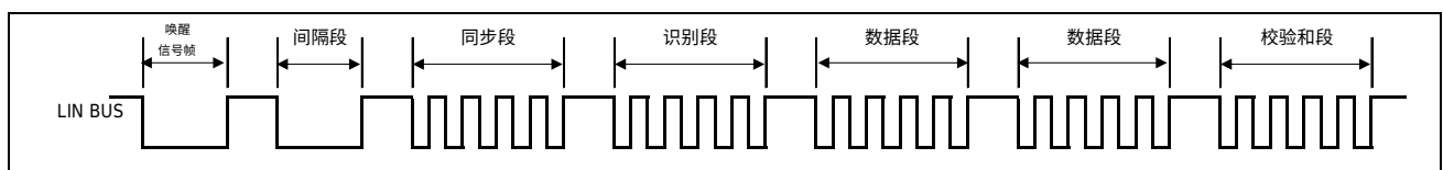
图 27-13 LIN 总线数据行为
