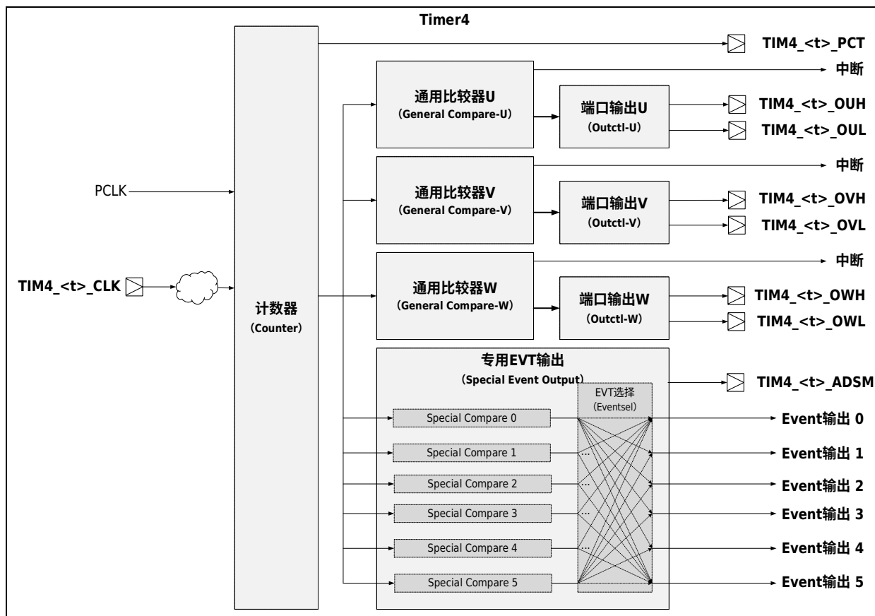
图 21-1 Timer4 基本框图
