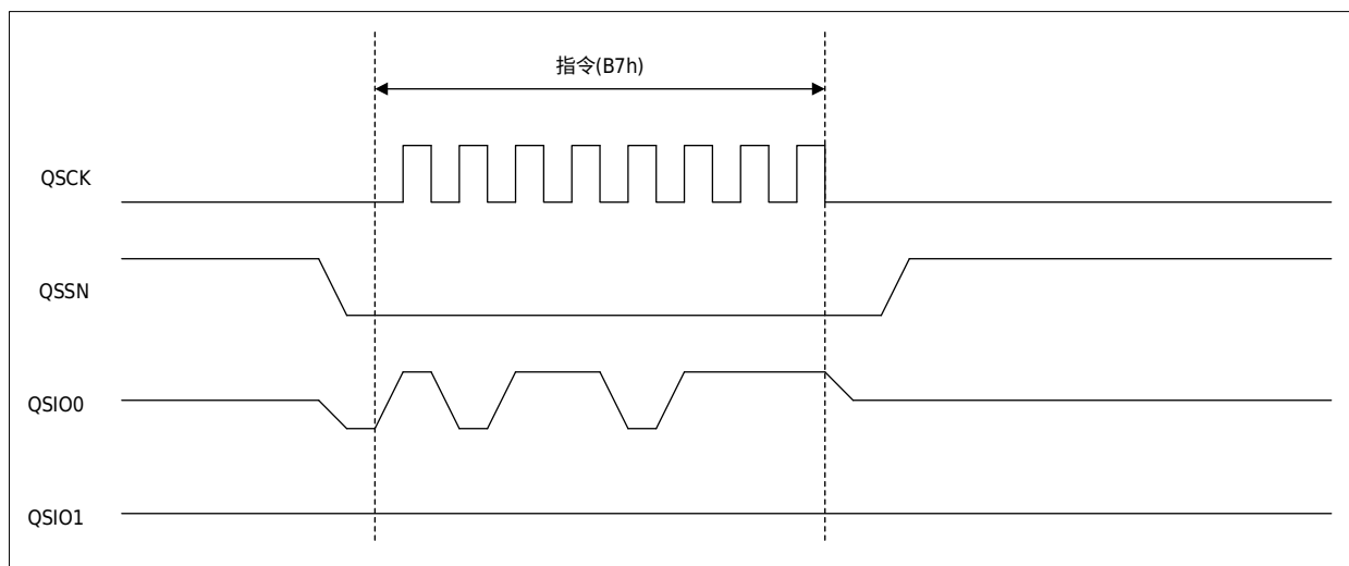
图 30-24 进入 4-Byte 模式指令总线周期示意图
