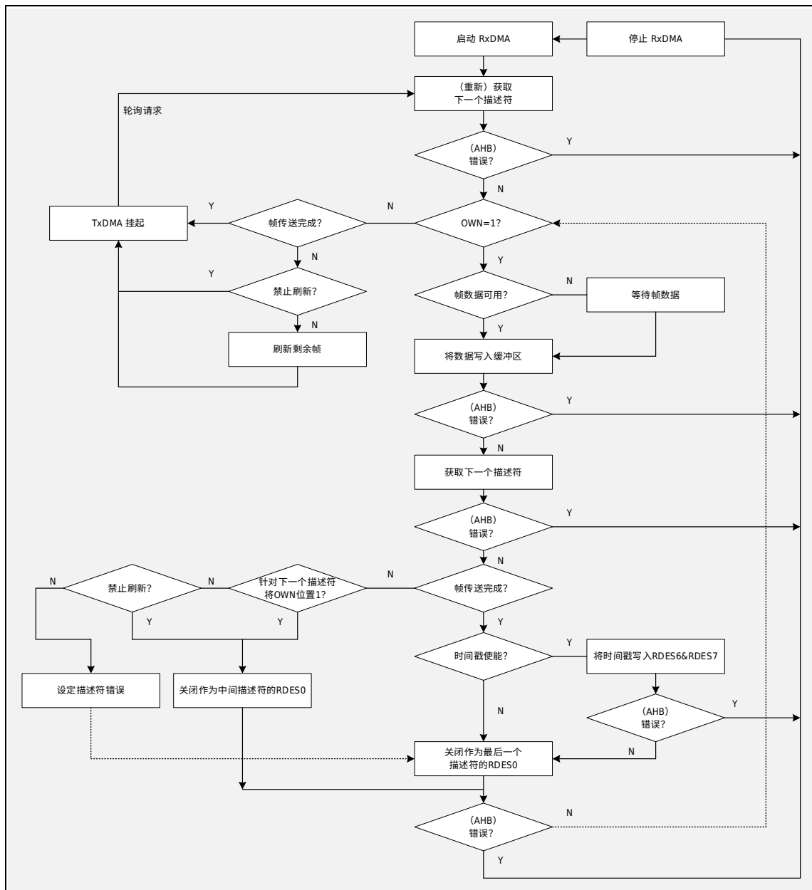
图 36-20 RxDMA 动作流程
