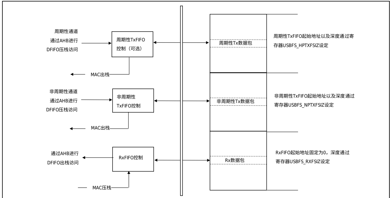
图 33-5 USBFS 主机模式下 FIFO 架构示意图
