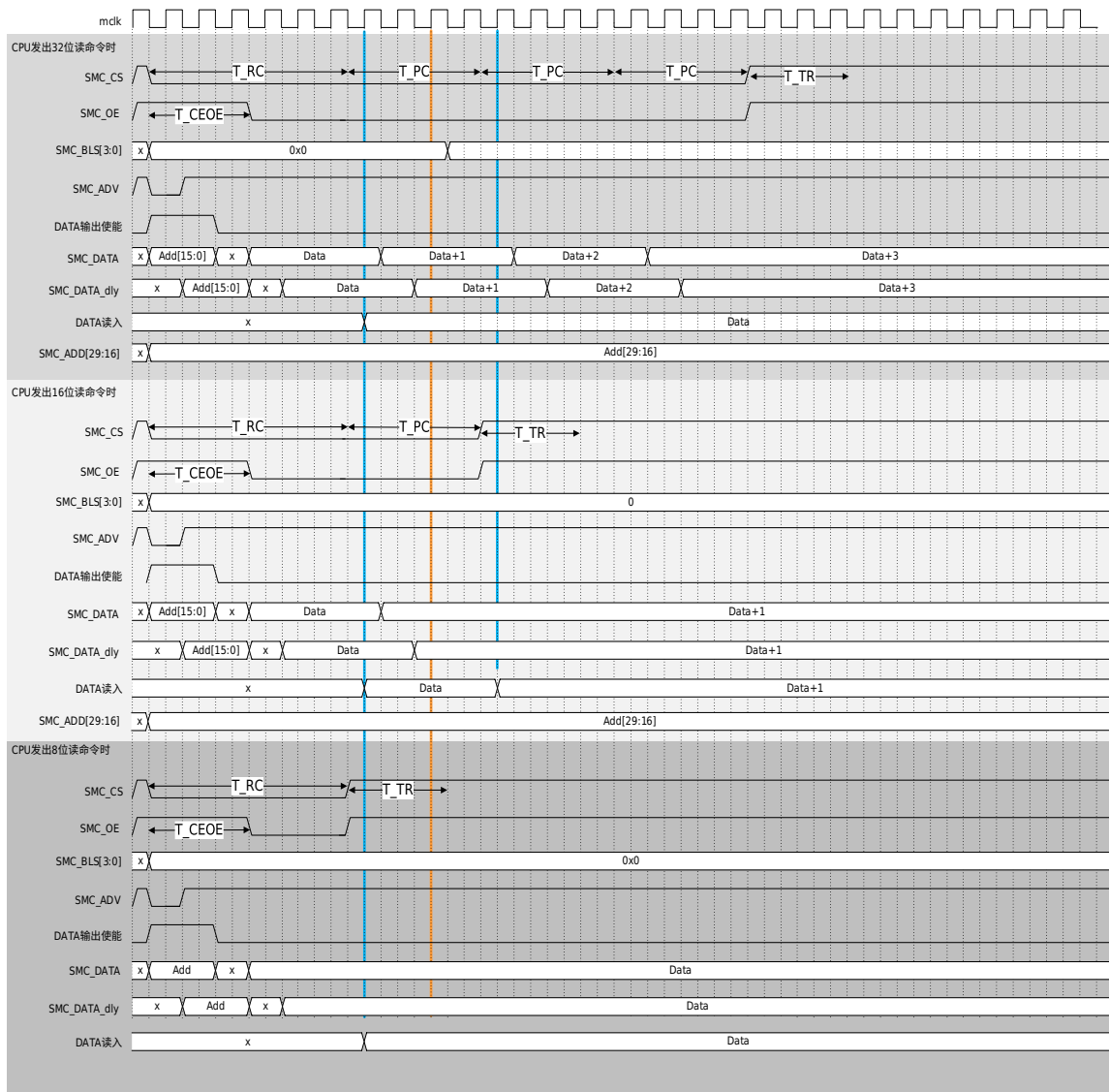
图 37-21 地址数据复用突发读动作基本时序（同/异步方式（RSYN=1/0）&32 位位宽（MW=10）&RBL=001）
