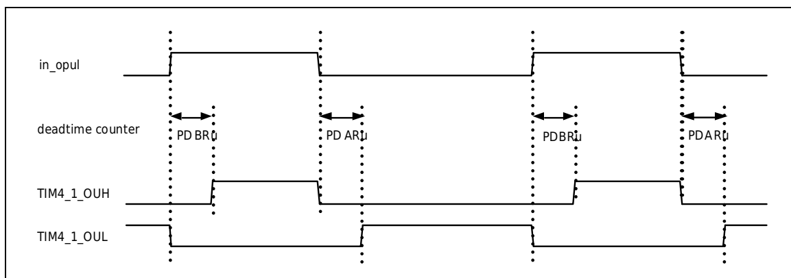
图 21-20 死区定时器模式下的互补 PWM 输出
