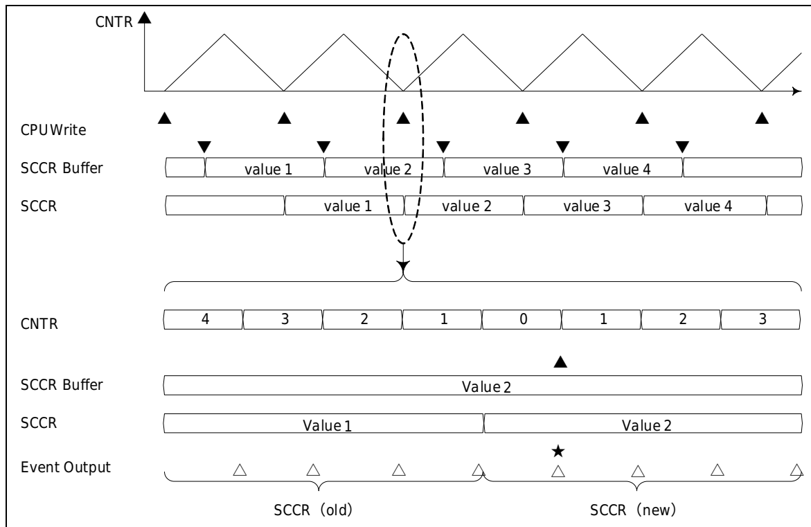
图 21-14 SCCR 缓冲传输操作（周期间隔响应链接传输禁止时）
