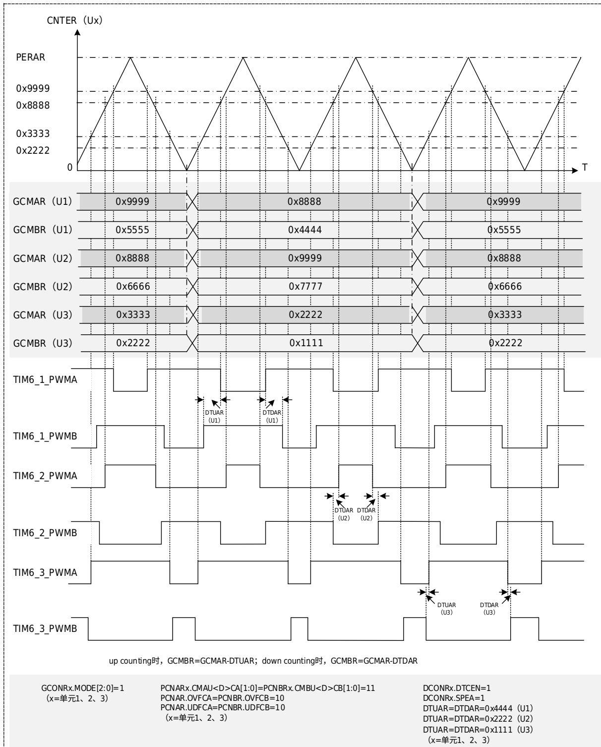
图 20-23 带死区时间 3 相双边对称互补 PWM
