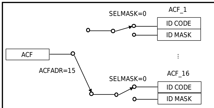
图 34-5 CAN ACF 寄存器访问筛选器组示意图
