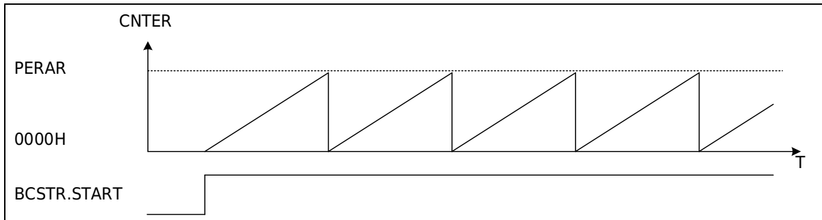
图 23-2 锯齿波波形（递增计数）
