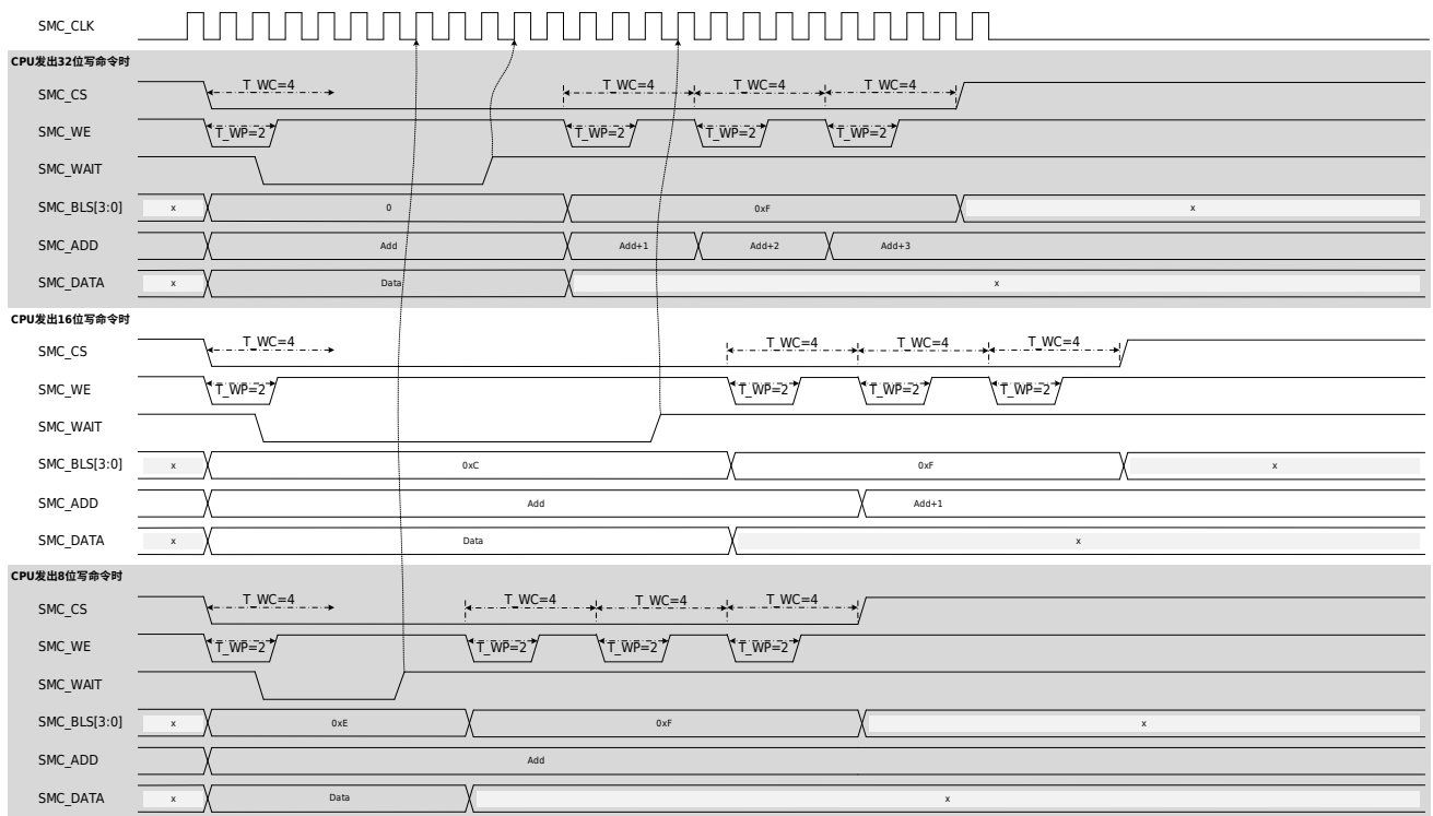
图 37-17 单次写动作基本时序（同步方式（WSYN=1）&32 位位宽（MW=10）&BLS=0）
