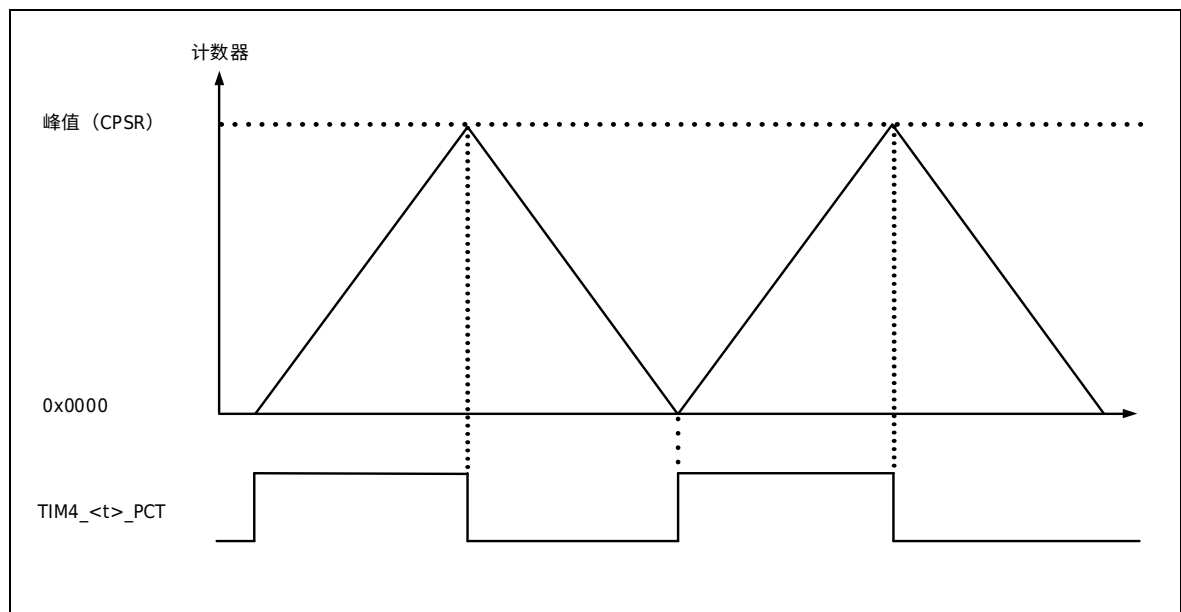
图 21-25 计数方向信号输出示例
