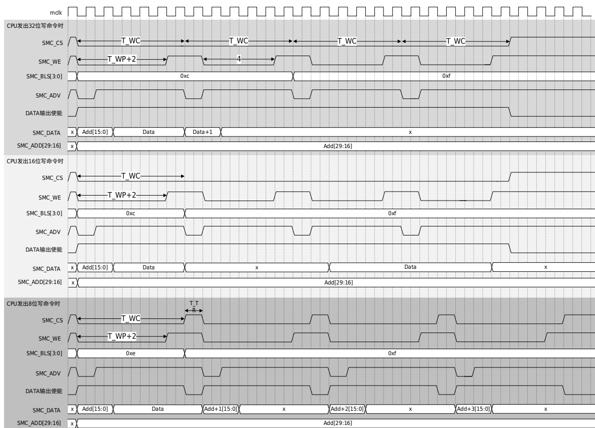
图 37-23 地址数据复用突发写动作基本时序（异步方式（WSYN=0）&16 位位宽（MW=01） &WBL=001&BLSS=0）
