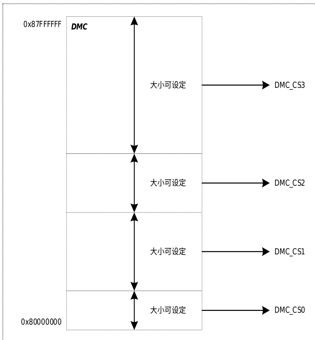
图 37-4 DMC 的地址空间划分
