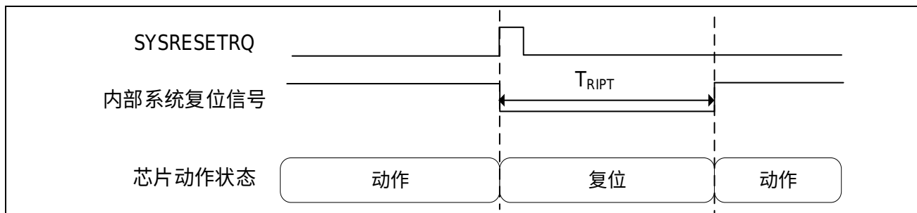
图 3-8 软件复位
