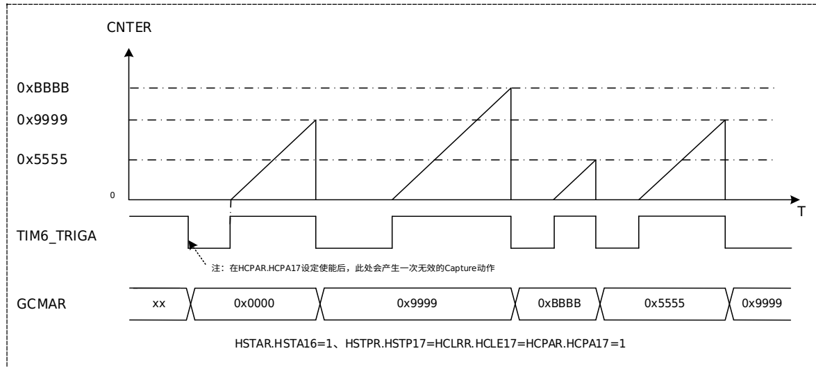
图 20-9 脉宽测量
