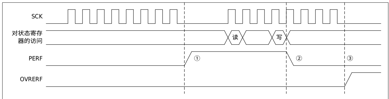
图 29-13 奇偶校验错误
