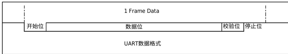
图 27-2 UART 数据格式
