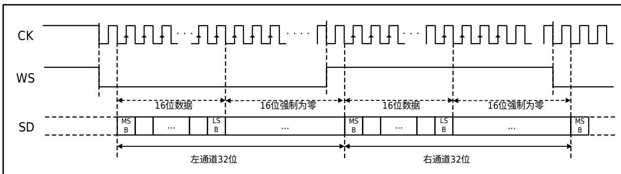
图 31-3 I2S Philips 协议波形 (16 位数据封装在 32 位帧中)
