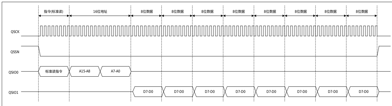
图 30-31 预读取功能有效时数据读取操作示意图
