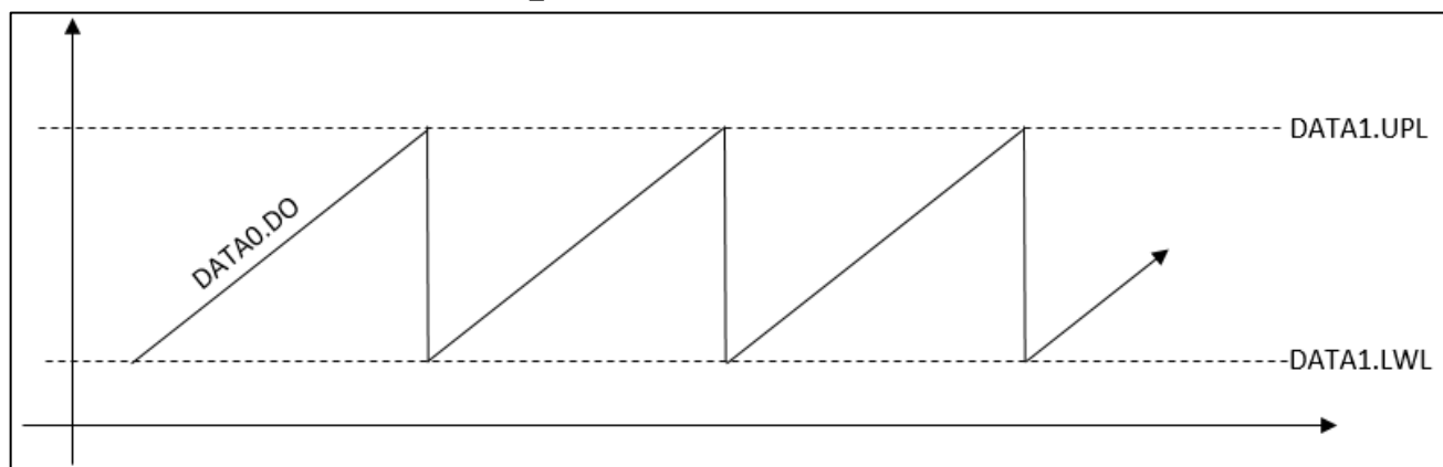
图 41-4 递增锯齿波输出模式
