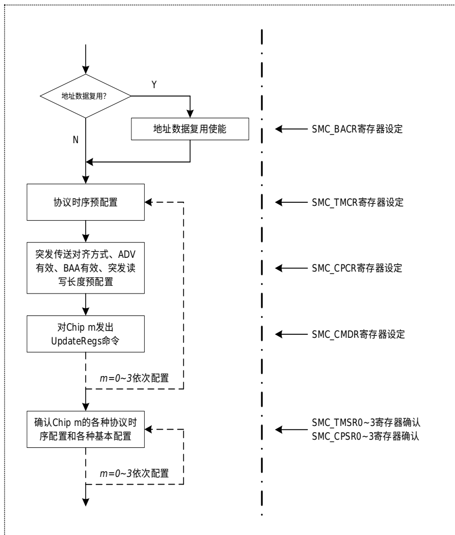
图 37-7 SMC 初始设定流程
