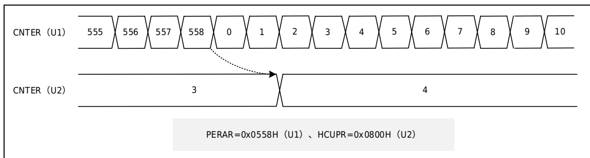
图 23-9 32 位级联计数动作
