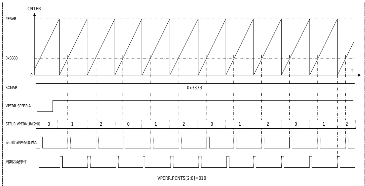
图 20-24 周期间隔有效请求信号动作
