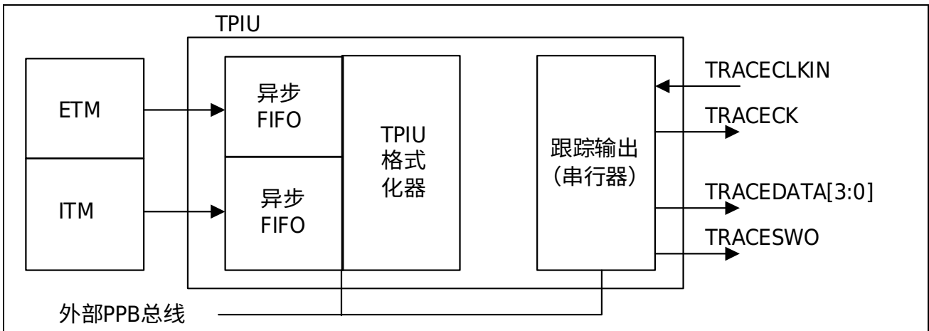
图 44-4 TPIU 框图
