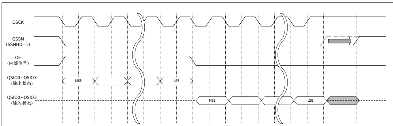
图 30-11 QSSN 保持时间配置示意图
