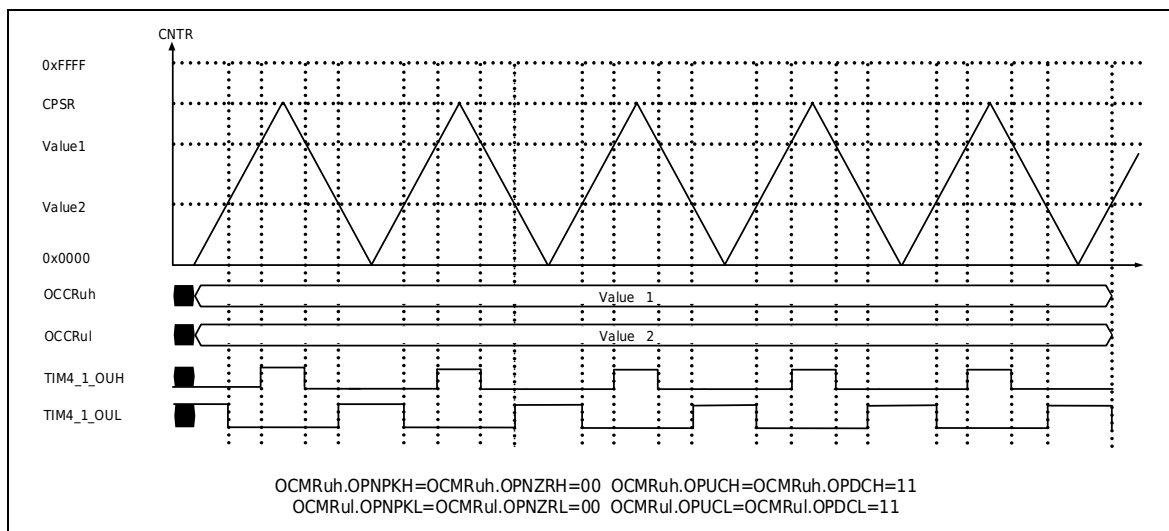
图 21-19 软件实现互补 PWM 输出
