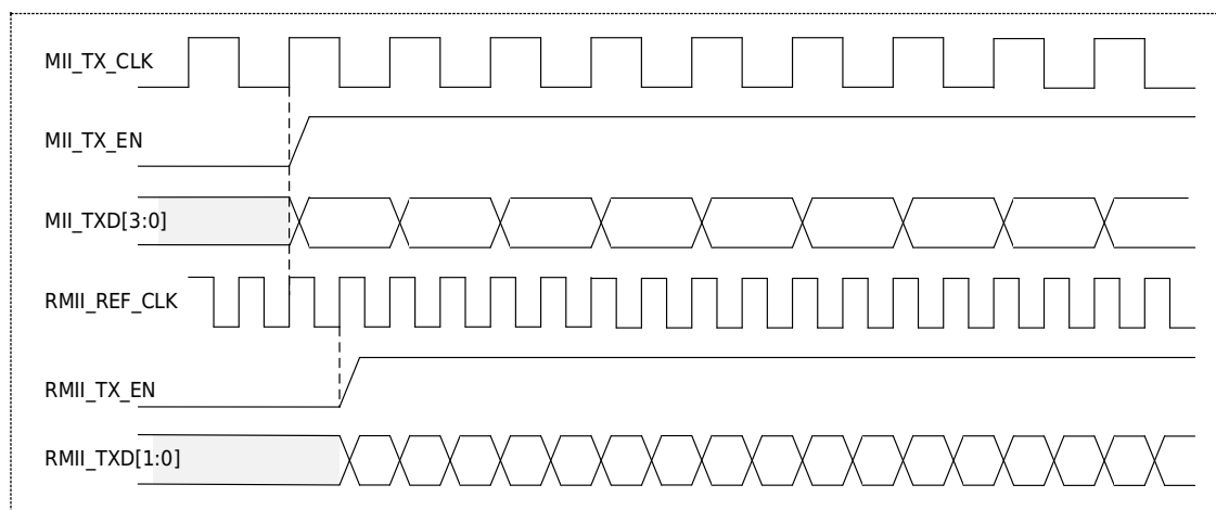
图 36-9 MII/RMII 模式下的发送图
