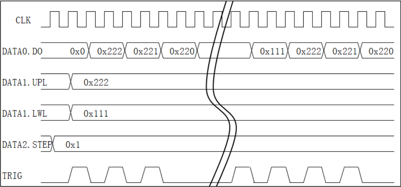
图 41-7 递减锯齿波输出示例时序图
