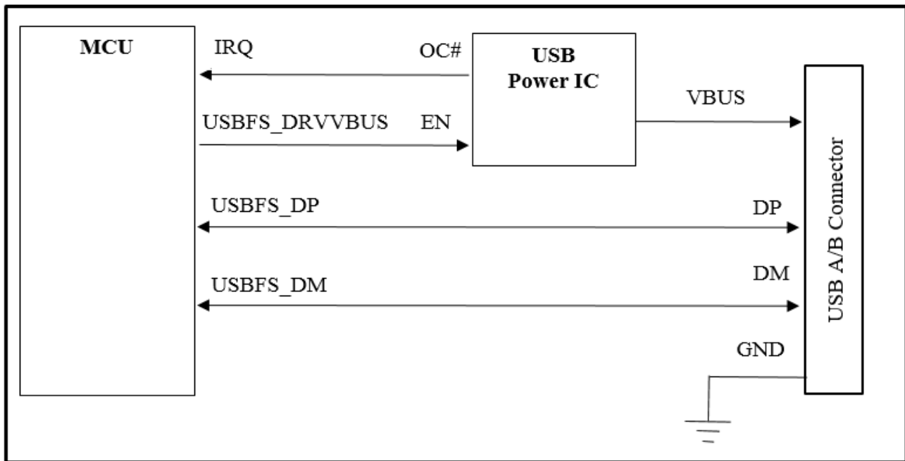
图 33-2 USBFS 主机模式系统构建图
