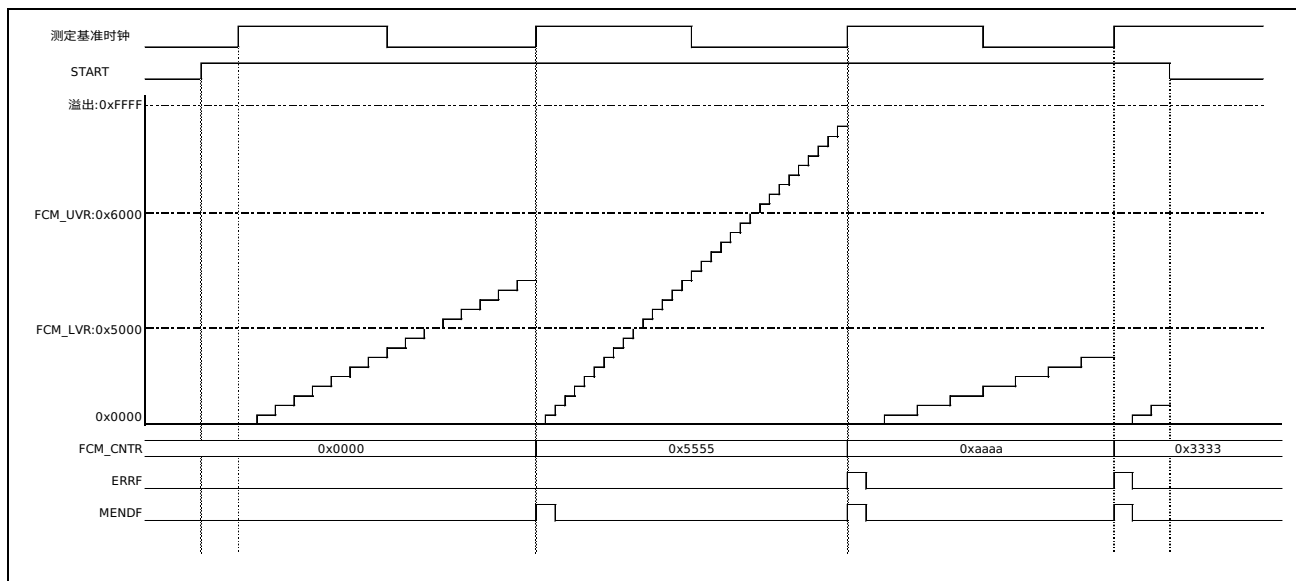
图 4-11 时钟频率测量时序图
