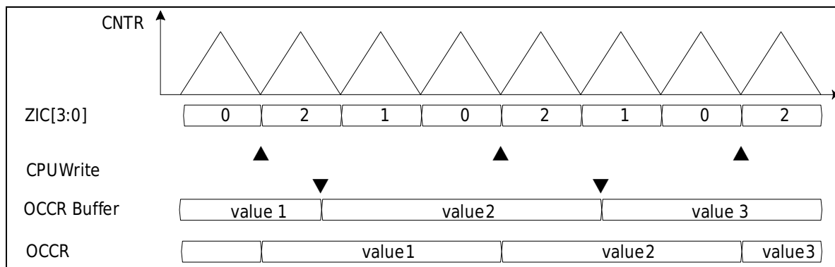
图 21-12 OCCR 缓冲数据传输(周期间隔响应链接使能)
