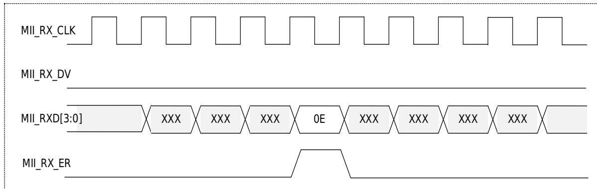
图 36-13 假载波指示下的接收图
