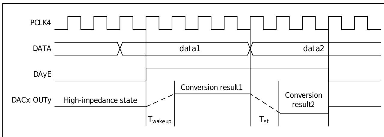
图 18-2 D/A 转换示意图
