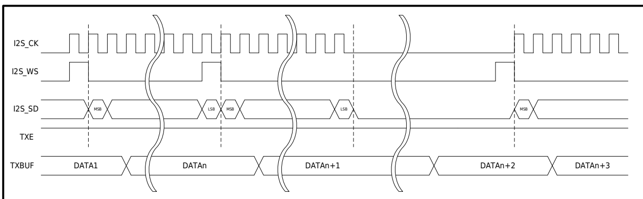
图 31-18 PCM 短帧主机发送暂停后重新发送方式二
