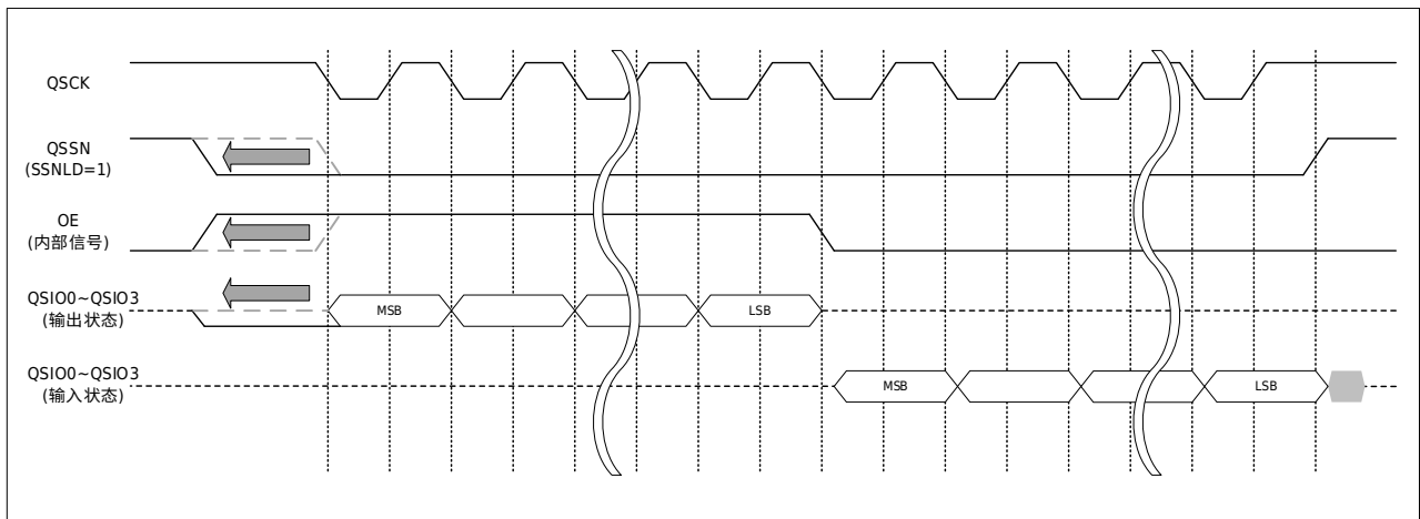
图 30-10 QSSL 建立时间配置示意图
