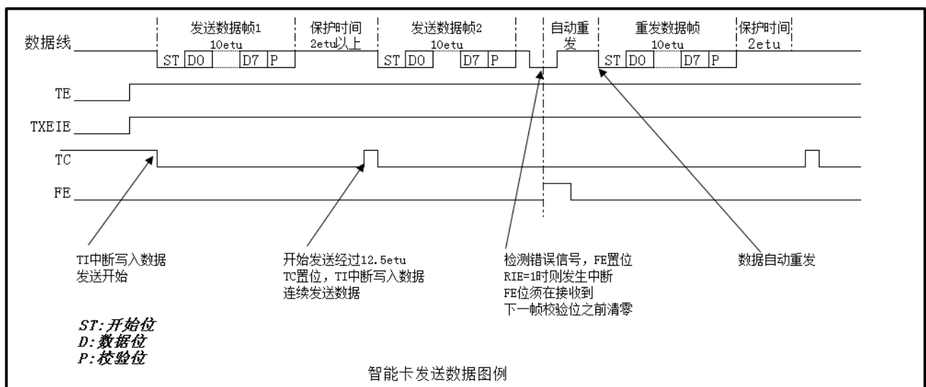
图 27-17 智能卡模式发送数据图例
