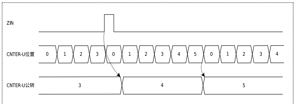
图 20-32 公转计数模式-混计数
