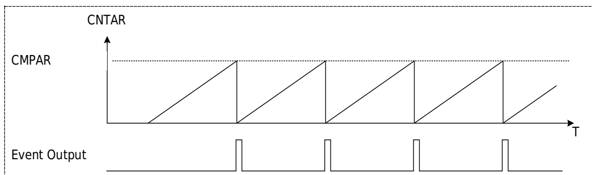
图 24-2 Timer0 计数时序图
