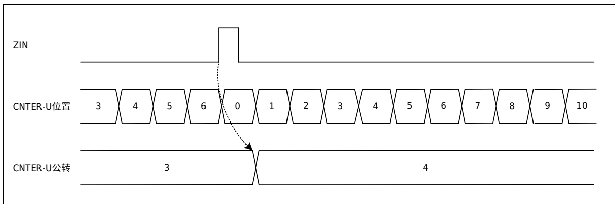
图 23-17 公转计数模式-Z 相计数
