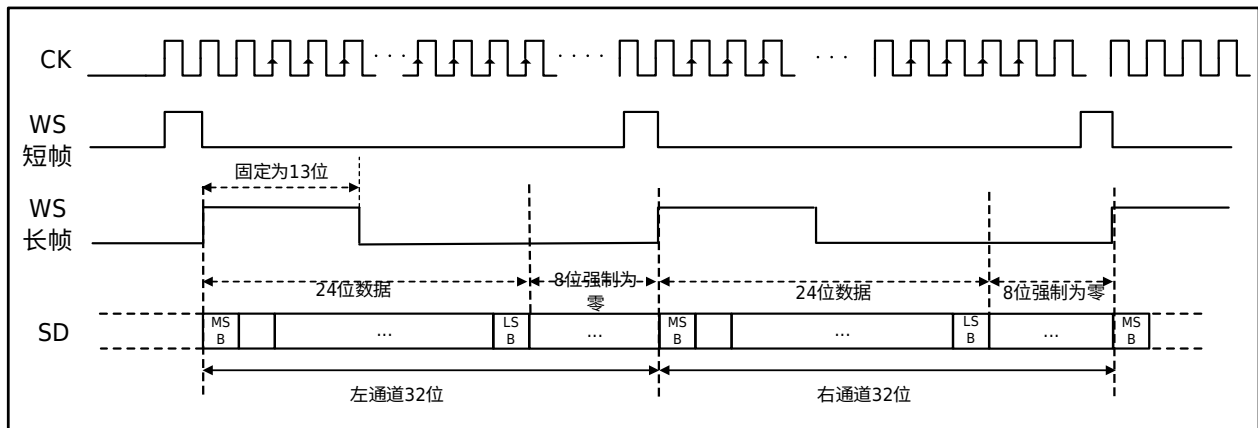
图 31-13 I2S PCM 协议波形 (24 位数据封装在 32 位帧中)
