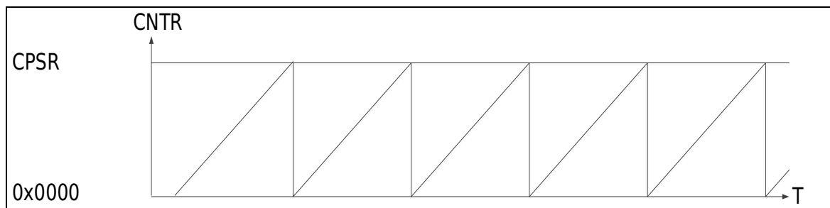
图 21-2 Timer4 锯齿波波形
