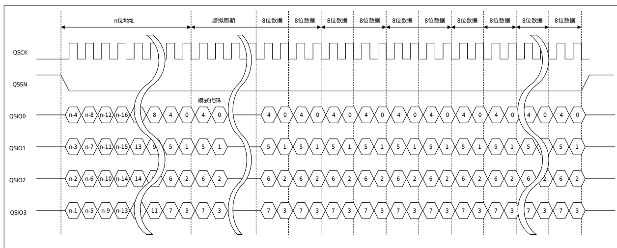
图 30-23 选择 XIP 模式的四线式输入输出快速读总线周期示意图
