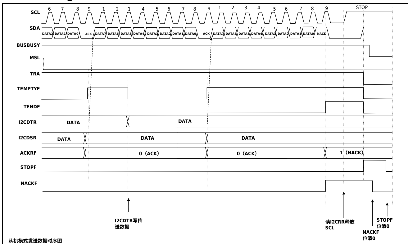
图 28-11 从机发送时序图 (2)
