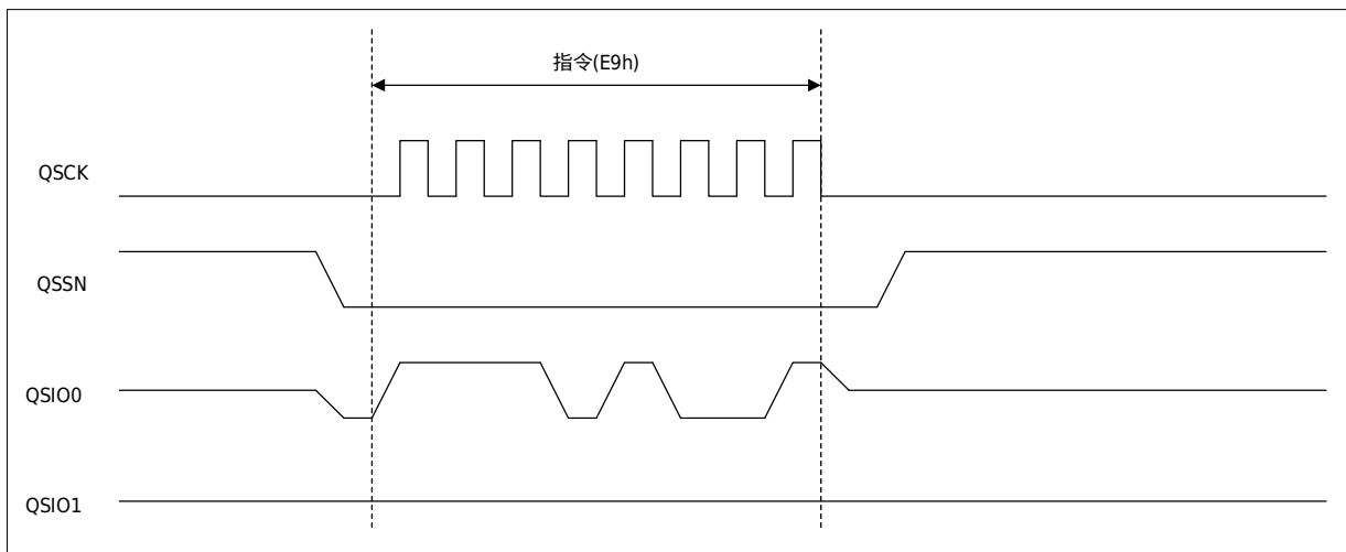
图 30-25 退出 4-Byte 模式指令总线周期示意图
