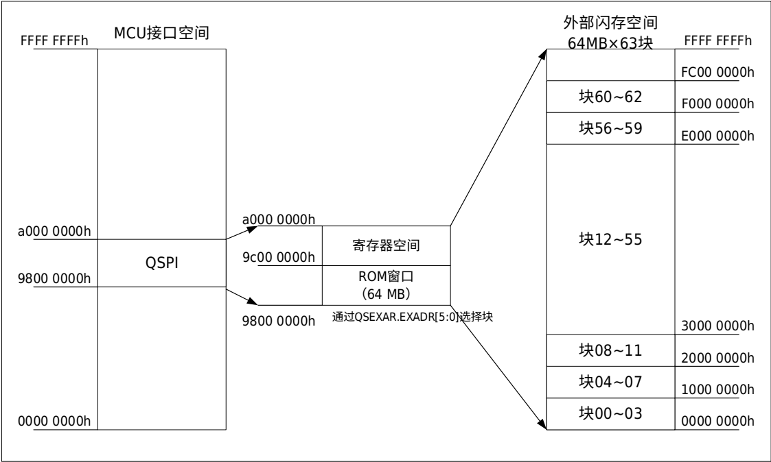
图 30-2 默认区域设定及 AHB 总线空间内存映射关系图
