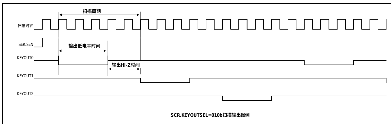
图 13-2 键盘扫描功能示意图
