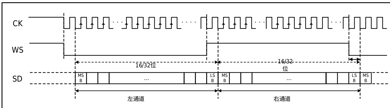
图 31-2 I2S Philips 协议波形 (16/32 位全精度)
