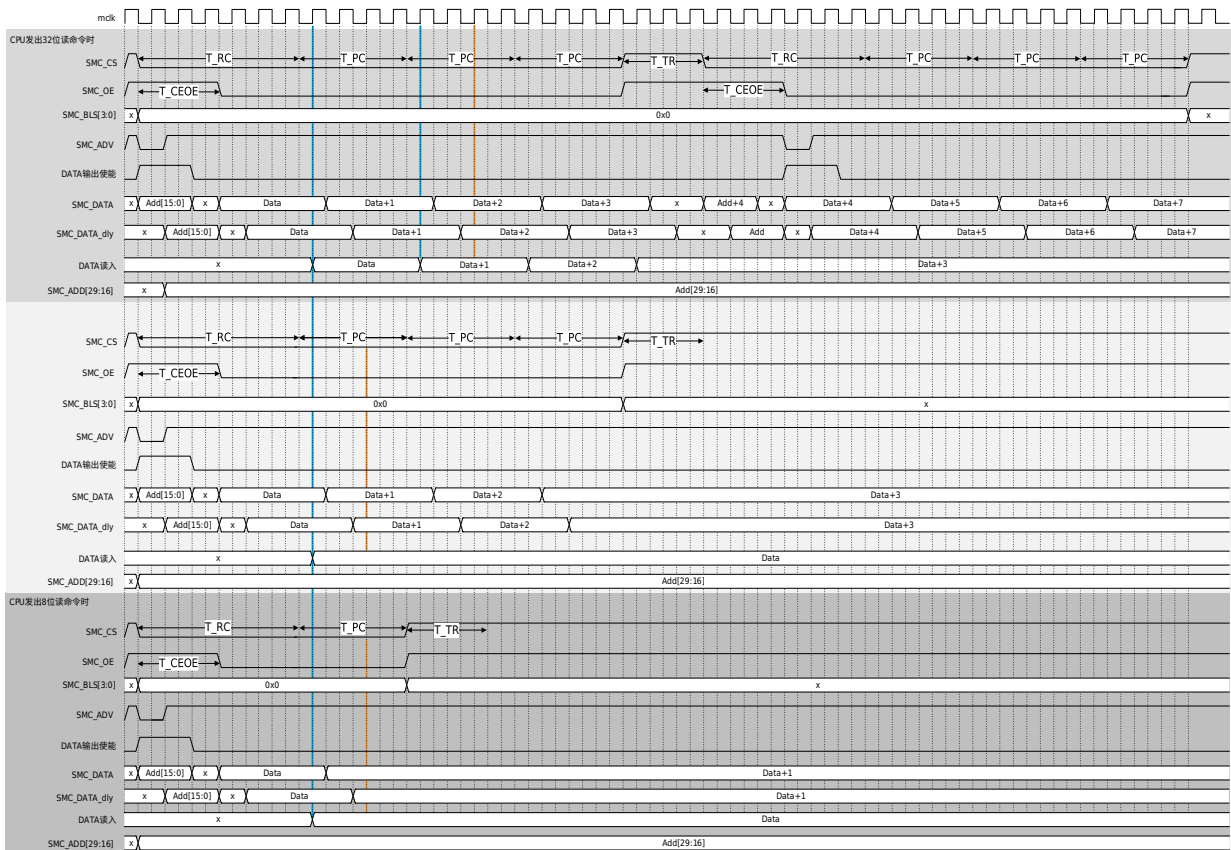
图 37-19 地址数据复用突发读动作基本时序（同/异步方式（RSYN=1/0）&16 位位宽（MW=01）&RBL=001）
