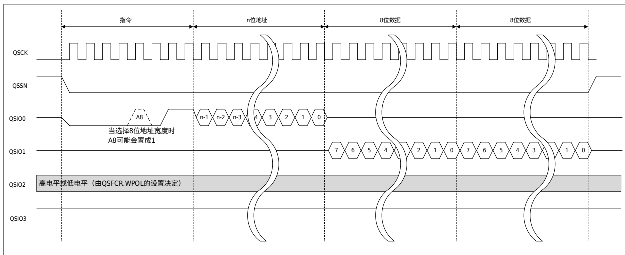
图 30-13 标准读总线周期示意图
