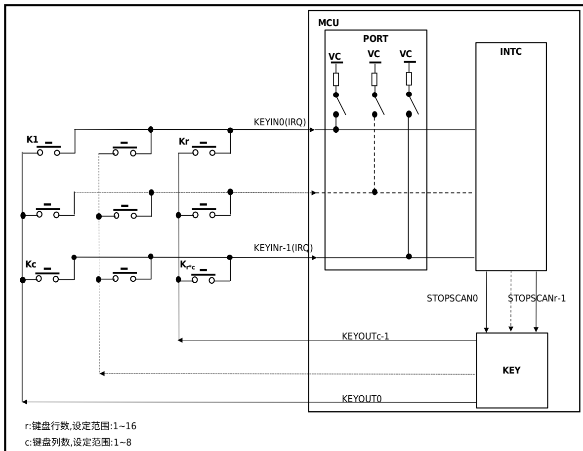
图 13-1 KEYSKAN 系统框图
