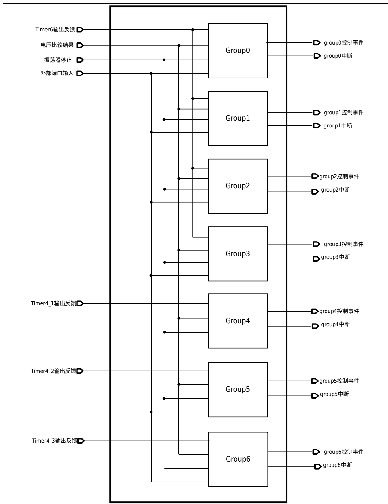
图 22-1 EMB 结构框图
