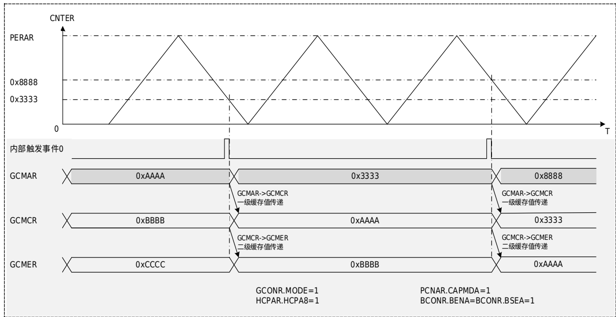
图 20-12 双缓存方式捕获输入时序
