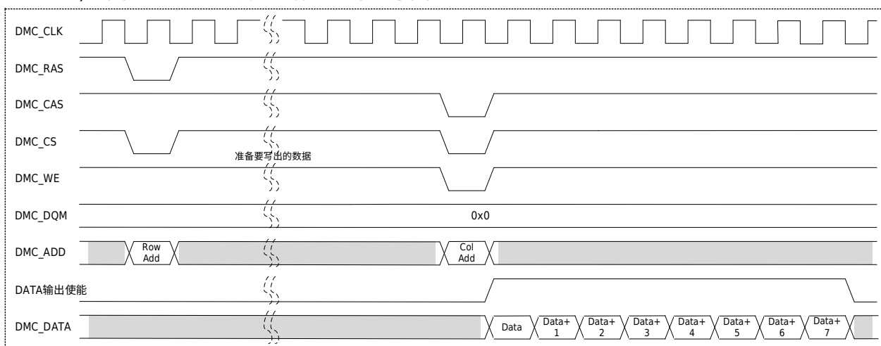
图 37-34 突发写动作基本时序 (32 位位宽 (DMCMW=10) & BURST=011)
