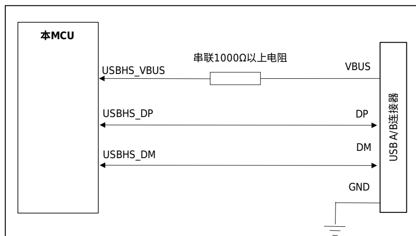
图 32-3 USBHS 设备模式系统构建图
