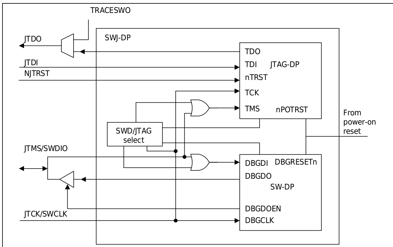
图 44-2 调试控制系统
