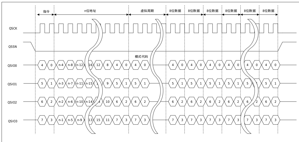
图 30-28 自定义快速读总线周期示意图
