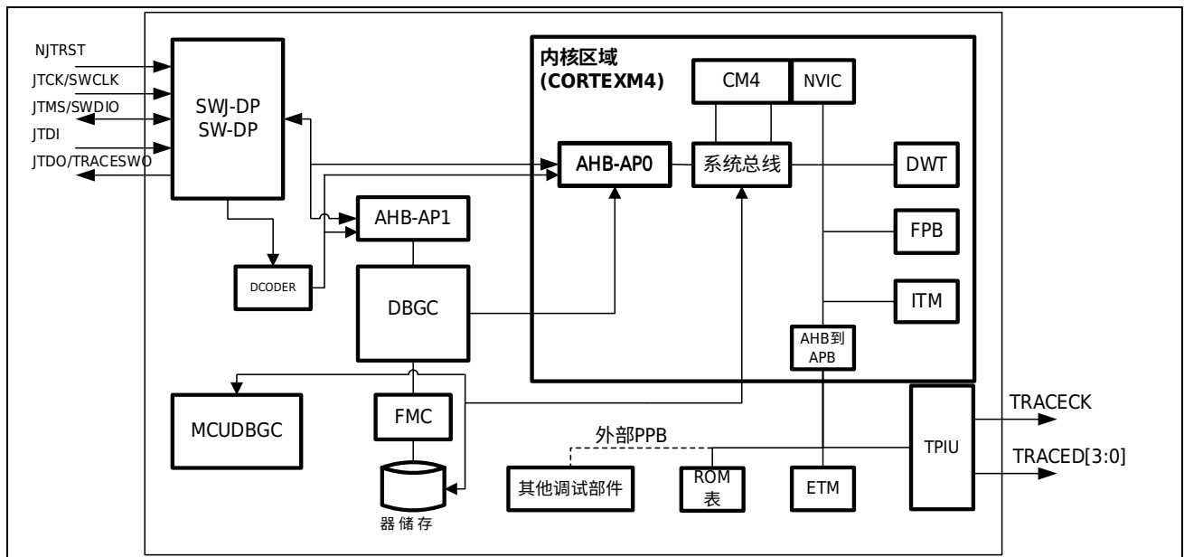
图 44-1 调试控制系统
