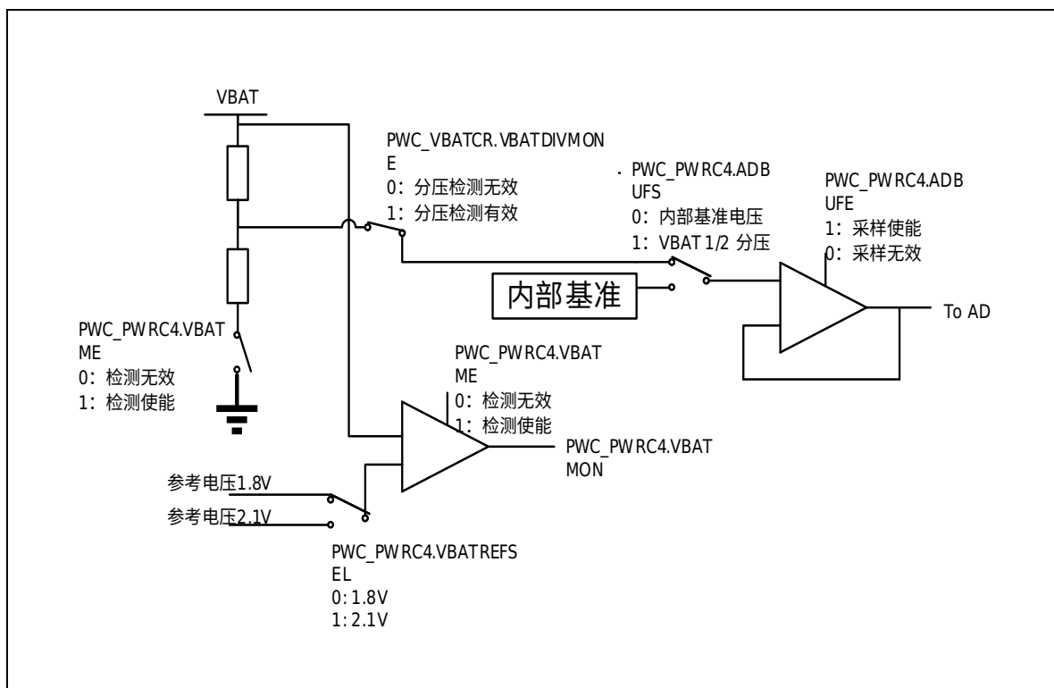
图 5-11 内部电压采样示意图
