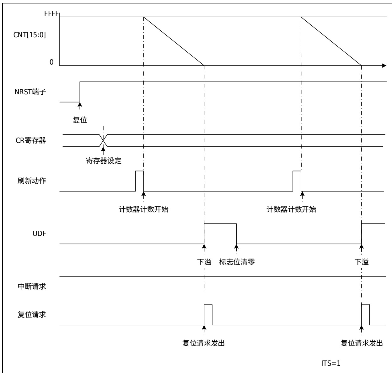
图 26-4 计数器下溢动作例
