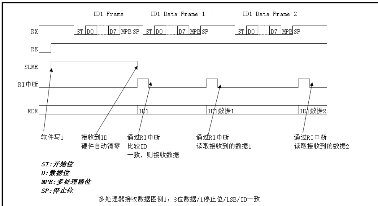
图 27-11 多处理器模式接收数据图例 1
