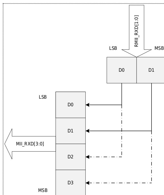
图 36-10 MII/RMII 接收位序
