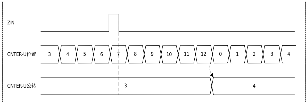
图 20-31 公转计数模式-位置溢出计数
