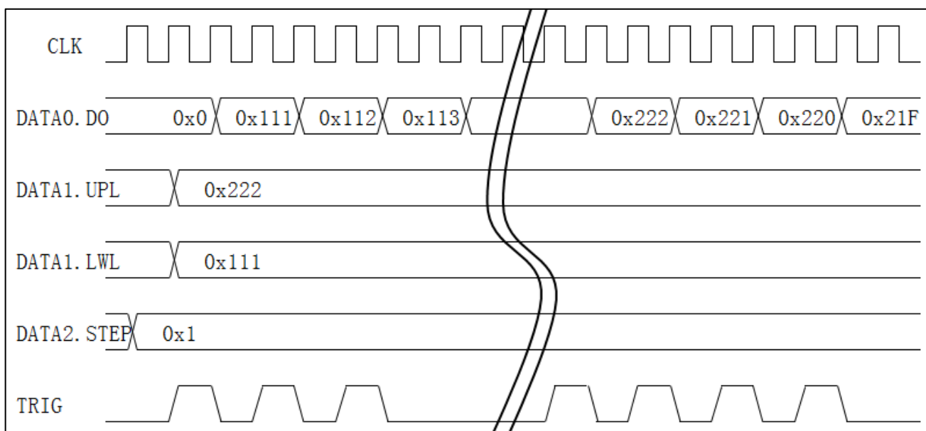
图 41-3 三角波输出示例时序图
