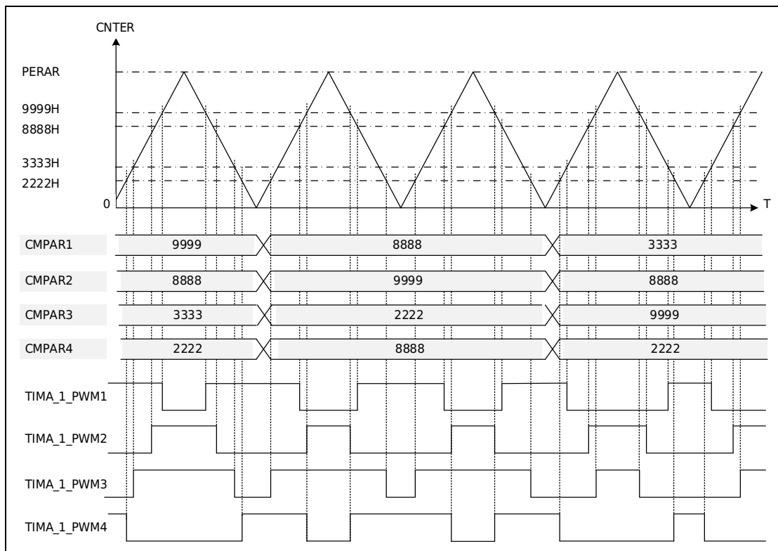
图 23-11 双边对称 PWM 输出例
