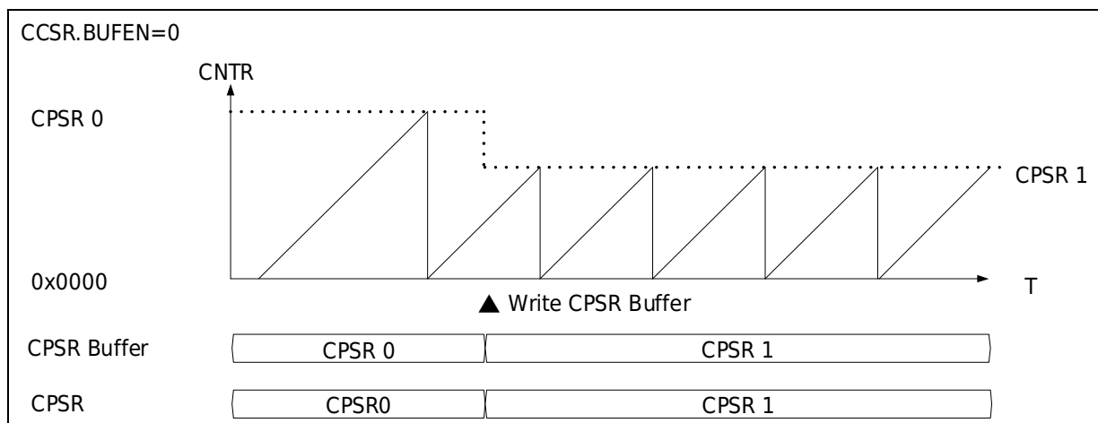
图 21-8 缓存无效时修改锯齿波计数周期
