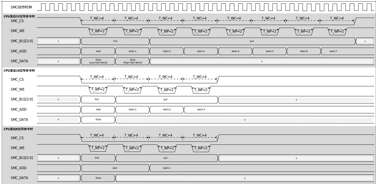
图 37-14 单次写动作基本时序（异步方式（WSYN=0）&16 位位宽（MW=01）&BLS=0）
