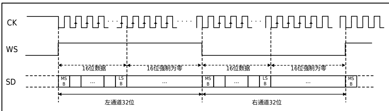
图 31-6 I2S MSB 协议波形（16 位数据封装在 32 位帧中）
