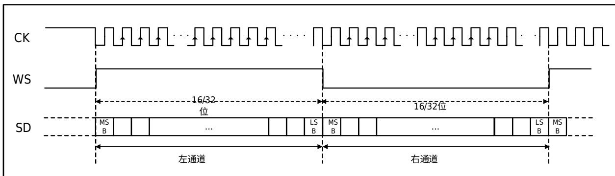
图 31-8 I2S LSB 协议波形（16/32 位全精度）
