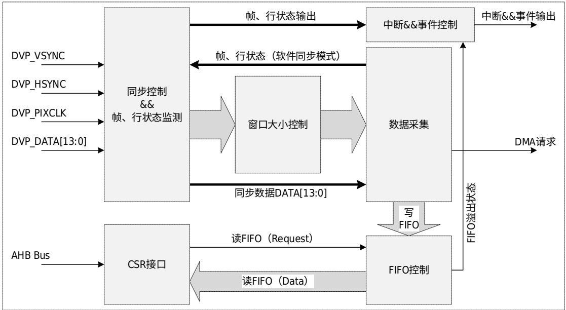
图 38-1 DVP 基本框图
