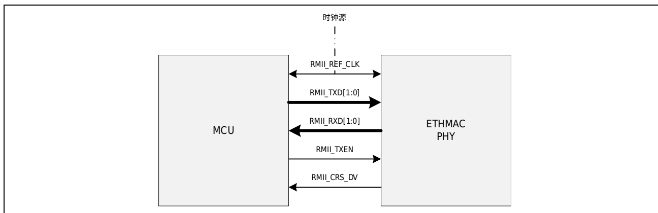
图 36-3 RMII 接口连接图
