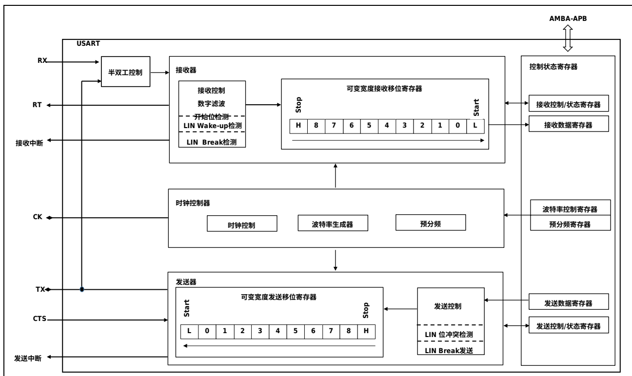
图 27-1 USART 系统框图
