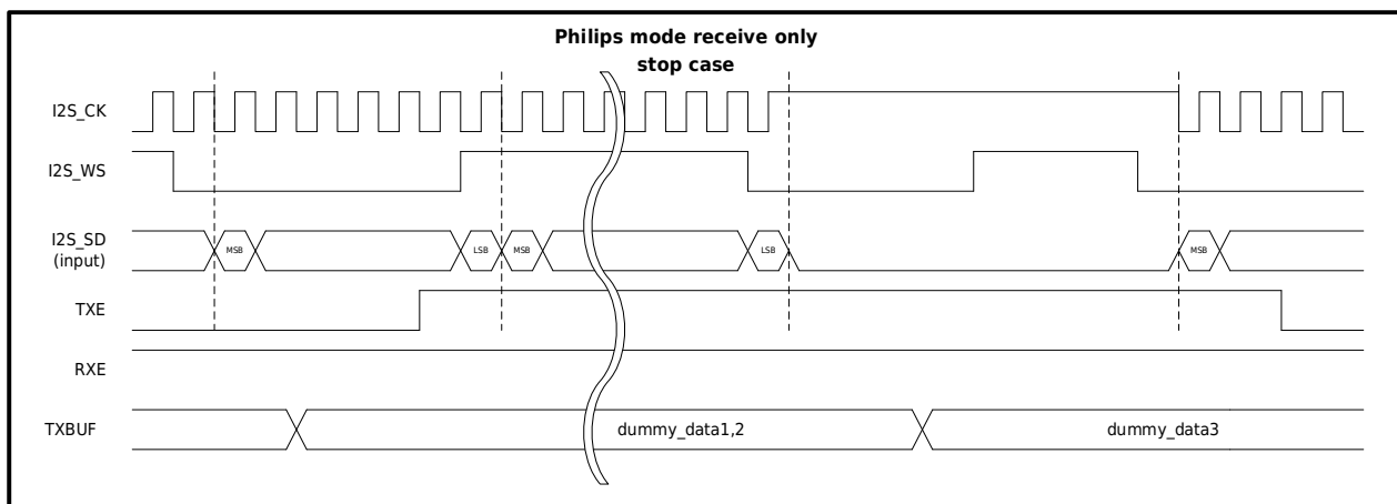
图 31-16 主机只接收暂时停止接收
