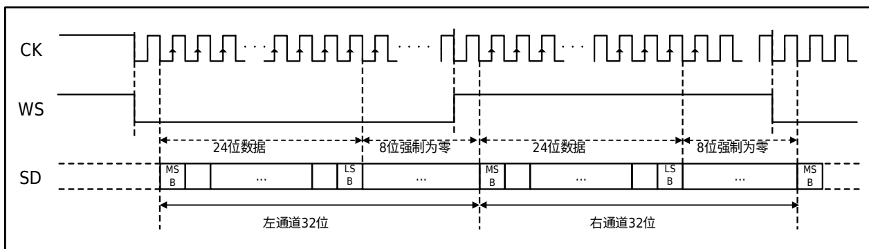
图 31-4 I2S Philips 协议波形 (24 位数据封装在 32 位帧中)
