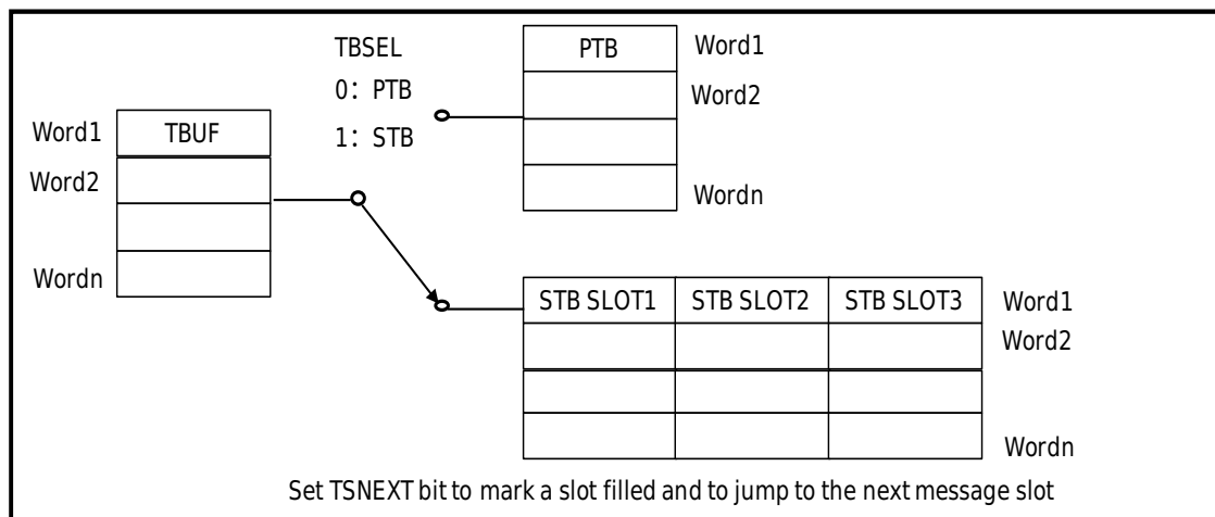
图 34-3 CAN TBUF 寄存器写发送缓冲器和示意图
