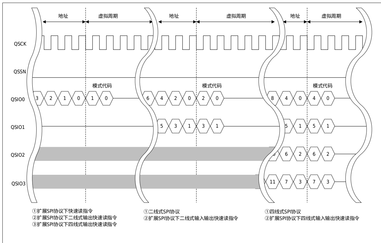
图 30-33 XIP 模式控制示意图
