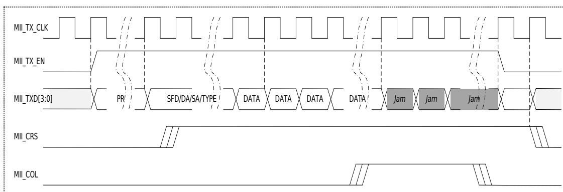
图 36-8 有冲突发送图
