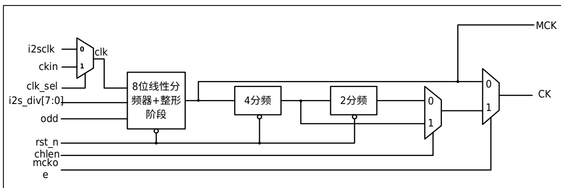
图 31-15 时钟发生器架构
