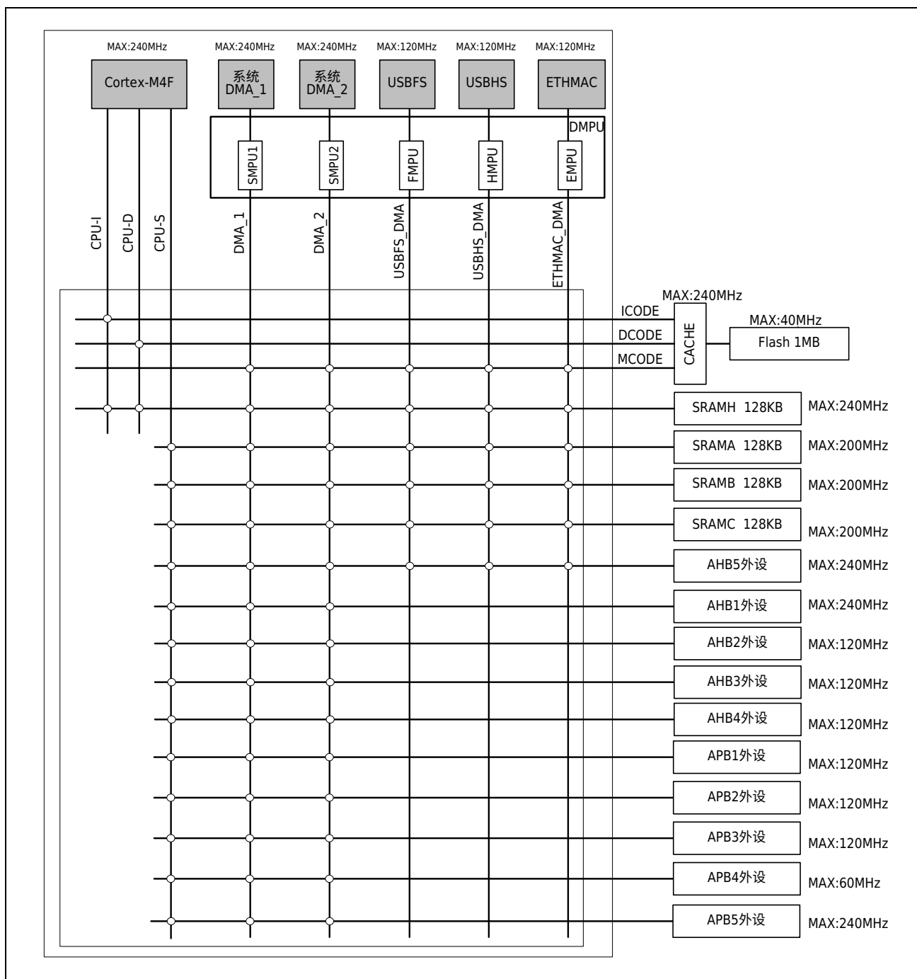
图 2-1 总线架构图
