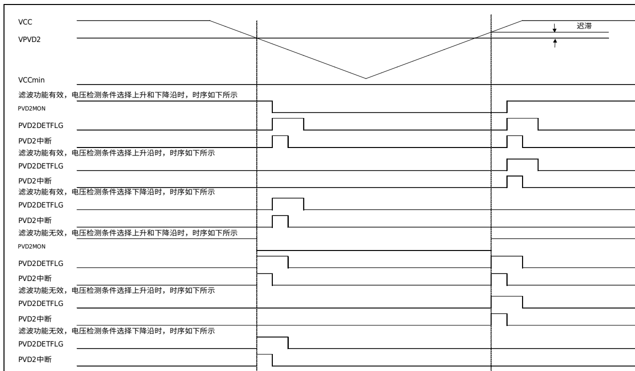
图 5-9 电源监视 2 中断运行时序图
