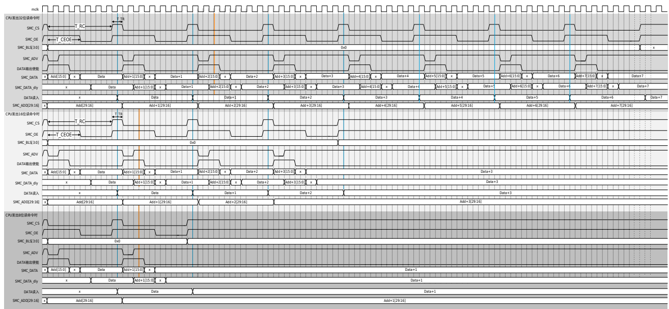
图 37-12 地址数据线复用单次读动作基本时序 (异步方式 (RSYN=0) &16 位位宽 (MW=01))
