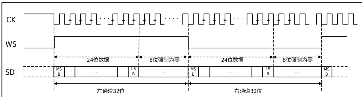
图 31-7 I2S MSB 协议波形（24 位数据封装在 32 位帧中）
