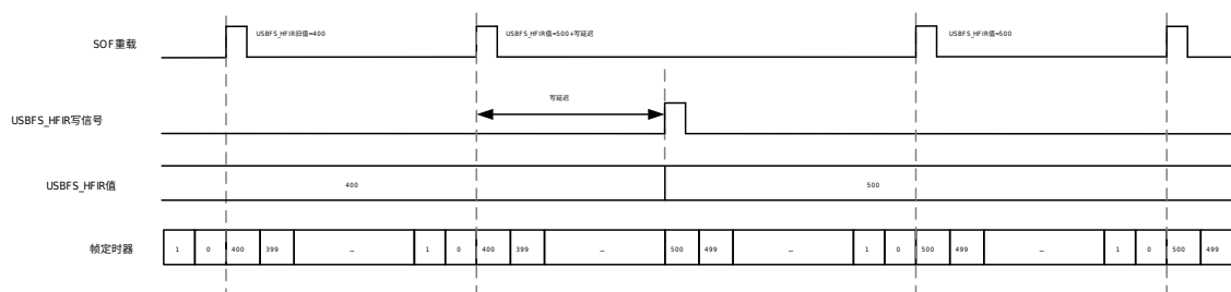
图 33-4 USBFS 动态更新 USBFS_HFIR 寄存器示意图
