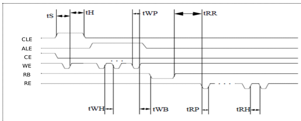
图 37-36 NFC 时序控制图
