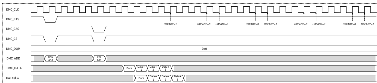
图 37-33 突发读动作基本时序 (32 位位宽 (DMCMW=10) & BURST=010)
