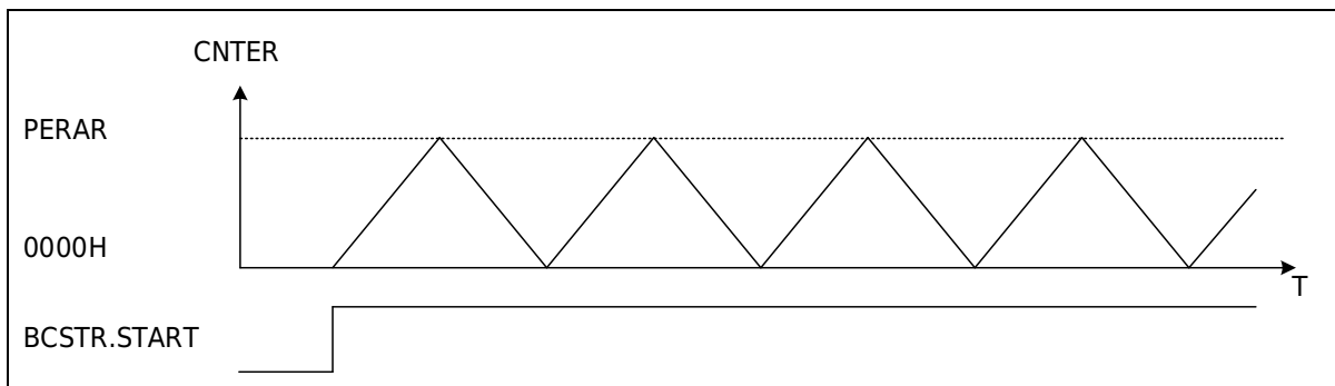
图 23-3 三角波波形
