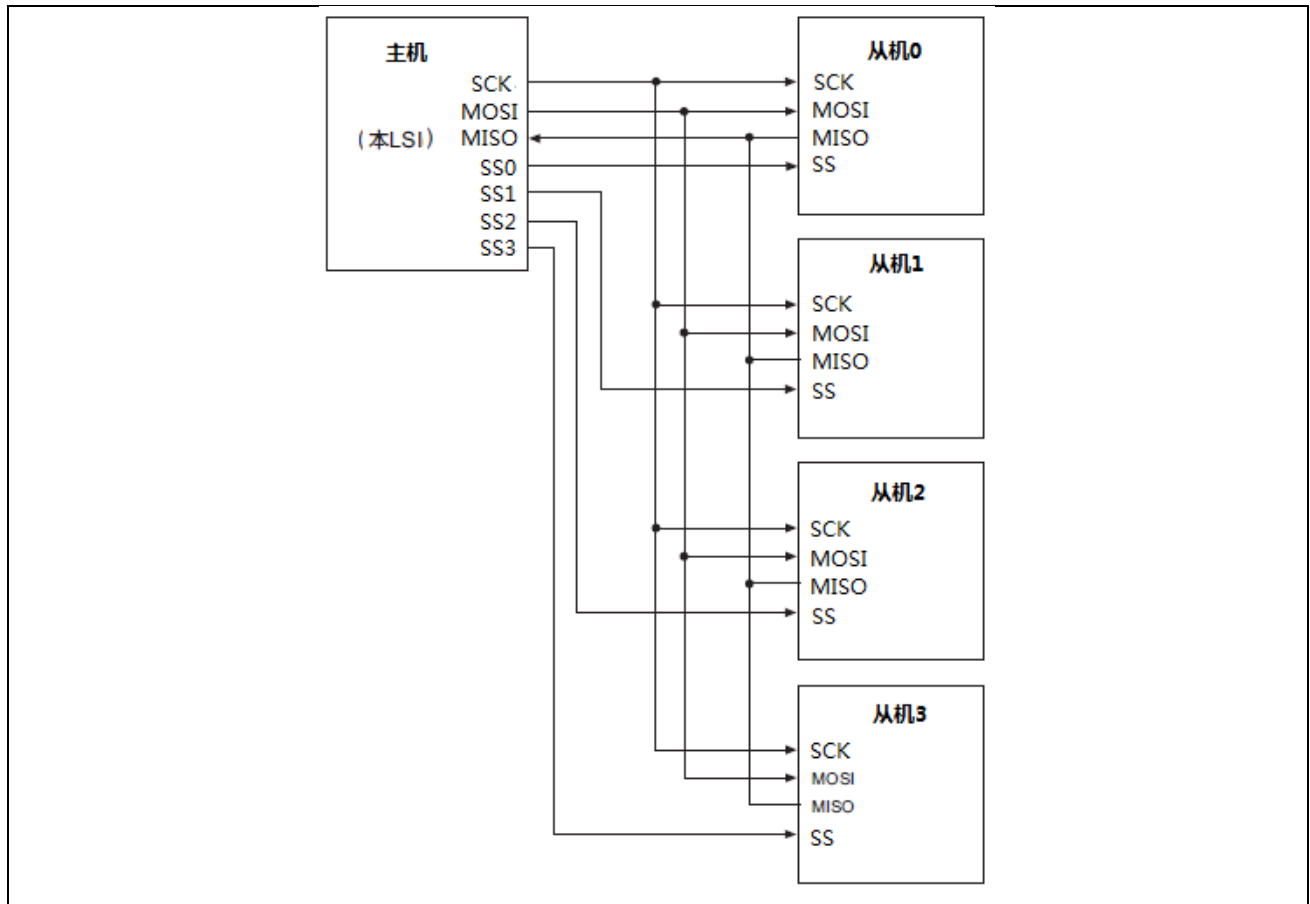
图 29-2 主机模式结构
