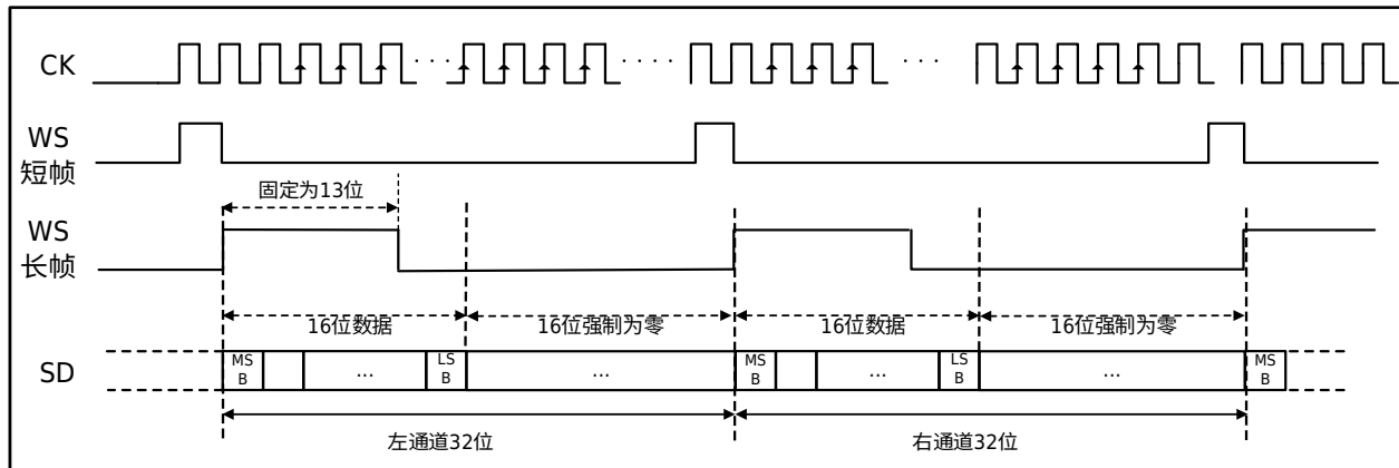
图 31-12 I2S PCM 协议波形（16 位数据封装在 32 位帧中）
