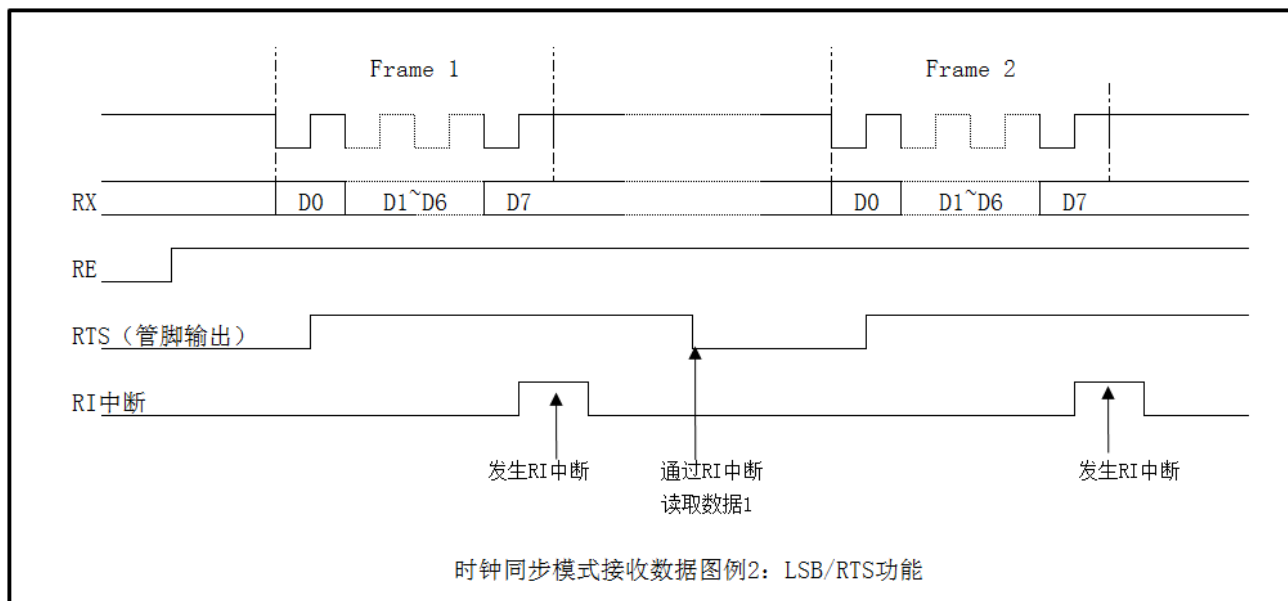
图 27-23 时钟同步模式接收数据图例 2
