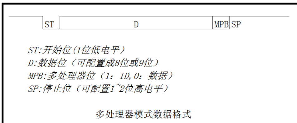
图 27-9 多处理器模式数据格式
