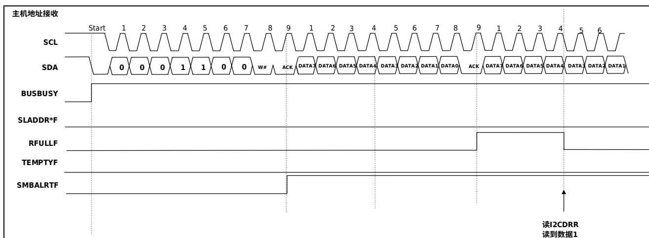
图 28-18 SMBus 报警响应地址接收时序图
