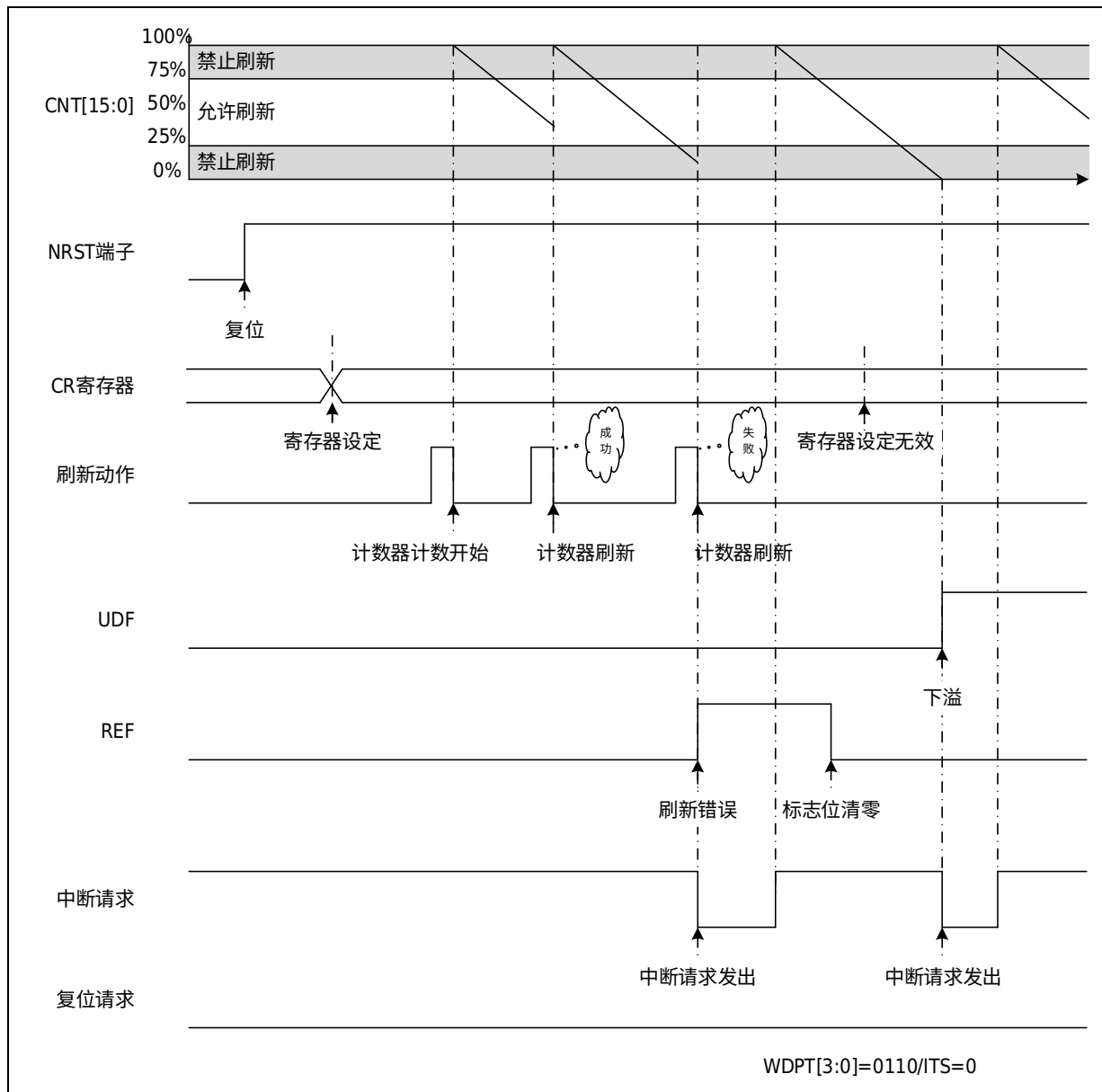
图 26-5 计数器刷新动作例
