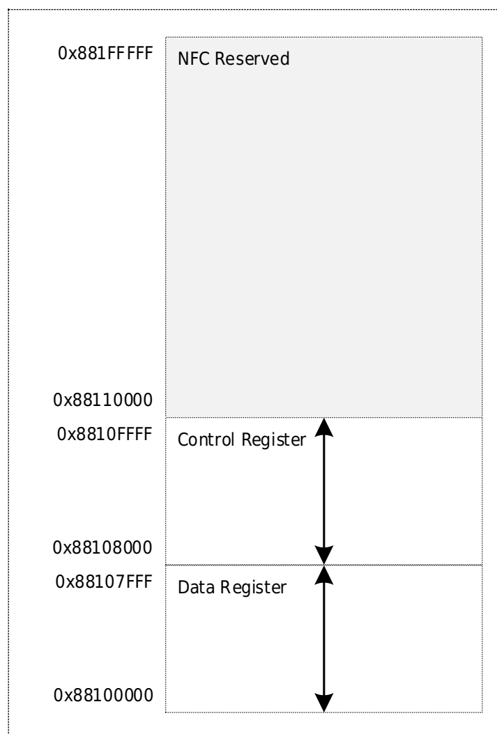
图 37-5 NFC 的地址空间划分
