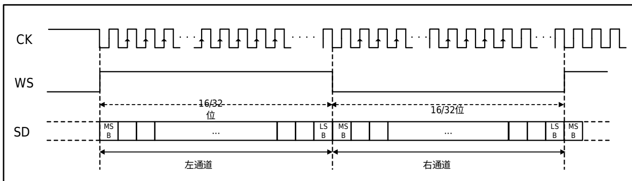
图 31-5 I2S MSB 协议波形（16/32 位全精度）
