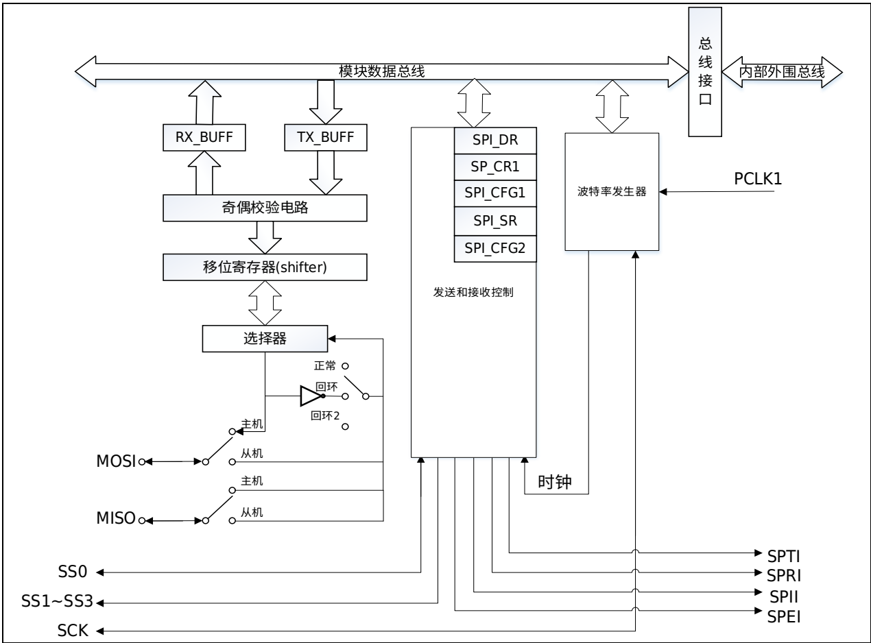
图 29-1 系统框图
