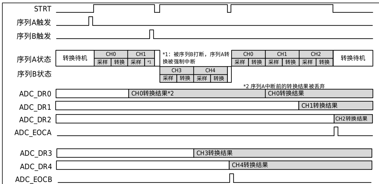
图 17-7 双序列扫描模式 (序列 A 从第一个通道重新启动)
