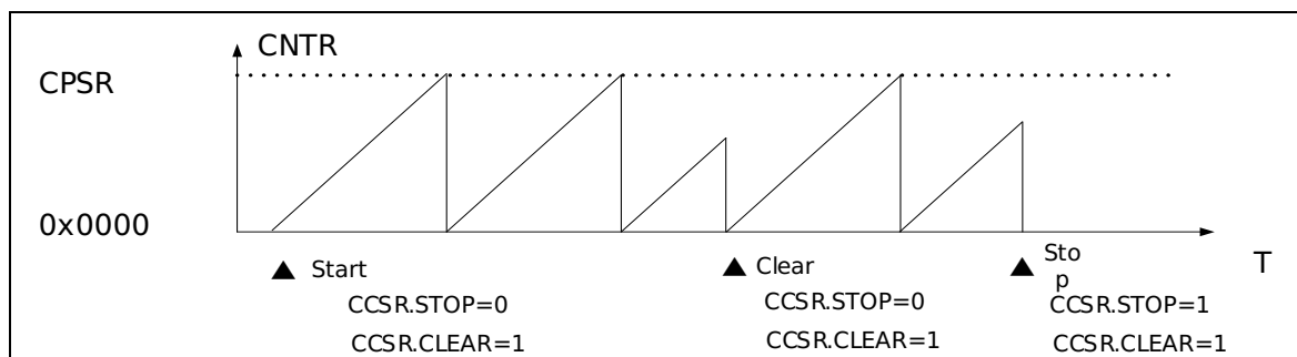
图 21-4 Timer4 锯齿波模式计数动作
