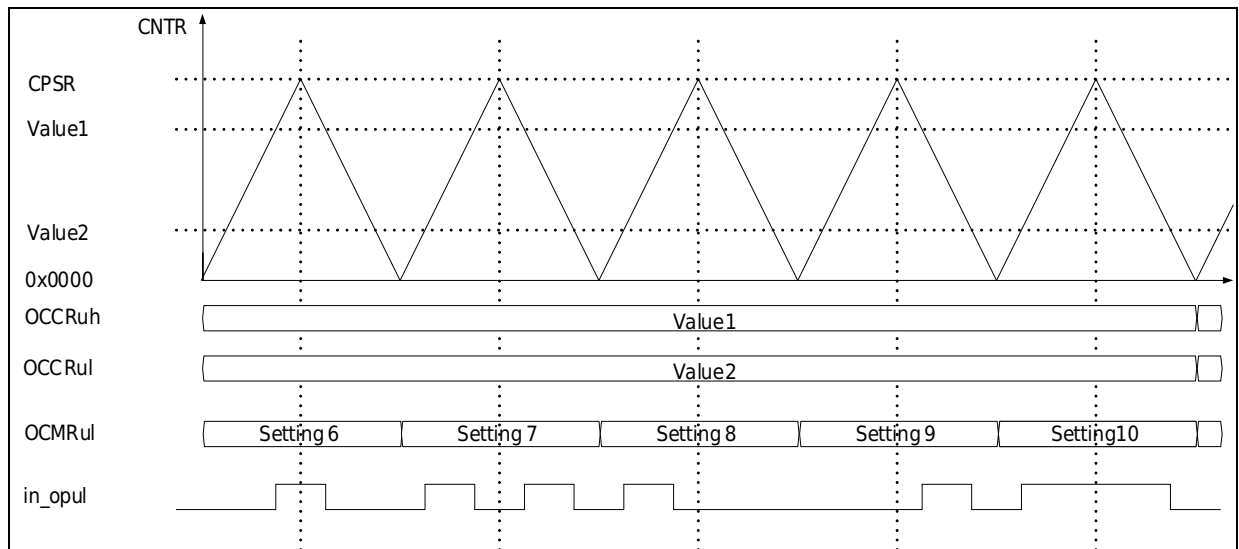
图 21-13 输出比较缓冲数据传输 (OCMR 缓冲使能)
