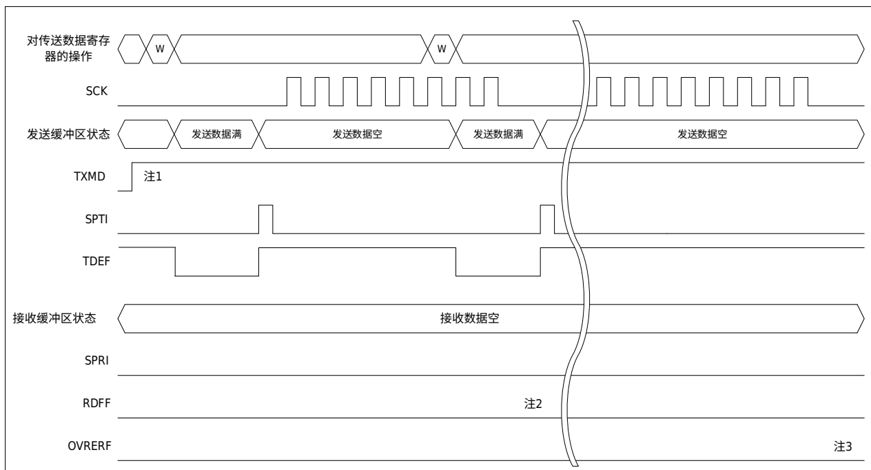
图 29-8 只进行发送通信
