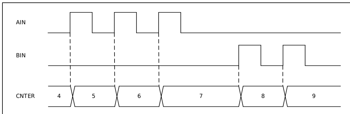
图 23-12 位置模式-基本计数
