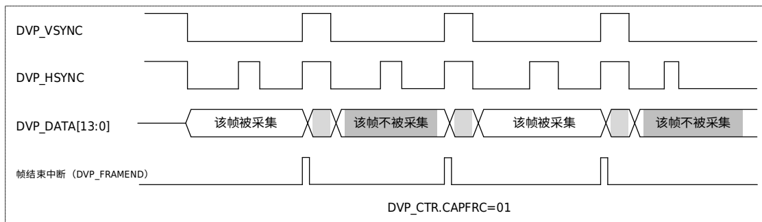
图 38-5 帧采集频率控制
