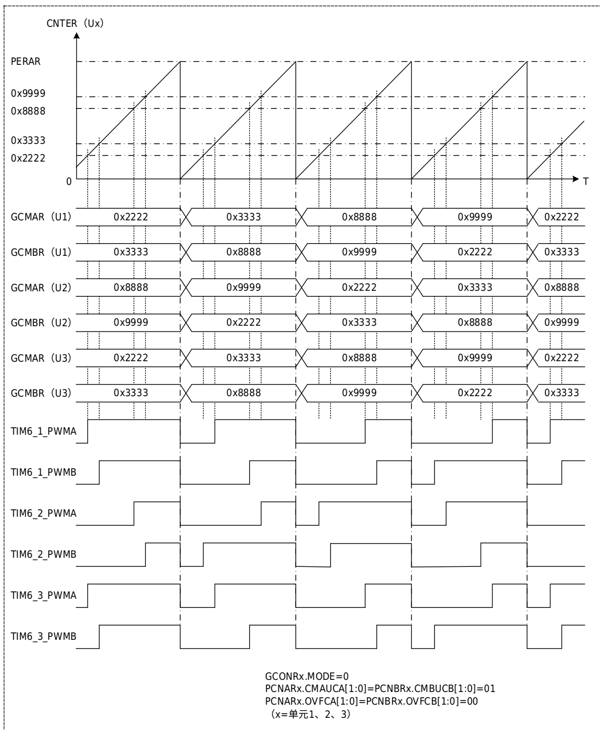
图 20-22 6 相单边对齐独立 PWM
