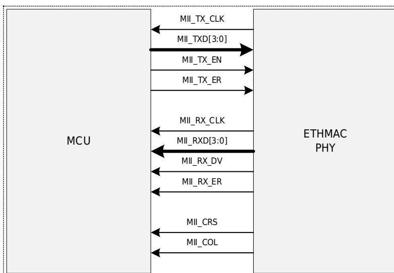
图 36-2 MII 接口连接图
