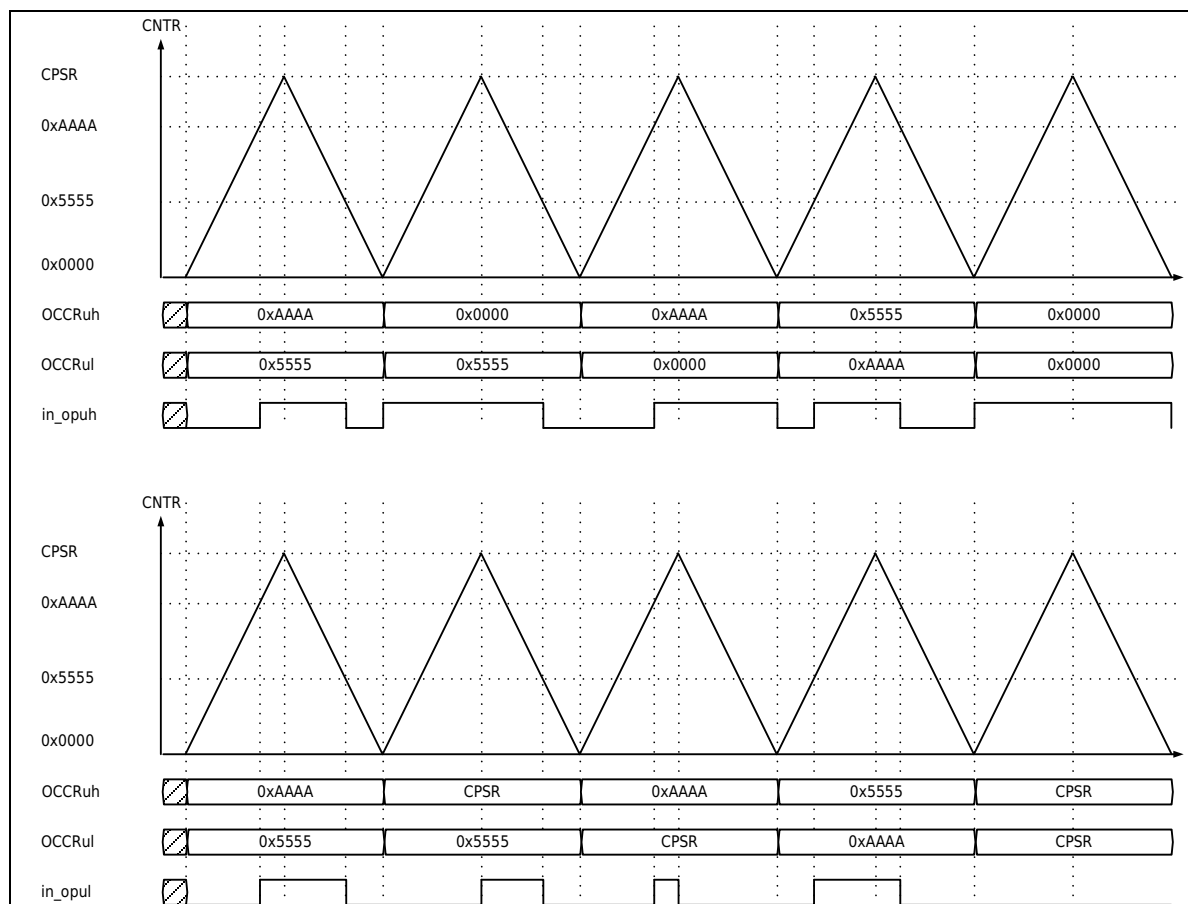
图 21-7 三角波模式波形输出例
