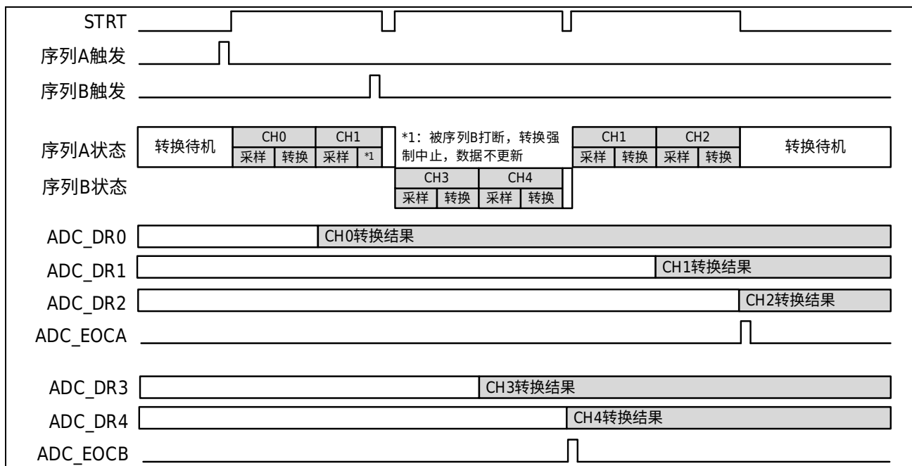
图 17-6 双序列扫描模式 (序列 A 从被中断通道重新启动)
