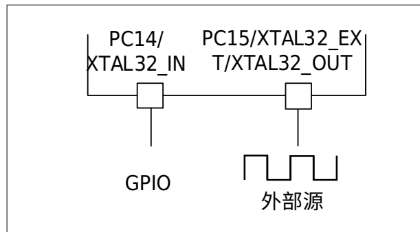
图 4-8 外部低速时钟输入的连接示例
