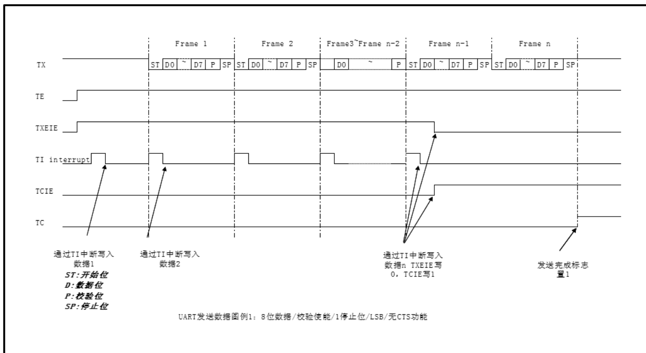
图 27-3 UART 发送数据图例 1
