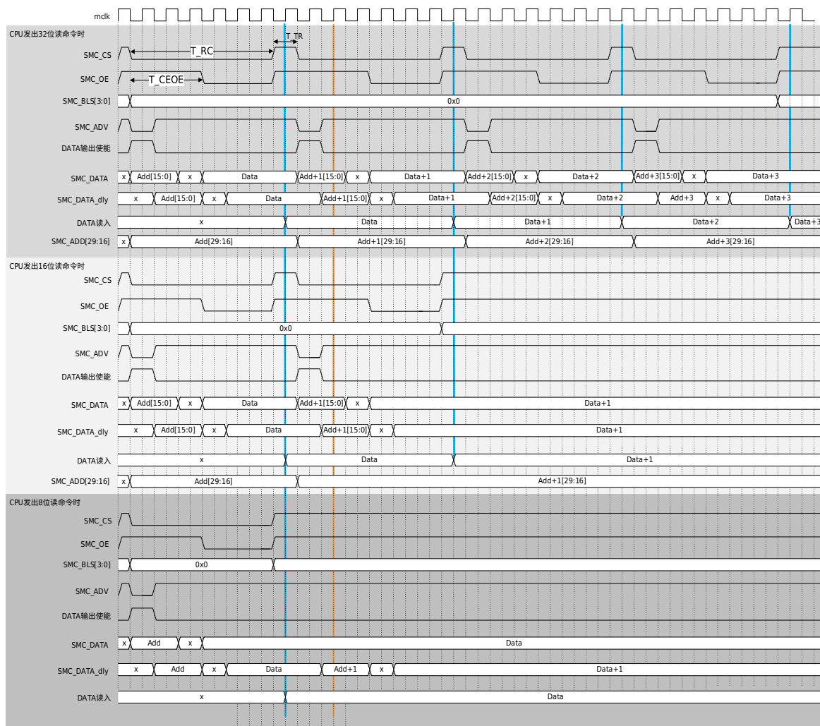
图 37-13 地址数据线复用单次读动作基本时序（异步方式（RSYN=0）&32 位位宽（MW=10））
