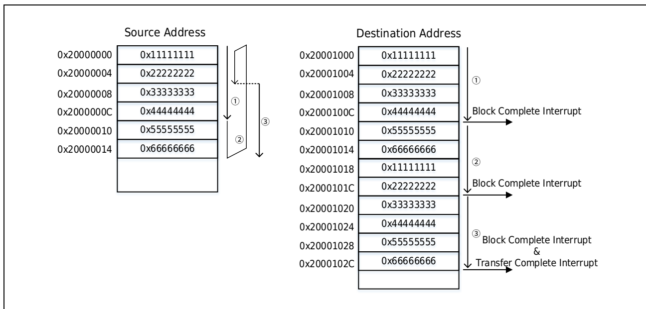
图 15-5 应用例 1：存储器到存储器传输
