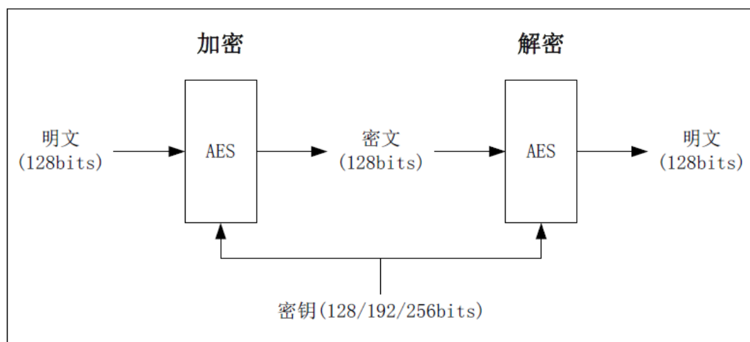
图 39-1 AES 加解密流程示意图
