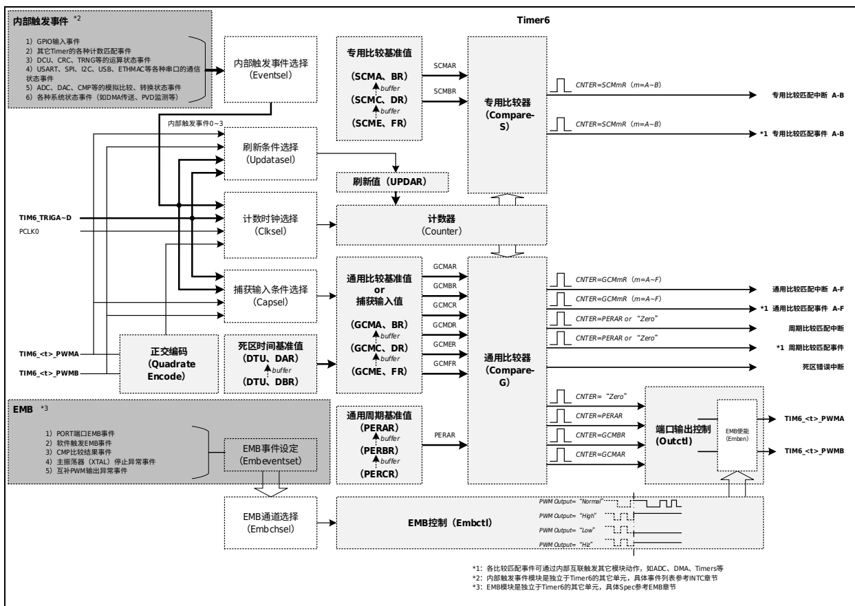
图 20-1 Timer6 基本框图
