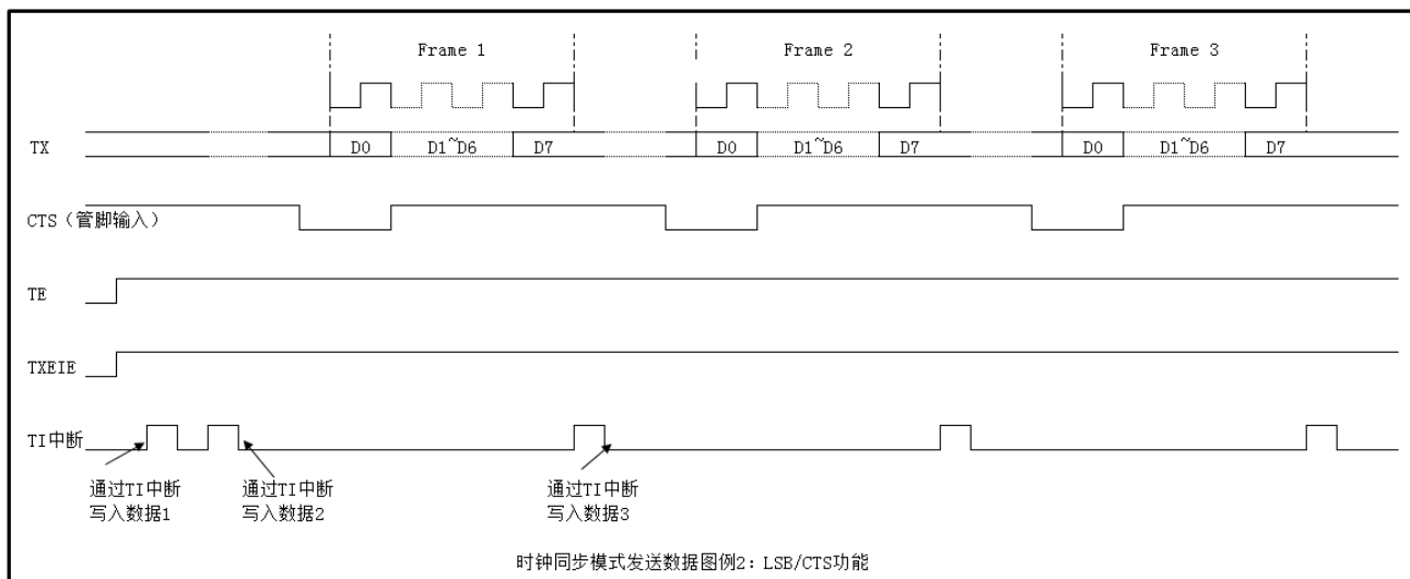
图 27-21 时钟同步模式发送数据图例 2
