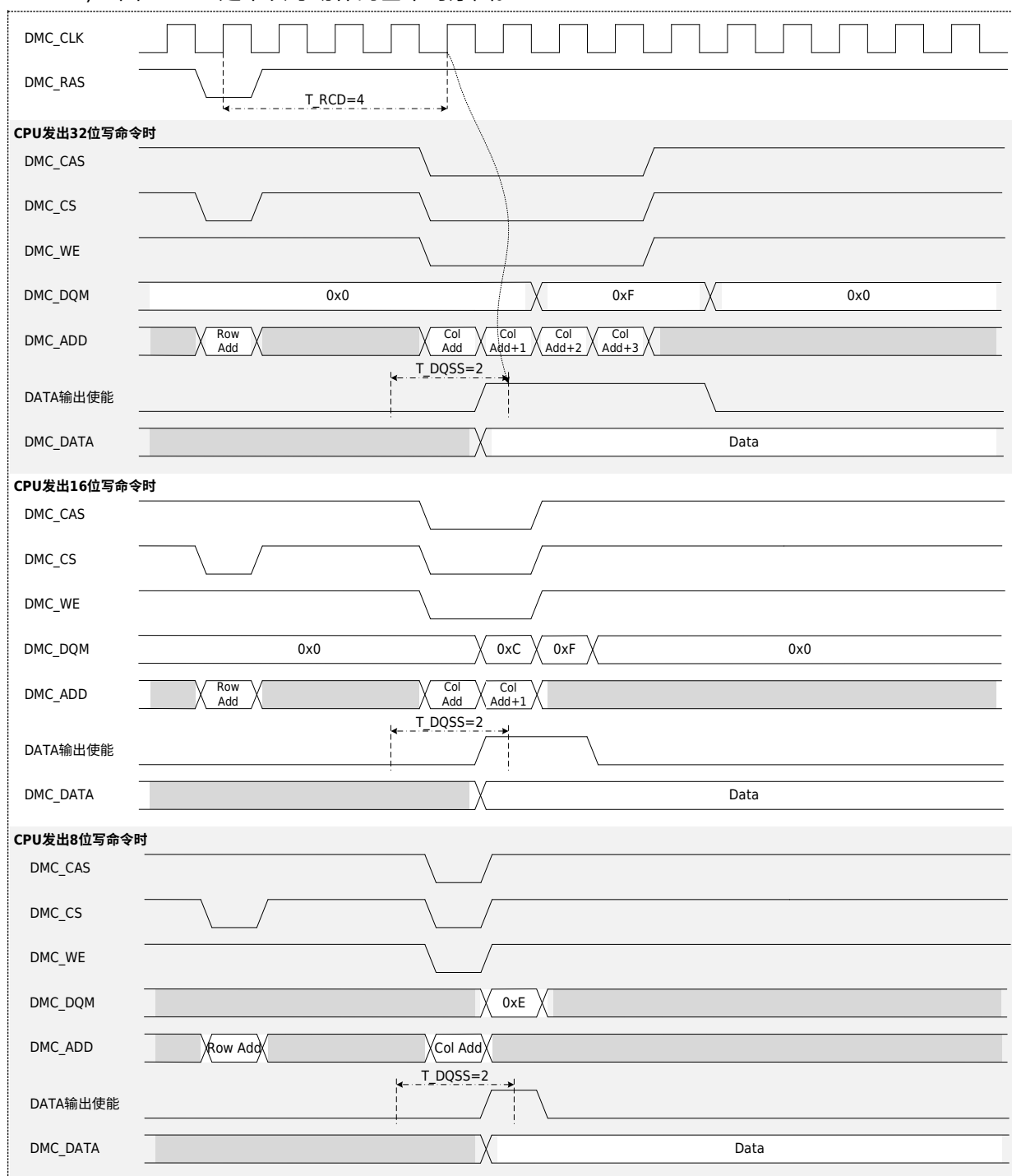
图 37-32 单次写动作基本时序 (32 位位宽 (DMCMW=01))
