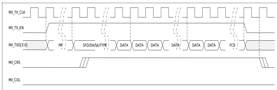
图 36-7 无冲突发送图
