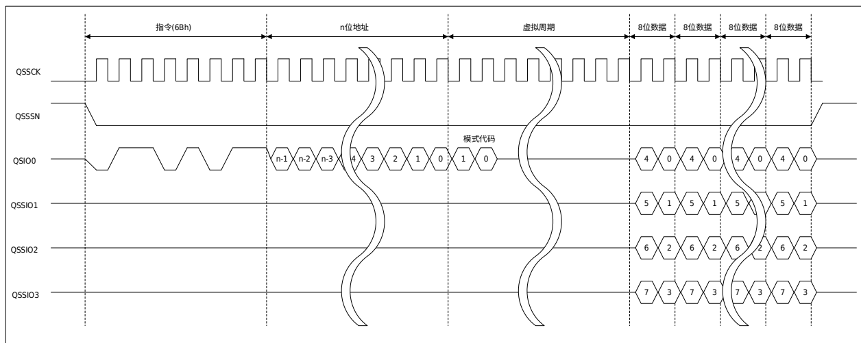
图 30-20 四线式输出快速读总线周期示意图
