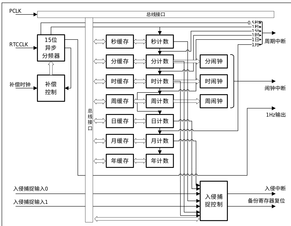
图 25-1 RTC 的基本框图
