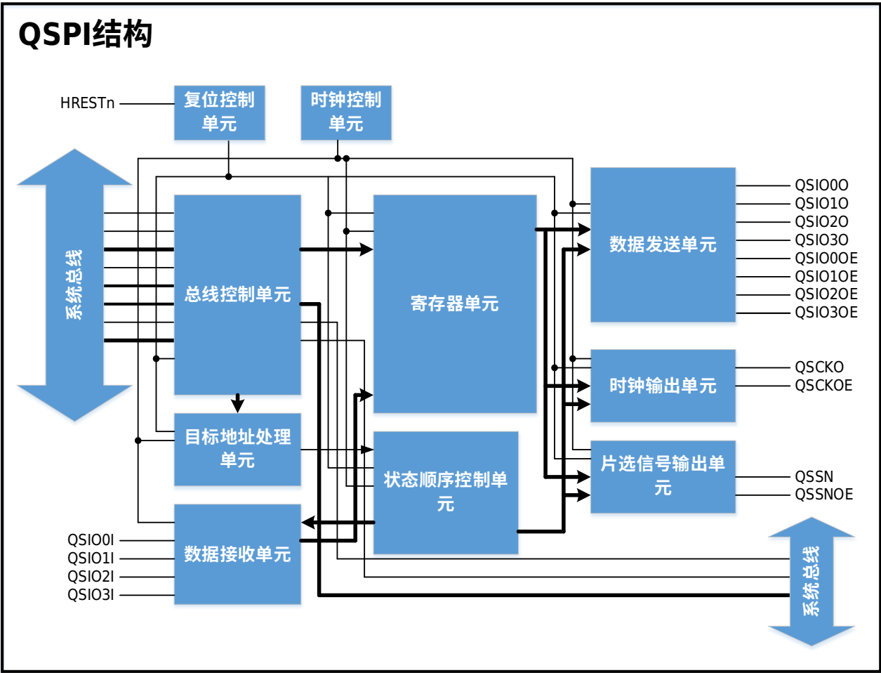
图 30-1 QSPI 的模块构成图
