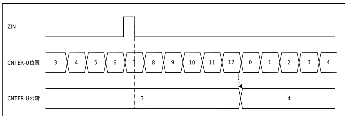
图 23-18 公转计数模式-位置溢出计数
