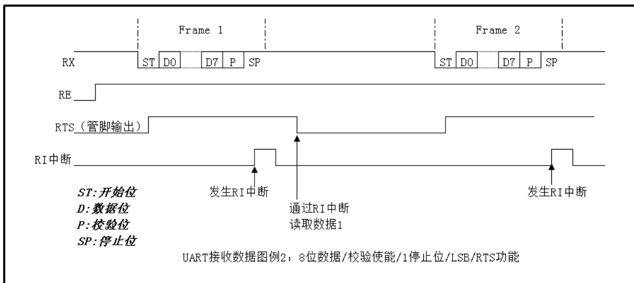
图 27-7 UART 接收数据图例 2
