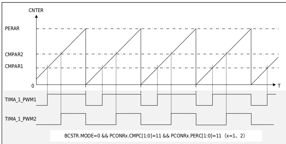
图 23-10 单边对齐 PWM 输出例
