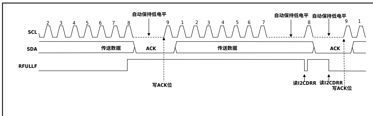
图 28-13 快速 ACK/NACK 时序图
