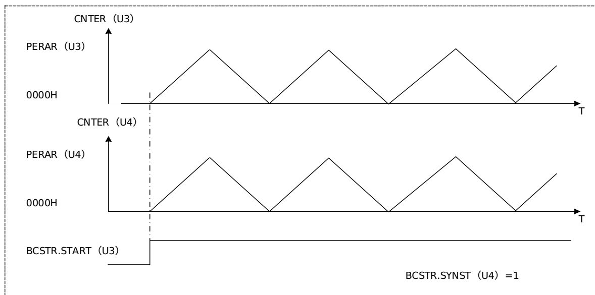
图 23-6 软件同步动作
