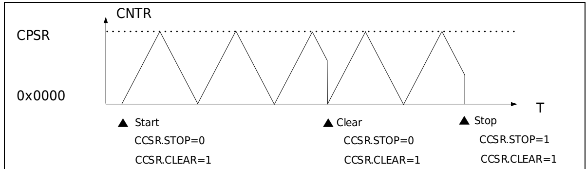
图 21-5 Timer4 三角波模式计数动作
