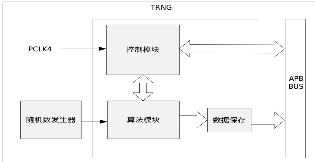
图 39-4 TRNG 系统框图
