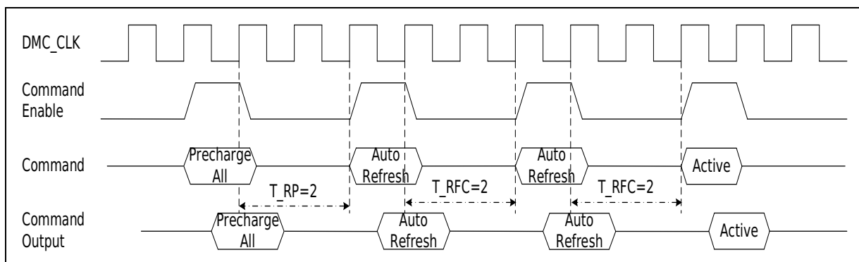
图 37-26 命令方式预充电
