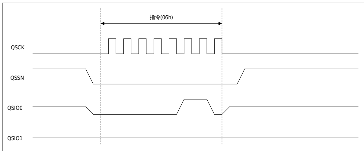
图 30-26 写许可指令总线周期示意图
