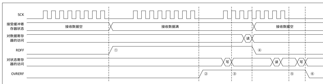
图 29-10 过载错误处理
