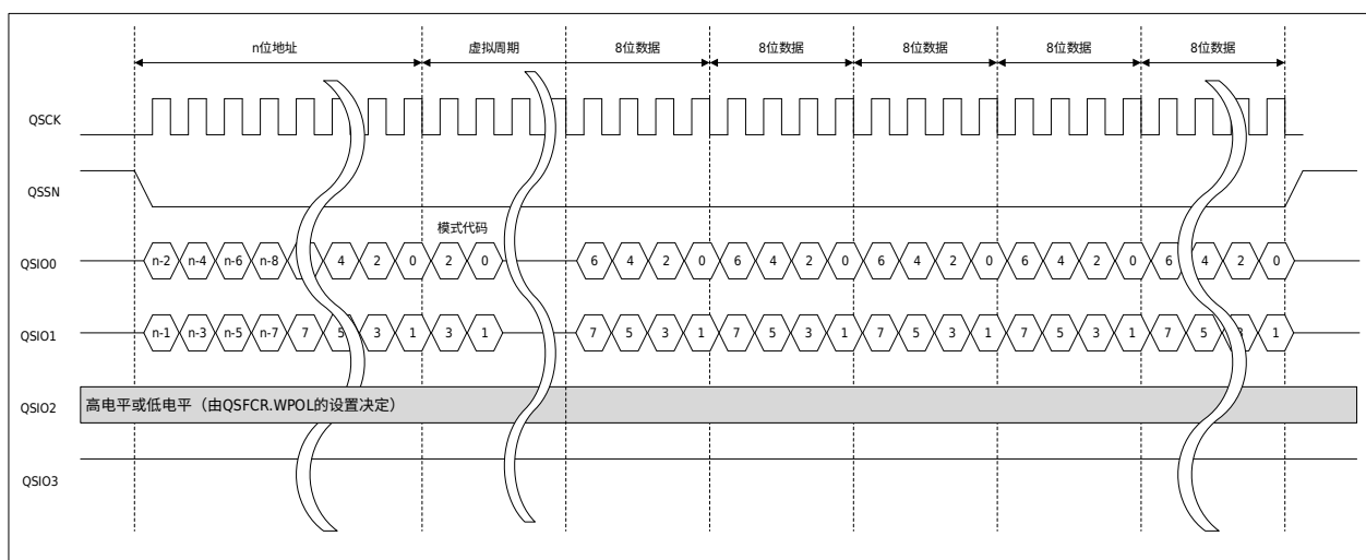
图 30-19 选择 XIP 模式的二线式输入输出快速读总线周期示意图
