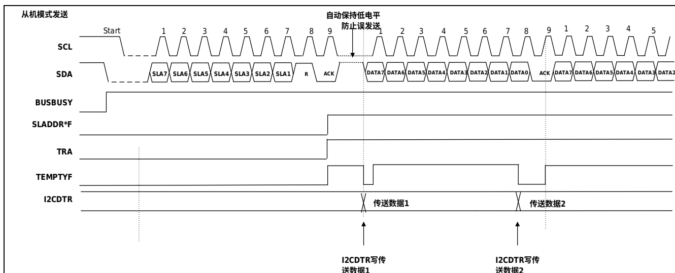
图 28-10 从机发送时序图 (1)
