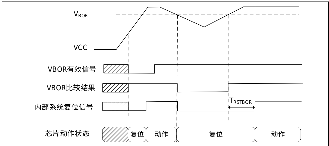
图 3-3 欠压复位
