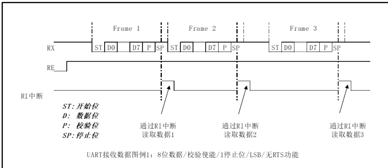
图 27-6 UART 接收数据图例 1
