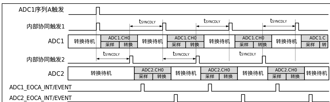
图 17-16 循环延迟触发模式 (两 ADC)
