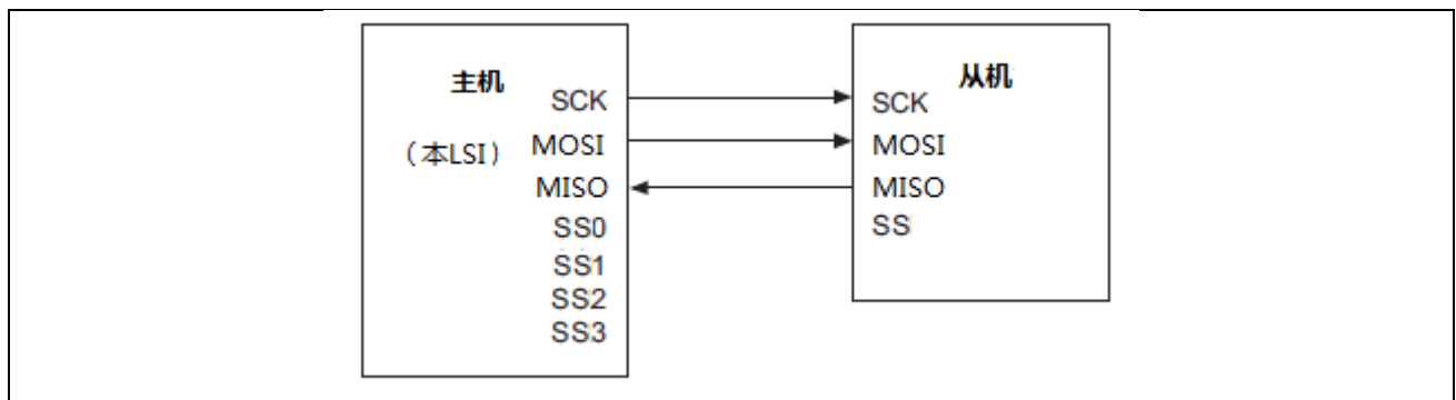
图 29-3 三线式时钟同步运行
