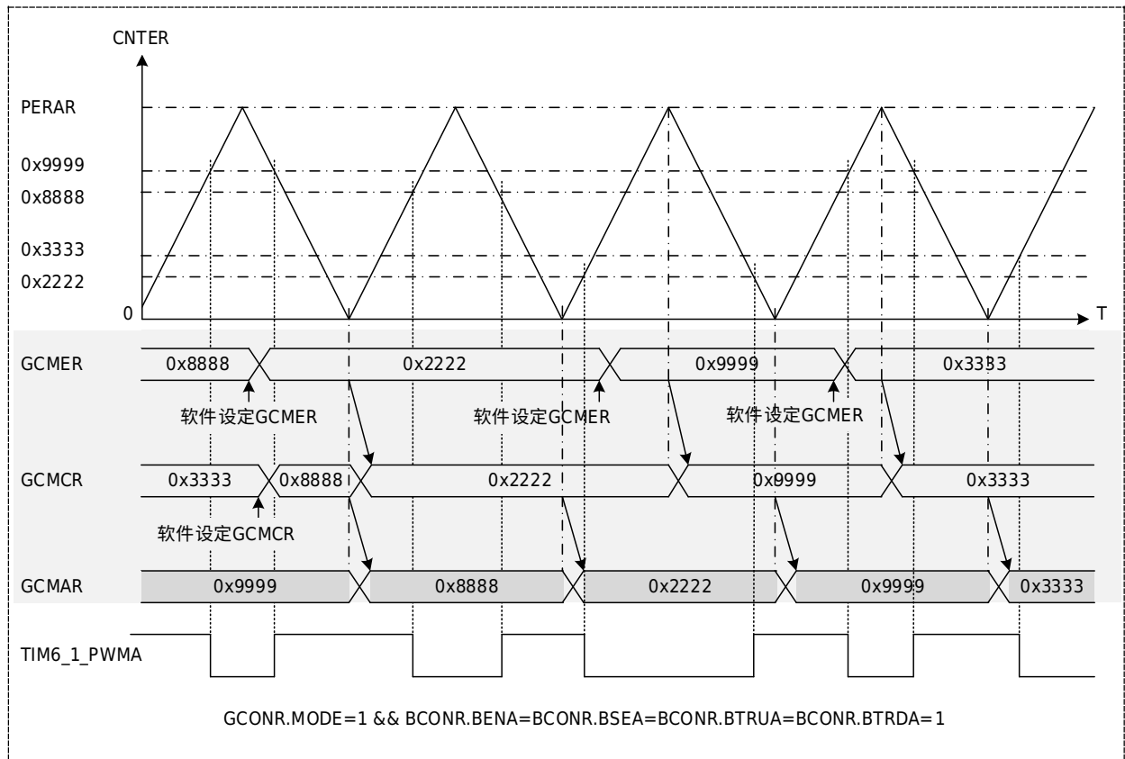
图 20-15 三角波模式时计数缓存动作 2
