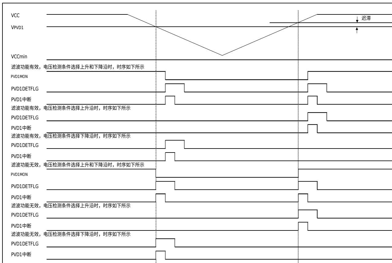
图 5-7 电源监视 1 中断时序图
