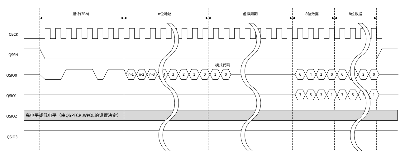
图 30-16 二线式输出快速读总线周期示意图
