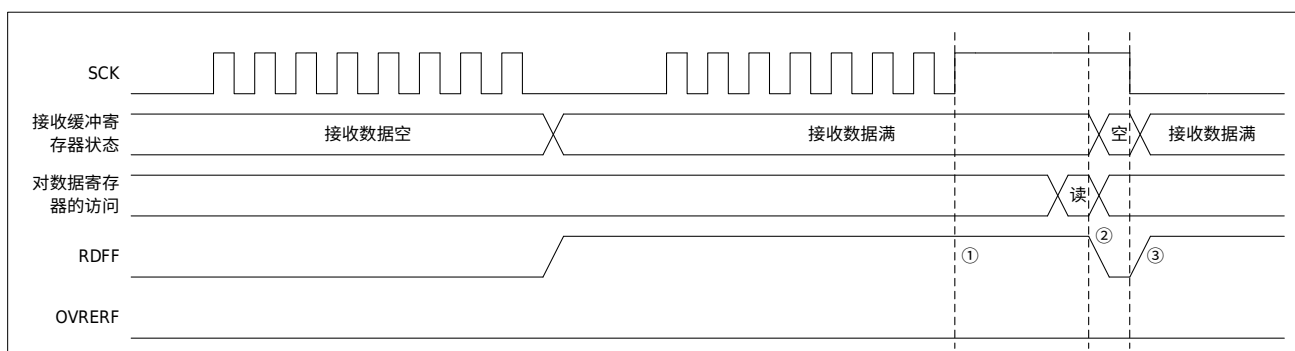
图 29-11 启用时钟自动停止功能时的动作示意图 (CPHA=1)
