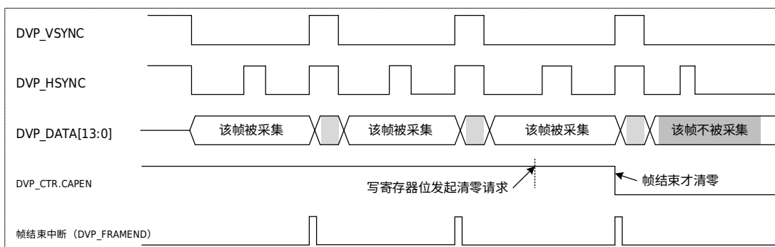
图 38-4 连续模式数据采集动作
