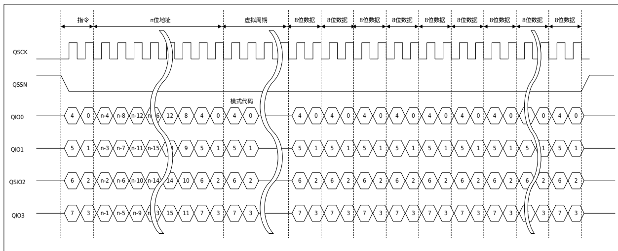
图 30-7 四线式 SPI 协议动作示意图（快速读模式）
