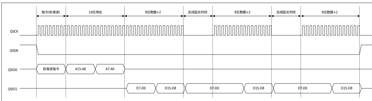
图 30-32 使用 QSPI 总线周期延长功能的数据读取操作示意图
