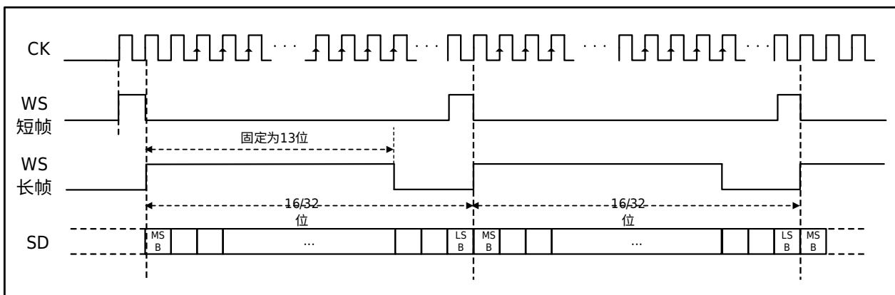
图 31-11 I2S PCM 协议波形（16/32 位全精度）
