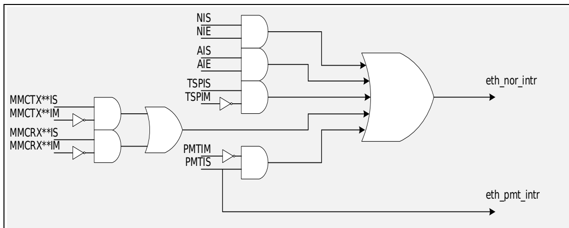
图 36-21 ETHMAC 中断方案
