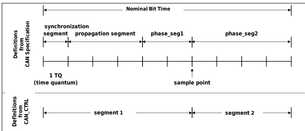
图 34-2 CAN 位时间定义图
