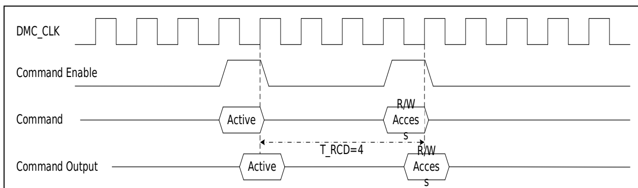
图 37-25 行激活到读写操作时序
