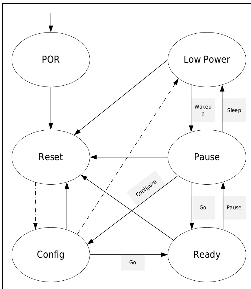
图 37-29 DMC 状态图
