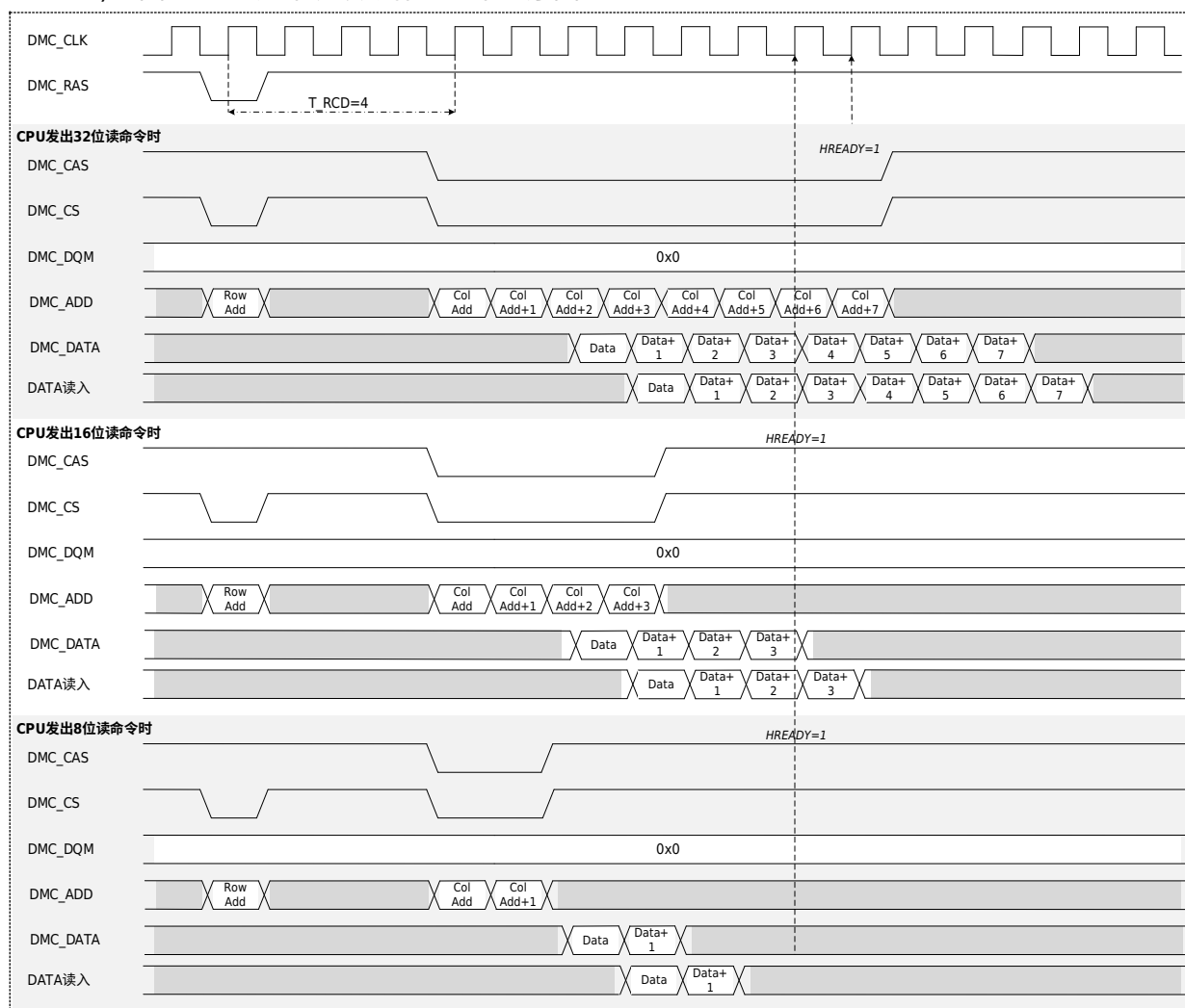
图 37-31 单次读动作基本时序（16 位宽（DMCMW=00））
