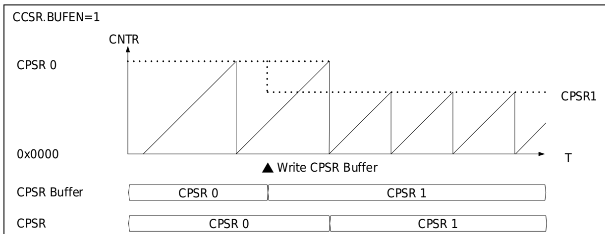
图 21-9 缓存使能时修改锯齿波计数周期
