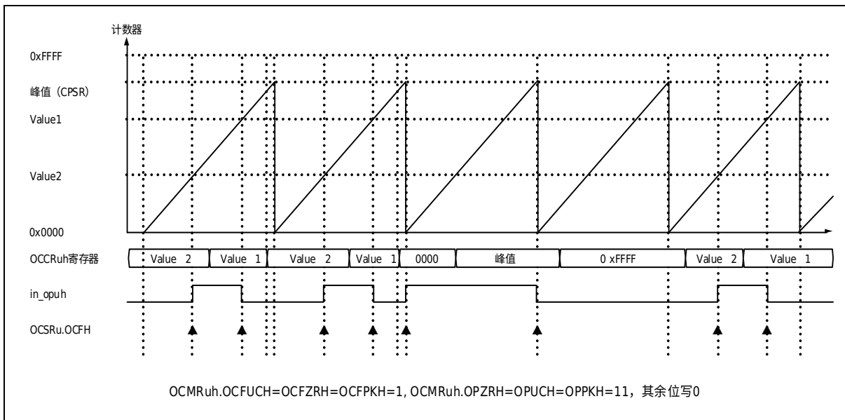
图 21-16 锯齿波独立 PWM 输出例
