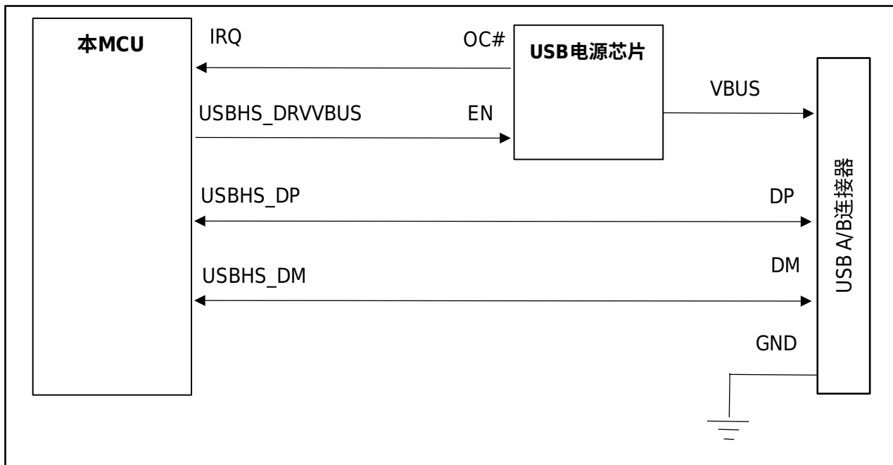
图 32-2 USBHS 主机模式系统构建图
