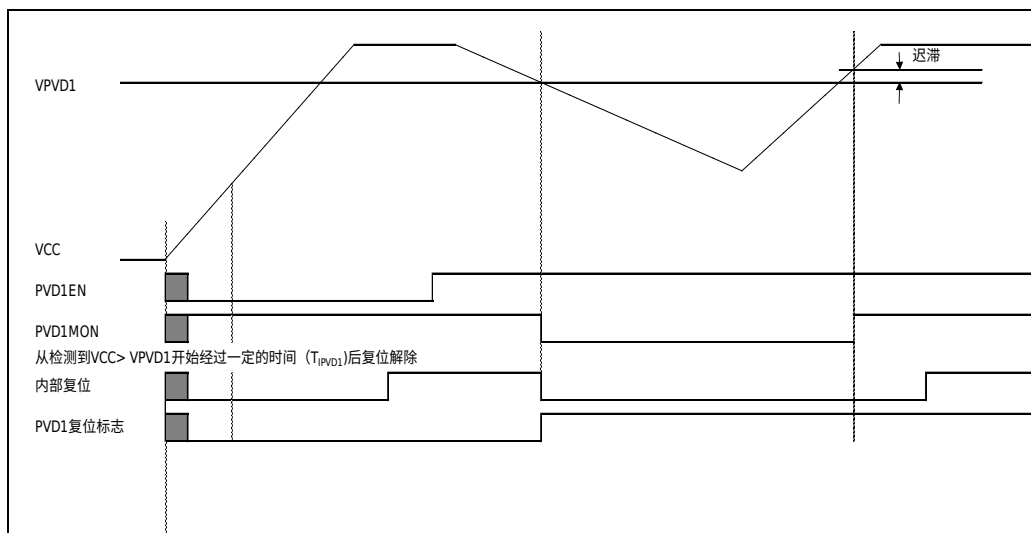
图 5-8 电源监视 1 复位时序图
