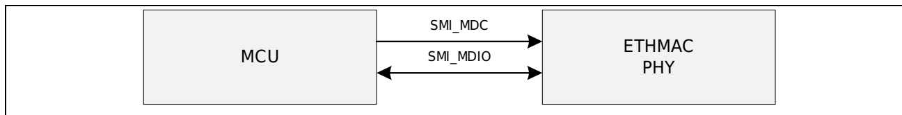
图 36-4 SMI 接口连接图
