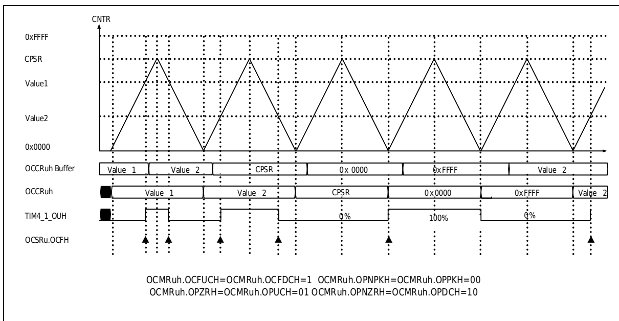
图 21-17 三角波独立 PWM 输出例
