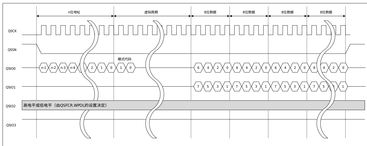
图 30-17 选择 XIP 模式的二线式输出快速读总线周期示意图
