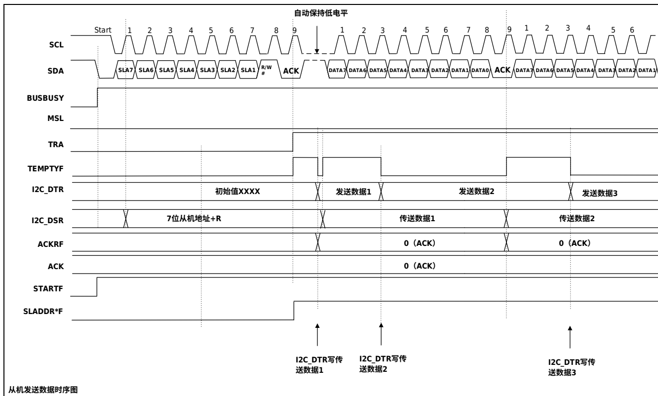
图 28-7 7 位地址格式的从机发送模式时序图（例）
