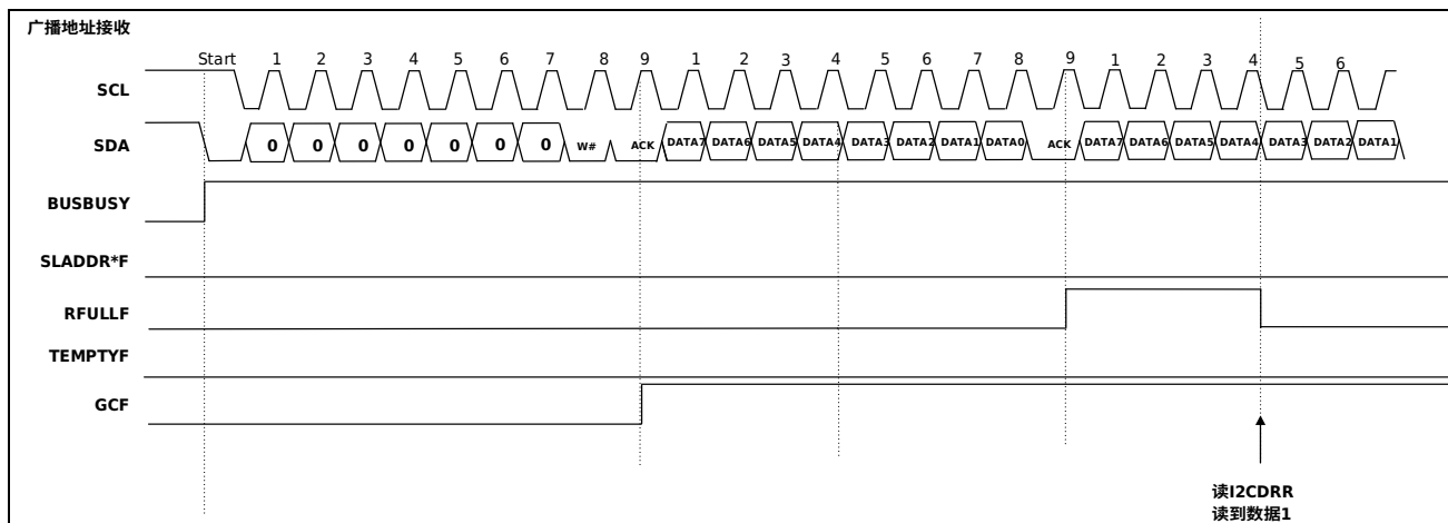
图 28-16 广播地址接收时序图
