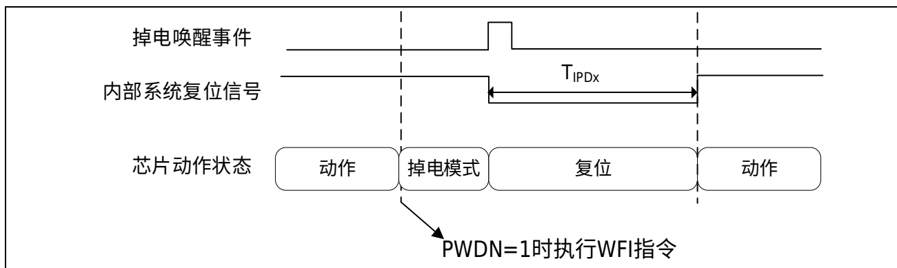
图 3-7 掉电唤醒复位
