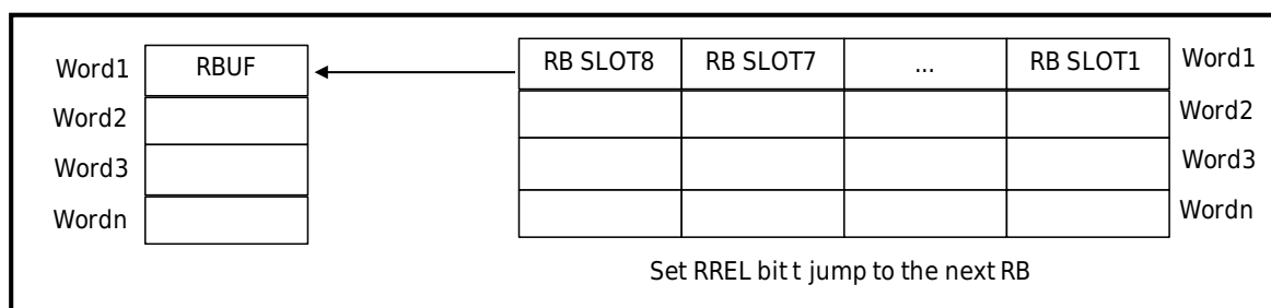
图 34-4 CAN RBUF 寄存器读接收缓冲器示意图
