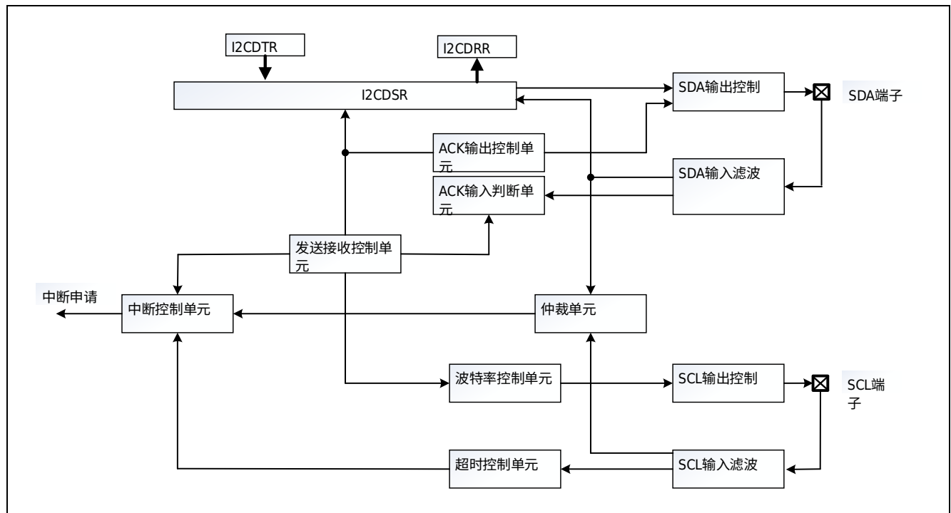
图 28-1 I2C 系统框图
