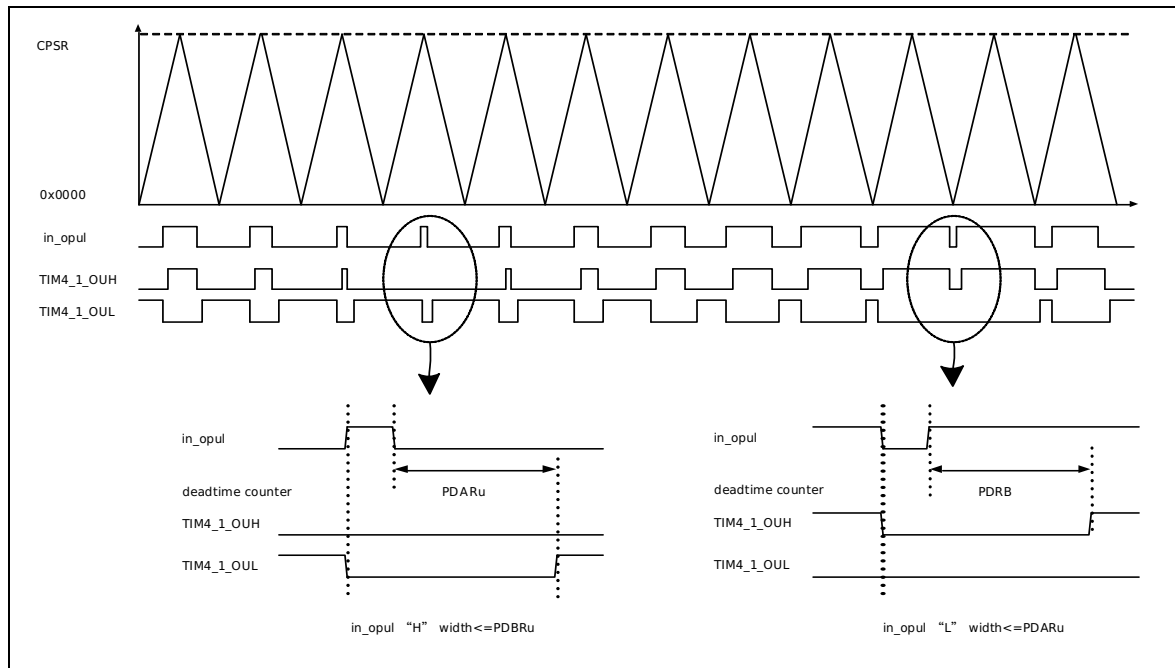
图 21-21 脉宽异常时的死区定时器模式下的波形输出
