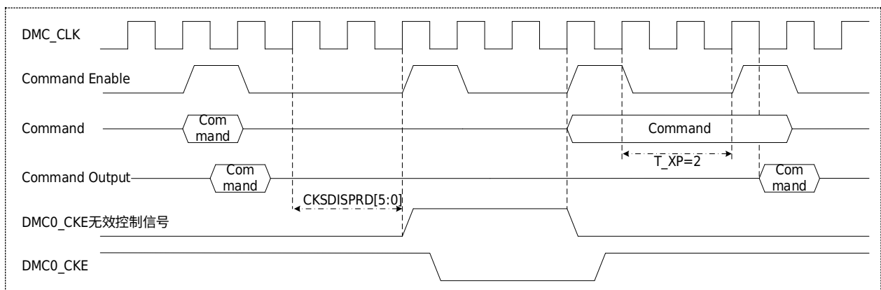
图 37-35 DMC_CKE 端口输出控制时序
