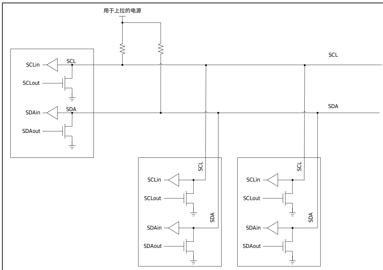
图 28-2 I2C 总线的结构例
