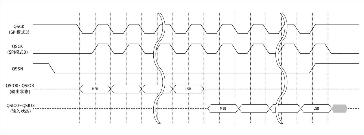
图 30-8 串行接口的基本时序图
