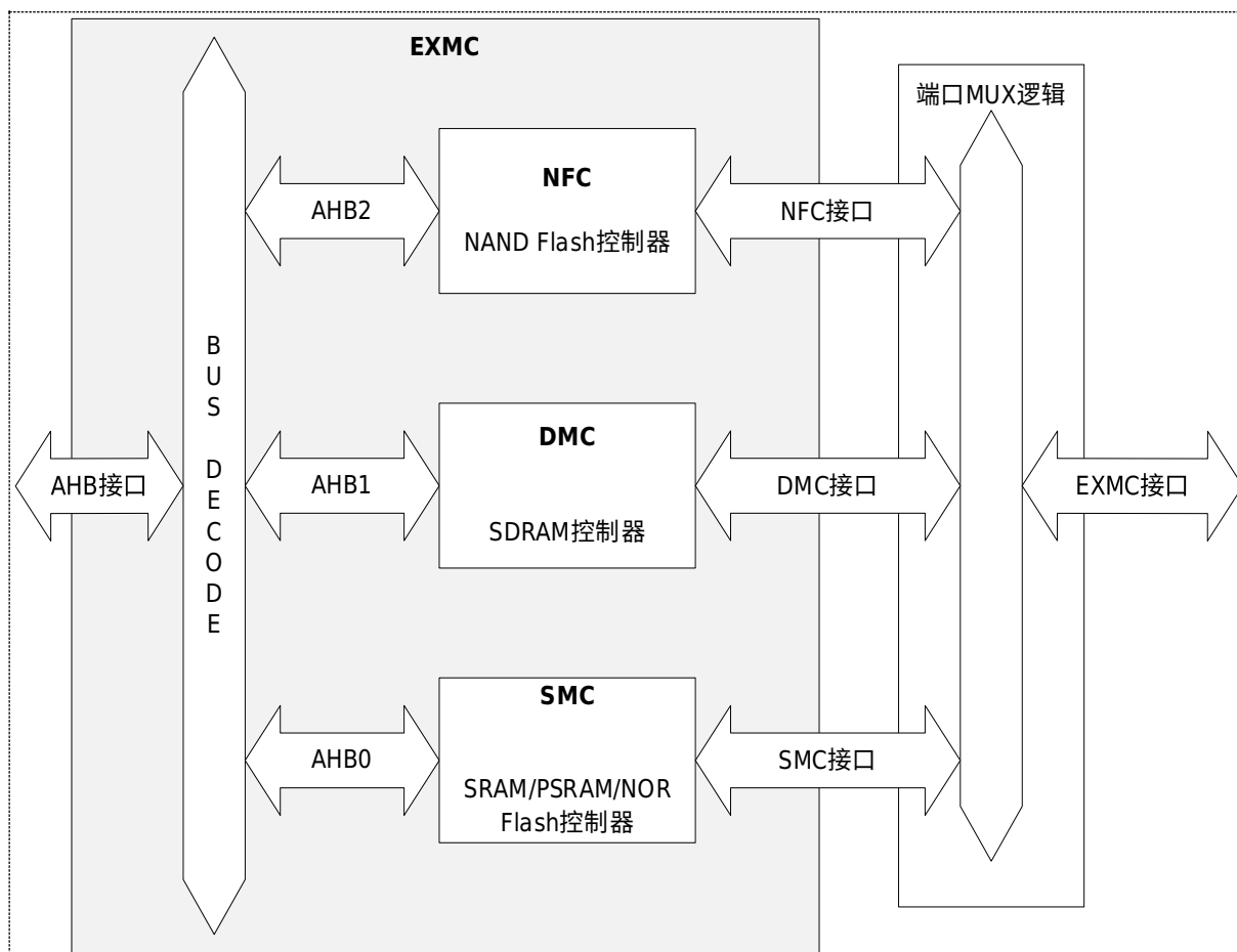
图 37-1 EXMC 架构图
