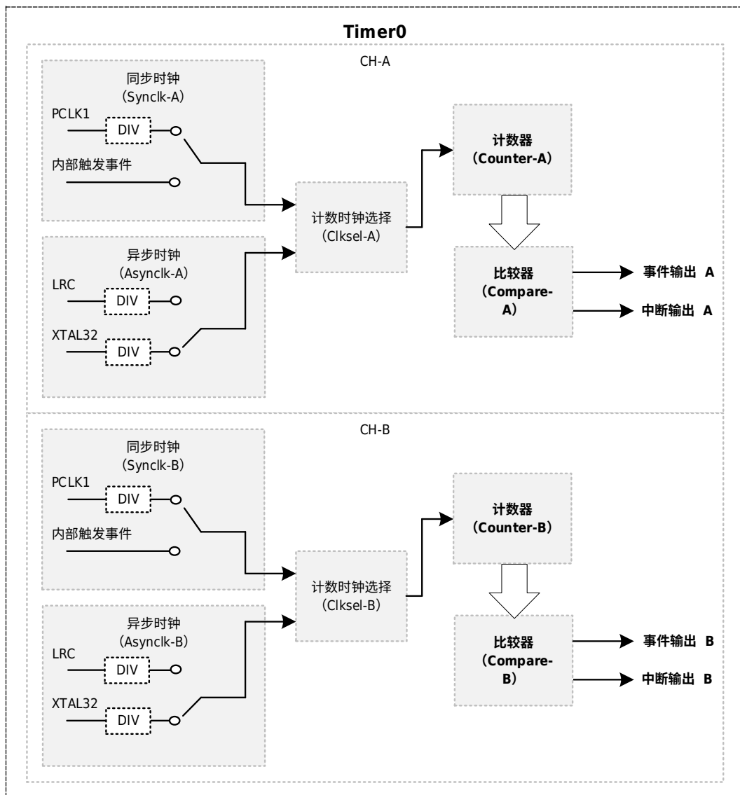
图 24-1 Timer0 基本框图
