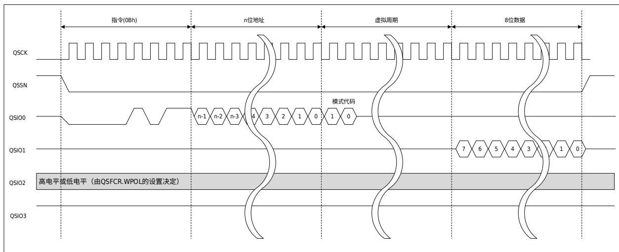
图 30-14 快速读总线周期示意图
