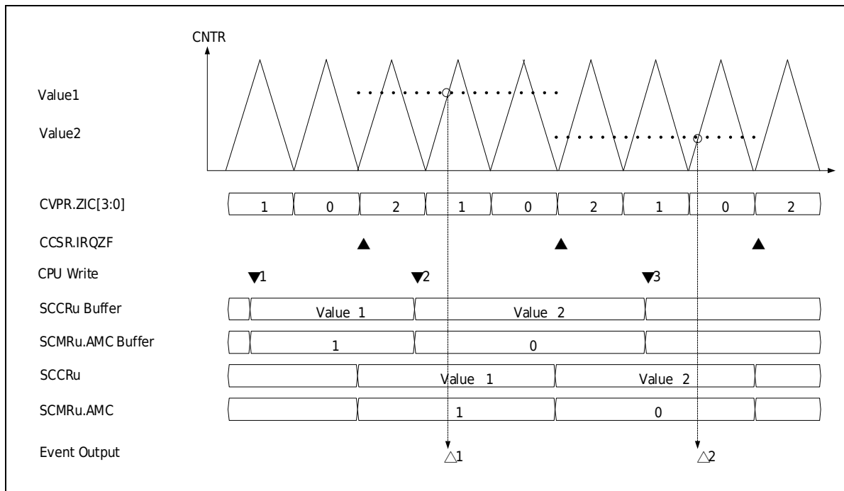
图 21-24 专用事件输出信号周期间隔响应输出
