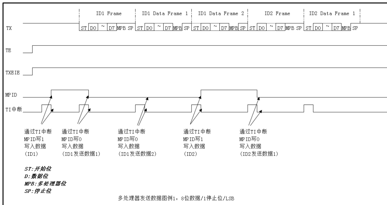
图 27-10 多处理器模式发送数据图例
