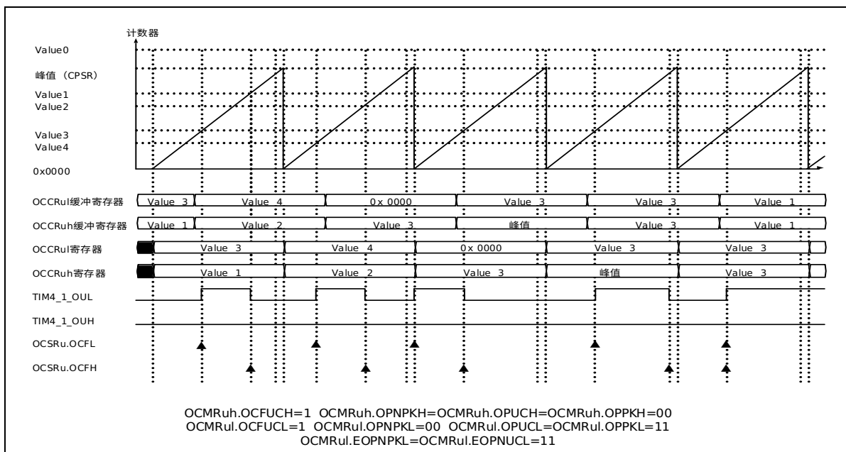
图 21-18 三角波扩展 PWM 输出
