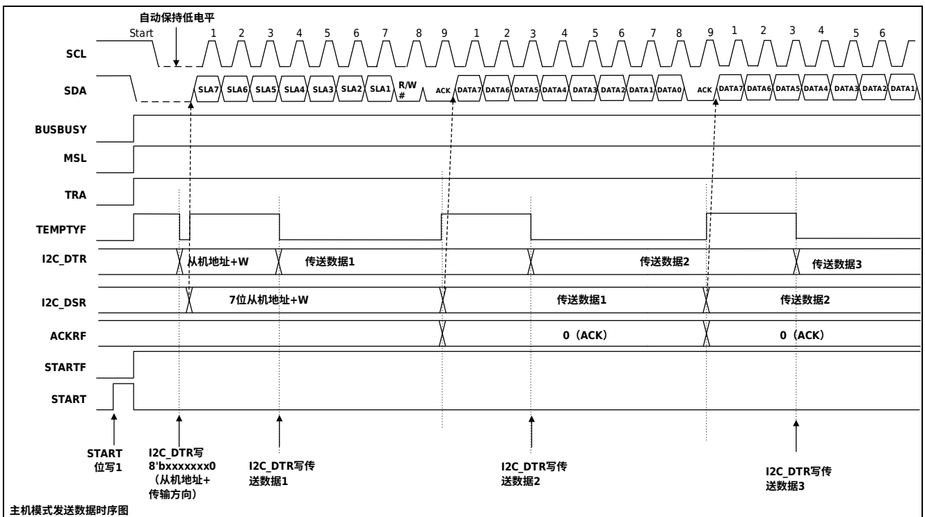
图 28-5 7 位地址格式的主机发送数据时序图（例）
