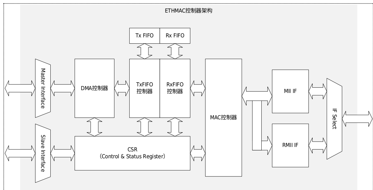
图 36-1 以太网 MAC 控制器架构图
