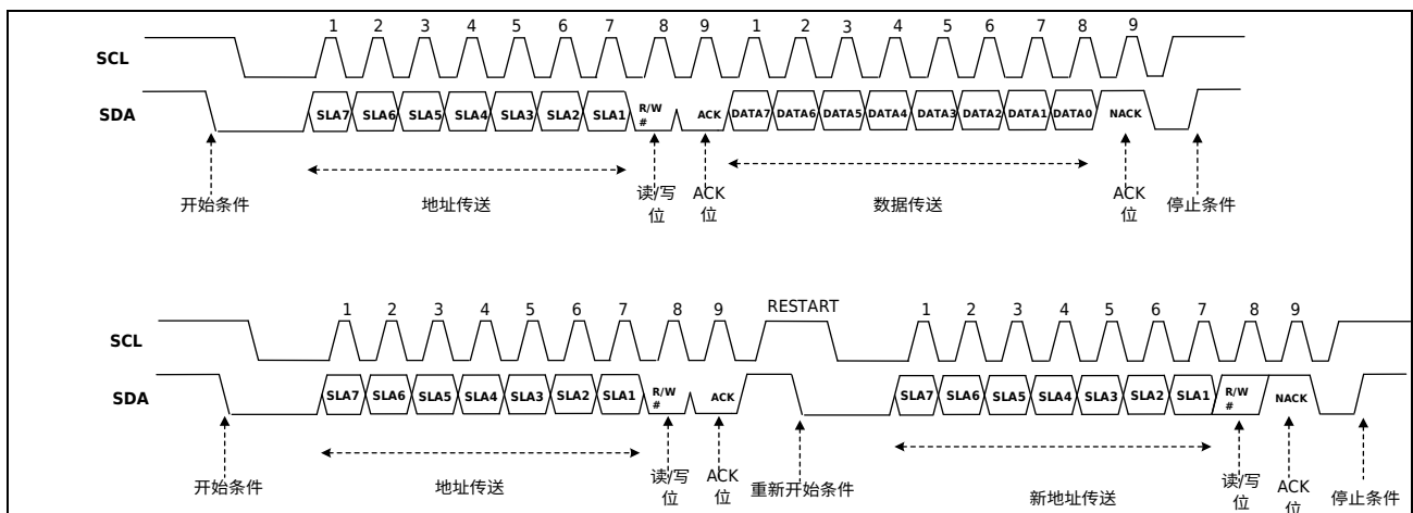
图 28-3 I2C 总线的时序图
