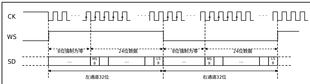
图 31-10 I2S LSB 协议波形（24 位数据封装在 32 位帧中）
