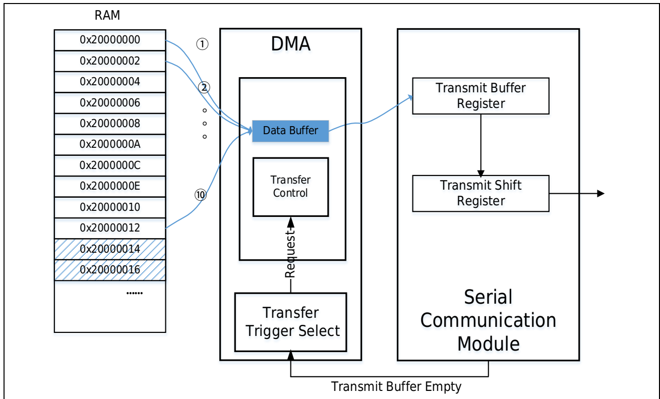
图 15-6 应用例 2：存储器到外围电路的传输
