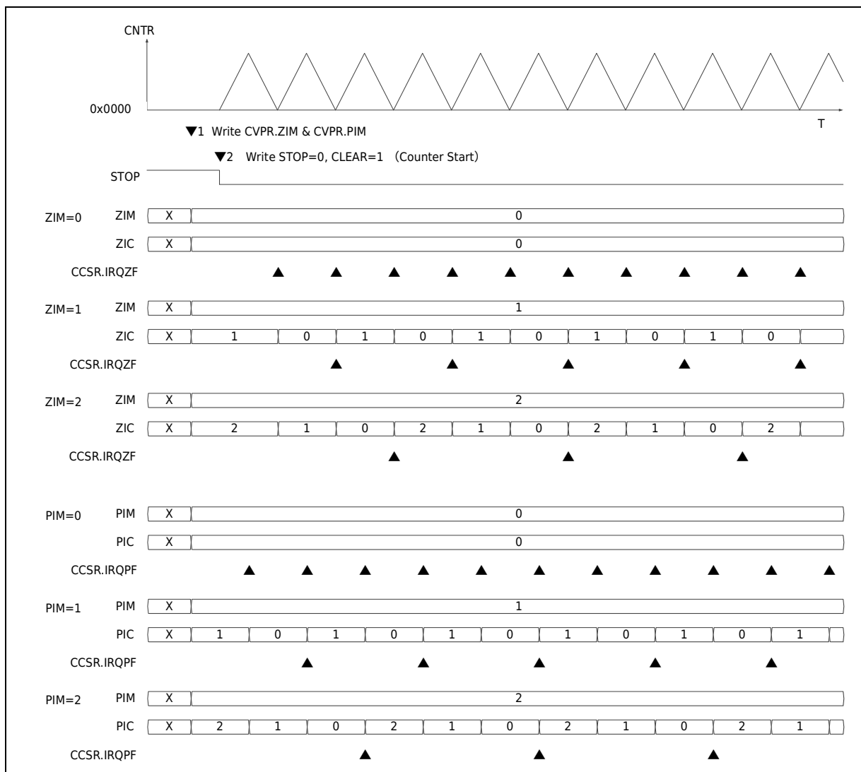
图 21-23 周期间隔响应时序图
