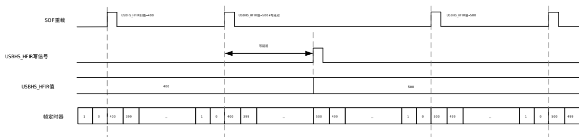
图 32-4 USBHS 动态更新 USBHS_HFIR 寄存器示意图
