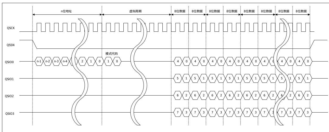
图 30-21 选择 XIP 模式的四线式输出快速读总线周期示意图
