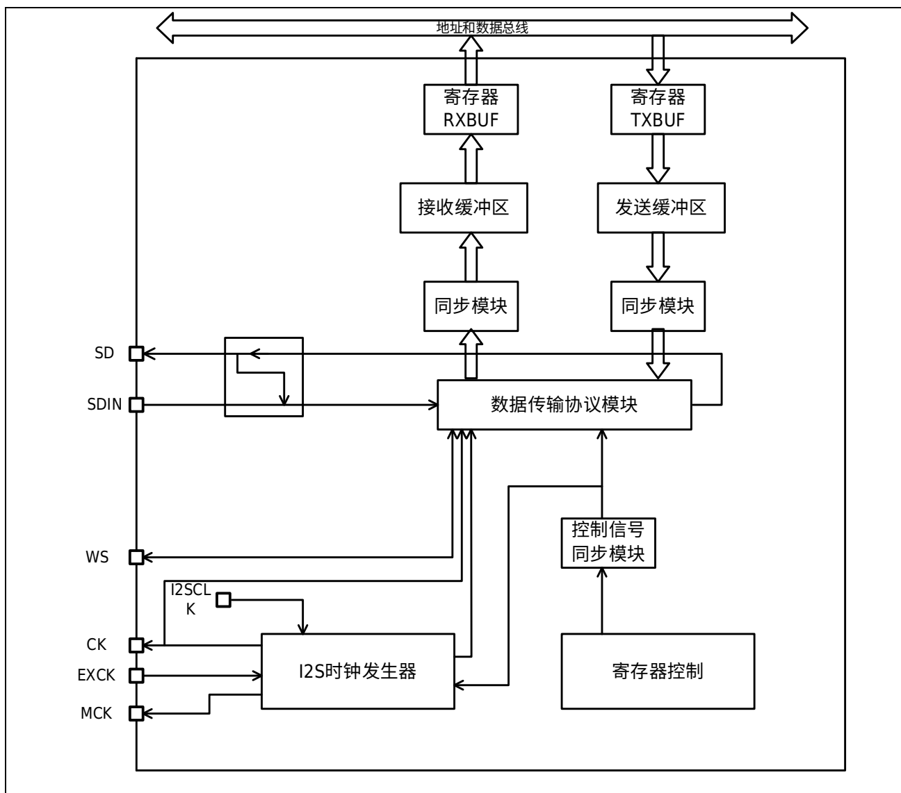
图 31-1 I2S 系统框图
