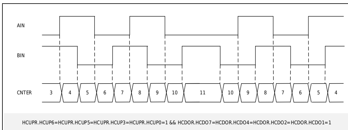
图 23-15 位置计数模式-相位差计数（4 倍计数）
