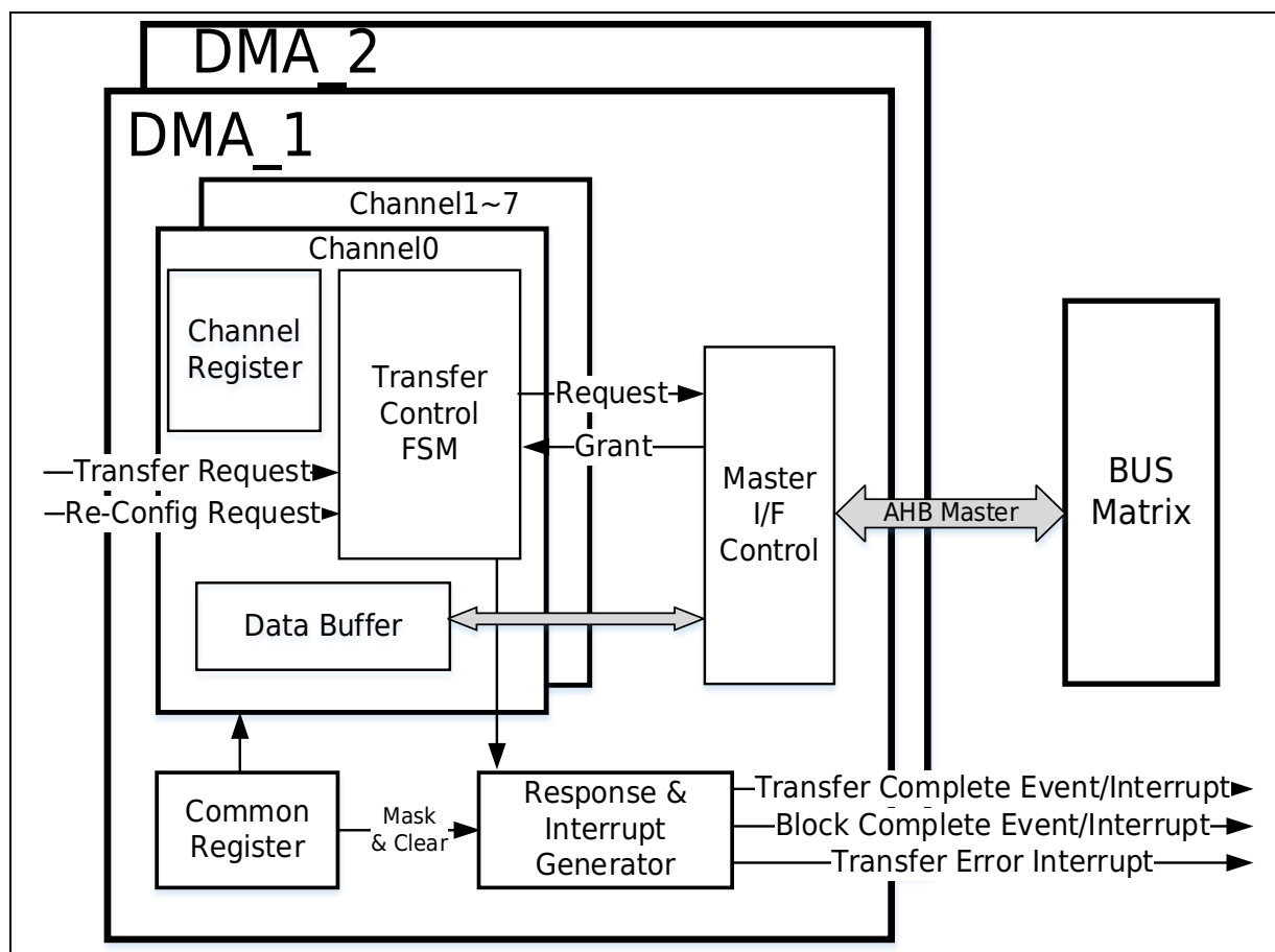
图 15-1 DMA 结构图
