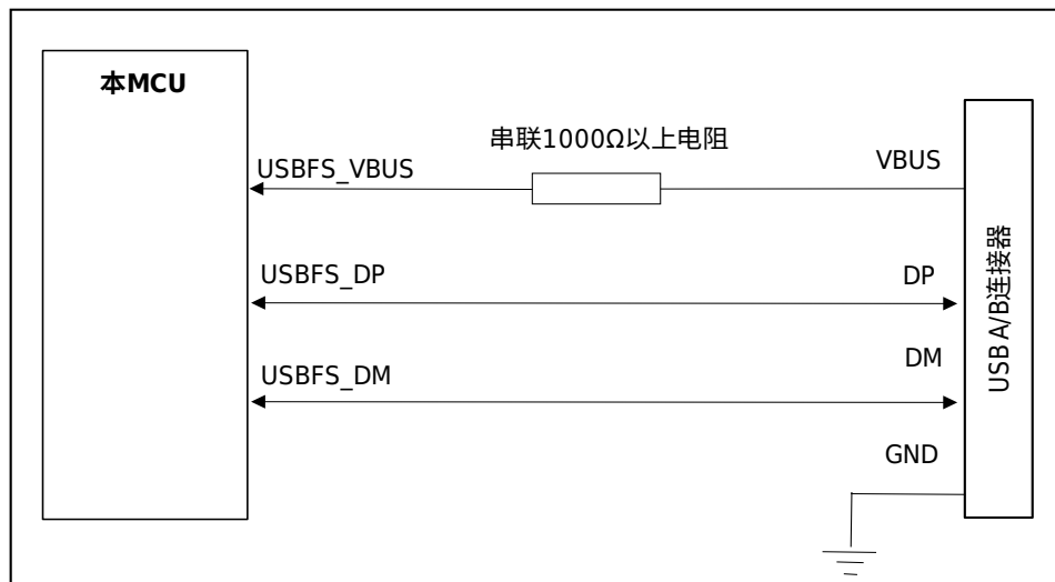
图 33-3 USBFS 设备模式系统构建图
