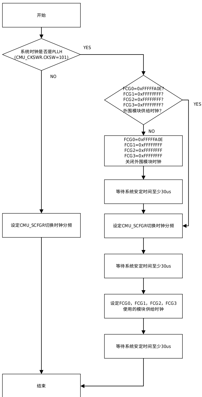
图 4-10 时钟分频切换
