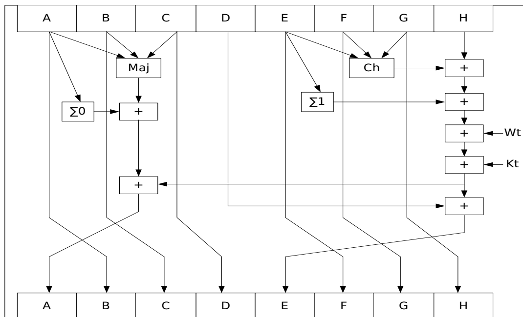
图 39-3 HASH 算法流程图
