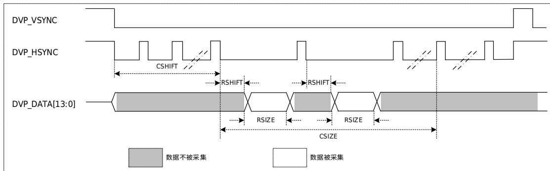
图 38-7 窗口裁剪数据采集图
