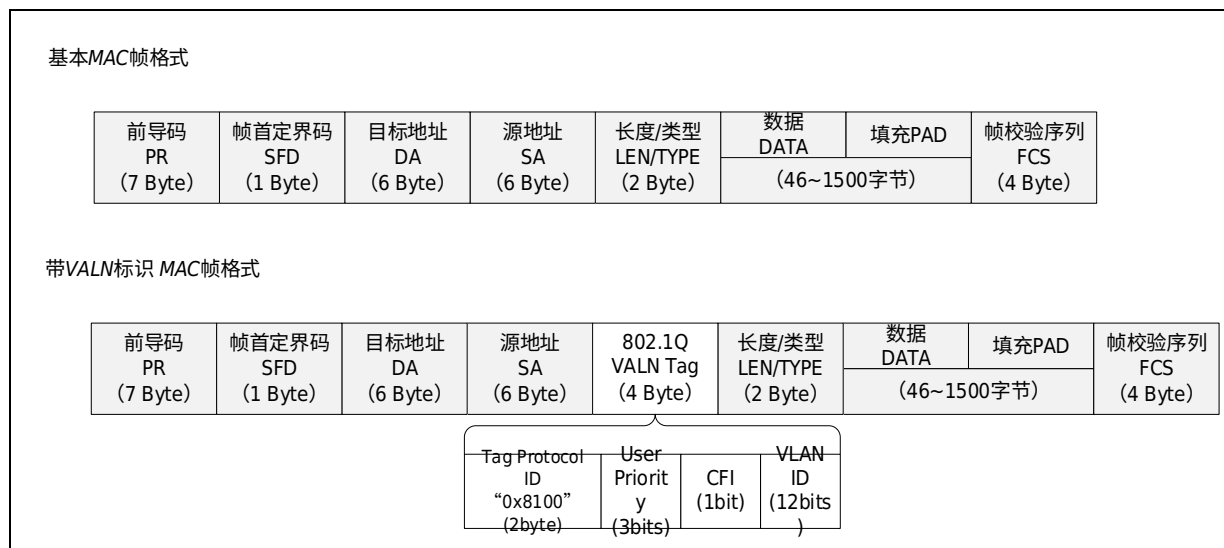
图 36-5 MAC 帧结构
