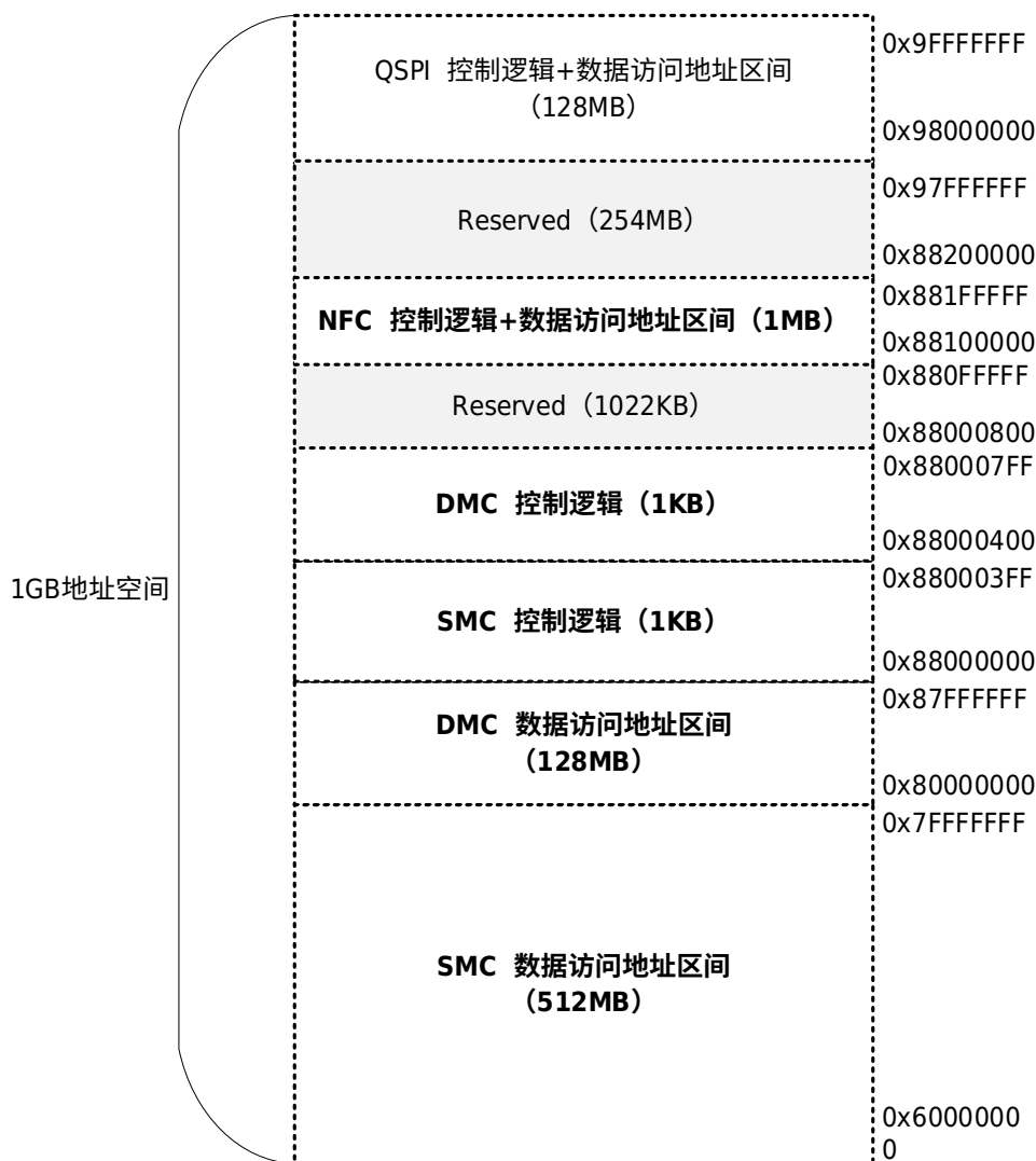
图 37-2 外部空间地址分配
