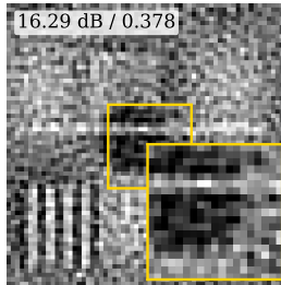
Wiener
