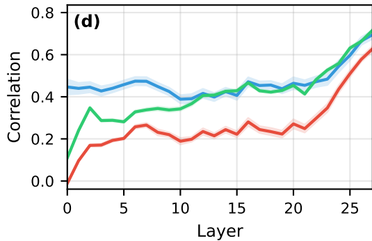
InternVL3-2B
