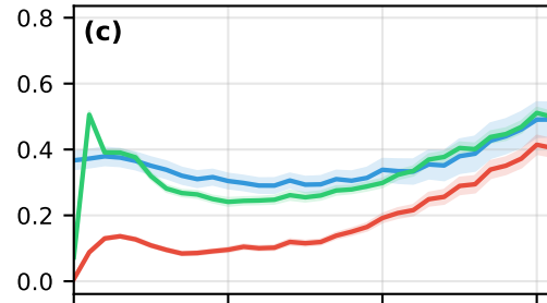
LLaVA-1.5-7B
