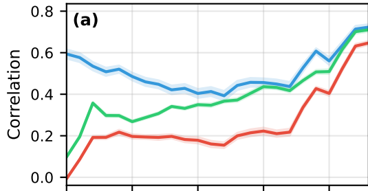
InternVL3-1B
