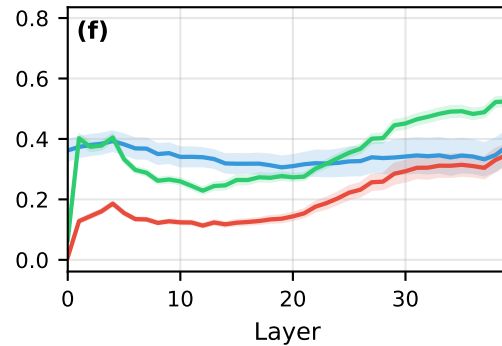
LLaVA-1.5-13B
