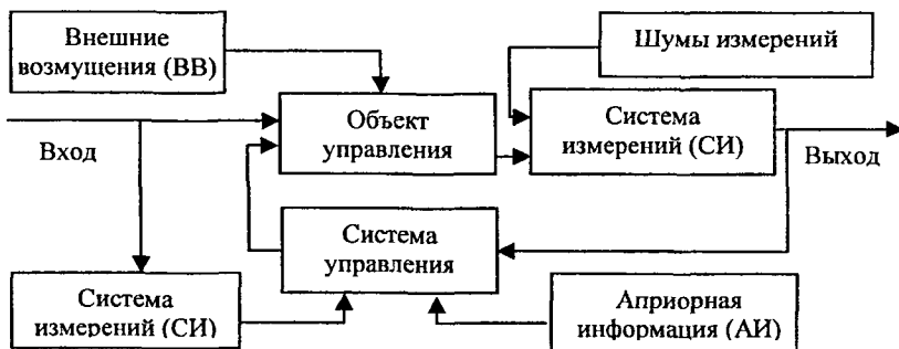
Рис 2 Схема информационных потоков системы управления
