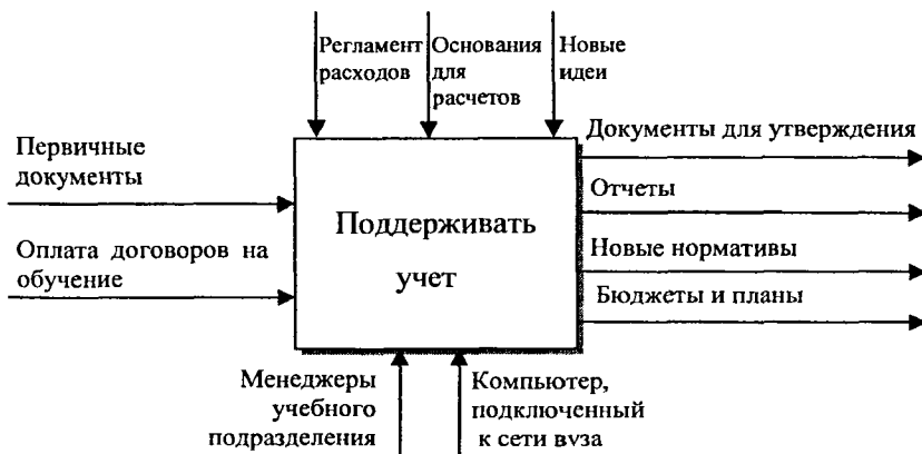
Рис. 3 Первый уровень функциональной модели УУ ВОД
