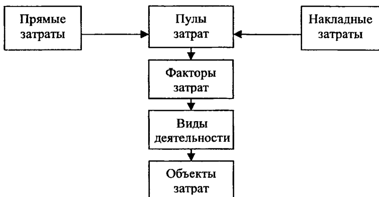
Рис. 4 Графическое представление метода ABC
