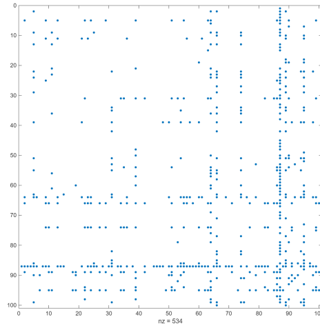
Figura 1: Sparsità del complementare della matrice di adiacenza del grafo sp_500_2022_2023 di densità 93%. In blu sono indicati gli elementi non nulli del complementare (e quindi quelli nulli della matrice di adiacenza). Per semplicità e chiarezza è visibile solo il minore principale dettato dalle prime 100 colonne e dalle prime 100 righe.
