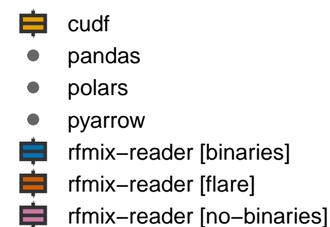
Parser
