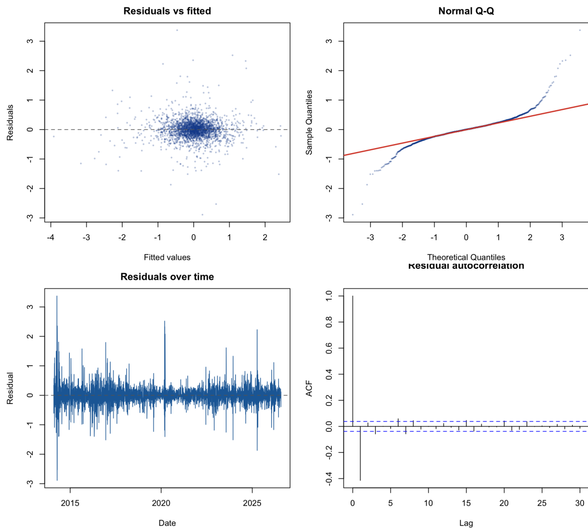
图 2：未修正初步 OLS 模型的残差-拟合值、Q-Q、时间顺序与自相关图。
