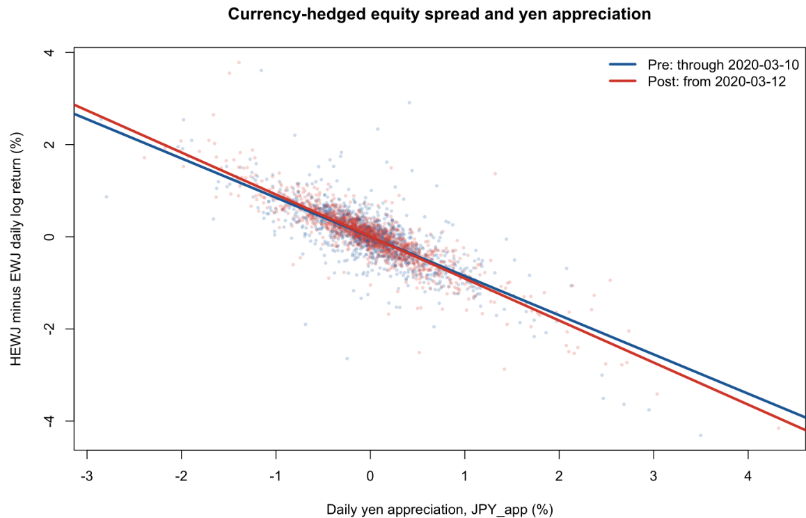
图 1：日元升值与 HEWJ-EWJ 日度收益差，以及分时期 OLS 斜率。
