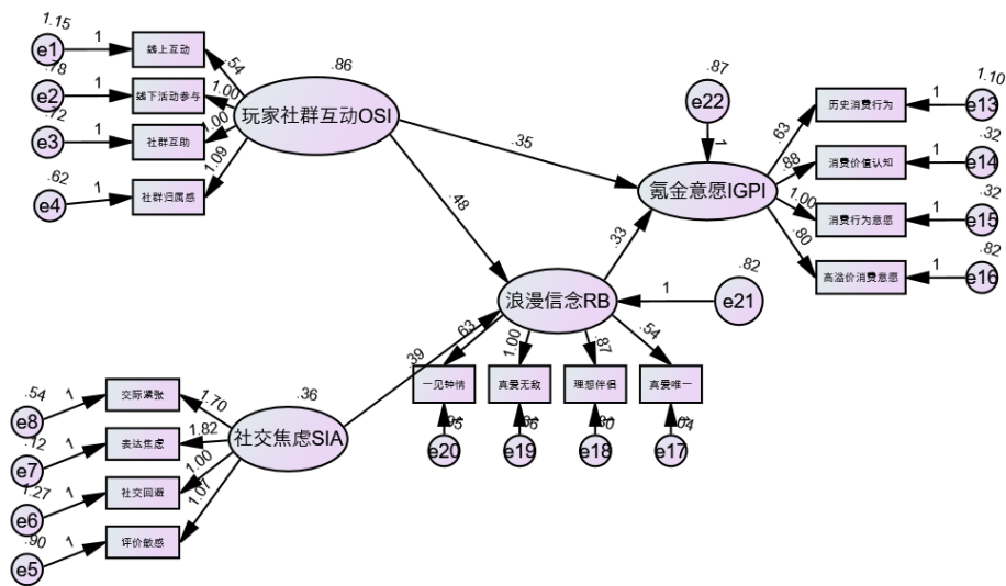
图 4 研究成果：以 RB 为关键的国乙玩家模型
