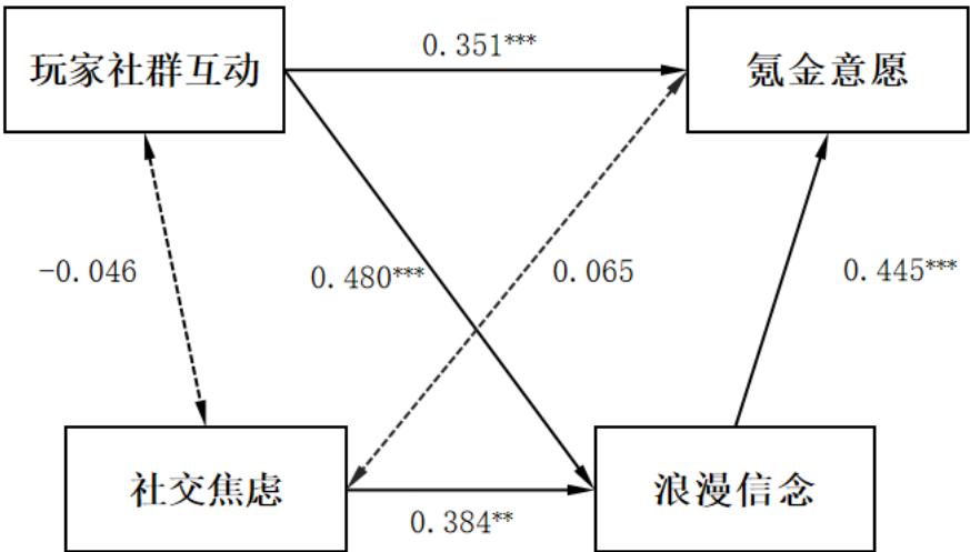
图 5 乙游玩家的玩家社群互动、社交焦虑、浪漫信念、氪金意愿的显著路径
