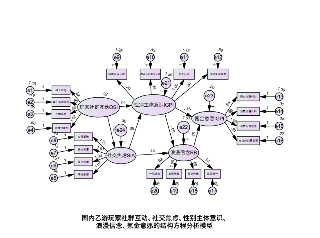
图 2 五变量假设的验证
