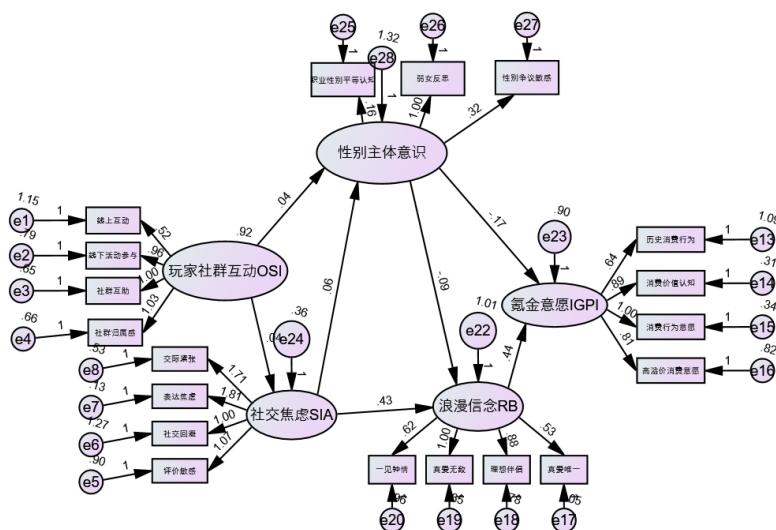
图 3 删掉可能误差 FIC1 后的五变量假设结构方程模型
