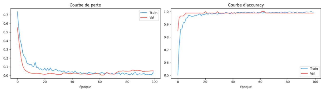
Figure 1.3 — Courbes de perte et d'accuracy train/Val (MLP final, 100 époques)
