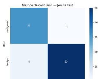
Figure 1.5 — Matrice de confusion sur le jeu de test
