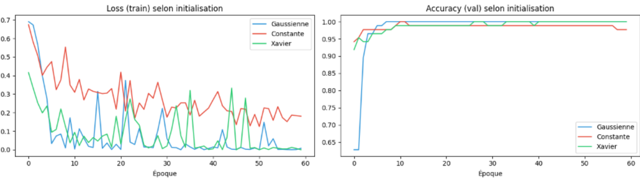
Figure 1.2 — Loss et accuracy selon la stratégie d'initialisation (Gaussienne / Constante / XaVier)
