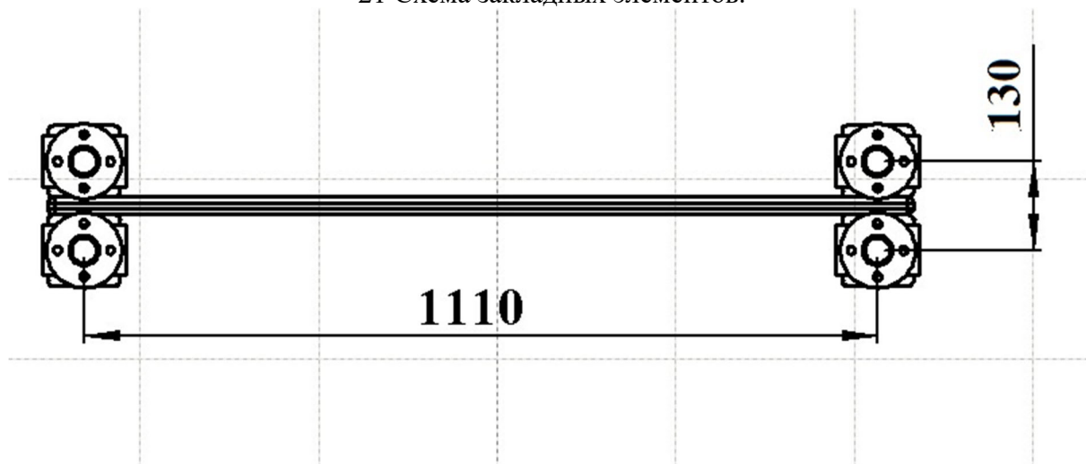
21 Схема закладных элементов.
