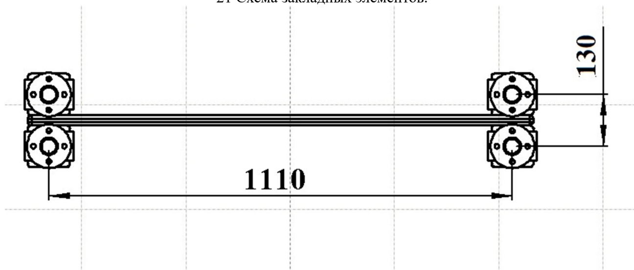
21 Схема закладных элементов.
