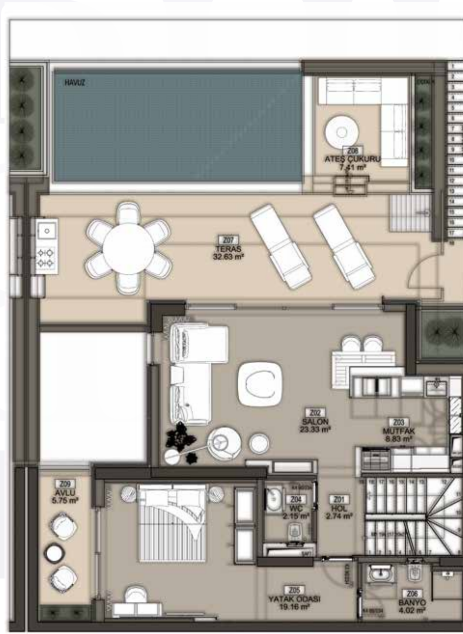
B Blok Zemin Kat Planı
