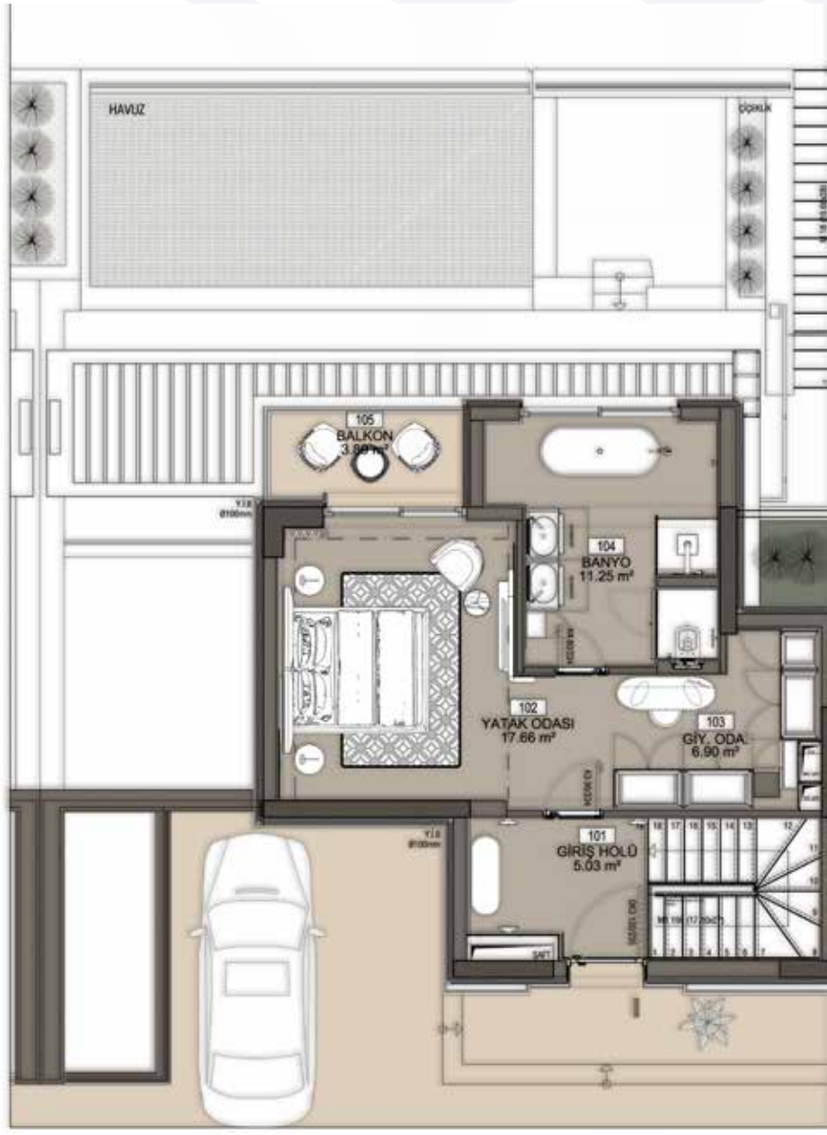
B Blok Birinci Kat Planı
