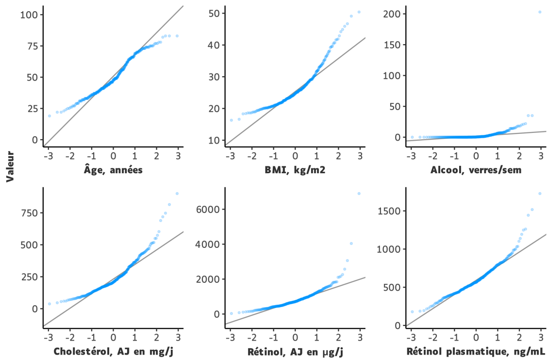
Figure 2. – Diagrammes Q-Q. Distribution théorique en abscisses, distribution observée en ordonnées. n : nombre d'évènements ; BMI : indice de masse corporelle ; AJ : apport journalier.
