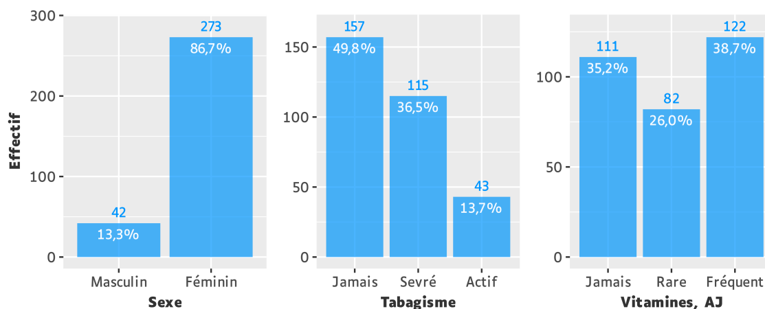
Figure 1. – Caractéristiques des variables qualitatives. n : nombre d'événements ; AJ : apport journalier.
