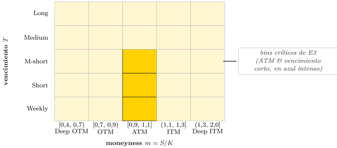
Figura 5: Partición 5 \times 5 del dominio en bins de moneyness y vencimiento. Los bins ATM combinados con weekly, short y medium-short (sombreados en amarillo intenso) son los bins donde se ha centrado el muestreo en el experimento 3.
