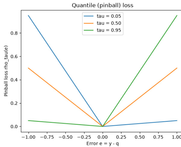
Figura 46. Pérdida cuantílica para \tau = 0.05, 0.50 y 0.95 . Su asimetría es la que hace que el minimizador sea el cuantil \tau .
