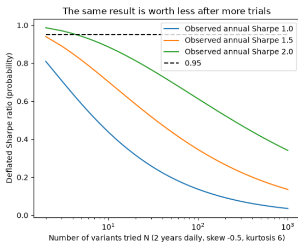
Figura 75. Sharpe deflactado de un mismo resultado observado según el número de variantes probadas (supuestos en el eje).
