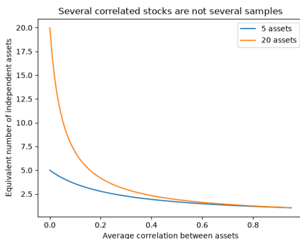
Figura 72. Activos independientes equivalentes según la correlación media. Cinco acciones con correlación 0.6 equivalen a menos de dos.
