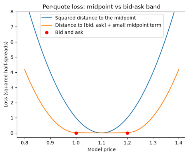
Figura 11. Pérdida de una cotización con bid 1.00 y ask 1.20. La pérdida cuadrática al mid penaliza precios perfectamente compatibles; la distancia a la banda es casi nula dentro del intervalo y crece fuera de él.
