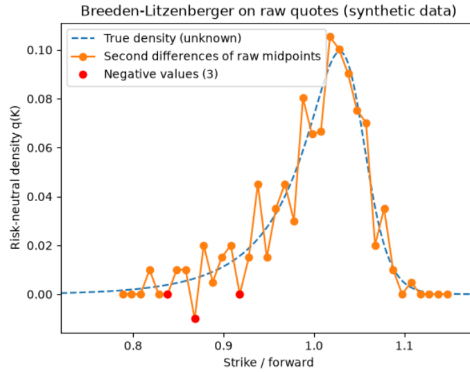
Figura 17. Segundas diferencias de los mid crudos (mundo sintético con strikes cada punto). La curva discontinua es la densidad verdadera, desconocida en la práctica; los puntos rojos son valores negativos, imposibles para una densidad.
