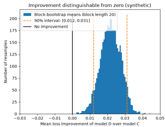
Figura 76. Distribución bootstrap de la mejora media del modelo D sobre el C (serie sintética con autocorrelación). El intervalo del 90 % excluye el cero.
