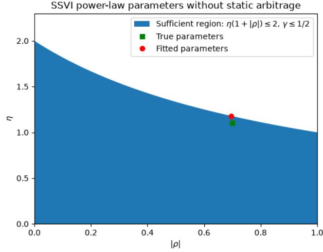
Figura 13. Región suficiente de la función de potencia en el plano (|\rho|, \eta) con \gamma \leq 1/2 . El cuadrado es el valor verdadero del mundo sintético; el círculo, el ajuste, que queda en la frontera.
