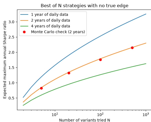
Figura 74. Sharpe anual máximo esperado entre N estrategias sin ninguna ventaja real. Con dos años de datos diarios y cien variantes, el mejor resultado ronda 1.8 por puro azar; los puntos confirman la aproximación por simulación.
