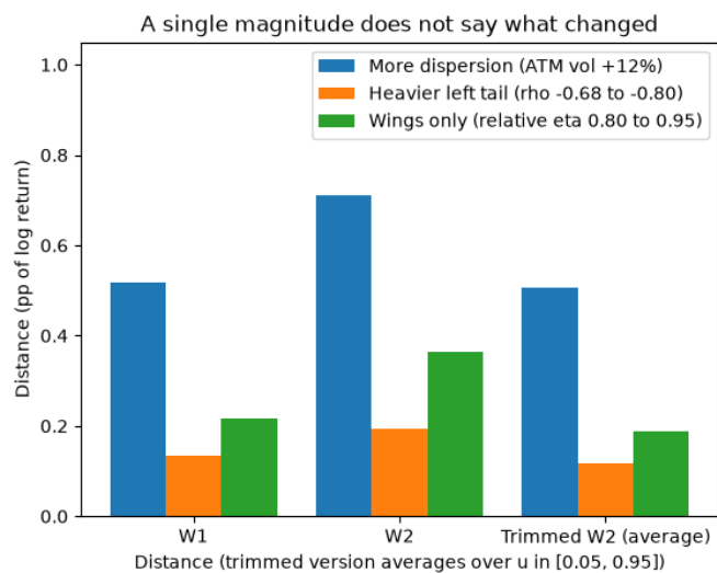
Figura 25. Distancias de los tres arquetipos. W_2 pesa más el cambio en las alas que W_1 ; la versión recortada casi no lo ve. Ninguna cifra aislada identifica el tipo de cambio.
