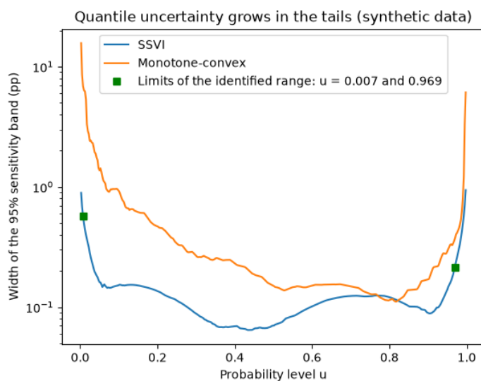
Figura 20. Ancho de la banda de sensibilidad de cada cuantil. Los cuadrados marcan el rango identificado [u_{\min}, u_{\max}] , definido por los strikes fiables más extremos; fuera de él los cuantiles se reportan como no identificados.
