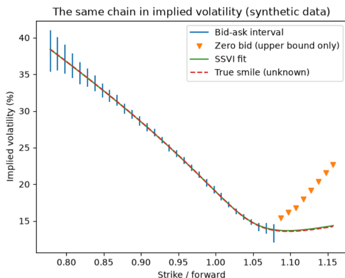
Figura 10. La misma cadena en volatilidad implícita. Los intervalos se ensanchan en las alas y las cotizaciones con bid nulo solo dan cotas superiores cada vez más altas: en volatilidad, esas cotas parecen “información” sobre la cola derecha que en realidad no existe.
