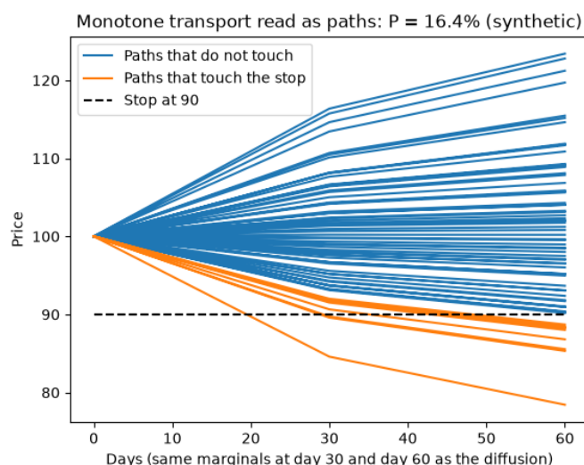
Figura 41. Las mismas marginales leídas como trayectorias del mapa monótono: la probabilidad de tocar el stop cae casi a la mitad. Las marginales no deciden cuál de las dos es la correcta.
