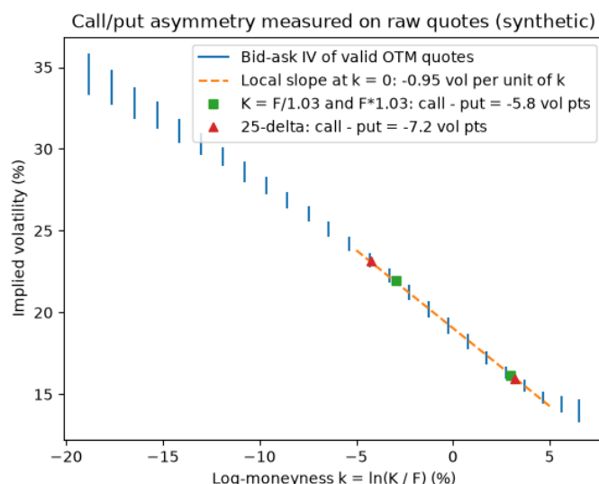
Figura 8. Volatilidades implícitas de bid y ask de las cotizaciones OTM válidas y las tres medidas de asimetría: strikes F/1.03 y 1.03 F , deltas de 25 y pendiente local. En este mundo sintético, la diferencia call menos put a distancia logarítmica simétrica es de -5.8 puntos, frente a -5.76 en la sonrisa verdadera.
