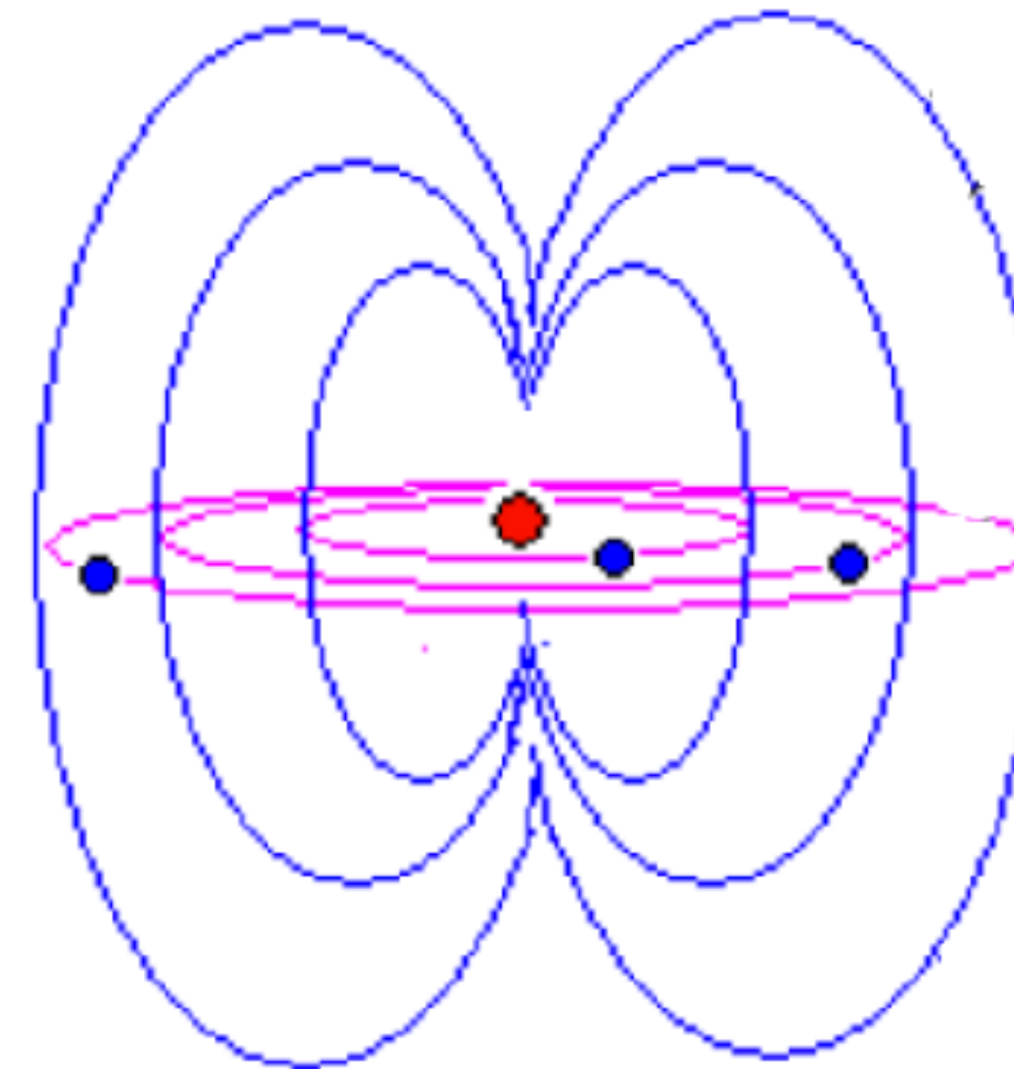
Átomo
