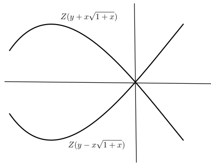
Figure 3.1: Componentes irreducibles locales de Z(y^2 - x^2 - x^3) .
