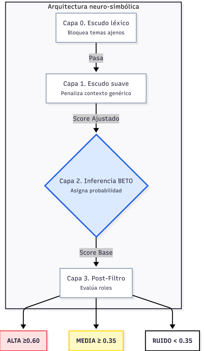
Fig. 1. Arquitectura del clasificador neuro-simbólico escalonado de cuatro capas. Las capas simbólicas (0 y 1) modulan la salida neuronal de BETO (Capa 2) mediante penalizaciones y bonificaciones aditivas antes del post-filtro (Capa 3).
