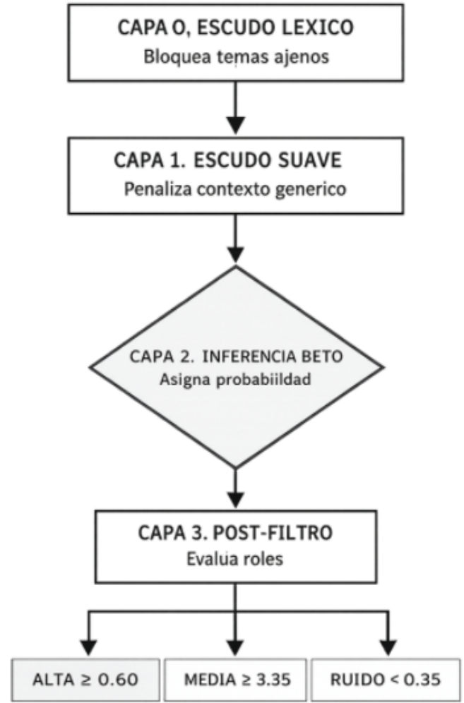
Fig. 1. Arquitectura del clasificador neuro-simbólico escalonado
