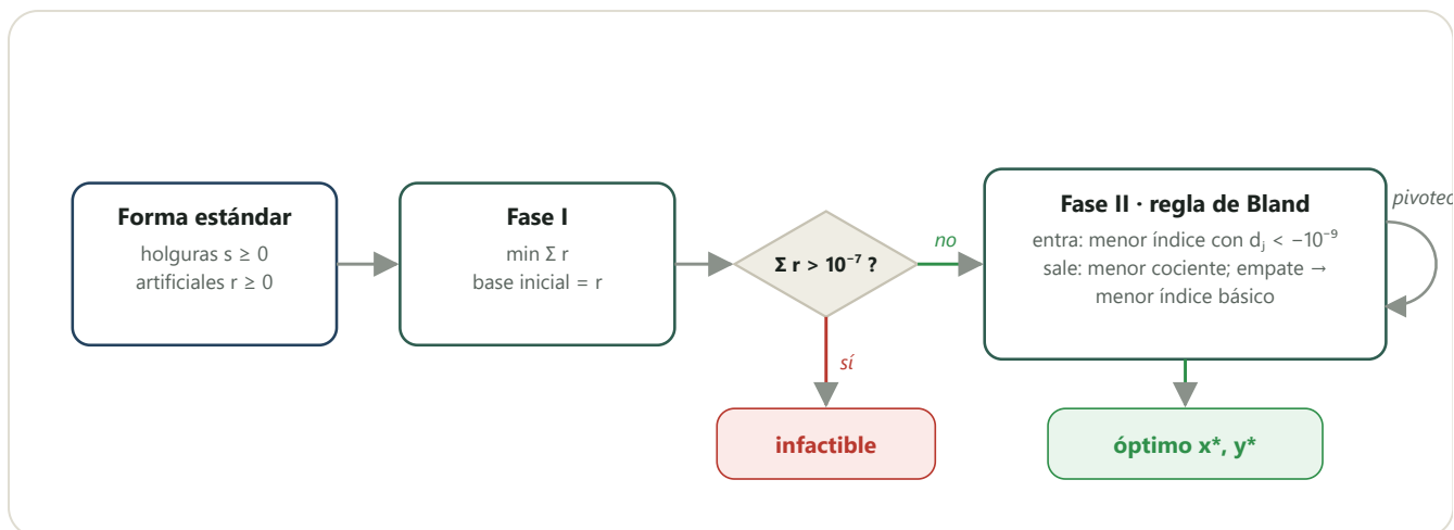
FIGURA 3 Flujo del símplex en dos fases. Las tolerancias son las del código fuente de RatioAvis 1.1.1.
