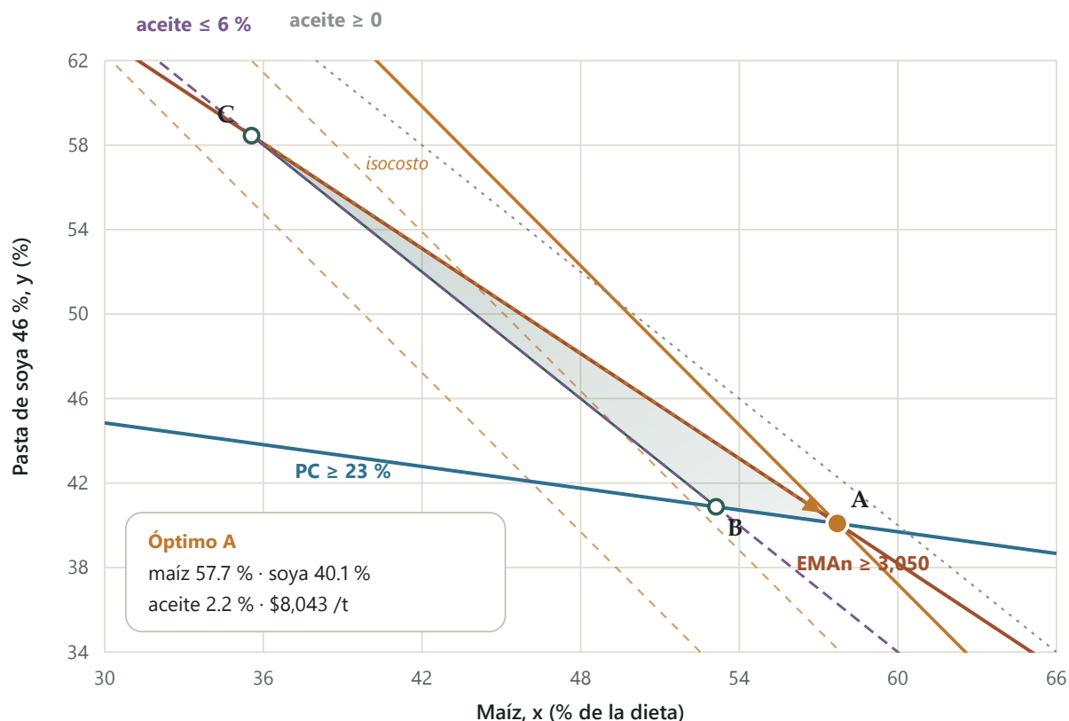
FIGURA 2 Región factible de un modelo didáctico reducido. Maíz ( x ) y pasta de soja 46 % ( y ); aceite = 100 - x - y , con un máximo de 6 %. Requisitos: proteína \geq 23\% y EMAn \geq 3,050 kcal/kg, con la matriz y los precios de la app. El simplex avanza de vértice en vértice hasta A , donde se cruzan la energía y la proteína: 57.7 % de maíz, 40.1 % de soja y 2.2 % de aceite. Es una ilustración; el caso real tiene 14 variables y 39 restricciones.
